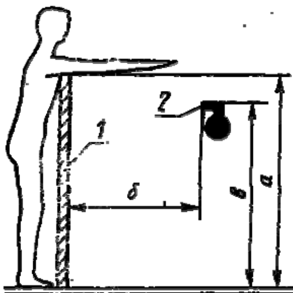
1 -ограждение; 2 -опасный элемент.
