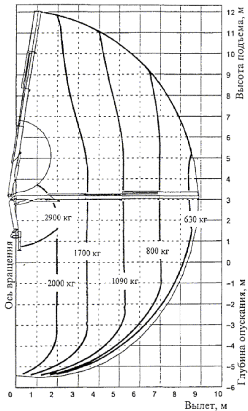
Рисунок 2 - Диаграмма грузоподъемности крана-манипулятора ПК 7000
