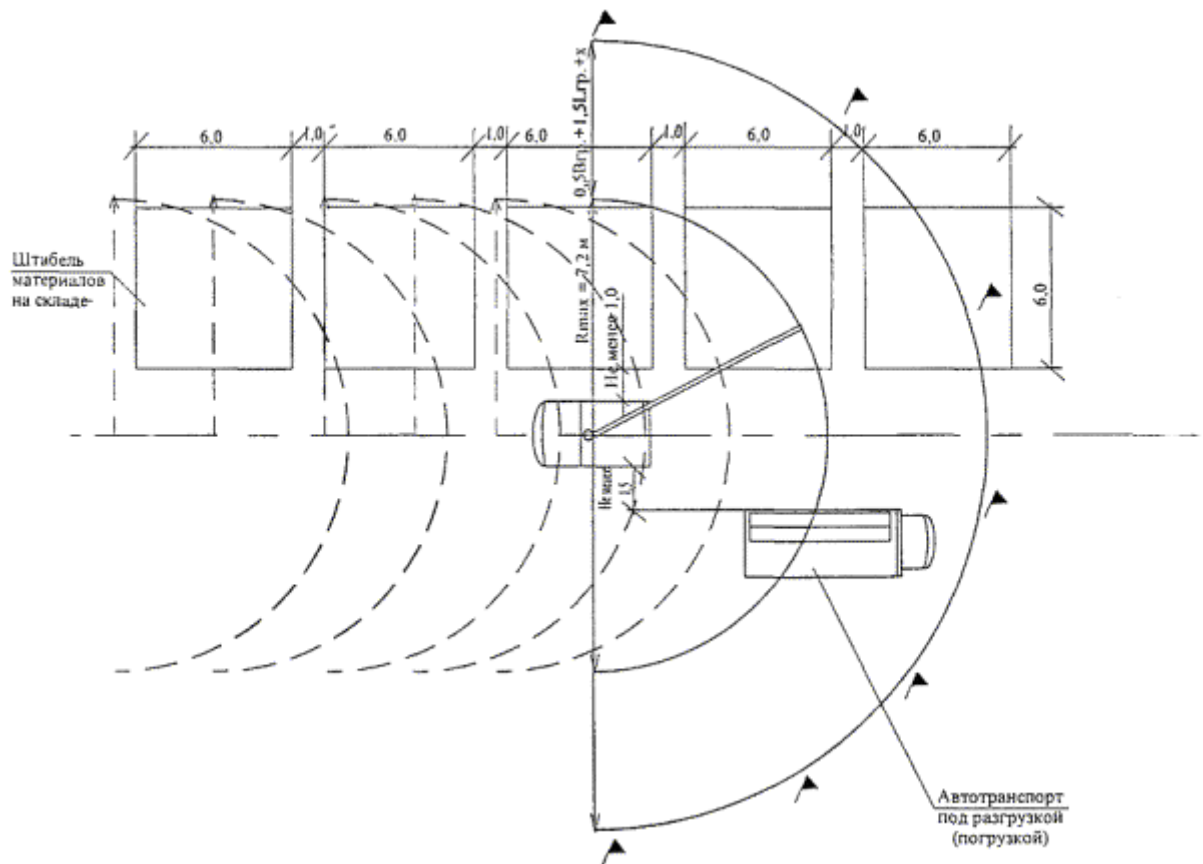
Рисунок 8 - Горизонтальная привязка крана-манипулятора ПКС 8000
