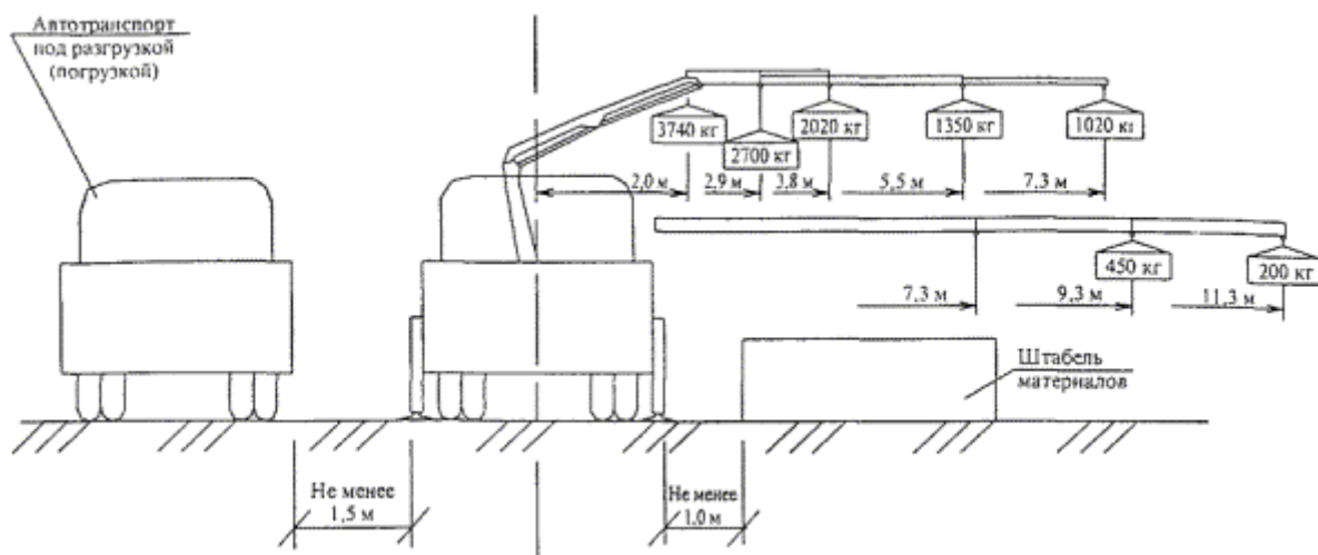
Рисунок 7 - Вертикальная привязка крана-манипулятора ПКК 8000
