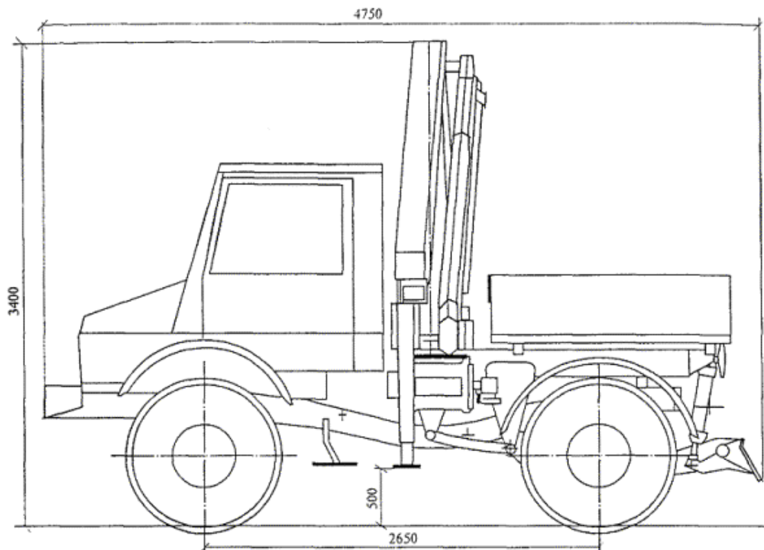
ОПОРНЫЙ КОНТУР
