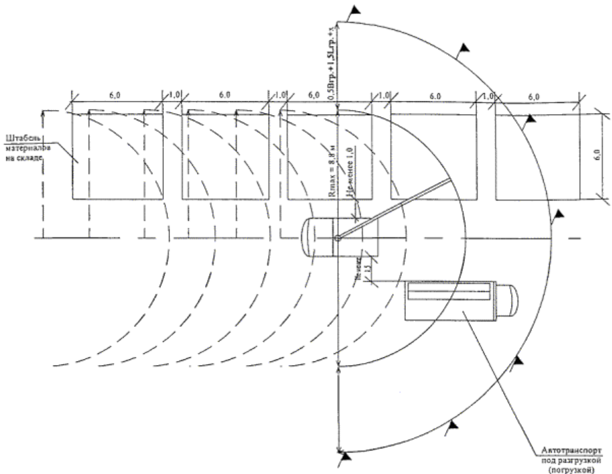
Рисунок 4 - Горизонтальная привязка крана-манипулятора ПК 7000
