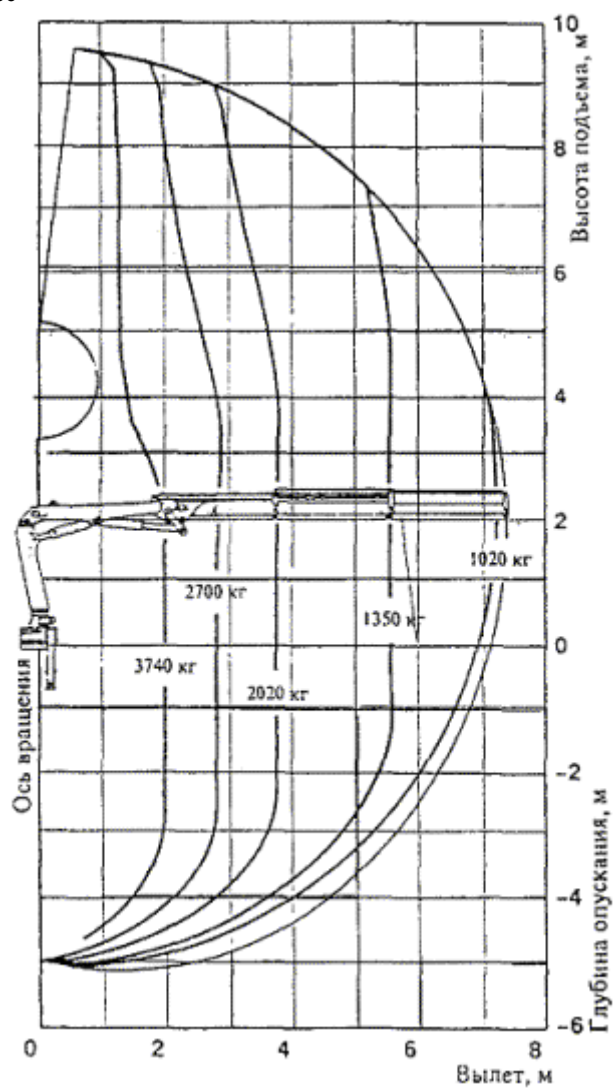
Рисунок 6 - Диаграмма грузоподъемности крана-манипулятора ПКК 8000
