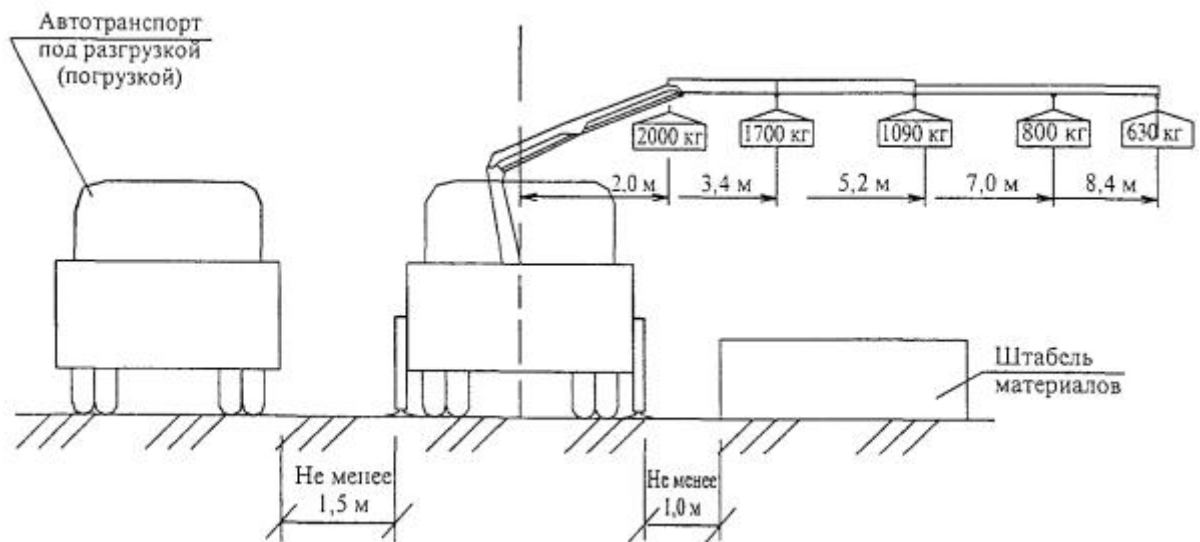
Рисунок 3 - Вертикальная привязка крана-манипулятора ПК 7000
