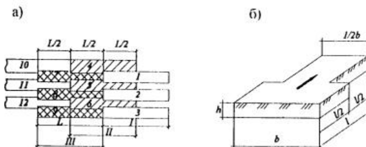
Рис. 3.8.2. Ребристо-шахматная схема резания грунта скрепером:
