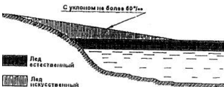
Рис. 16.1.1. Намораживание съездов
