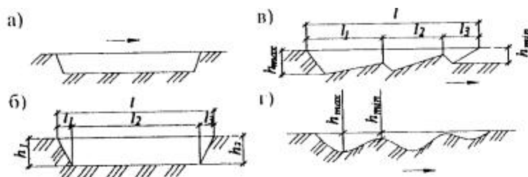
Рис. 3.8.1. Способы резания грунтов скрепером (стрелкой показано направление движения скрепера):
