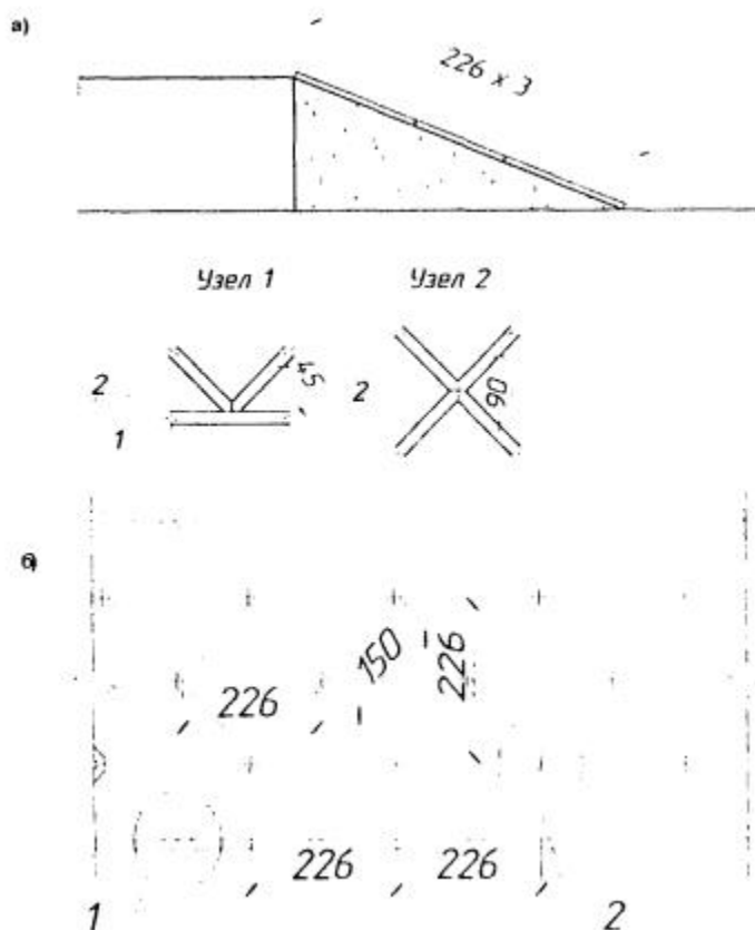
Рис. 5.2.2. Решетчатая конструкция с диагональным расположением элементов:
