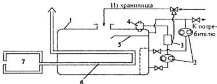
Рис. 7.3.4. Битумоплавильный агрегат непрерывного действия:
