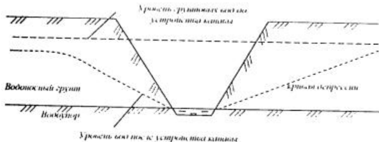
Рис. 2.2.1. Дренажная канавка
