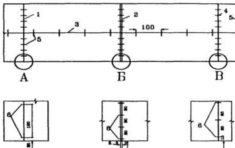
Рис. 8.6.3. Схема расположения штырей в деформационных швах:
