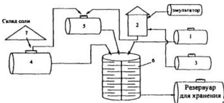
Рис. 7.3.6. Технология приготовления прямой высококонцентрированной эмульсии: 1 -обезвоженный и нагретый до 150-170°C битум; 2 - котёл для варки мыла, 3 - ёмкость для едкого натра; 4 - ёмкость для воды; 5 - ёмкость для раствора эмульгатора; 6 - мешалка; 7 - склад соли
