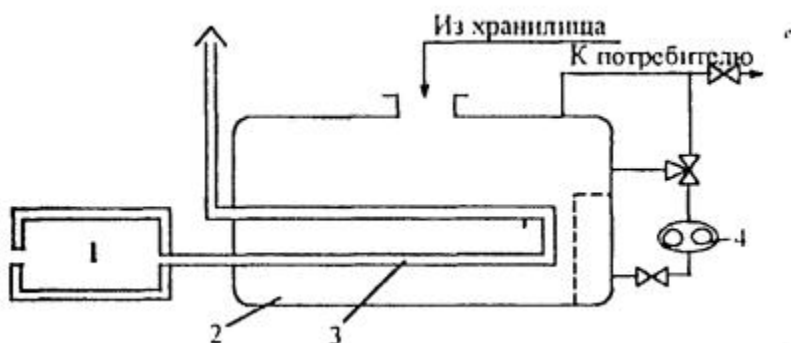
Рис. 7.3.3. Битумоплавильный агрегат циклического действия:
