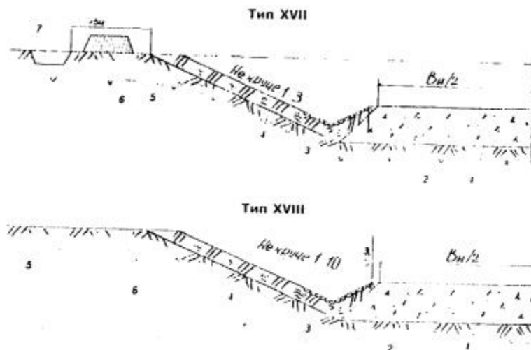
Рис. 4.4.10. Поперечные профили выемок в слабодонасыщенных грунтах: 1 - щебень или гравий; 2 - глинистый грунт; 3 - каменное мощение; 4 - теплоизоляция из мха по расчету; 5 - ВГВМ до устройства выемки, 6 - ВГВМ после устройства выемки; 7 - водоотводная канава
