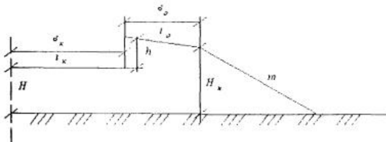
Рис. 3.3.2. Схема разбивки земельного полотна при устройстве дорожной одежды в корыте
