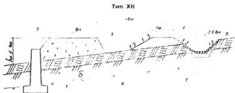
Рис. 4.4.7. Поперечный профиль насыпи на косогоре крутизной более 1:5: 1 - подпорная стенка; 2 - несцементированный обломочный грунт; 3 - мохорастительный покров; 4 - мерзлотный валик; 5 - каменное мощение; 6 - ВГВМ до постройки насыпи; 7 - ВГВМ после постройки насыпи
