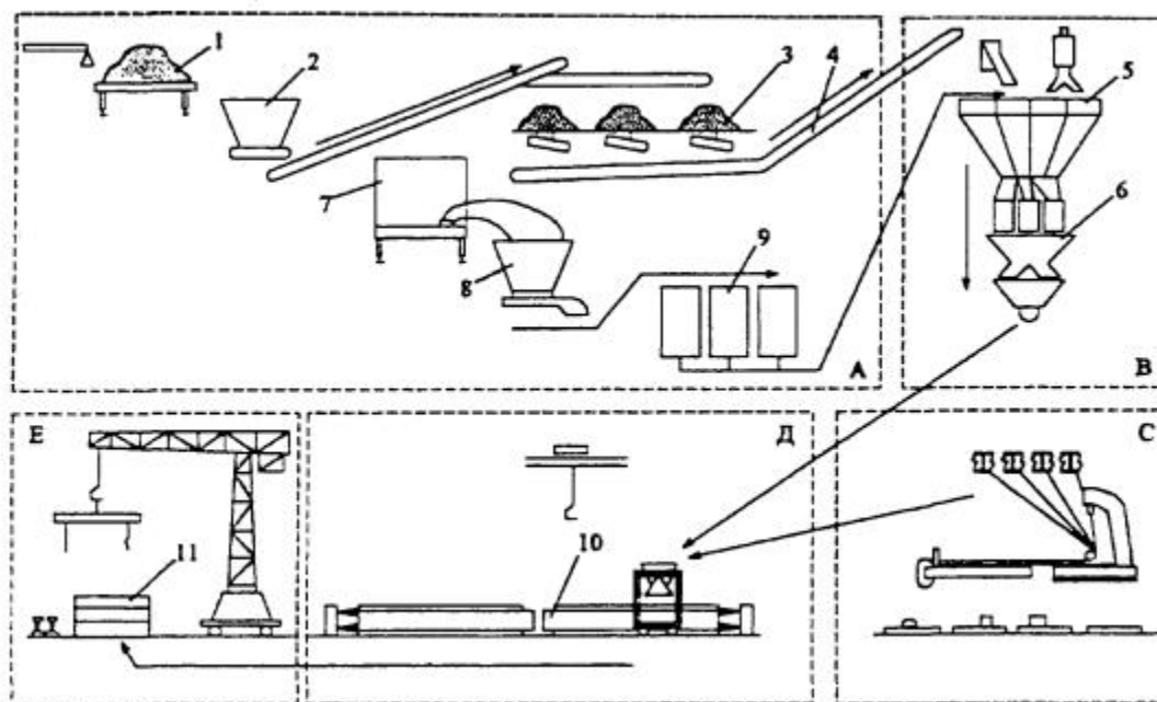
Рис. 7.6.3. Технологическая схема изготовления конструкций на стендах:
