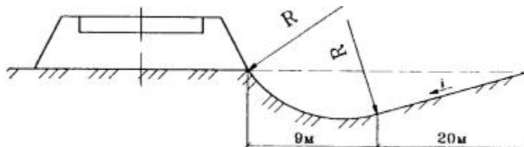
Рис. 9.6.1. Поперечное сечение рекультивированного притрассового бокового резерва
