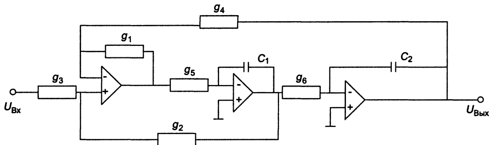
Рис. 3.4. Фильтр нижних частот
