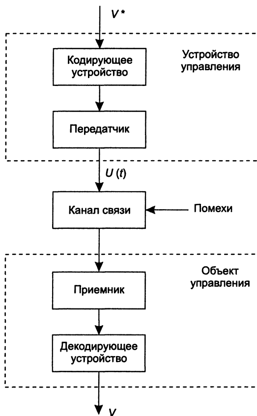
Рис. 1.4. Система радиосвязи
