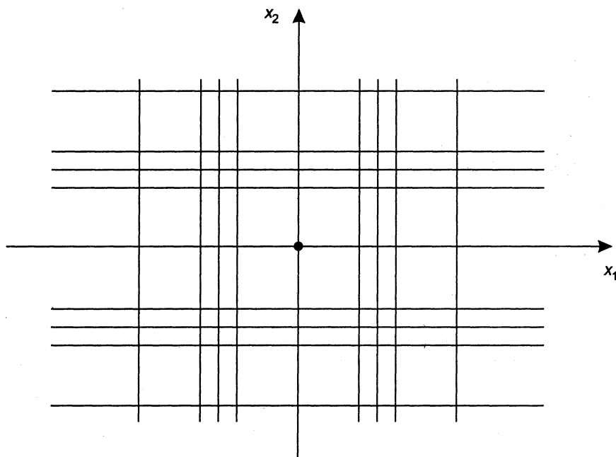
Рис. 4.2. Представление плоскости R^2 в памяти компьютера
