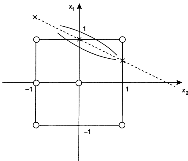
Рис. 6.1. План эксперимента
