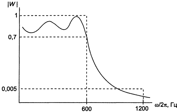
Рис. 7.4. Характеристика НЧ-фильтра
