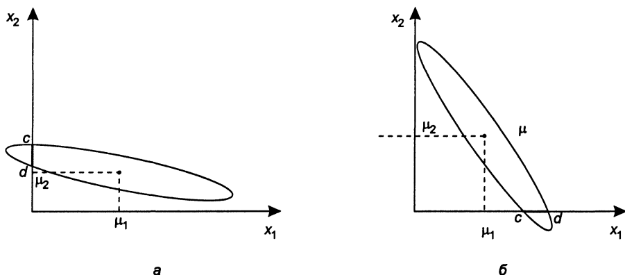
Рис. 6.2. Исключение переменных:
