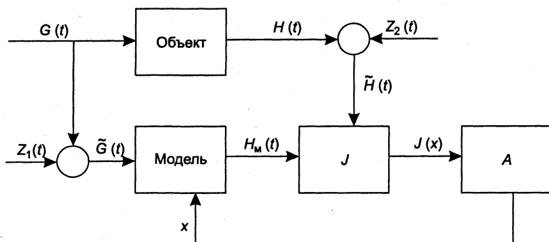
Рис. 1.10. Схема идентификации стохастического объекта
