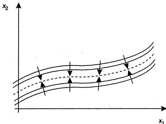
Рис. 3.1. Явление овражности
