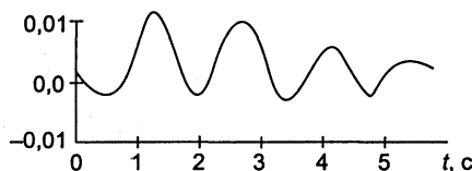
Рис. 7.3. График зависимости \omega_*(t) - \omega(x^*, t)
