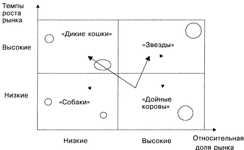
Рис. 4.11. Матрица БКГ
