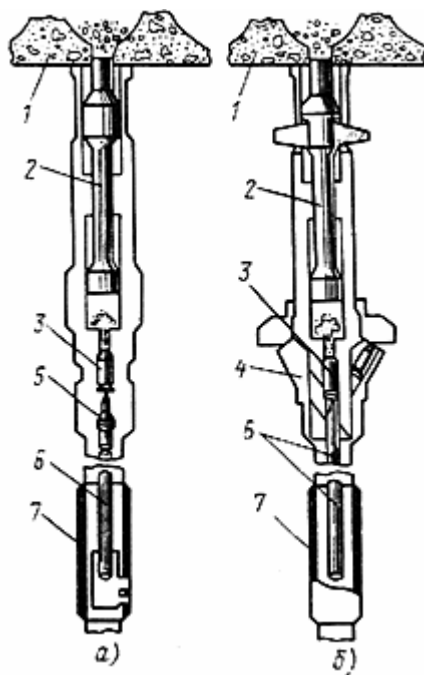
Рис. 5. Выполнение отверстий ударными колонками УК-6 (а) и УKM (б): 1 - многопустотная панель потолочного перекрытия; 2 - пробойник; 3 - патрон; 4 - боек; 5 - ударник; 6 - муфта; 7 - барабан с патронами
