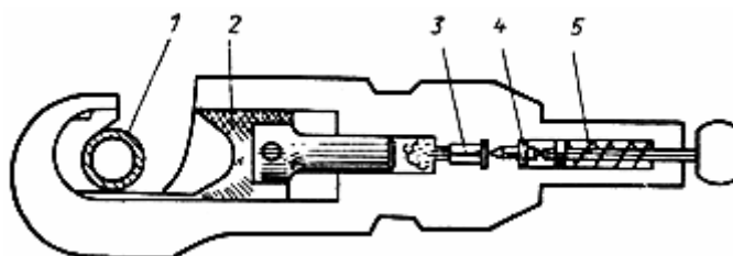
Рис. 7. Резка стальной трубы прессом ПРТ:
