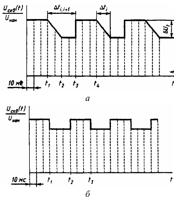
Рисунок Б.1. Колебания напряжения произвольной формы (а) и имеющие форму меандра (б)
