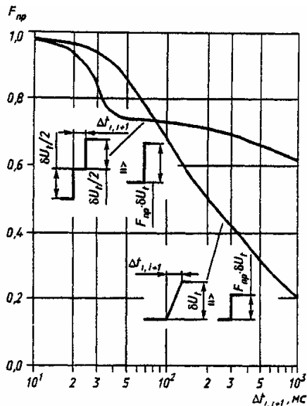
Рисунок В.1. Коэффициент приведения F_{пр} для периодических колебаний напряжения, имеющих двухступенчатую и пилообразную форму
