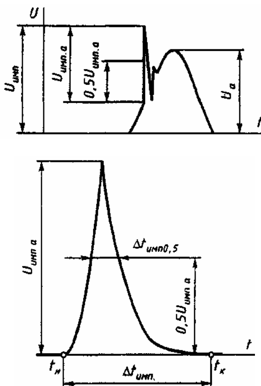
Рисунок Б.3. Параметры импульсного напряжения
