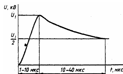
Рисунок Д.4. Форма грозовых импульсов, характерная для точек присоединения б, е, ж на рисунке Д.1
