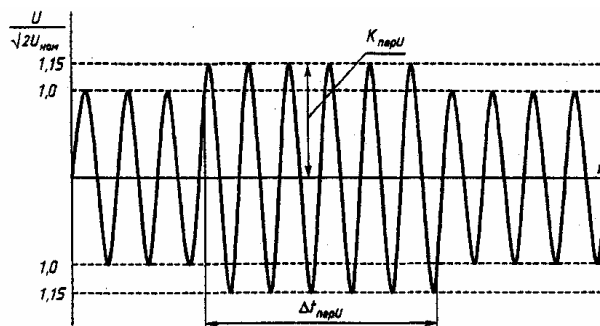
Рисунок Б.4. Временное перенапряжение
