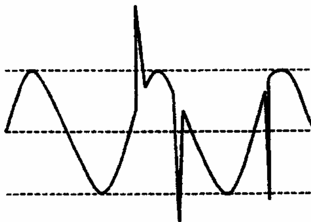
Рисунок А.3. Импульсы напряжения
