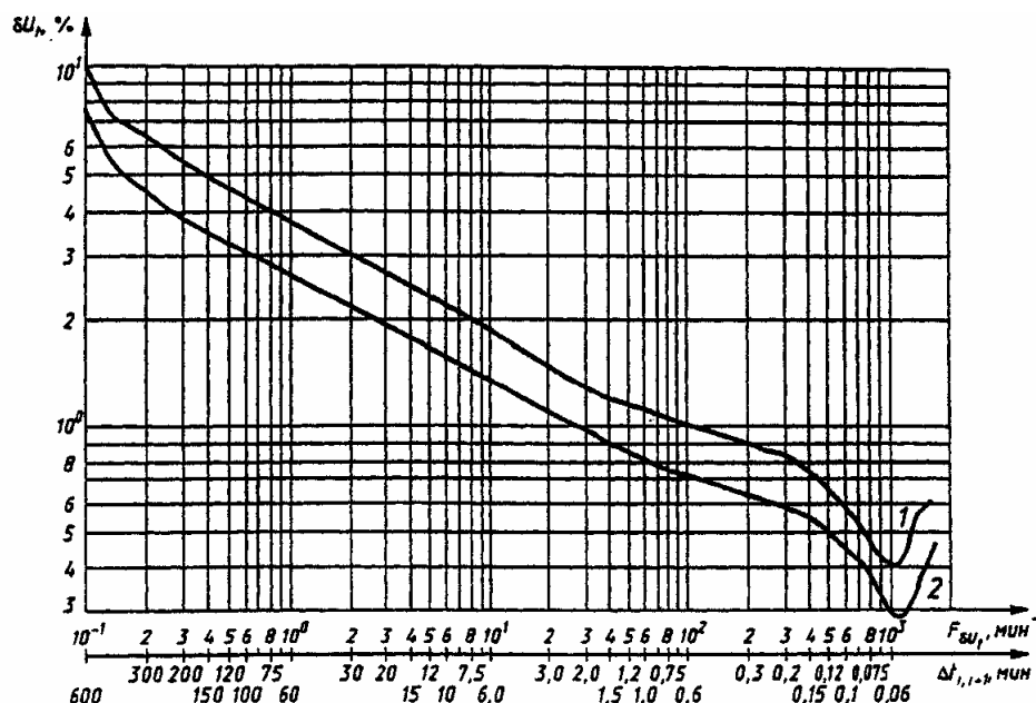
Рисунок 1. Предельно допускаемые размахи изменения напряжения в зависимости от частоты повторения изменений напряжения за минуту для колебаний напряжения, имеющих форму меандра
