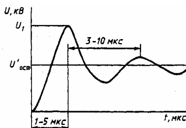
Рисунок Д.3. Форма грозовых импульсов, характерная для точек присоединения, проходящих через выводы силового трансформатора, рассматриваемая обмотка которого имеет связь с ВЛ (точки присоединения з, з', и на рисунке Д.1)
