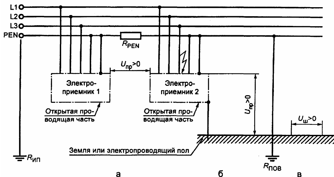
Рисунок В.3 — Сеть TN-C с однофазным замыканием на корпус Здесь и на следующих рисунках уравнивание и выравнивание потенциалов отсутствуют
