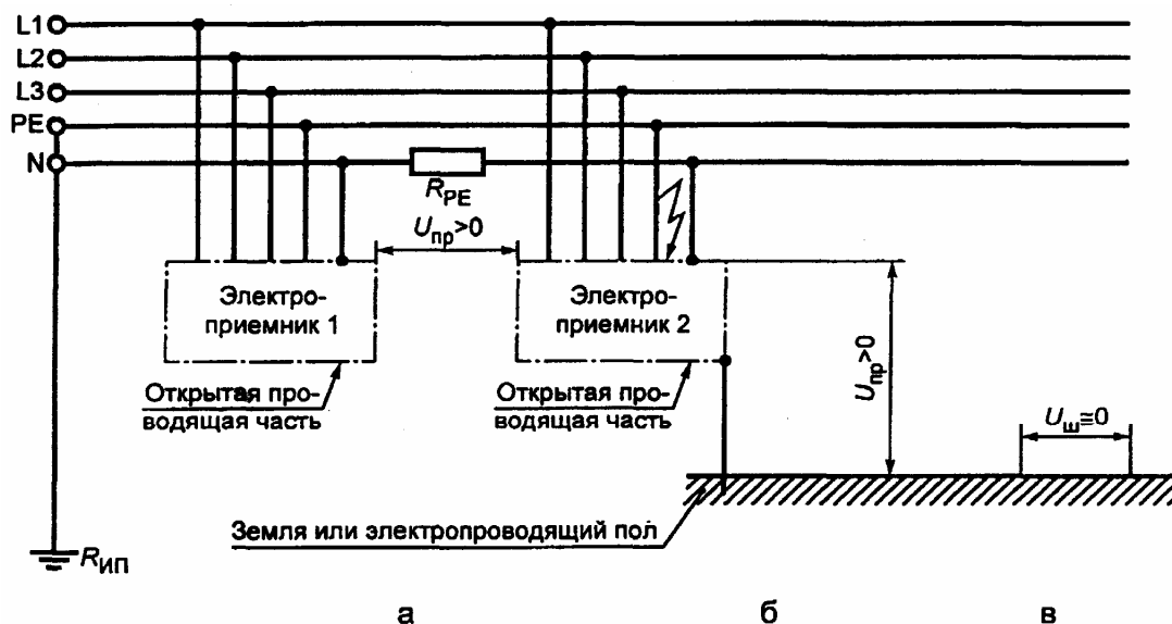
Рисунок В.6 — Сеть TN-S с однофазным замыканием на корпус
