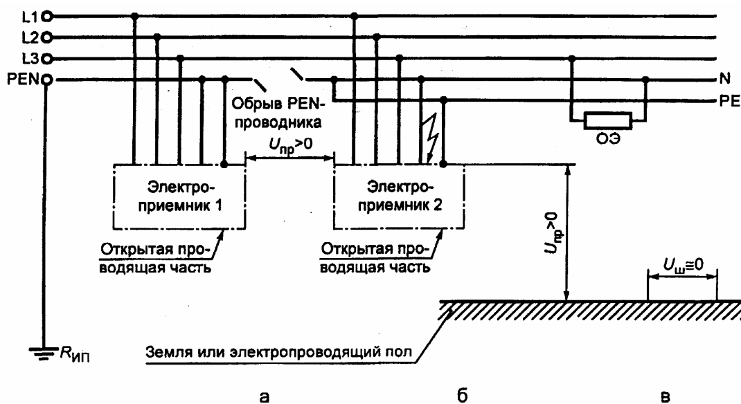
Рисунок В.7 — Сеть TN-C-S с обрывом PEN-проводника
