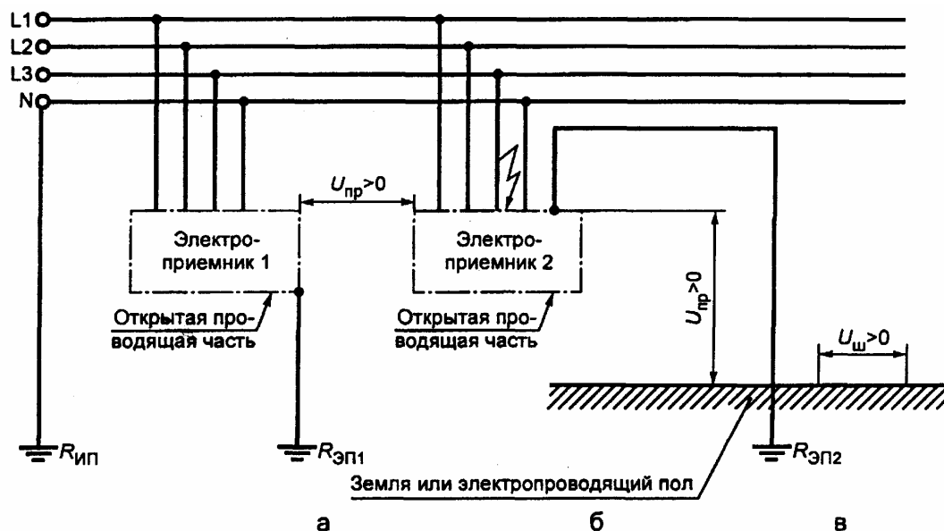
Рисунок В.10 — Сеть ТТ с нулевым рабочим проводником с однофазным замыканием на корпус
