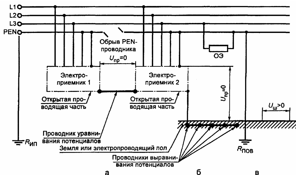
Рисунок В.2 — Сеть TN-C с оборванным PEN-проводником Имеется уравнивание потенциалов на участке а), выравнивание потенциалов на участке б). На участке в) выравнивание потенциалов отсутствует
