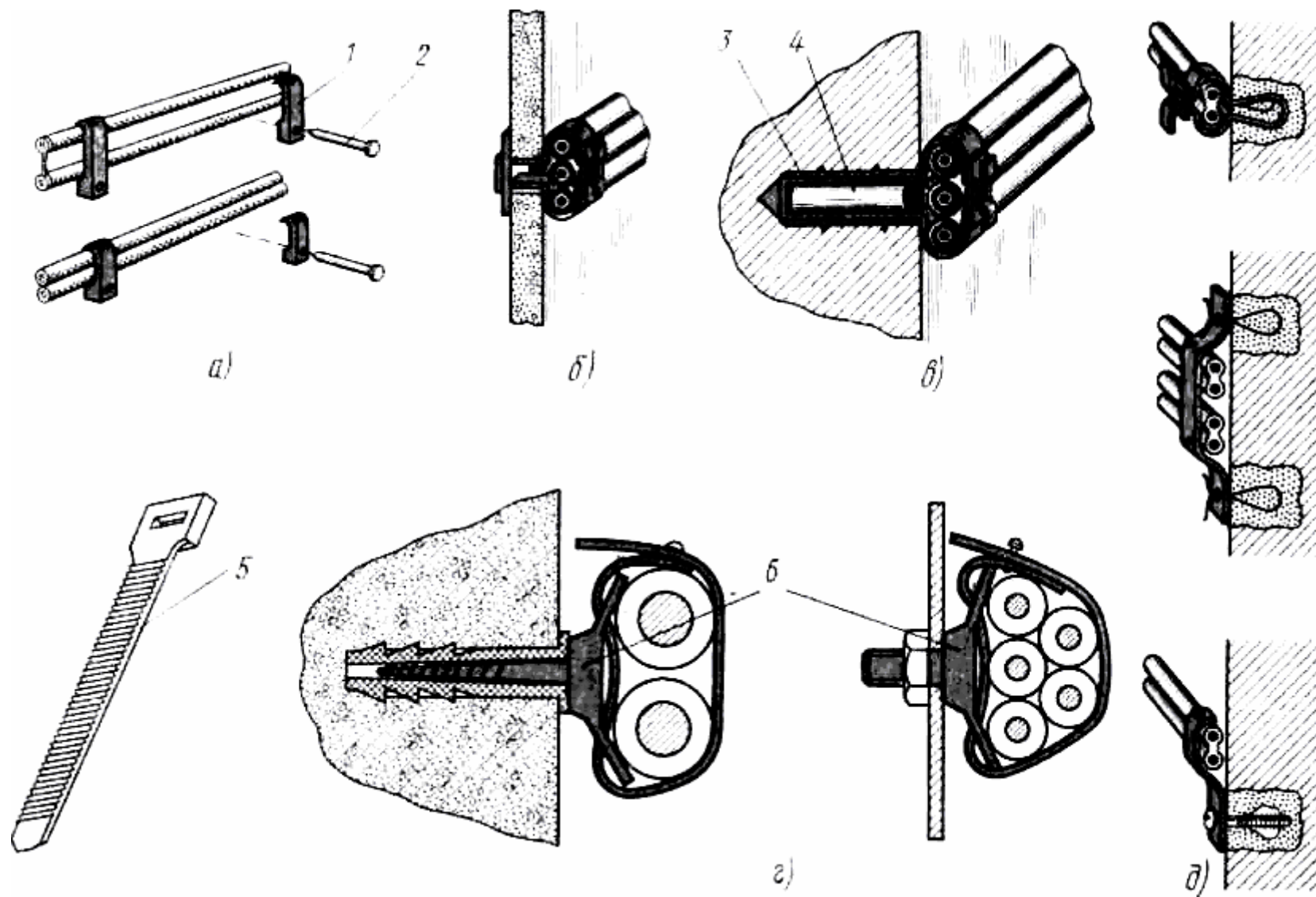
Рис.14. Способы крепления проводов к строительным конструкциям:
