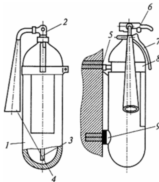
Рис.26. Ручной углекислотный огнетушитель ОУ-5 (ОУ-8):
