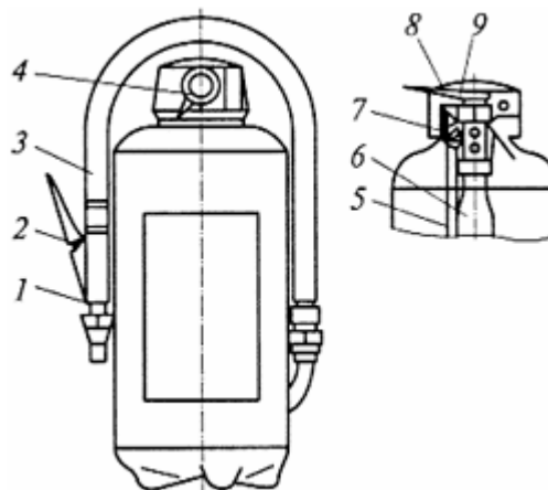
Рис.28. Ручной порошковый огнетушитель ОП-5:
