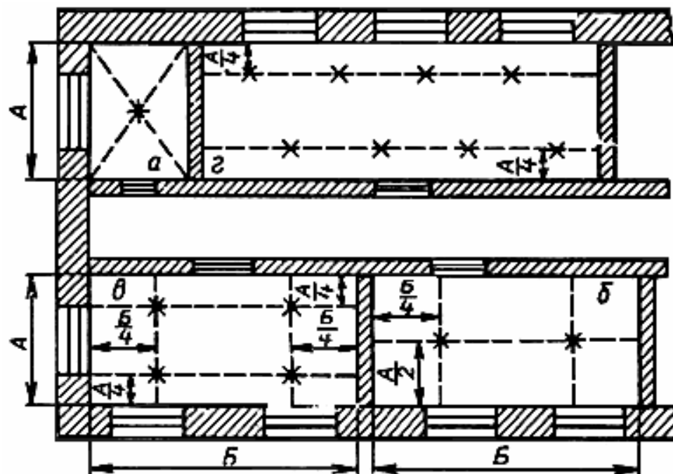
Рис.20. Разметка мест установки светильников в помещениях
