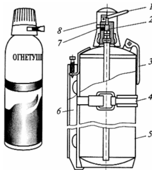
Рис.27. Хладоновый огнетушитель ОУБ-ЗА (ОУБ-7А):
