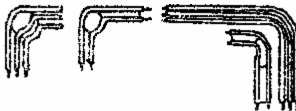
Рис.19. Изгибание проводов
