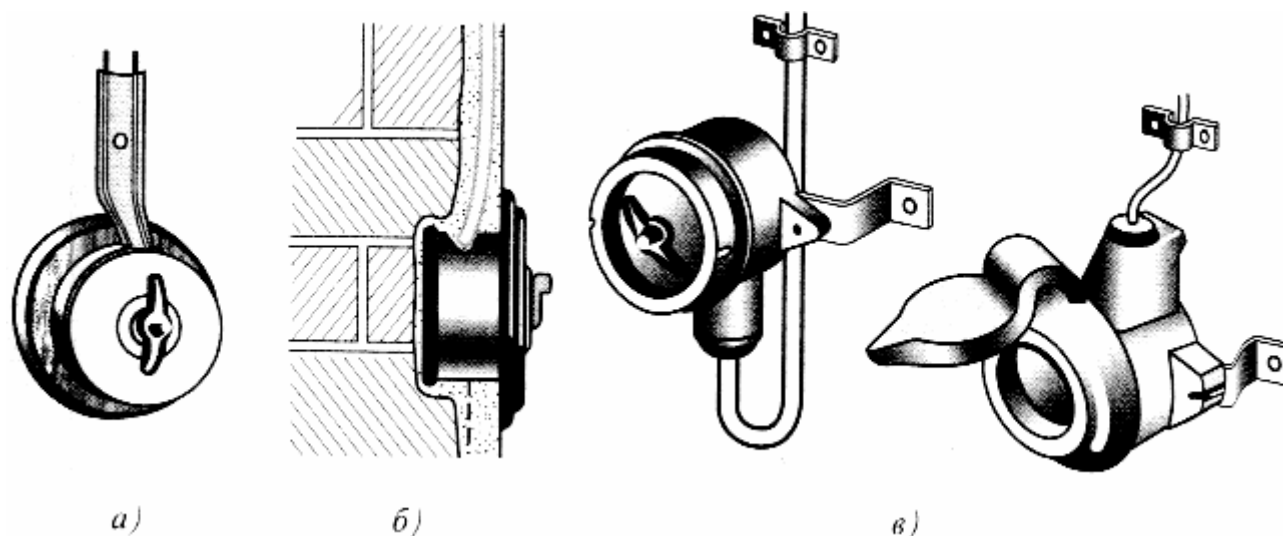
Рис.15. Примеры монтажа установочных приборов:
