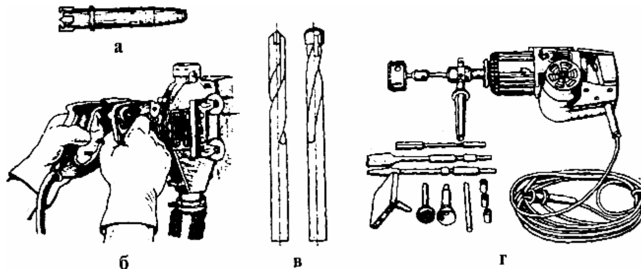
Рис.10. Инструмент, механизмы и приспособления для пробивных работ:
