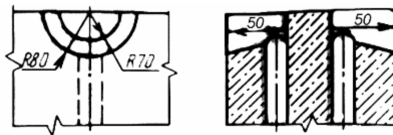
Рис.7. Протяжные ниши в стеновых железобетонных межквартирных панелях
