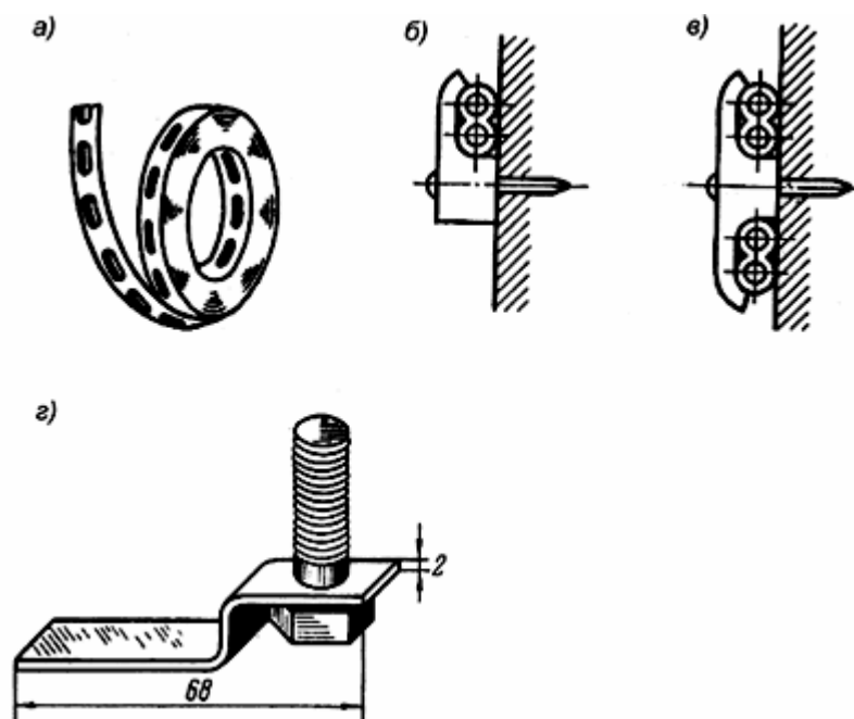
Рис. 6. Крепежные детали и электроустановочные изделия
