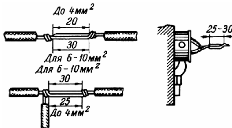
Рис.8. Соединение и ответвление алюминиевых однопроволочных жил пайкой
