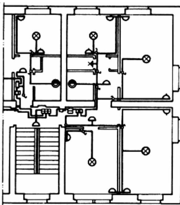
Рис. 1. Схема открытой электропроводки в квартире
