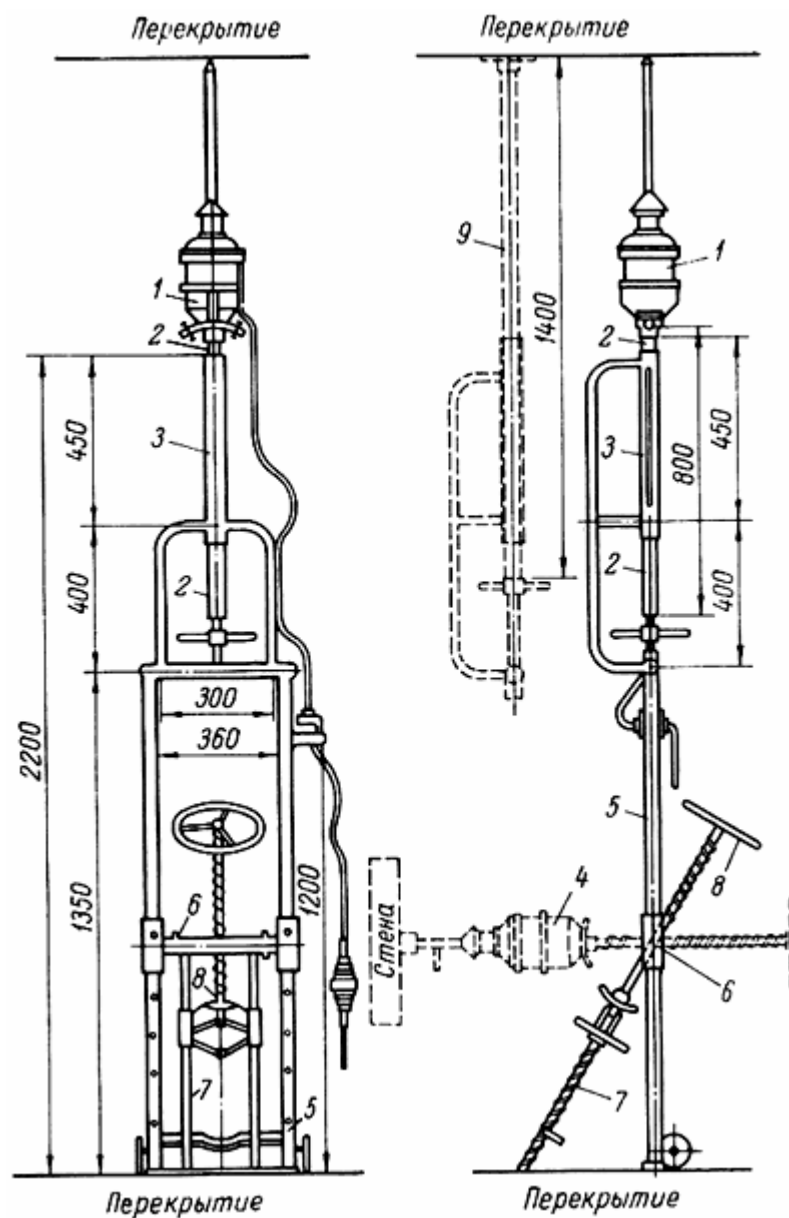
Рис. 2. Станок-стойка для сверления отверстий в полах, потолках и стенах
