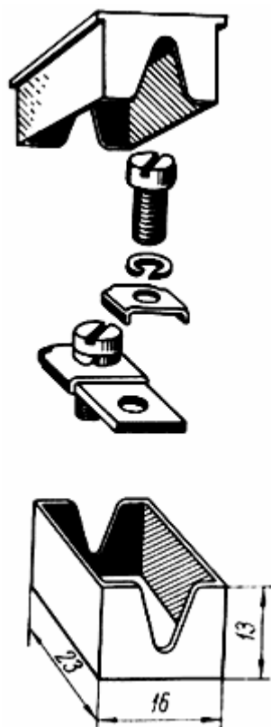
Рис. 11. Люстровый зажим в корпусе
