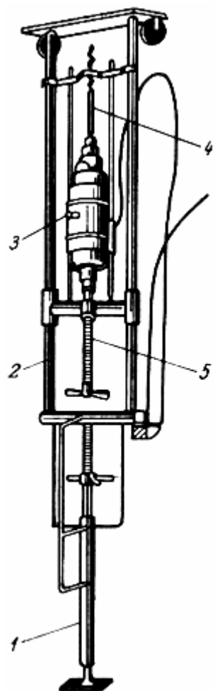
Рис. 3. Устройство для создания давления на сверло при сверлении отверстий в стенах и перекрытиях
