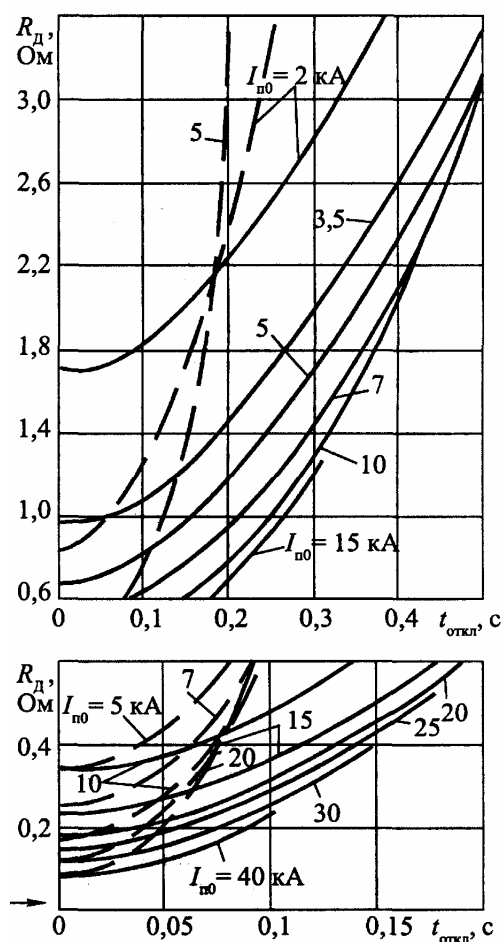
Рис. 5.19. Зависимость R_{\text{д}} = f(t_{\text{откл}}, I_{\text{п0}}) при КЗ на воздушных линиях 35 кВ (сплошные кривые) и 10 кВ (пунктирные кривые)
