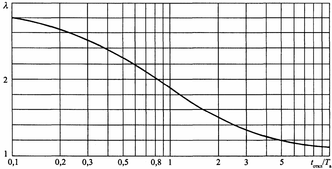
Рис. 7.10. Зависимость коэффициента приведения электродинамической нагрузки \lambda от t_{\text{откл}}/T_a
