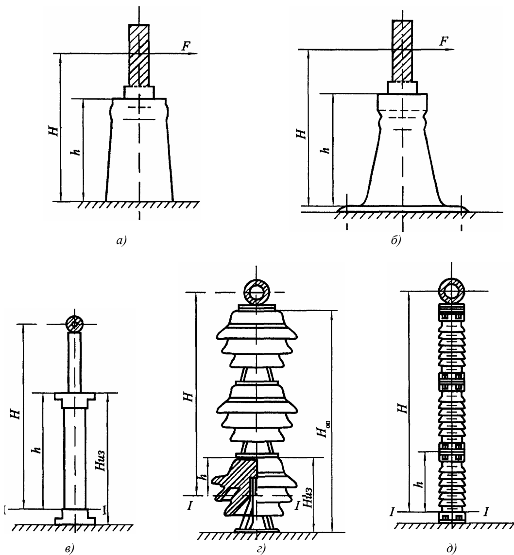
Рис. 7.1. К определению допустимых нагрузок на изоляторы и шинные опоры
