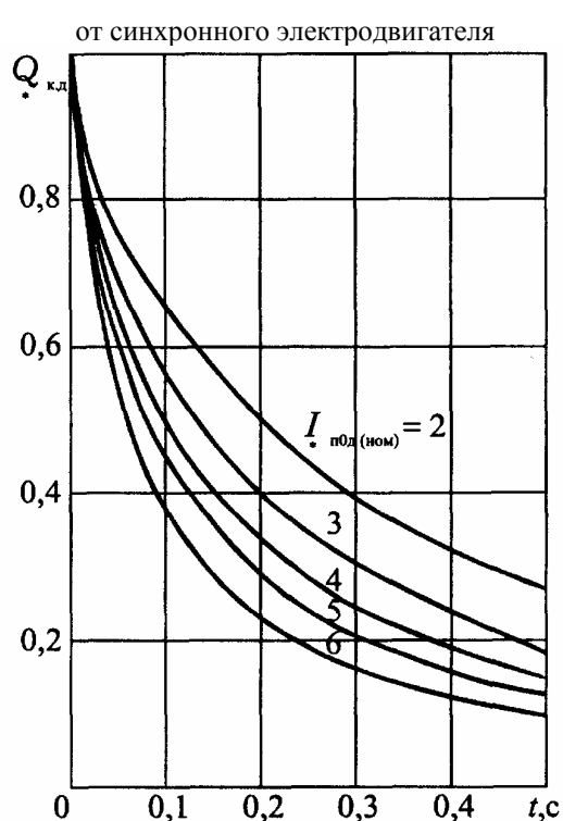
Рис. 8.5. Кривые для определения Q_{* \text{ к.д.}}
