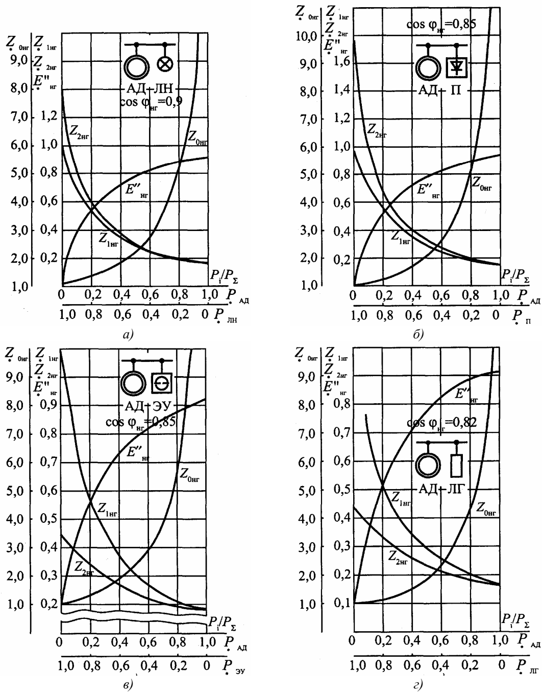
Рис. 6.5. Зависимость параметров комплексной нагрузки Z_{1нг} , Z_{2нг} , Z_{0нг} , E_{нг} от ее состава
