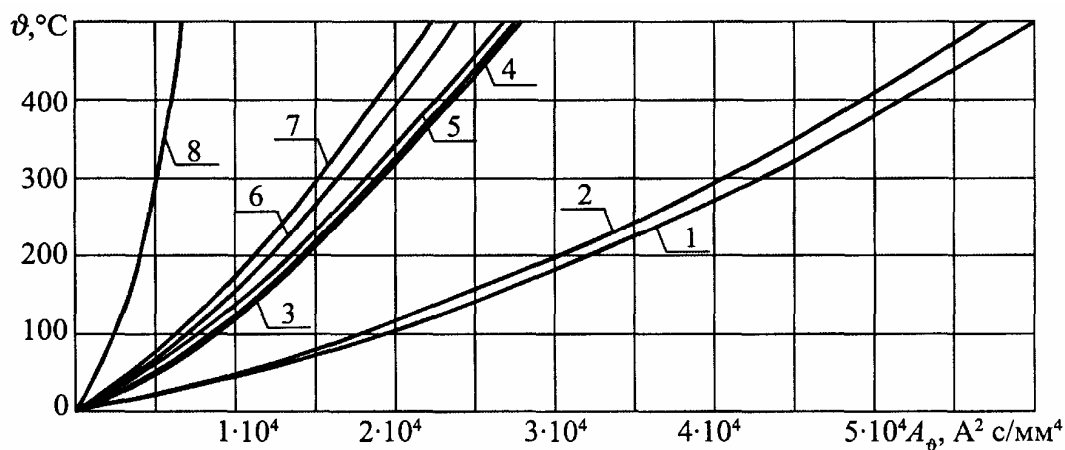
Рис. 8.8. Кривые для определения температуры нагрева проводников из различных
