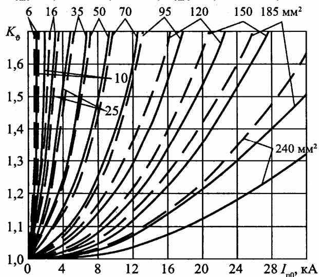
Рис. 6.10. Зависимости коэффициента увеличения активного сопротивления кабелей различных сечений с медными жилами от тока дугового устойчивого КЗ с учетом теплоотдачи при продолжительностях КЗ 0,2 с (сплошные кривые) и 0,6 с (пунктирные кривые)
