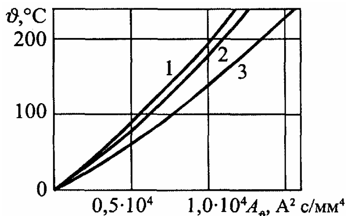
Рис. 8.9. Кривые для определения температуры нагрева проводов при коротких замыканиях Материалы проводов: 1 - сплавы АЖ и АЖКП; 2 - сплавы АН и АНКП; 3 - алюминий марок А, АКП, АПКП и сталеалюминий марок АС, АСКП, АСКС, АСК, АПС, АПСКС, АПСК
