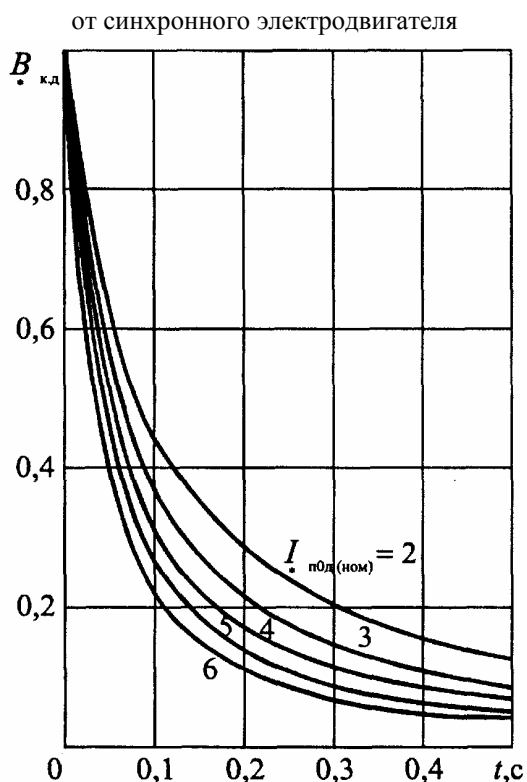
Рис. 8.6. Кривые для определения B_{* \text{ к.д.}}
