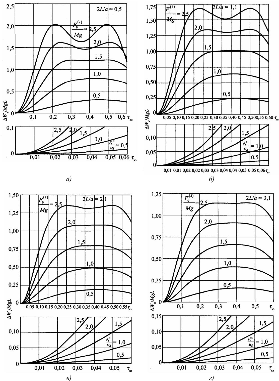
Рис. 7.11. Характеристики \Delta W_k / MgL при двухфазном КЗ
