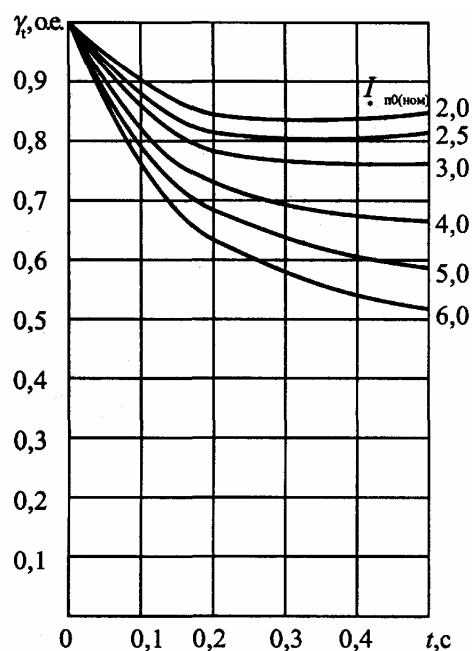
Рис. 5.3. Типовые кривые изменения периодической составляющей тока КЗ от турбогенераторов с диодной независимой (высокочастотной) системой возбуждения
