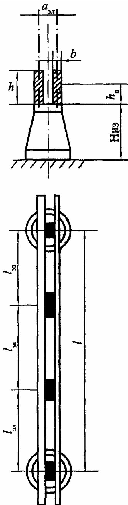
Рис. 7.4. Двухполосная шина
