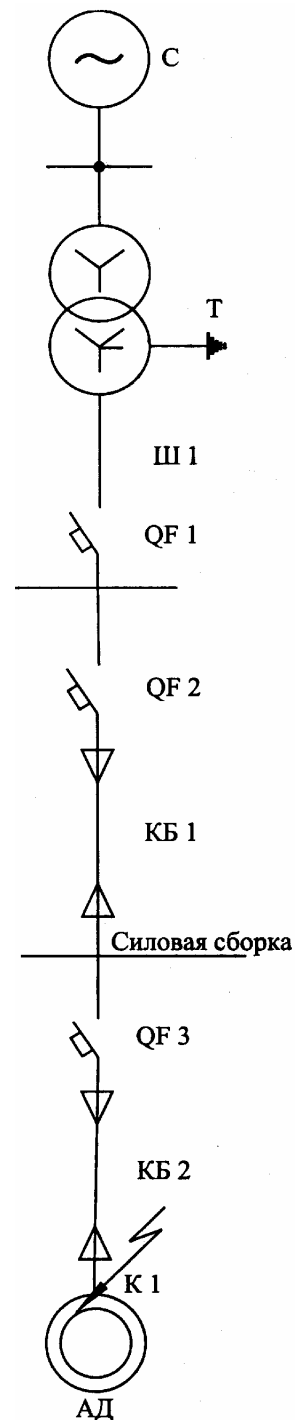
Рис. 6.12. Расчетная схема к примеру 6.11.1
