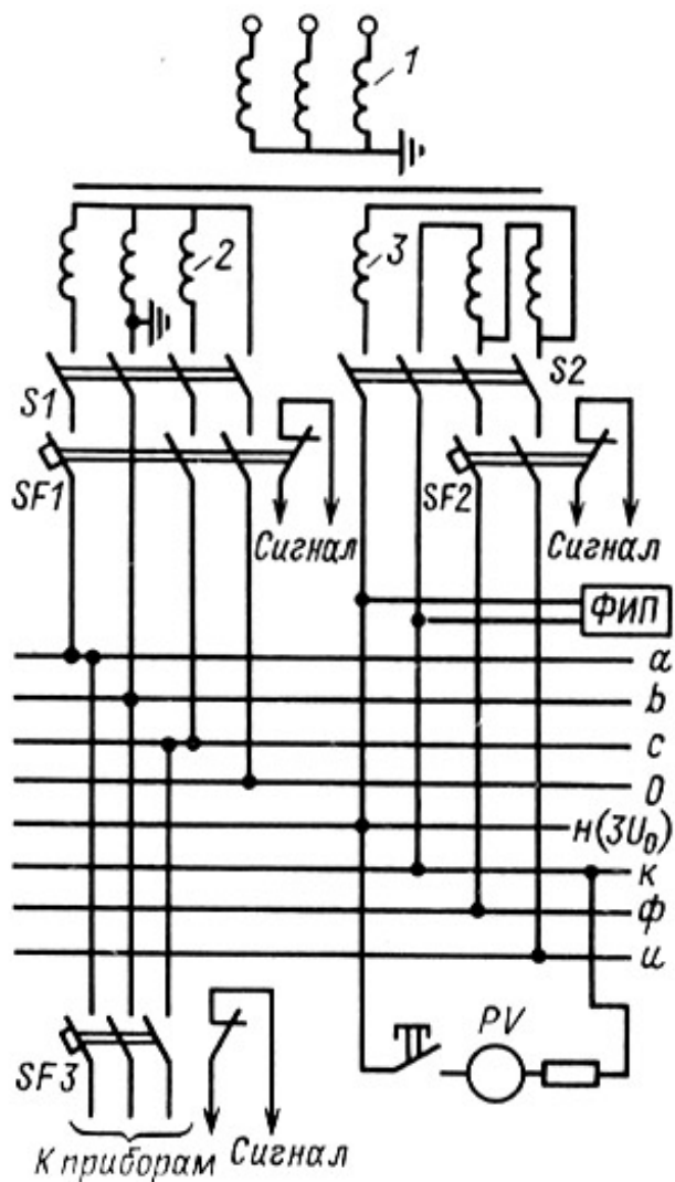
Рис. 4.5. Схема включения трансформаторов напряжения типа НКФ на 110-330 кВ:
