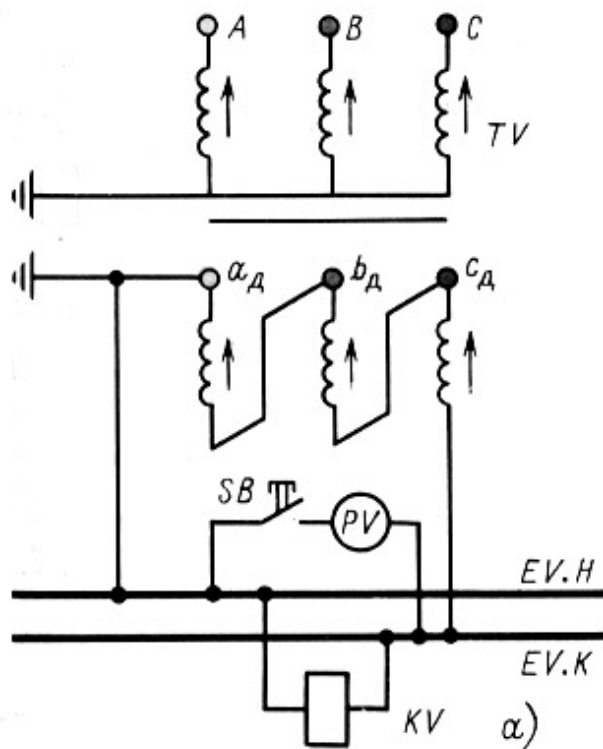
Рис. 7.12. Соединение однофазных трансформаторов напряжения в фильтр напряжения нулевой последовательности:
