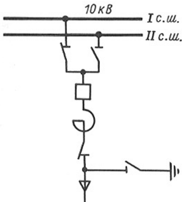
Рис. 9.2. Схема присоединения линии 10 кВ
