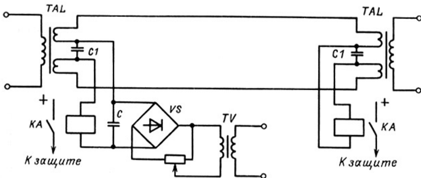
Рис. 7.20. Упрощенная схема контроля исправности соединительных проводов дифференциальной токовой защиты линии
