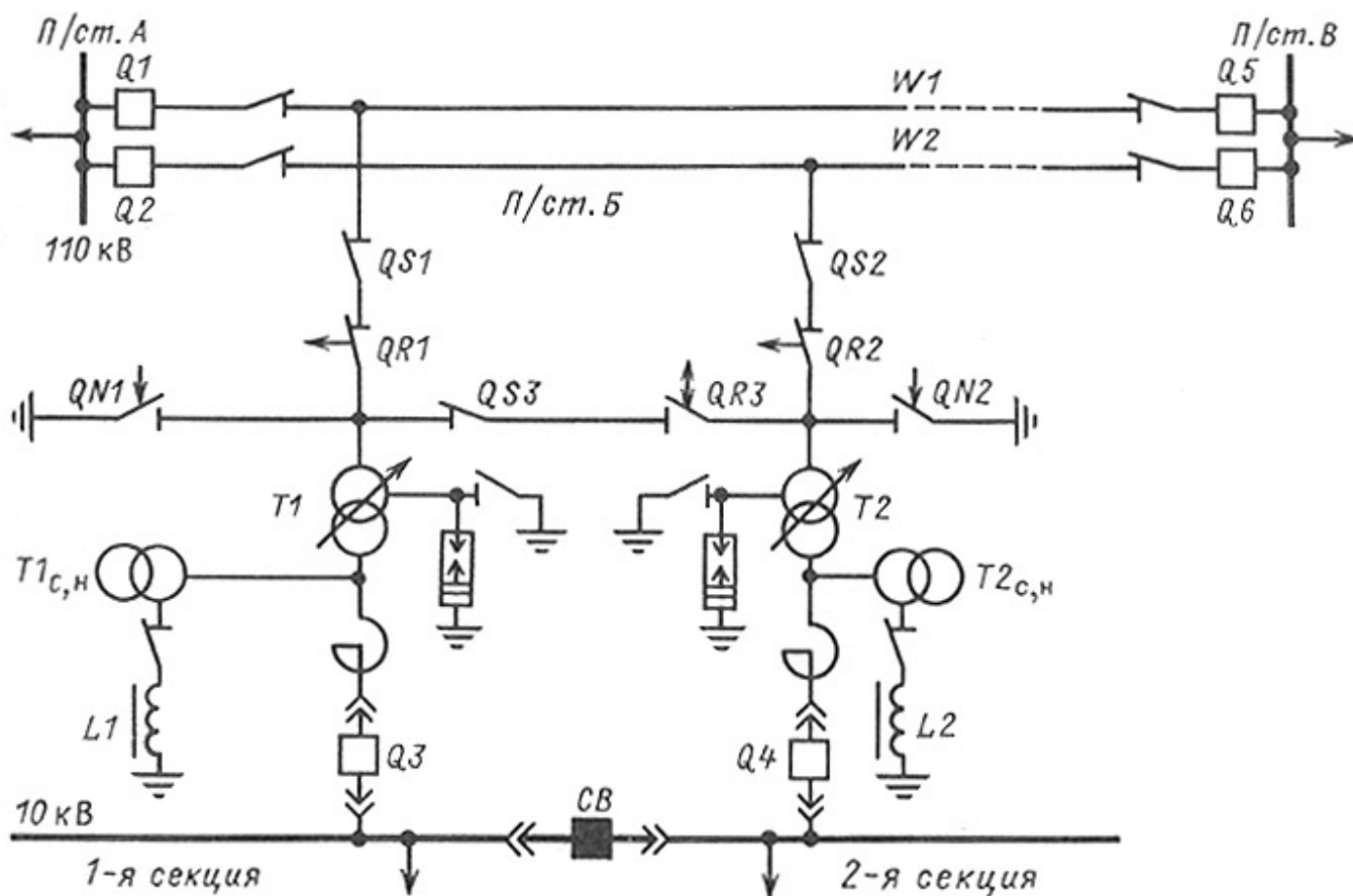
Рис. 9.5. Схема двух блоков с отделителями и неавтоматической перемычкой со стороны линий
