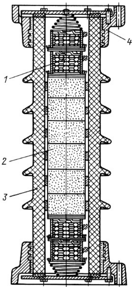
Рис. 4.11. Вентильный разрядник типа РВС-15:
