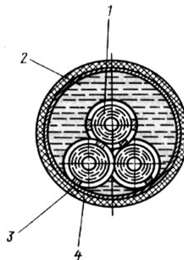
Рис. 4.14. Расположение кабелей высокого давления в стальном трубопроводе:
