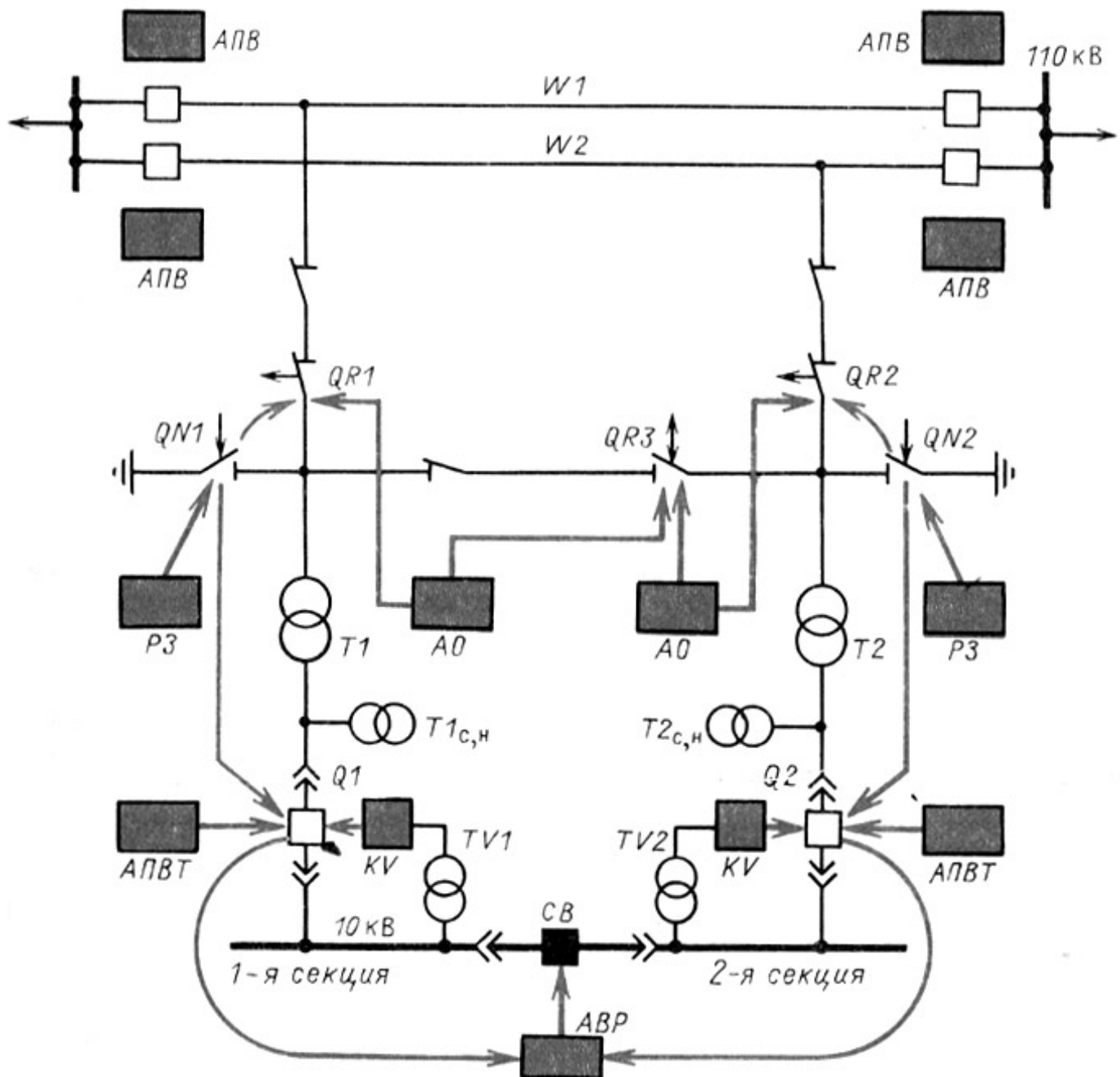
Рис. 7.30. Структурная схема автоматики двухтрансформаторной подстанции на отделителях и с короткозамыкателями
