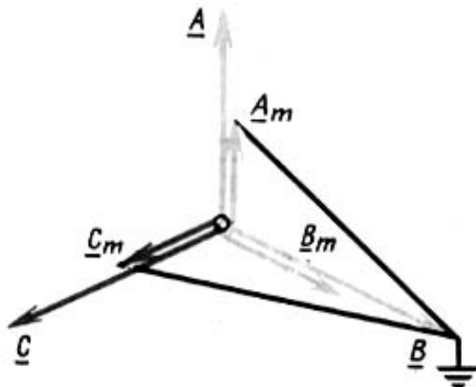
Рис. 1.3. Векторная диаграмма напряжения участка сети, питающегося от автотрансформатора с разземленной нейтралью при замыкании фазы на землю.
