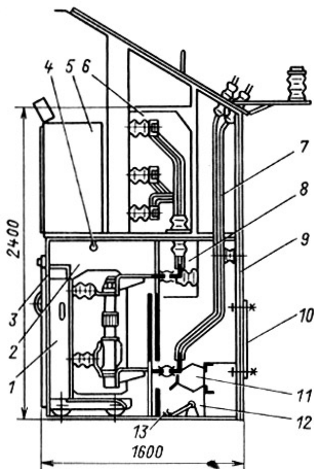
Рис. 5.5. Шкаф КРУН серии К-37:
