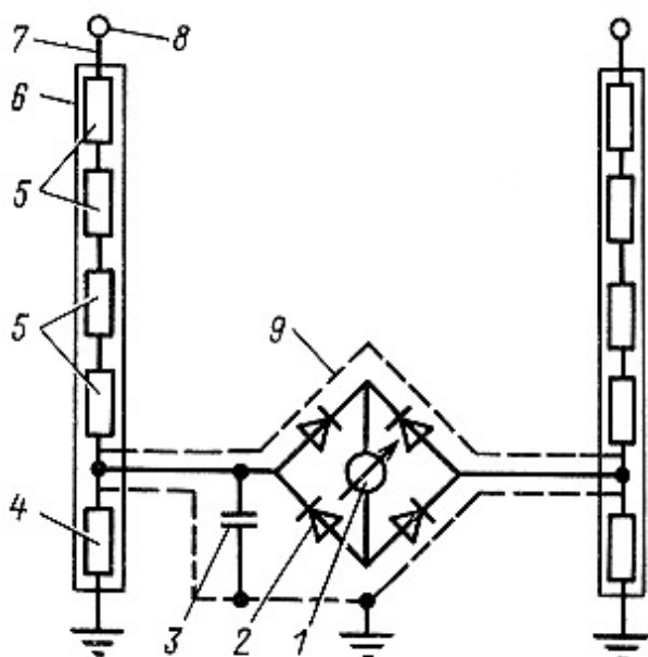
Рис. 8.7. Принципиальная схема индикатора напряжения Ленэнерго для фазировки в установках 35 и 110 кВ:
