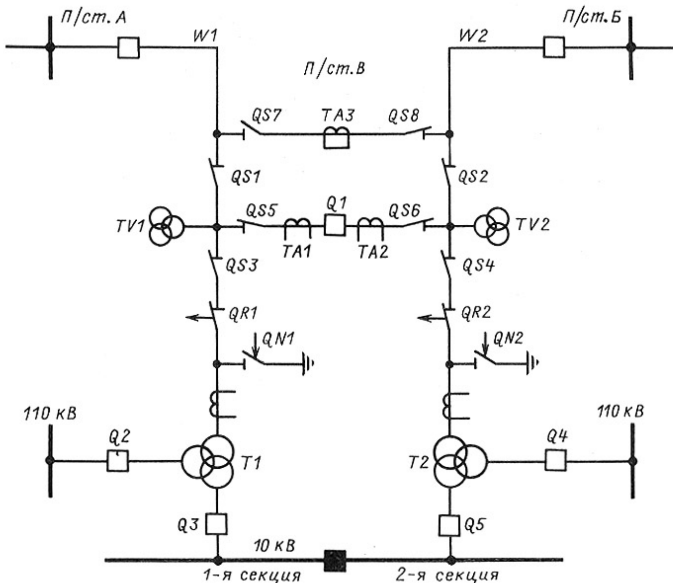
Рис. 9.14. Подстанция 220 кВ по схеме мостика с секционным выключателем и ремонтной перемычкой на разъединителях
