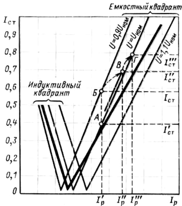
Рис. 2.3. Семейство V-образных нагрузочных характеристик синхронного компенсатора
