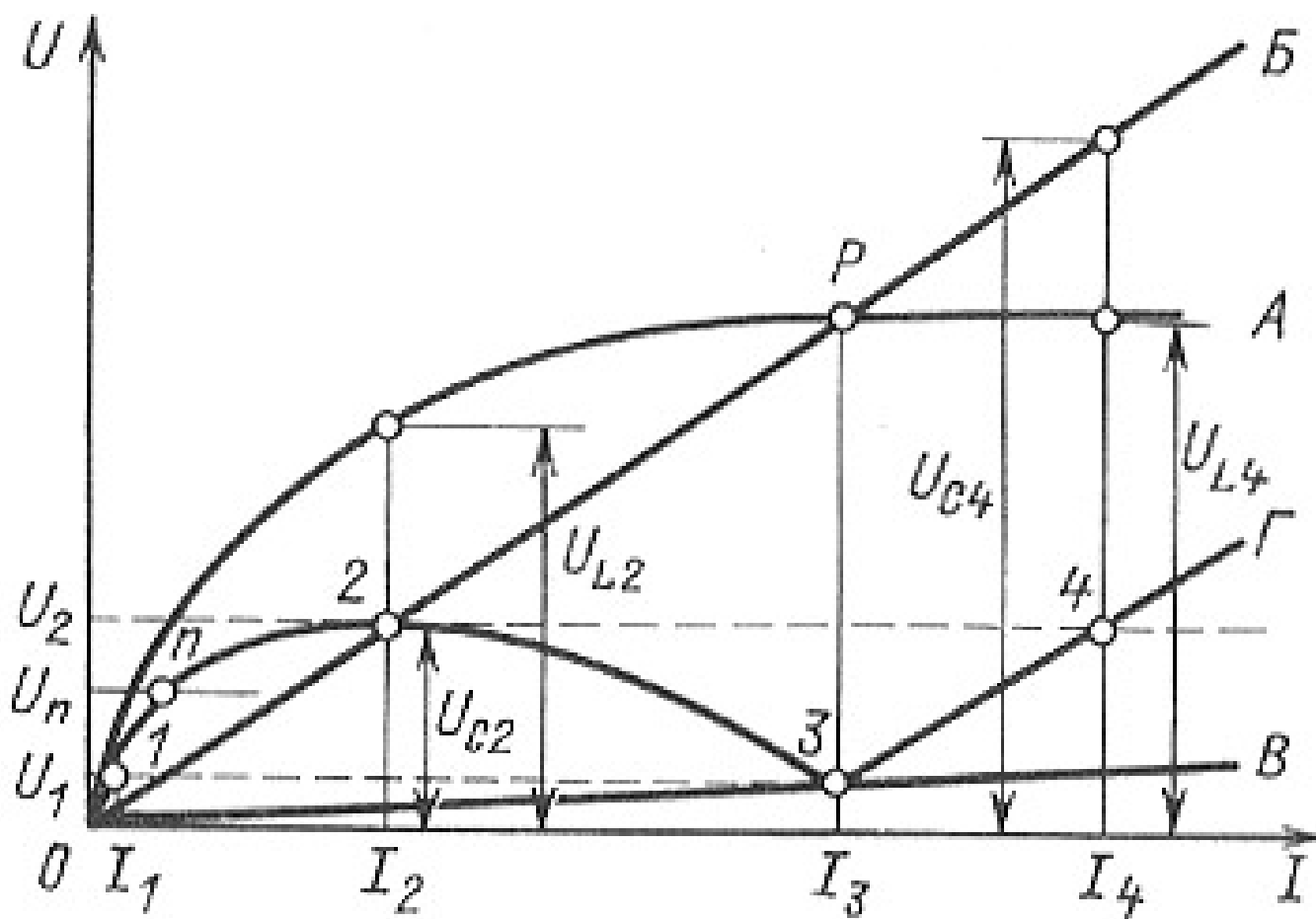
Рис. 10.4. Последовательная феррорезонансная цепь:
