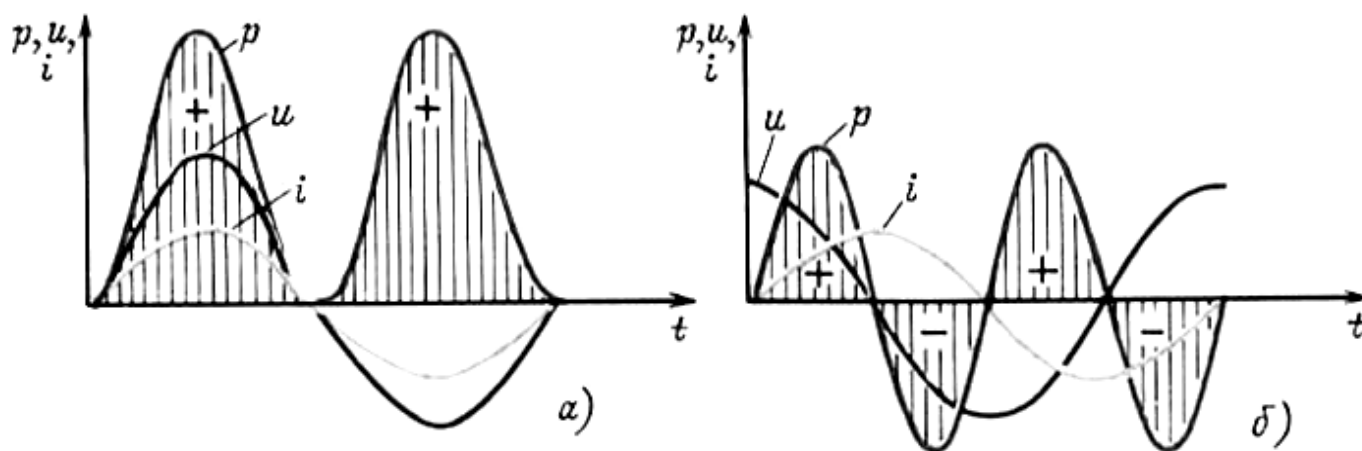
Рис. 2.2. Графики мгновенных значений мощности p=ui при u и i , совпадающих по фазе (а) и сдвинутых по фазе на 90^\circ (б): заштрихованная площадь, ограниченная кривой мощности и осью абсцисс, соответствует энергии, поступающей в цепь (отмечено знаком +) и возвращаемой источнику (отмечено знаком -)
