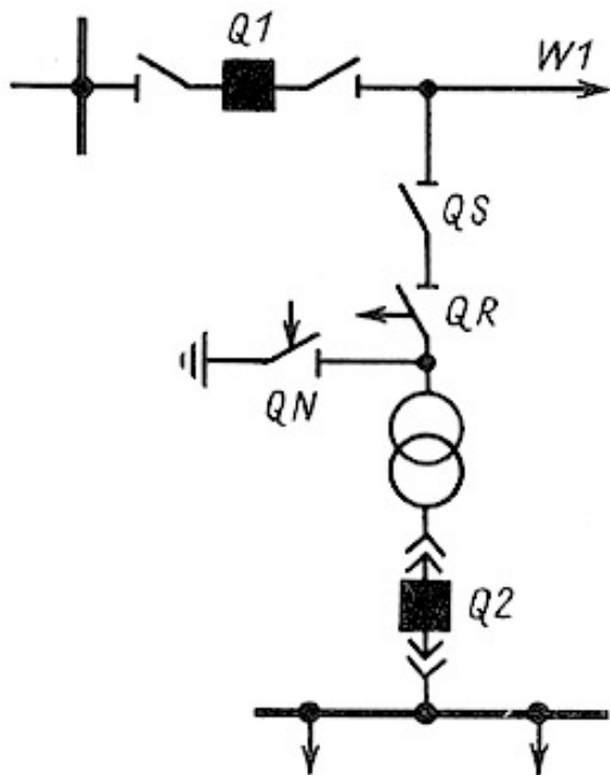
Рис. 9.4. Схема блока трансформатор-линия с отделителями и короткозамыкателем
