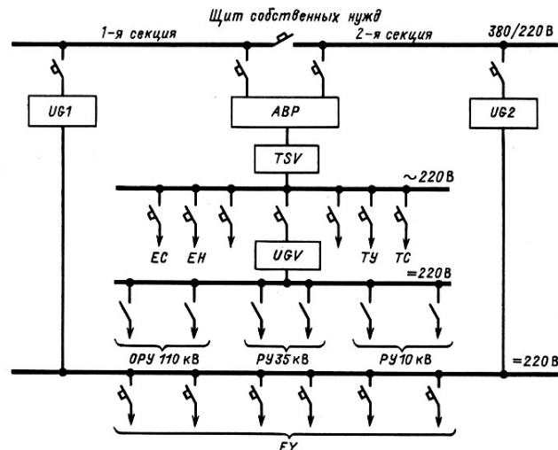
Рис. 6.5. Схема питания оперативных цепей на переменном токе
