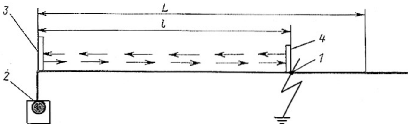
Рис. 11.3. Схема прохождения высокочастотного импульса при измерении на линии:
