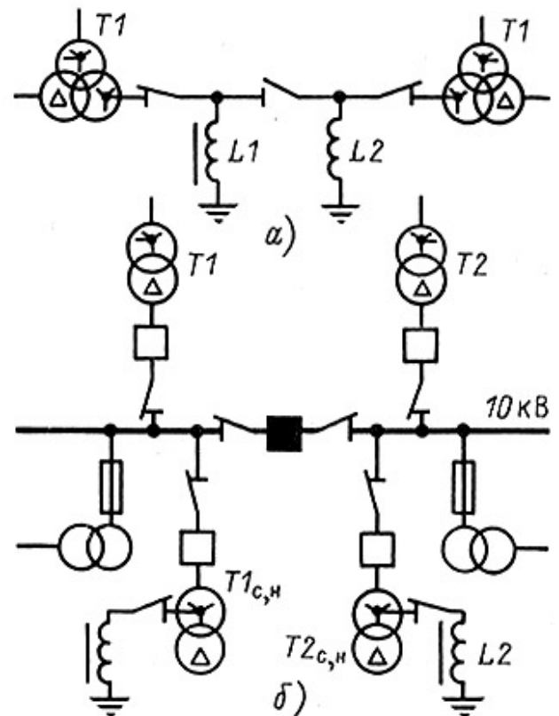
Рис. 10.2. Схема подключения дугогасящих реакторов к питающим сеть трансформаторам (а) и к вспомогательным трансформаторам (б)
