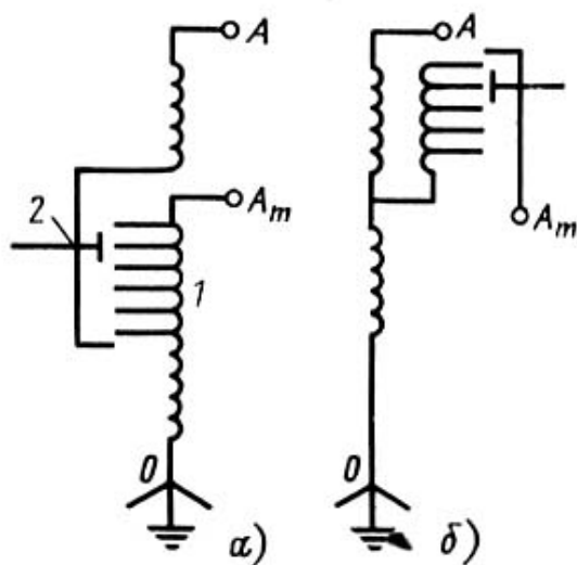
Рис. 1.12. Схема регулирования на автотрансформаторах: а - на стороне ВН; б - на стороне СН; 1 — регулировочная обмотка с отведениями; 2 — переключающее устройство
