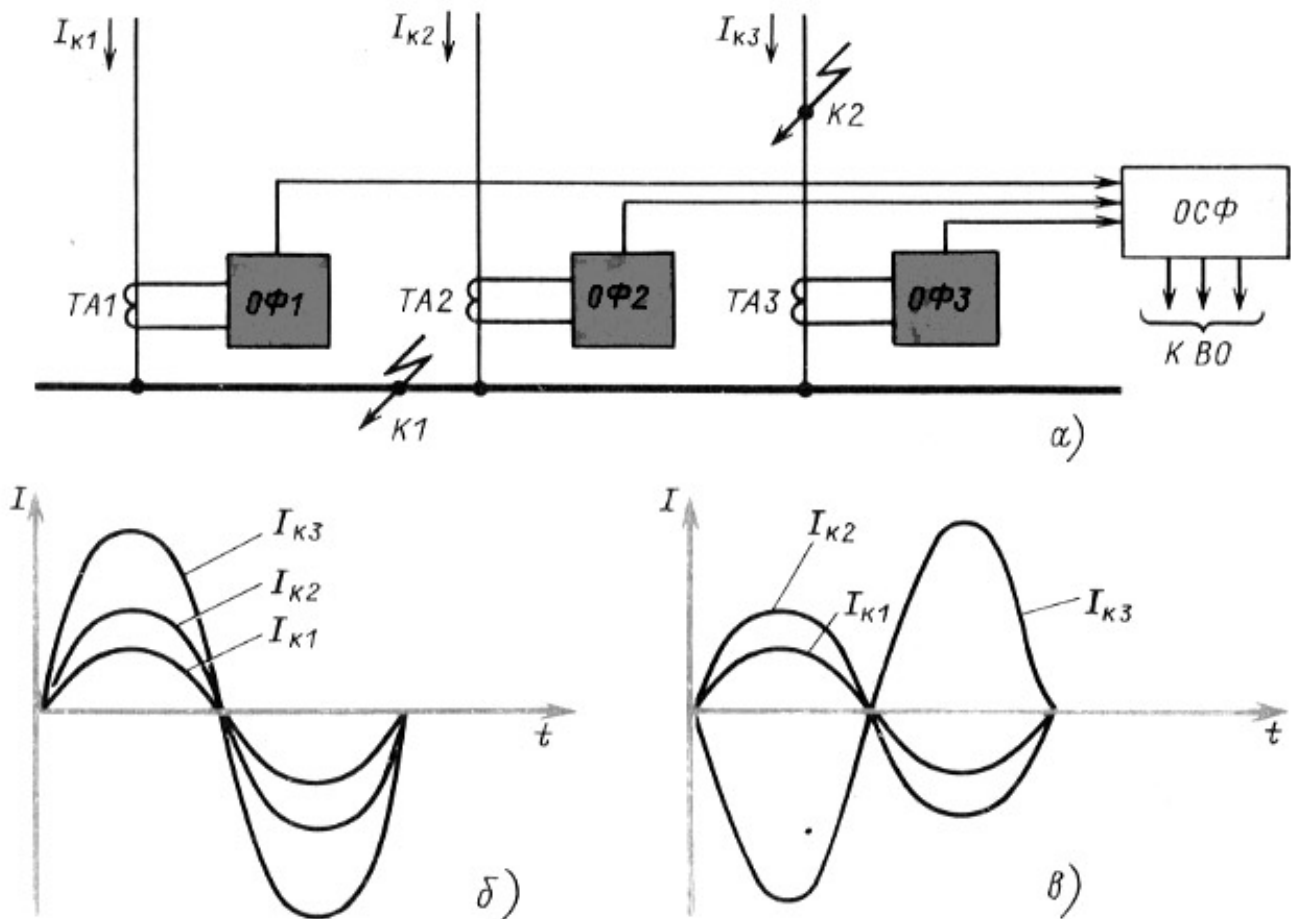
Рис. 7.28. Принцип действия дифференциально-фазной защиты шин (а) и фазы токов в присоединениях при КЗ в зоне действия защиты (б) и вне зоны (в)
