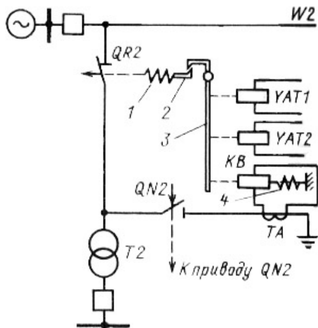
Рис. 7.31. Принципиальная схема действия отключающих электромагнитов на защелку привода отделителей:
