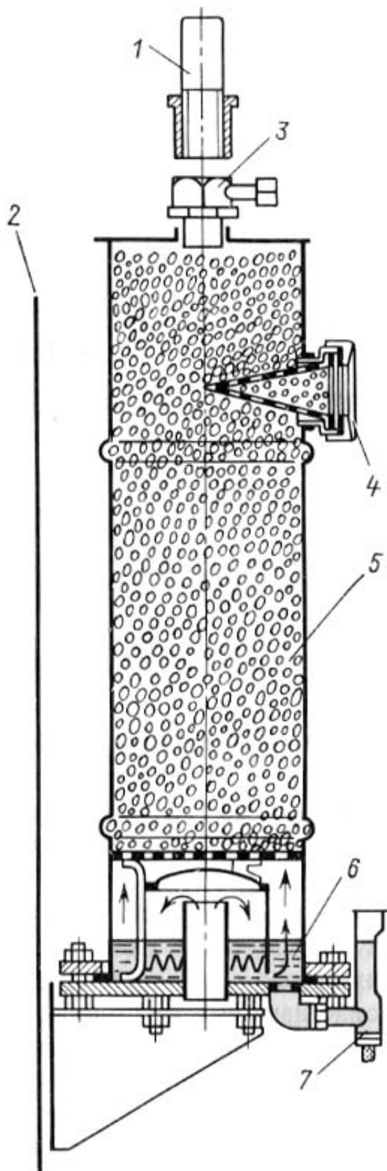
Рис. 1.25. Воздухоочистительный фильтр трансформатора: 1 - дыхательная трубка трансформатора; 2 - стенка бака; 3 - соединительная гайка; 4 - смотровое окно патрона с индикаторным силикагелем; 5 - зерна силикагеля; 6 - масляный затвор; 7 - указатель уровня масла в затворе
