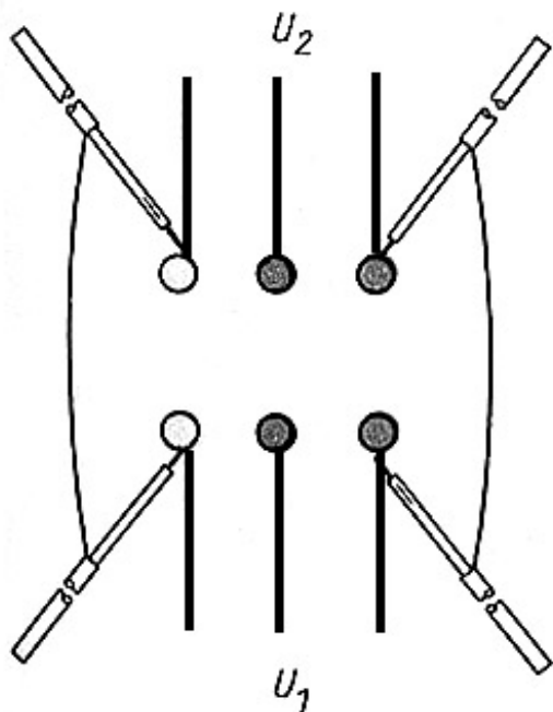
Рис. 8.6. Подключение индикатора Мосэнерго к выводам разъединителей при фазировке линий 35-110 кВ
