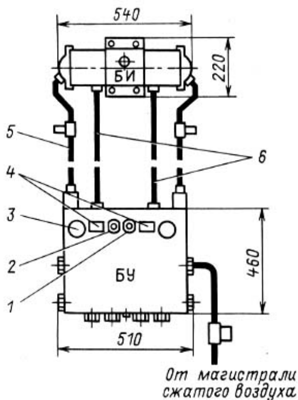
Рис. 3.14. Пневматический привод типа ПВ-20У2
