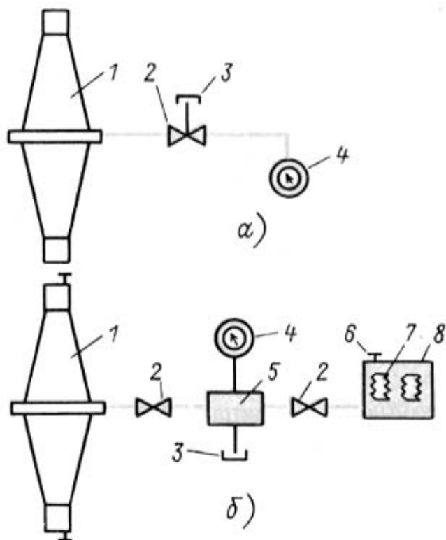
Рис. 1.29. Схемы масляных систем герметичных вводов со встроенным сифоном (а) и с выносным баком давления (б):
