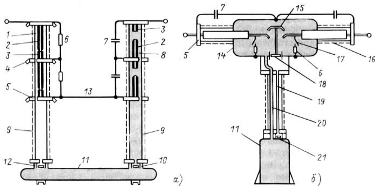
Рис. 3.6. Принципиальные конструктивные схемы воздушных выключателей на напряжение 110 кВ:
