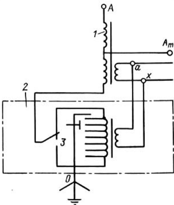
Рис. 1.14. Схема регулирования напряжения на автотрансформаторе при помощи последовательного регулировочного трансформатора в нейтрали: 1 - главный автотрансформатор; 2 - регулировочный трансформатор; 3 - реверсор
