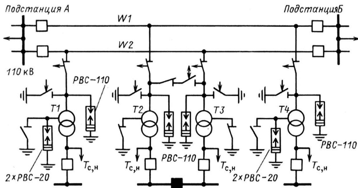
Рис. 1.21. Схема питания ответвительных подстанций от проходящей линии
