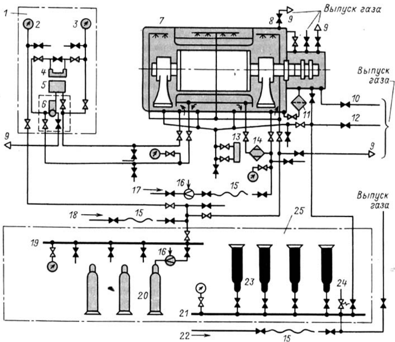
Рис. 2.9. Принципиальная схема газоснабжения синхронного компенсатора 50 МВ·А:
