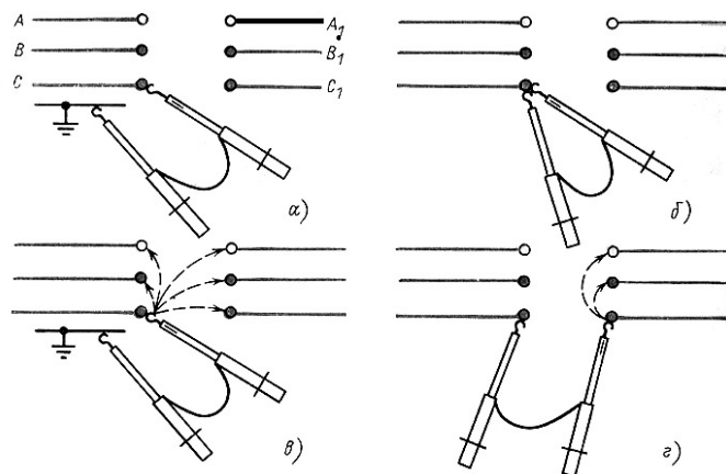
Рис. 8.5. Последовательность операций при фазировке линий 10 кВ индикатором типа УВНФ:
