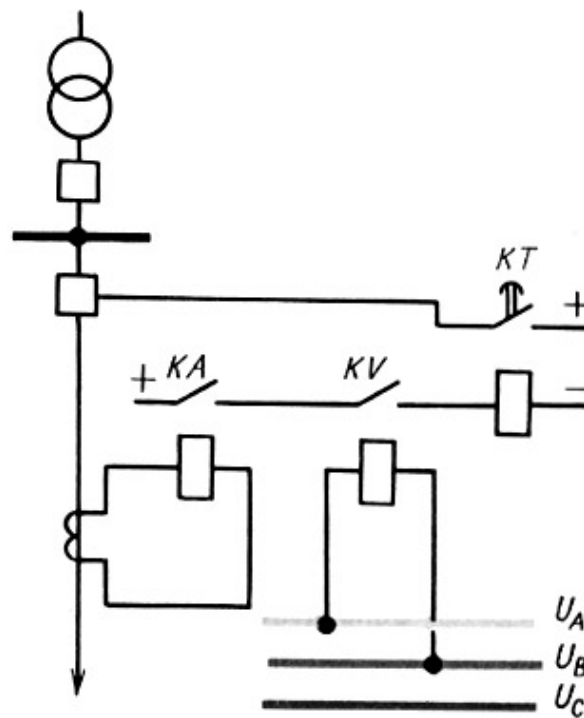
Рис. 7.8. Принципиальная схема максимальной токовой защиты с пуском от реле минимального напряжения:
