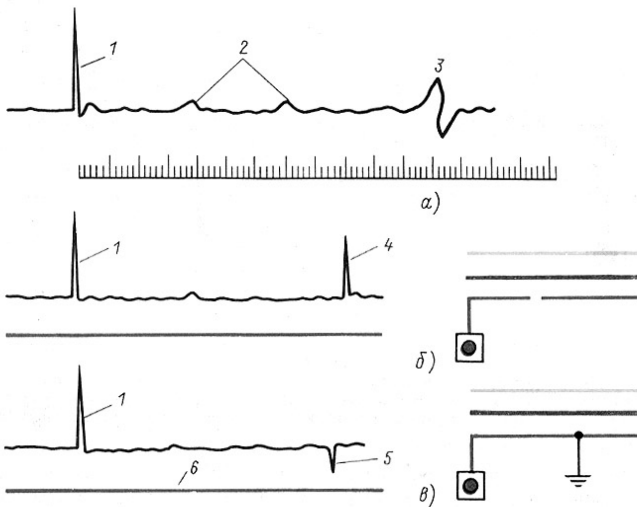
Рис. 11.4. Импульсные характеристики линии электропередачи:
