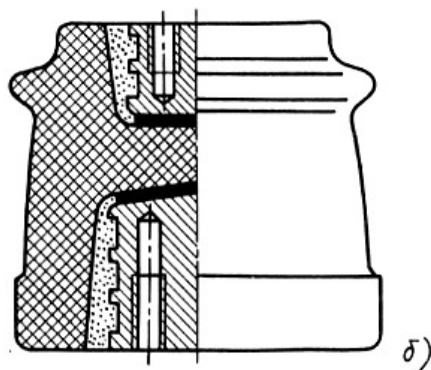
Рис. 5.1 Опорно-стержневой изолятор на напряжение 10 кВ серии ОФ для внутренней установки (а), серии ОФ с внутренней арматурой для КРУ (б)
