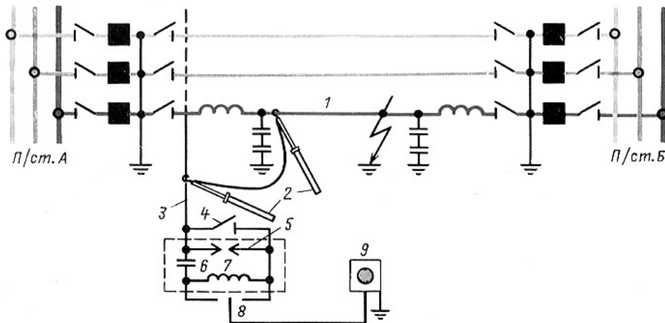
Рис. 11.2. Измерения локационных искателем на воздушной линии:
