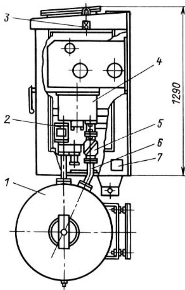
Рис. 3.5. Пневматический привод типа ШПВ-46П для масляного выключателя с большим объемом масла типа У-220
