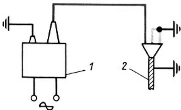
Рис. 4.15. Схема испытания кабеля:
