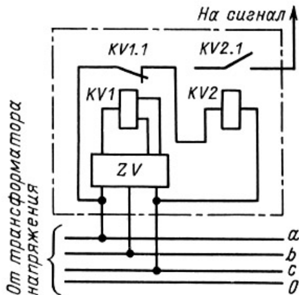
Рис. 4.6. Схема включения реле для контроля исправности цепей напряжения: ZV - фильтр напряжения обратной последовательности; KV1 , KV2 - реле напряжения
