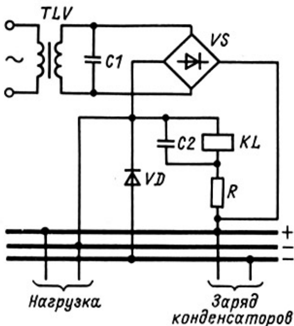
Рис. 6.4. Принципиальная упрощенная схема устройства БПЗ 401
