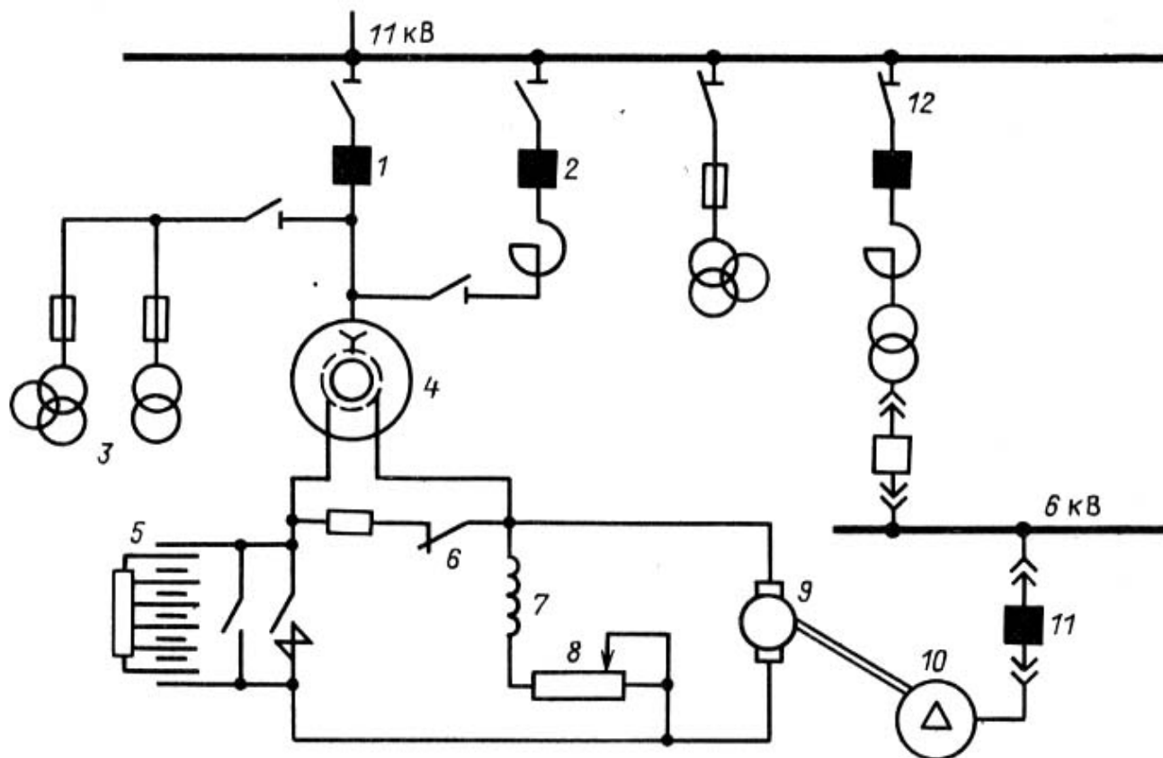
Рис. 2.12. Схема отключенного от сети синхронного компенсатора:
