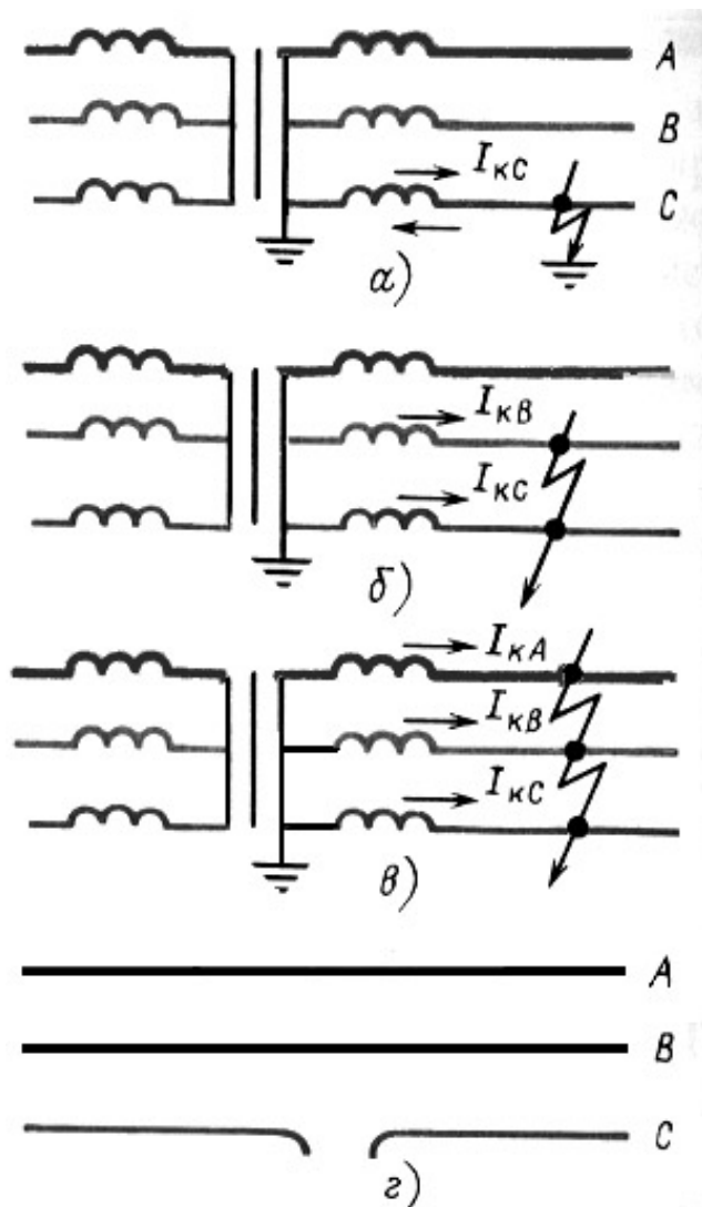
Рис. 7.1. Повреждения в электрической сети с заземленной нейтралью:
