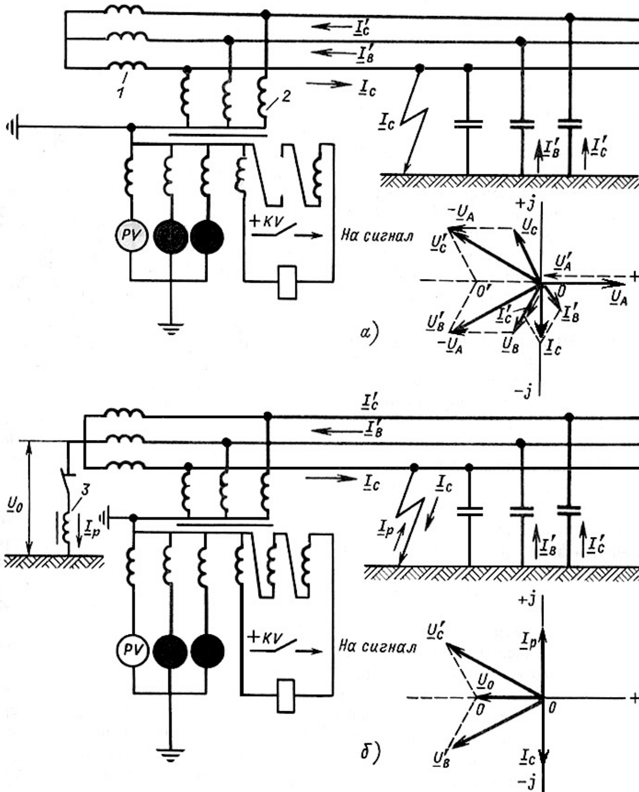
Рис. 10.1. Замыкание фазы на землю в сети с изолированной нейтралью (а) и с компенсацией емкостных токов (б): 1 - трансформатор, питающий сеть; 2 - измерительный трансформатор напряжения; 3 - дугогасящий реактор; KV - реле напряжения
