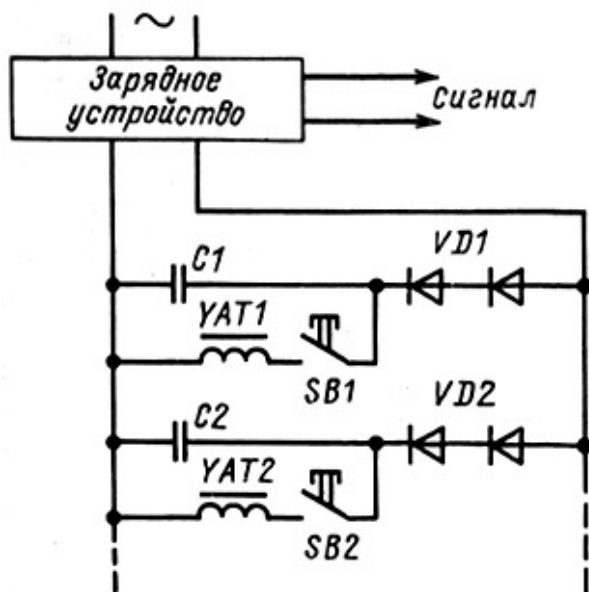
Рис. 6.3. Схема включения конденсаторов с разделительными диодами
