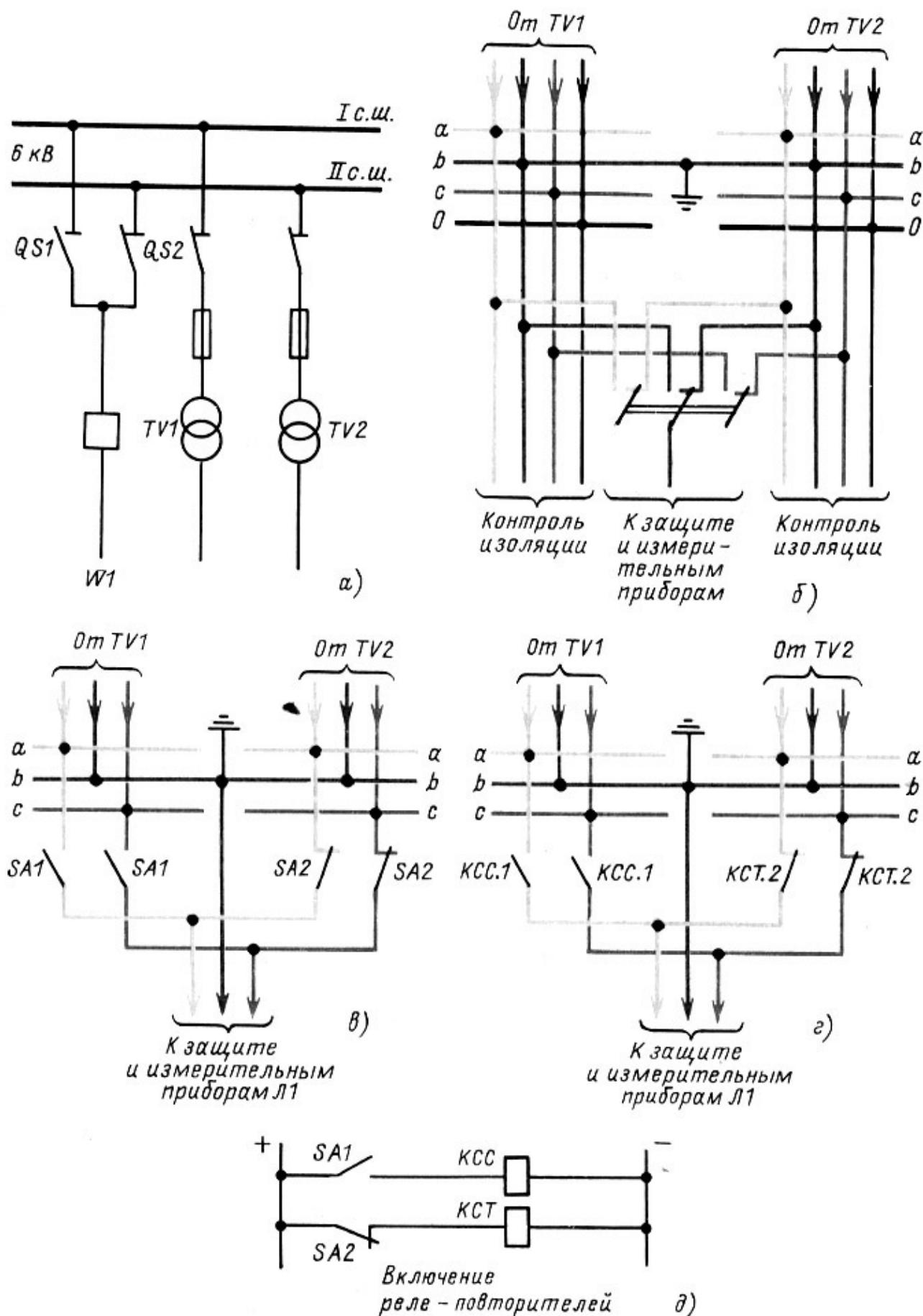
Рис. 4.4. Принципиальные схемы переключения цепей напряжения с одного трансформатора напряжения TV1 на другой TV2:
