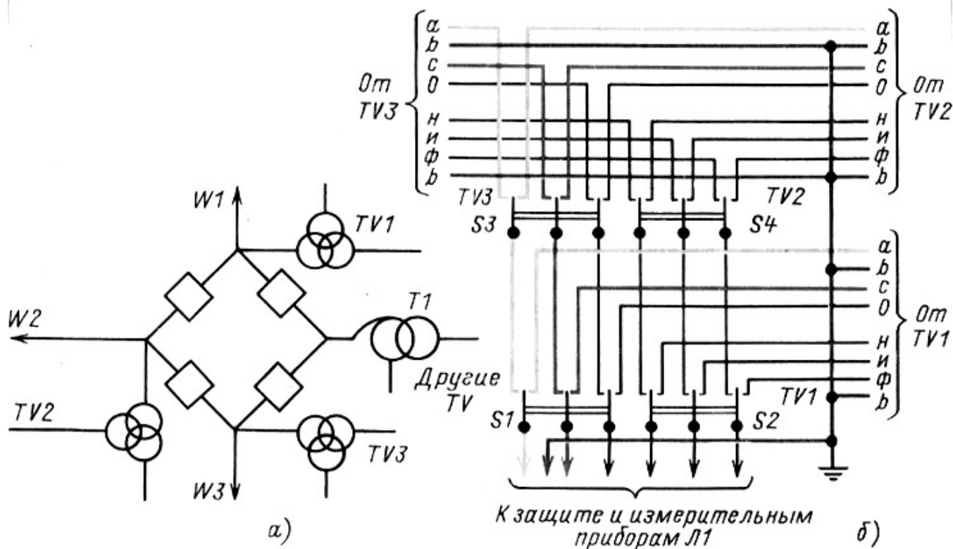
Рис. 4.7. Переключение цепей напряжения с одного трансформатора напряжения TV1 , подключенного к линии W1 , на другие ( TV2 или TV3 ): а - схема первичных соединений подстанции 500 кВ; б - схема цепей напряжения линии
