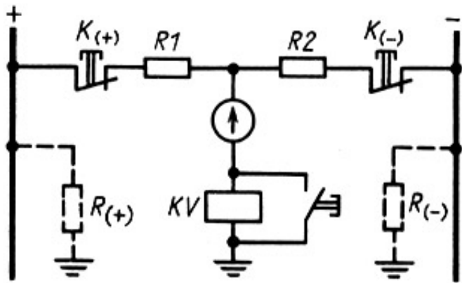
Рис. 6.12. Схема устройства непрерывного автоматического контроля состояния изоляции цепей постоянного оперативного тока
