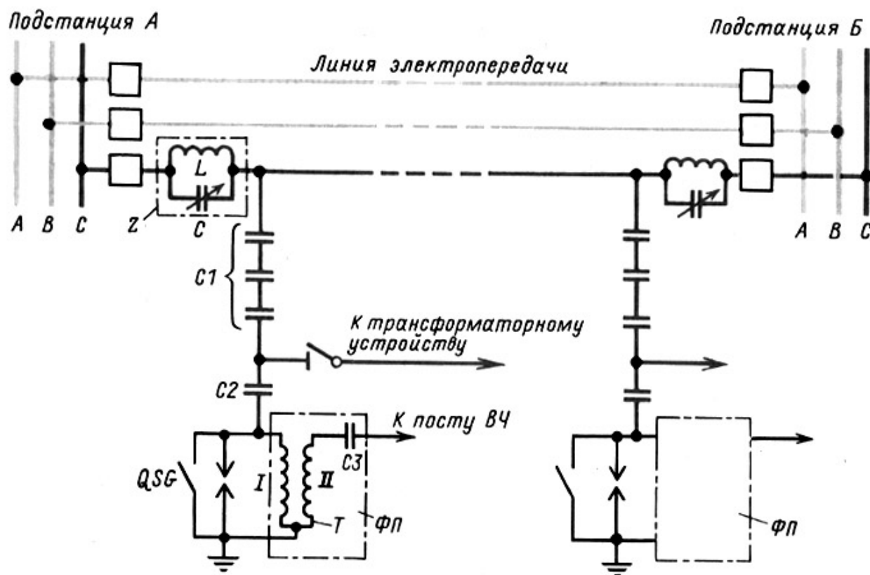
Рис. 4.8. Принципиальная схема высокочастотного канала по линии электропередачи:
