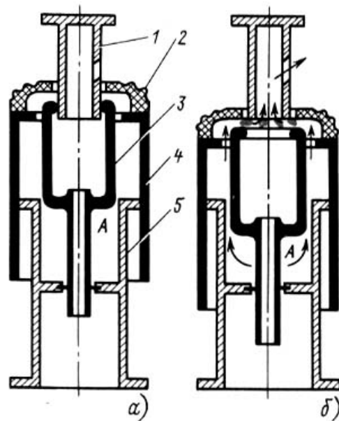
Рис. 3.11. Автопневматическое дугогасительное устройство элегазового выключателя 110 кВ:
