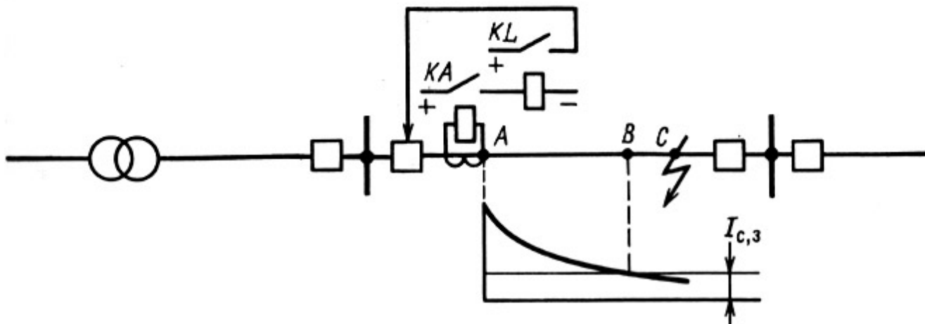
Рис. 7.6. Зона действия отсечки на линии с односторонним питанием
