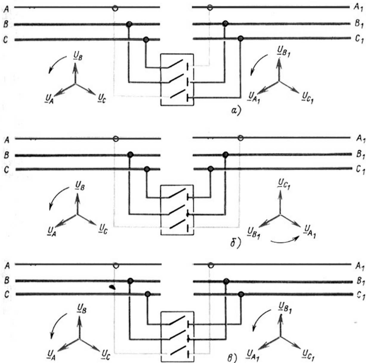
Рис. 8.2. Варианты несовпадения (а, б) и совпадения (в) фаз двух частей электроустановки
