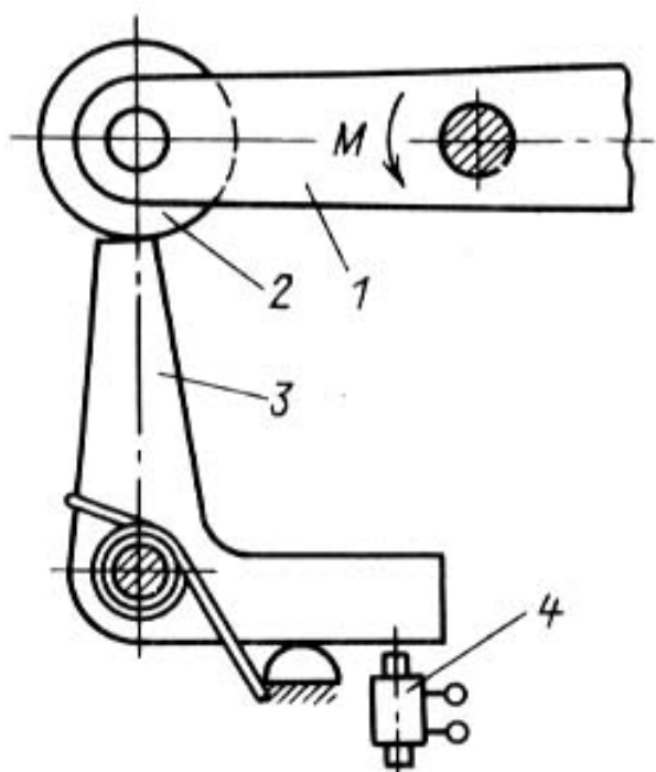
Рис. 3.2. Запирающий механизм
