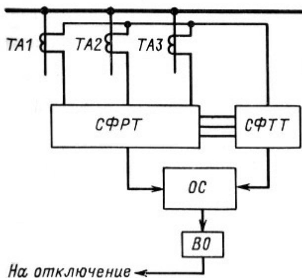
Рис. 7.29. Структурная схема дифференциальной защиты шин с торможением
