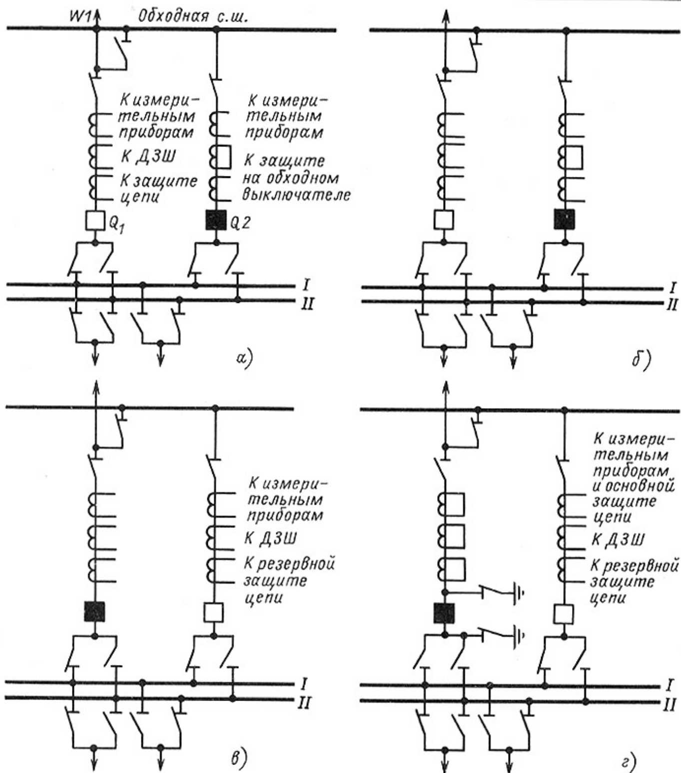
Рис. 9.10. Основные группы операций при замене выключателя электрической цепи обходным выключателем:
