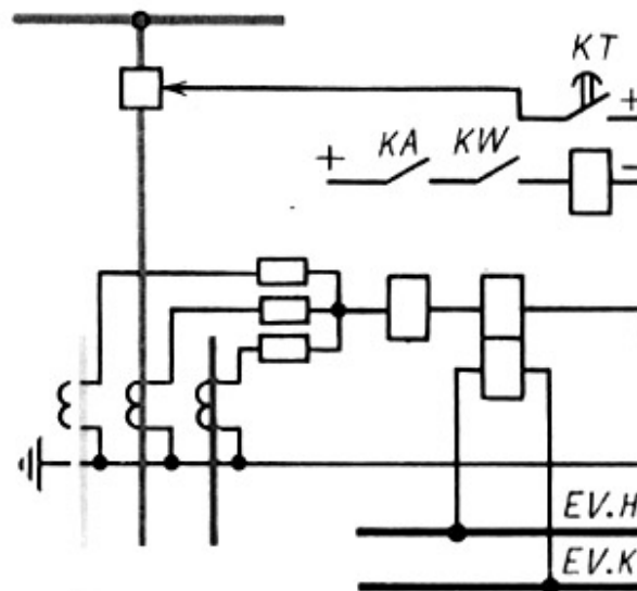
Рис. 7.13. Схема токовой направленной защиты нулевой последовательности
