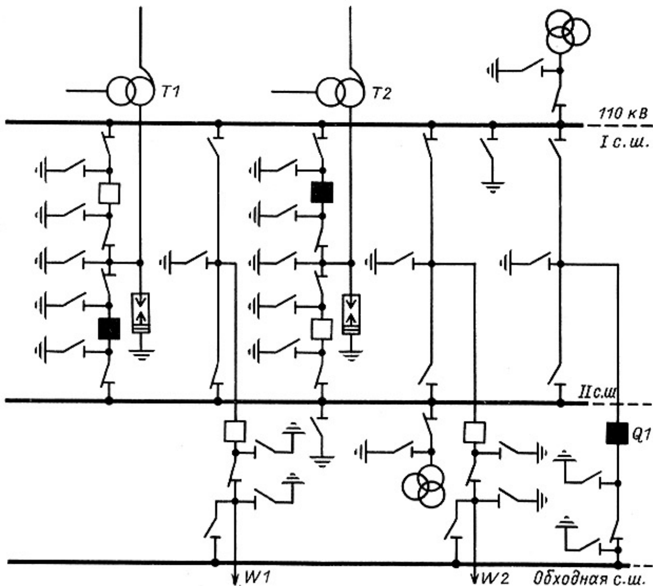
Рис. 9.8. Схема РУ 110 кВ с двумя системами шин, работающими раздельно, к началу перевода присоединений с одной системы шин на другую без ШСВ, но при наличии присоединений с двумя выключателями на цепь
