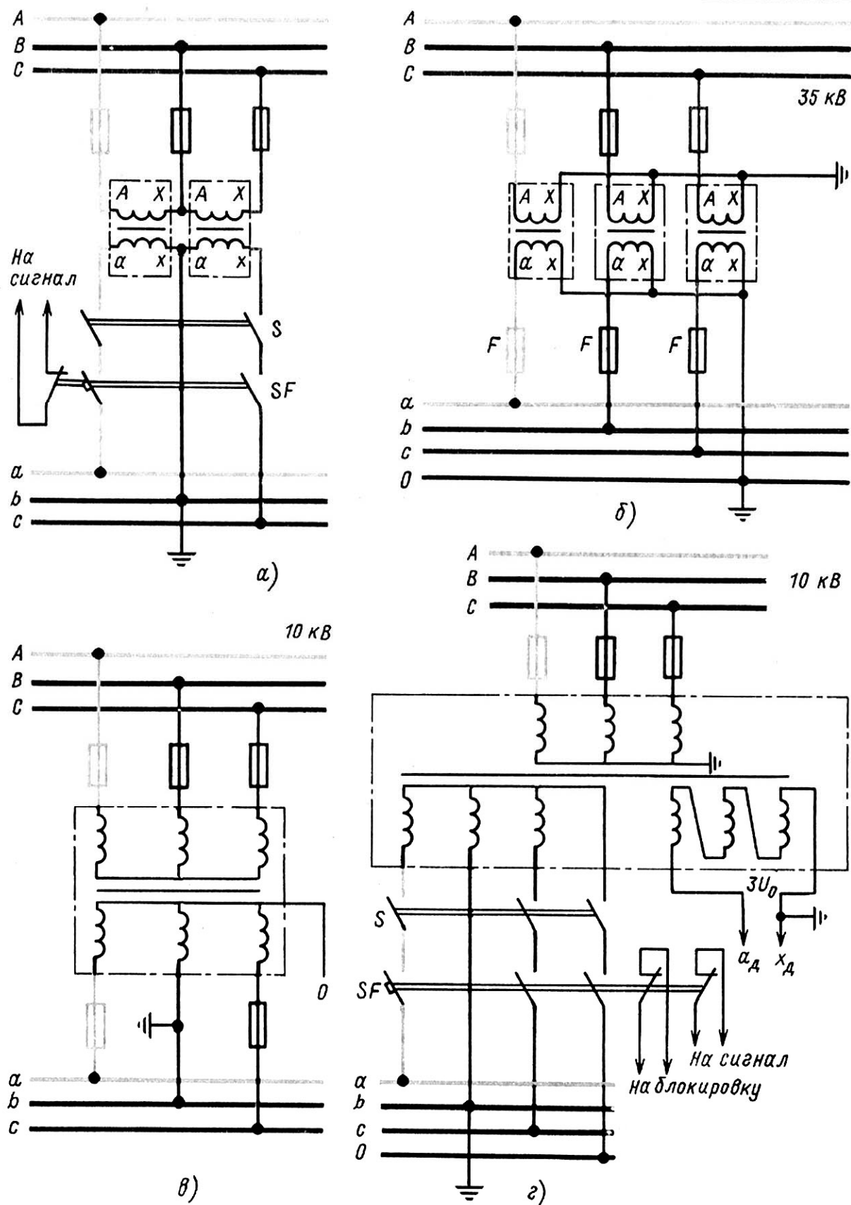
Рис. 4.3. Схемы включения однофазных и трехфазных трансформаторов напряжения
