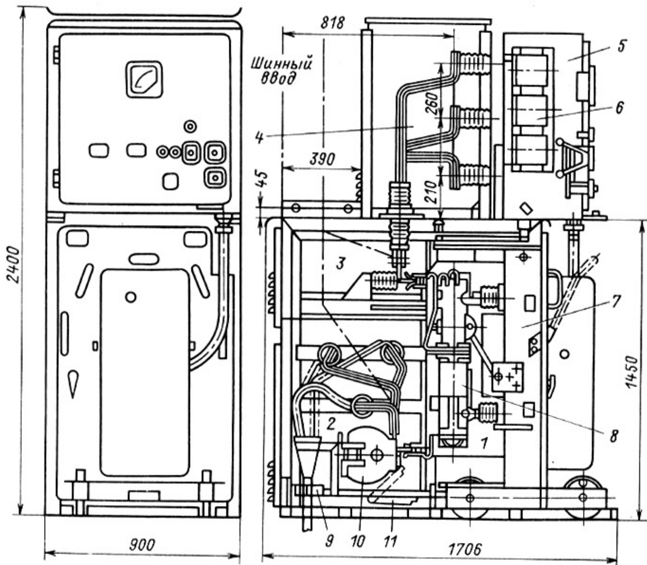
Рис. 5.4. Шкаф КРУ серии К-ХП с выключателем ВМП-10:
