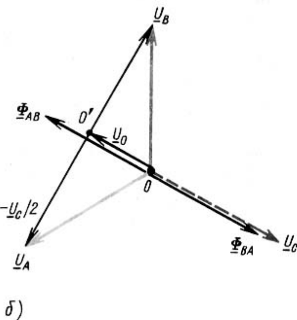
Рис. 1.20. Полнофазный (а) и двухфазный (б) режимы включения ненагруженного трансформатора с изолированной нейтралью
