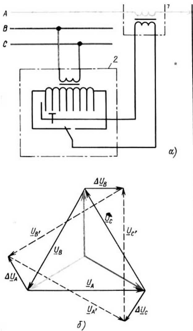
Рис. 1.15. Последовательный регулировочный трансформатор для поперечного регулирования напряжения: а - схема включения в фазу А (для фаз В и С схемы включения аналогичны); б - векторная диаграмма; 1 - последовательный регулировочный трансформатор; 2 - регулировочный трансформатор
