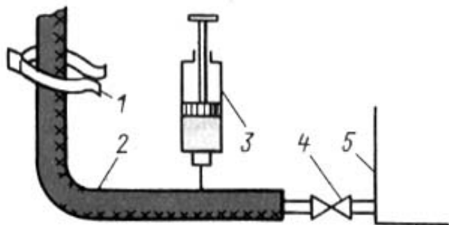
Рис. 1.31. Отбор проб масла из трансформатора с помощью шприца: 1 - зажим; 2 - резиновый шланг; 3 - шприц; 4 - кран; 5 - бак трансформатора
