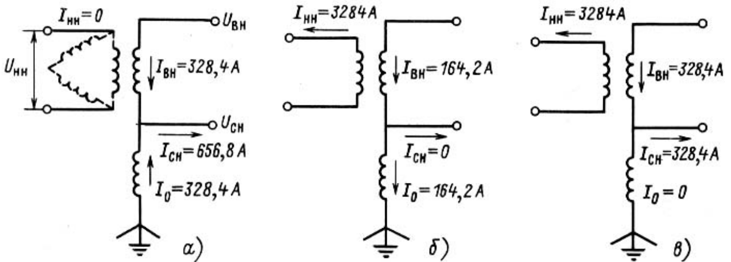
Рис. 1.4. Распределение токов в обмотках автотрансформатора в различных режимах выдачи мощности: а - ВН→СН; б - ВН→НН; в - ВН→СН и одновременно ВН→НН. Показаны обмотки одной фазы
