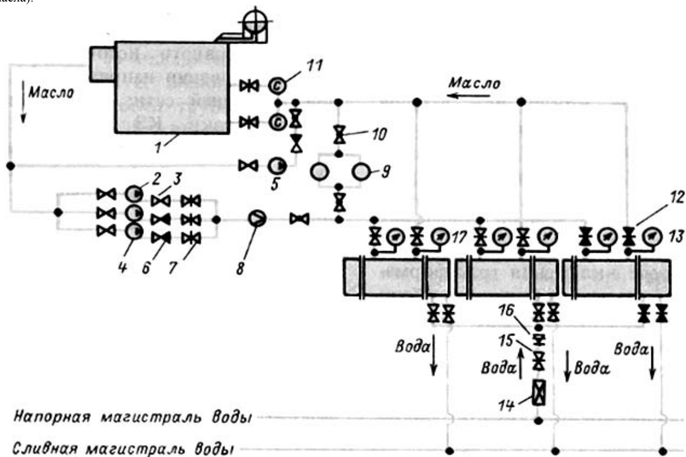
Рис. 1.7. Принципиальная схема охлаждения Ц:
