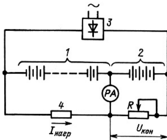
Рис. 6.6. Принципиальная схема подзаряда концевых элементов батареи от общего подзарядного агрегата:
