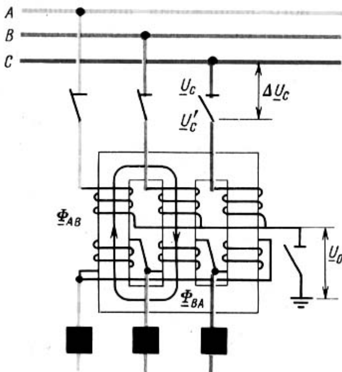
Рис. 1.20. Полнофазный (а) и двухфазный (б) режимы включения ненагруженного трансформатора с изолированной нейтралью
