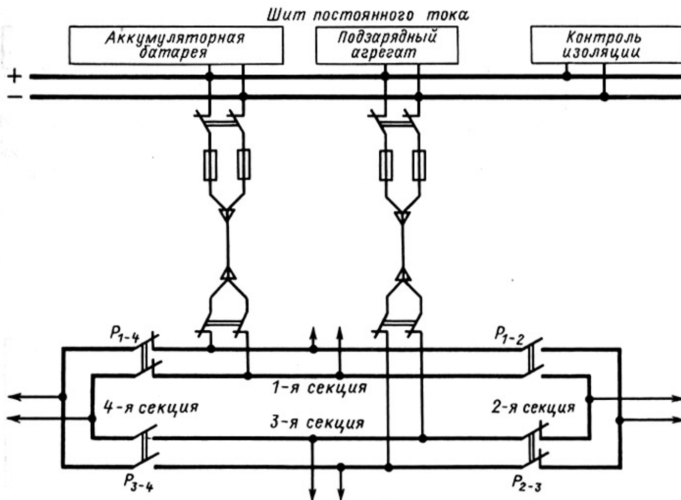
Рис. 6.10. Схема питания электромагнитов включения приводов выключателей на открытом РУ 110 кВ
