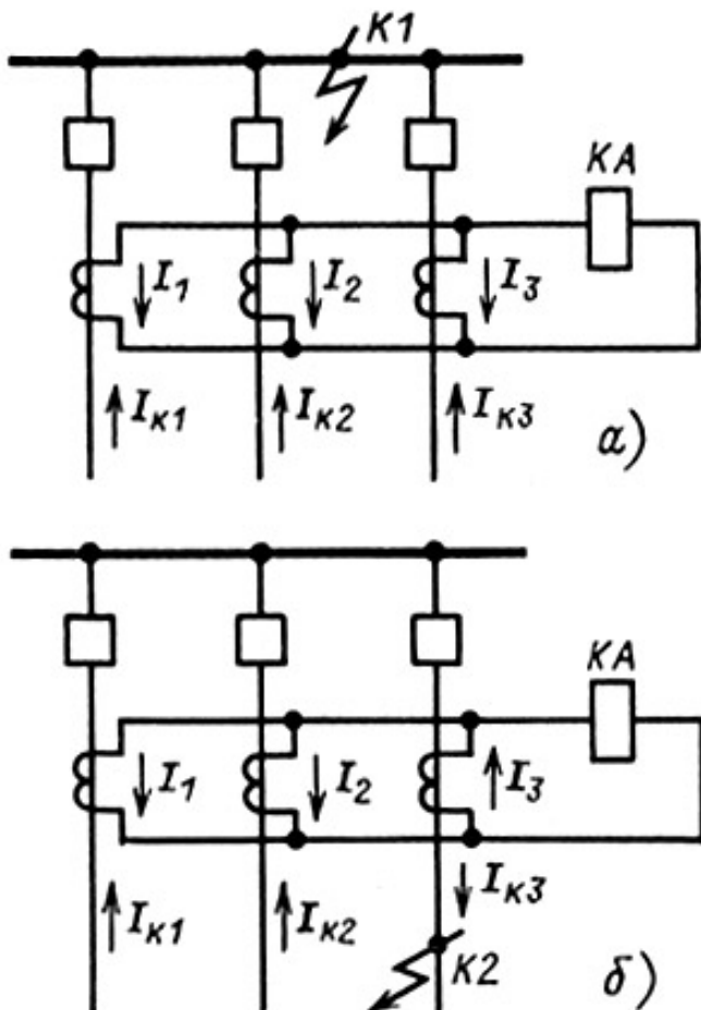
Рис. 7.26. Токи в реле дифференциальной токовой защиты тин
