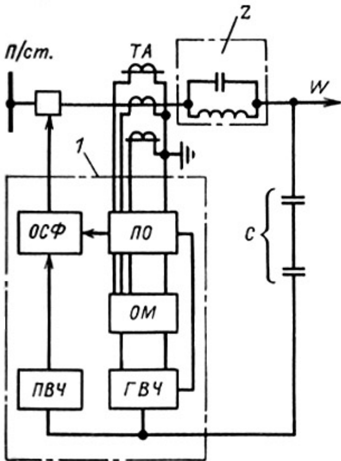
Рис. 7.25. Структура полукомплекта дифференциально-фазной защиты:
