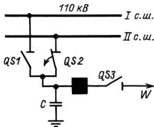
Рис. 3.15. Схема, поясняющая отключение шинным разъединителем SW2 небольшого зарядного тока:
