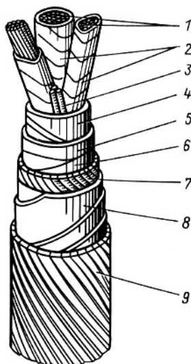
Рис. 4.13. Трехжильный кабель с поясной изоляцией из пропитанной бумаги:
