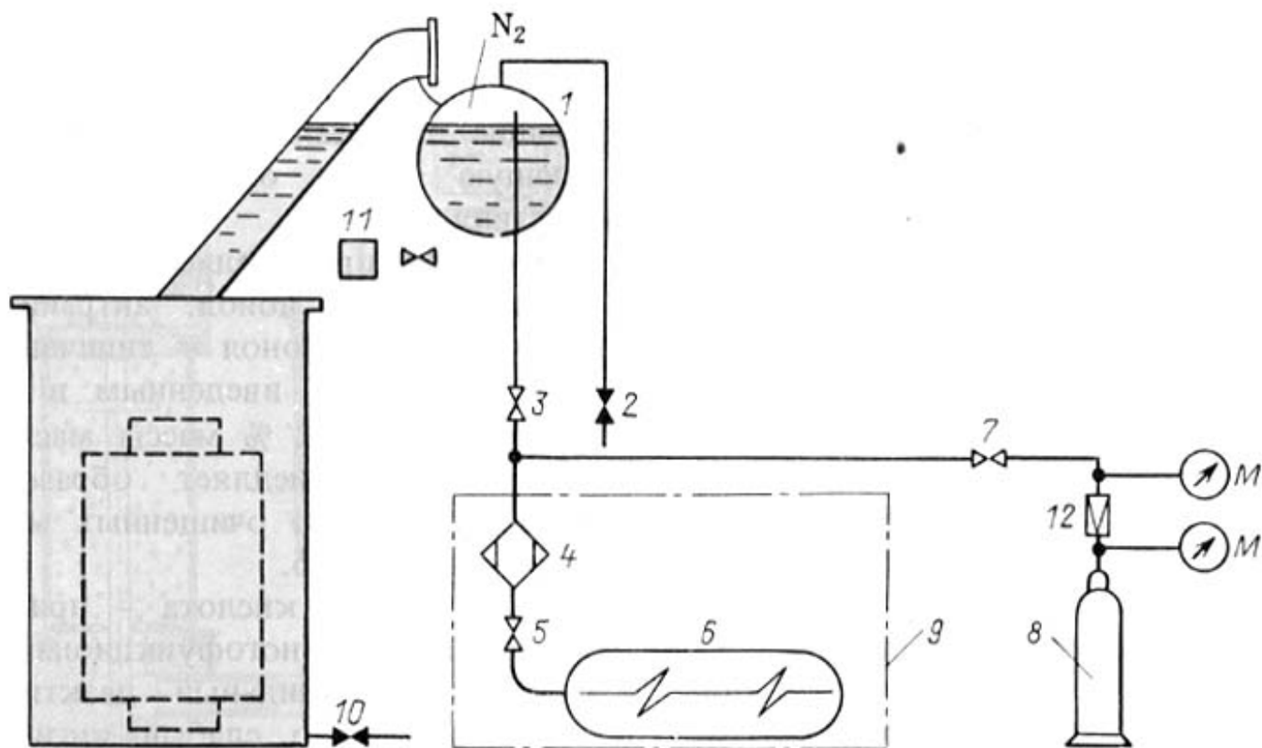
Рис. 1.26. Схема азотной защиты масла в трансформаторе с применением эластичной емкости: 1 - расширитель трансформатора; 2 - вентиль продувки азотом надмасляного пространства; 3 - кран питания системы азотом; 4 - осушитель силикагелевый (или цеолитовый); 5 - вентиль эластичного резервуара; 6 - эластичный резервуар; 7 - кран подключения баллона с редуктором и манометрами давления; 8 - газовый баллон; 9 - защитный металлический кожух; 10 - сливной кран; 11 - газовое реле; 12 - редуктор
