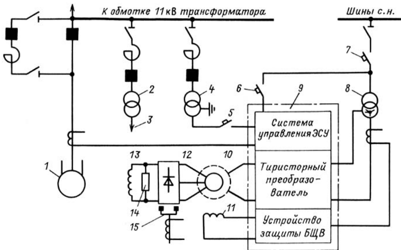
Рис. 2.8. Принципиальная схема бесщеточного положительного возбуждения синхронного компенсатора 50 МВ·А:
