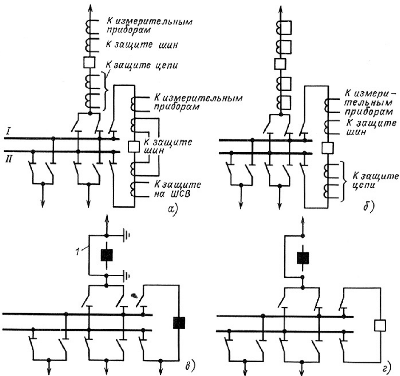
Рис. 9.9. Основные группы операций при замене выключателя электрической цепи шиносоединительным выключателем: а - подготовка схемы первичных соединений; б - переключение защит и устройств автоматики на трансформаторы тока ШСВ; в - установка токопроводящих перемычек; г - включение электрической цепи в работу с помощью ШСВ; 1 – перемычка
