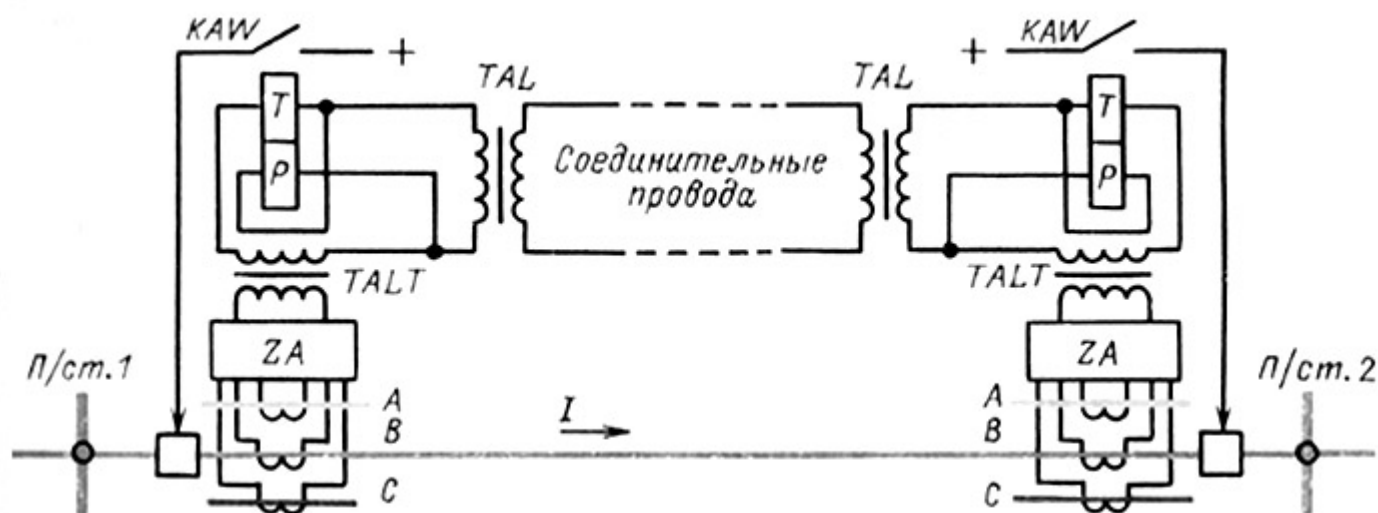
Рис. 7.18. Принципиальная схема продольной дифференциальной защиты линии:
