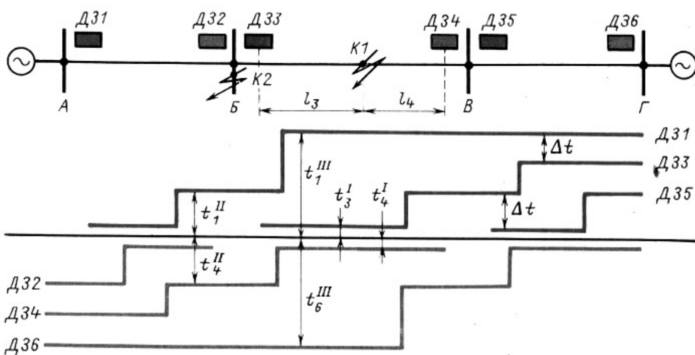
Рис. 7.15. Защита участка сети дистанционными защитами и характеристики выдержек времени этих защит:
