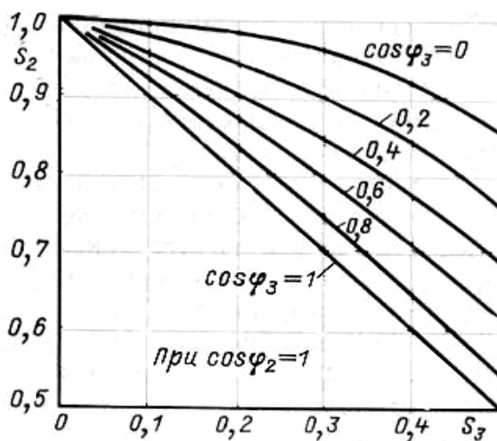
Рис. 1.5. Кривые допустимых нагрузок S_2 и S_3 автотрансформатора в режиме ВН→СН и одновременно ВН→НН
