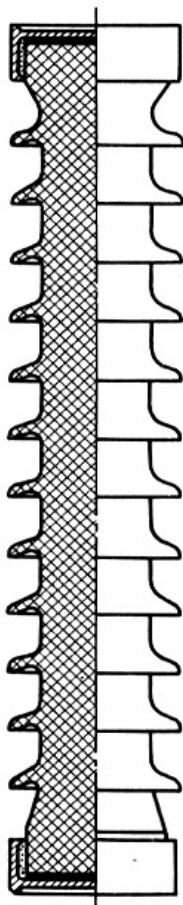
Рис. 5.2. Опорно-стержневой изолятор на напряжение 110 кВ серии ОНС
