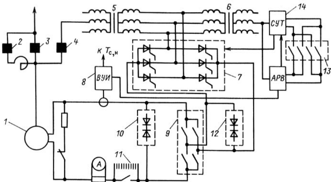
Рис. 2.7. Принципиальная схема тиристорного возбуждения синхронного компенсатора 100 МВ·А:
