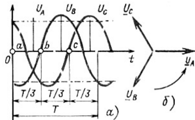
Рис. 8.1. Синусоидальное (а) и векторное (б) изображение трехфазной симметричной системы напряжений
