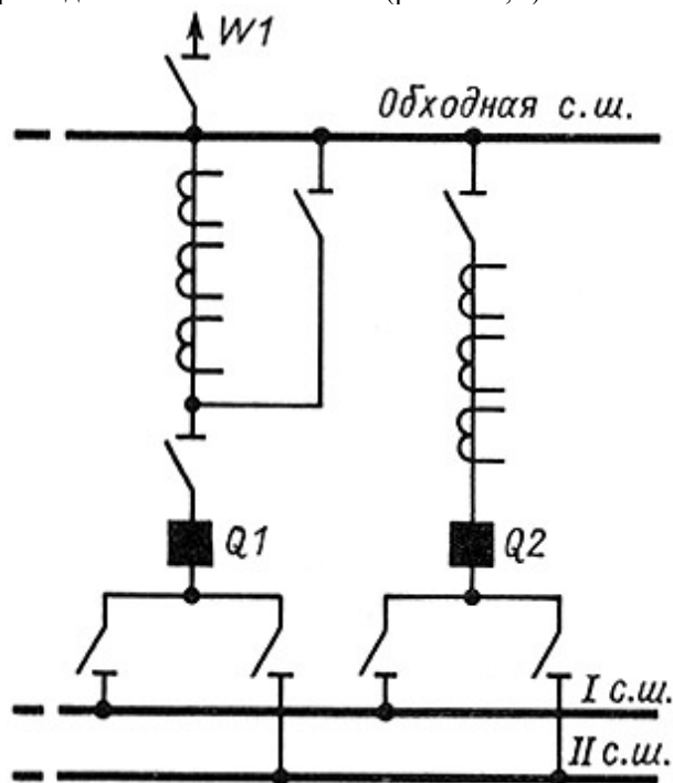
Рис. 9.11. Схема установки трансформаторов тока, при которой в случае замены выключателя линии W1 обходным выключателем Q2 достаточно действие защит переключить на выключатель Q2 только по оперативным цепям
