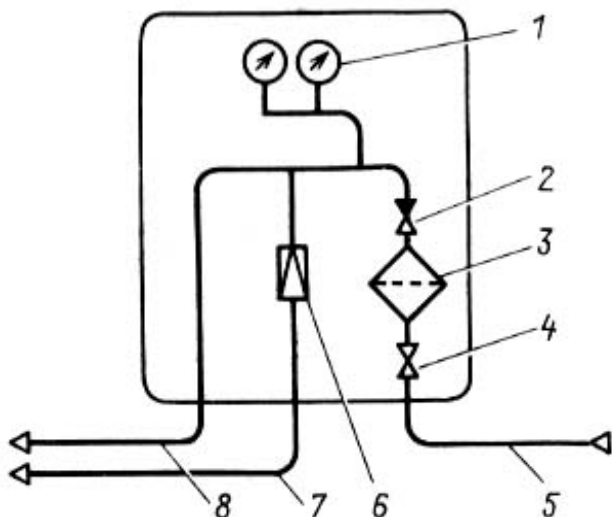
Рис. 3.7. Схема распределительного шкафа для воздушного выключателя серии ВВШ (ВВН):
