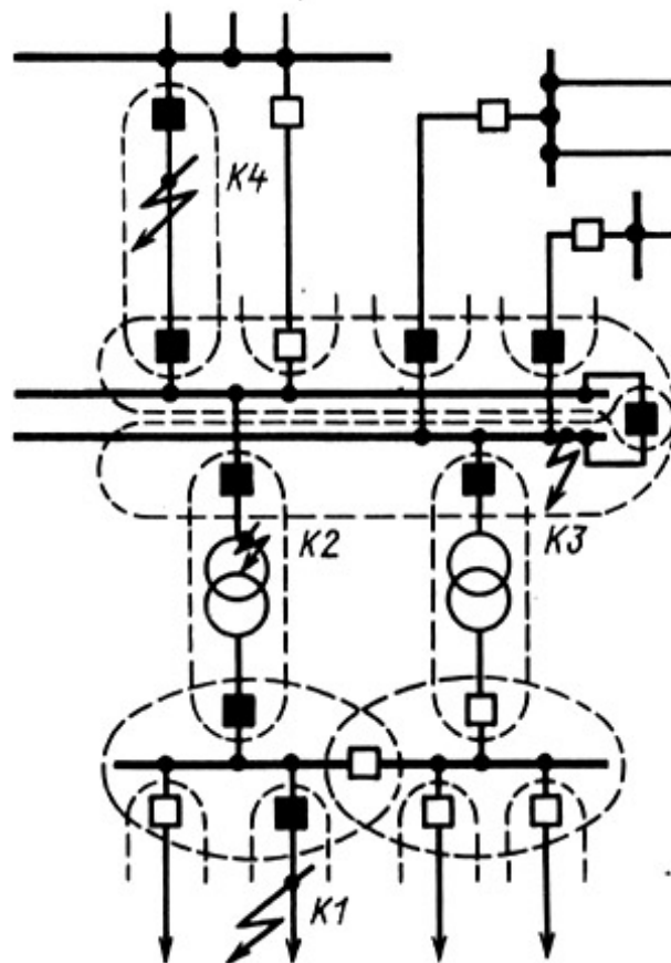
Рис. 7.4. Участки схемы, отключаемые при КЗ: K1-K4 - точки КЗ. Выключатели, отключившиеся при КЗ, зачернены
