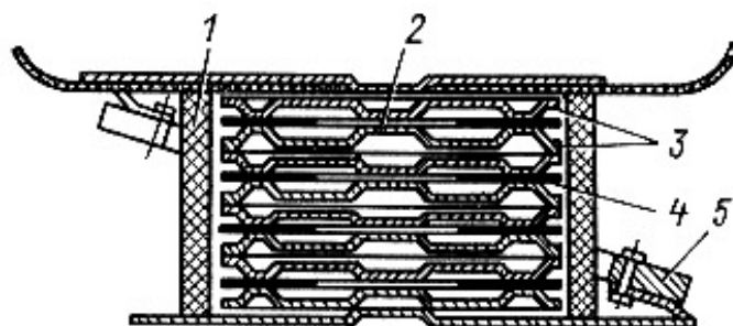
Рис. 4.10. Блок искровых промежутков вентильного разрядника серии РВС
