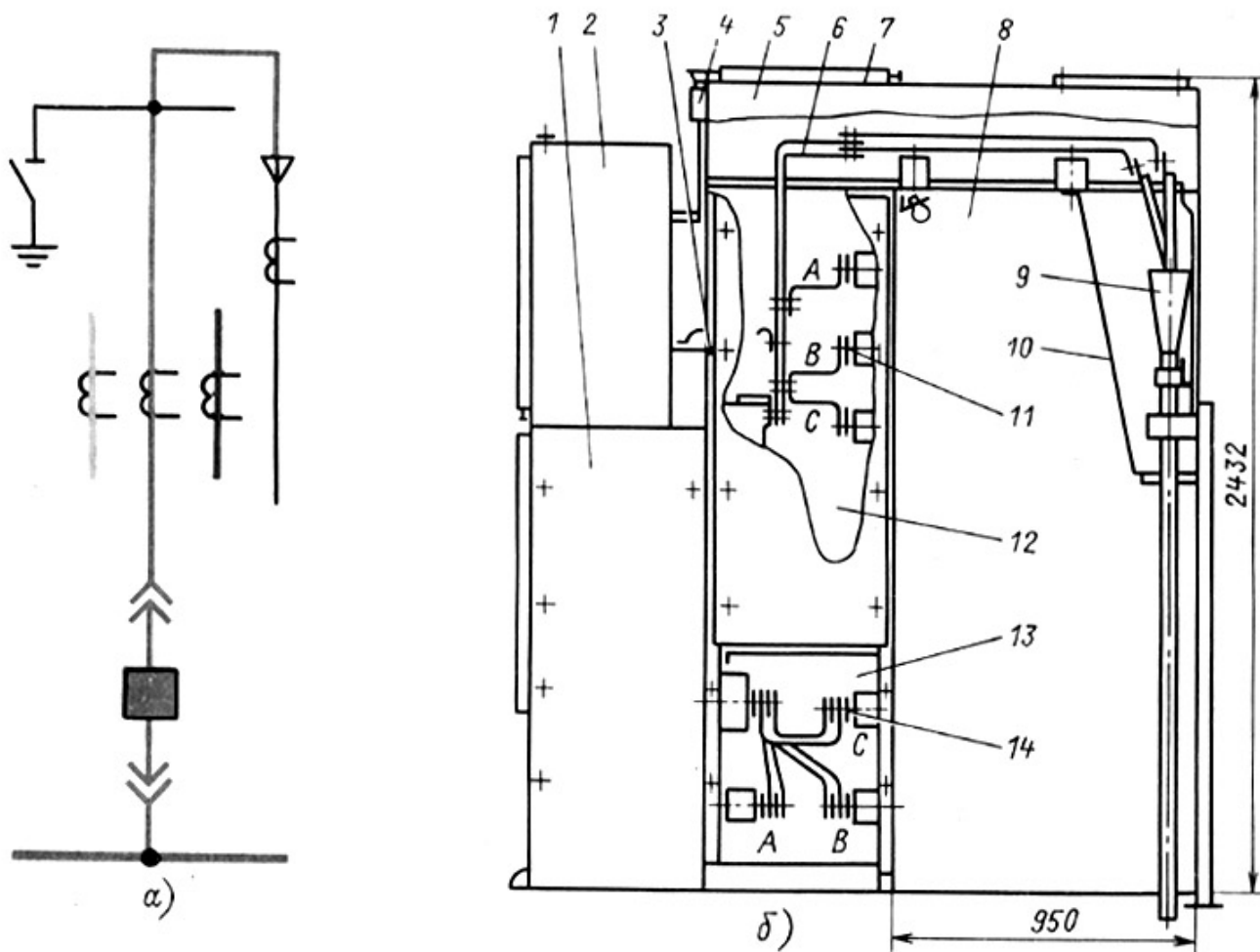
Рис. 5.6. Шкаф КРУ серии К-104 с выключателем ВК-10:
