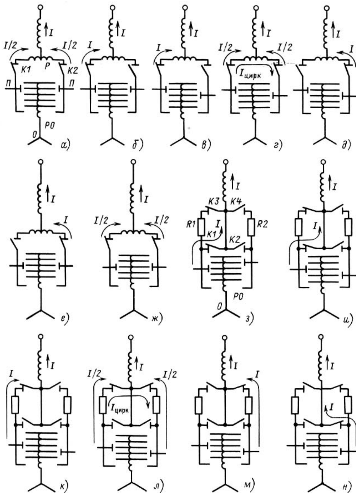
Рис. 1.16. Последовательность работы переключающих устройств РПН с реактором (а-ж) и резистором (з-н): P - реактор; R1 и R2 - резисторы; П - переключатели (избиратели); K1-K4 - контакторы; PO - регулировочная обмотка
