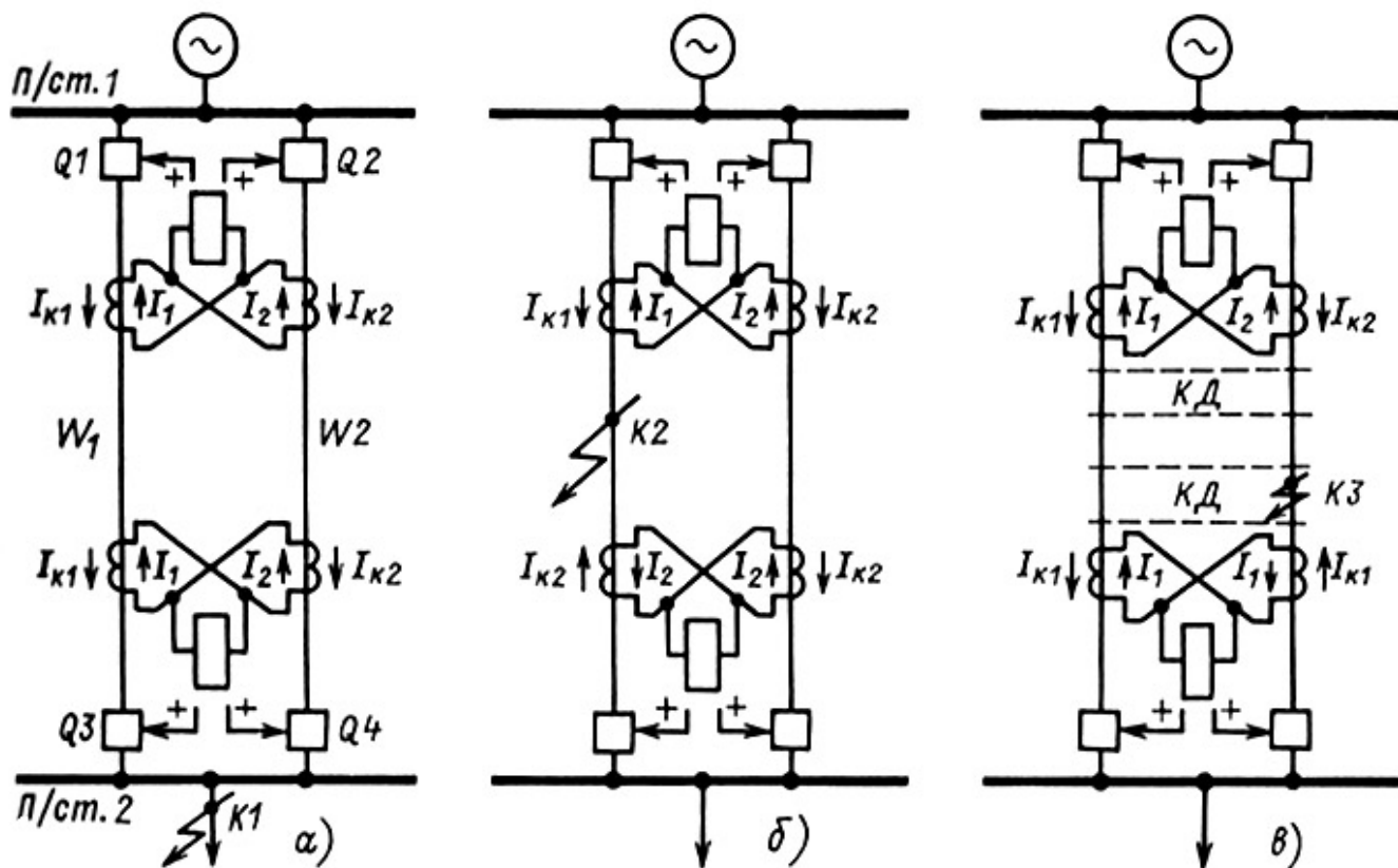
Рис. 7.22. Распределение тока в схемах поперечных токовых направленных защит при КЗ: а - во внешней сети; б - в зоне действия защиты; в - в зоне каскадного действия; КД - зона каскадного действия
