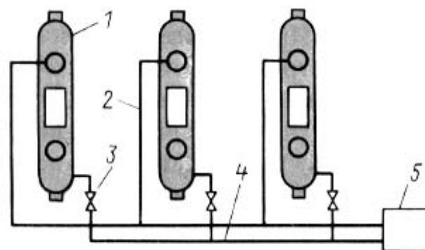
Рис. 3.8. Схема соединения распределительного шкафа с выключателем серии ВВБ:
