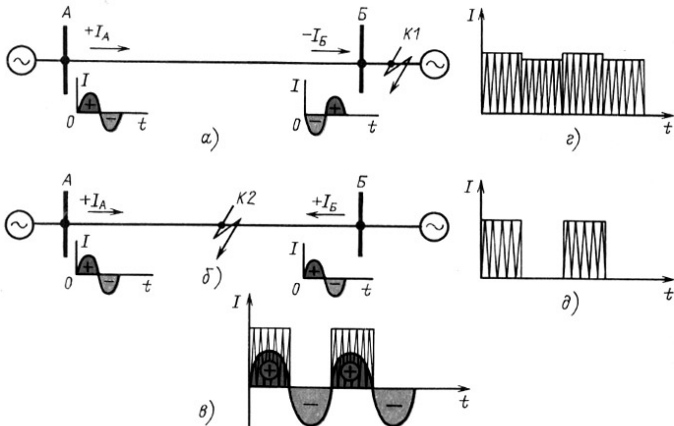
Рис. 7.24. Сравнение защитных высокочастотных сигналов при КЗ:
