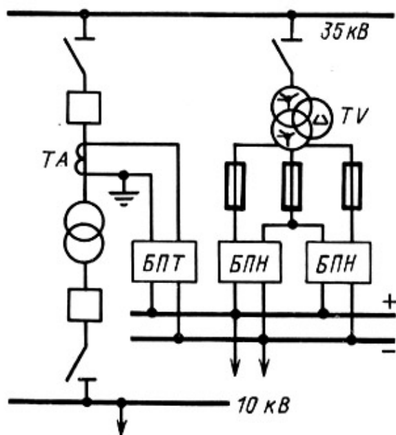
Рис. 6.2. Принципиальная схема комбинированного питания оперативных цепей
