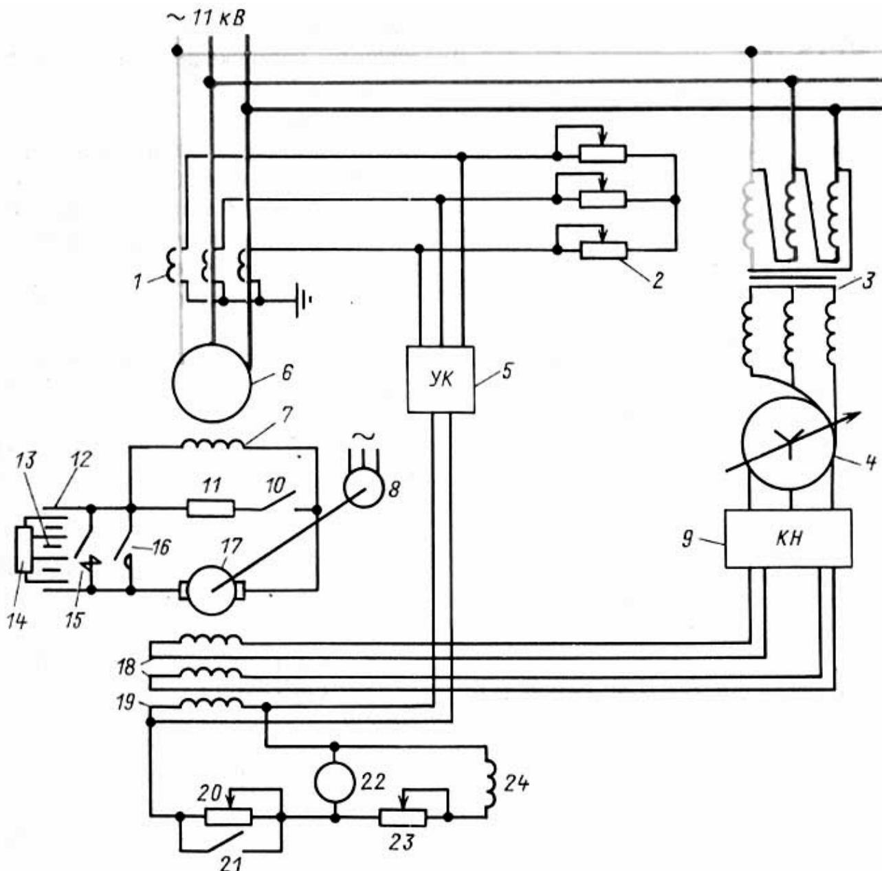
Рис. 2.6. Принципиальная схема машинного возбуждения синхронного компенсатора мощностью 50 МВ·А:
