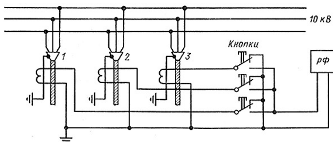
Рис. 10.3. Схема сигнализации замыкания на землю с применением разделительного фильтра (РФ): 1-3 - отходящие кабельные линии
