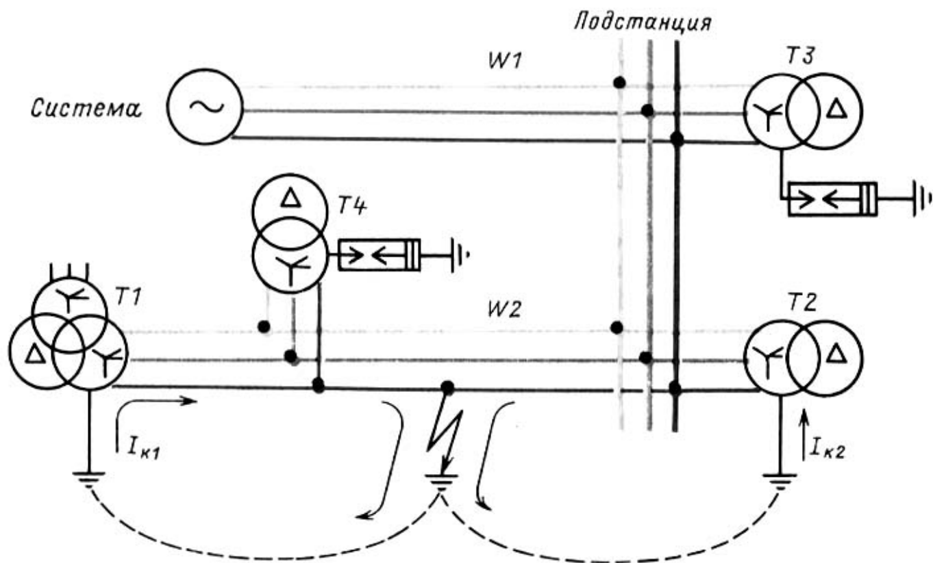
Рис. 1.19. Однофазное короткое замыкание в сети с эффективным заземлением нейтрали.
