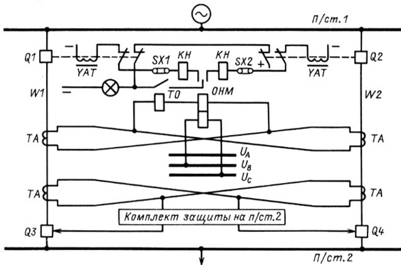
Рис. 7.21. Принципиальная схема поперечной токовой направленной защиты двух параллельных линий
