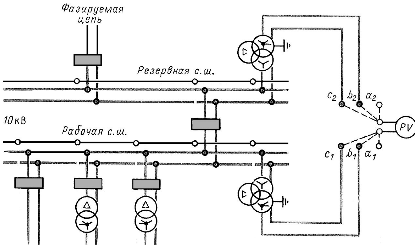
Рис. 8.9. Схема фазировки косвенным методом на выводах вторичных обмоток шинных трансформаторов напряжения
