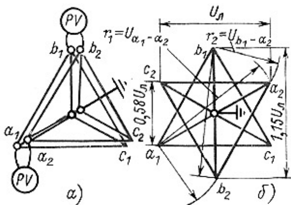
Рис. 8.4. Векторные диаграммы напряжений обмоток НН фазированных трансформаторов при совпадении фаз (а) и при сдвиге векторов на 180^\circ , например, при группах соединений \Delta/Y_H - II и \Delta/Y_H - 5 (б)
