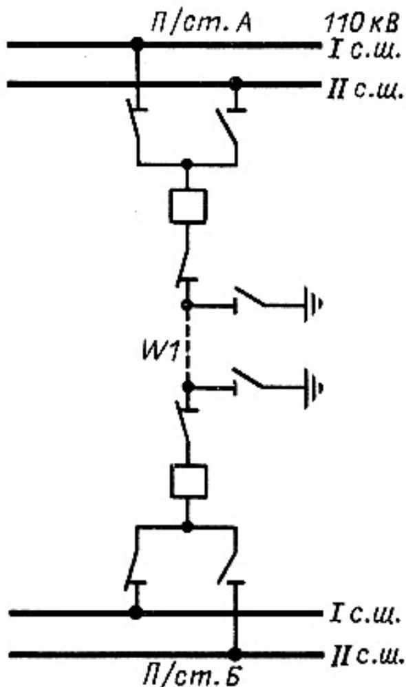
Рис. 9.1. Схема включенной в работу линии 110 кВ
