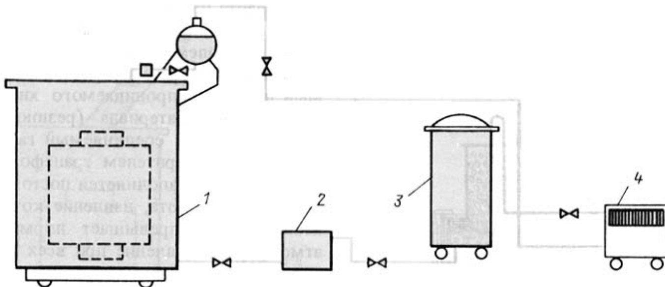
Рис. 1.24. Схема установки для регенерации масла в трансформаторе, находящемся в работе: 1 - трансформатор; 2 - маслоподогреватель; 3 - адсорбер; 4 - фильтр-пресс
