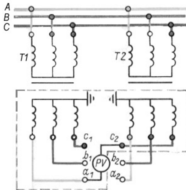
Рис. 8.3. Схема фазировки двух трансформаторов, имеющих заземленные нулевые точки вторичных обмоток (штриховой линией показан путь прохождения тока через прибор при несовпадении фаз)
