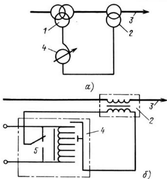
Рис. 1.13. Схема регулирования напряжения при помощи последовательного регулировочного трансформатора (а) и схема регулировочного автотрансформатора (б): 1 — главный трансформатор без РПН; 2 — последовательный регулировочный трансформатор; 3 — линия, в которой регулируется напряжение; 4 — регулировочный автотрансформатор; 5 — реверсор
