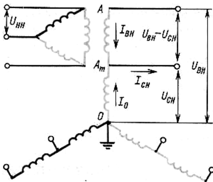
Рис. 1.1. Принципиальная схема трехфазного автотрансформатора
