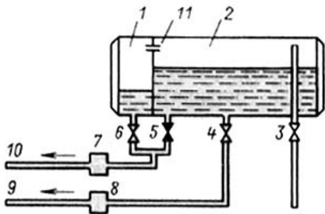
Рис. 1.17. Подключение расширителя для компенсации температурных изменений объема масла в трансформаторе и баке контактора РПН: 1 - малый отсек расширителя; 2 - большой отсек расширителя; 3 - кран для доливки масла в расширитель; 4 - кран маслопровода к баку трансформатора; 5 - кран подпитки маслом масляного отсека (кран нормально закрыт, на рисунке изображение крана зачернено); 6 - кран маслопровода к баку контактора; 7 - газовое реле РПН; 8 - то же трансформатора; 9 - маслопровод к баку трансформатора; 10 - то же к баку РПН; 11 - отверстие
