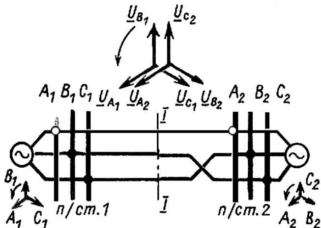
Рис. 8.10. Изменение порядка чередования фаз на линии при включении на параллельную работу двух электроустановок, имеющих прямой и обратный порядок следования фаз
