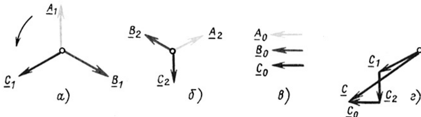
Рис. 7.9. Симметричные составляющие:
