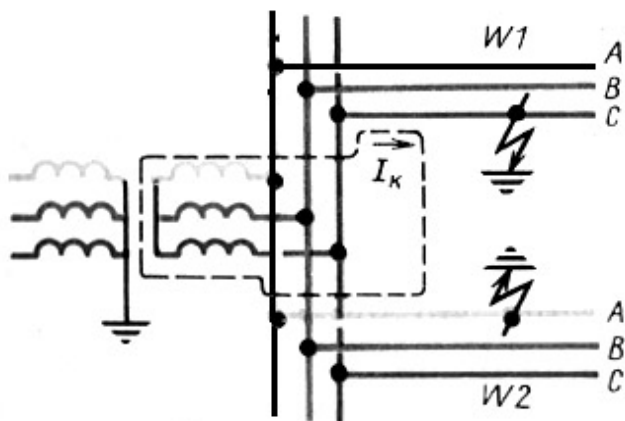
Рис. 7.3. Замыкание двух фаз на землю в сети с изолированной нейтралью приводит к КЗ. Штриховой линией показан путь тока КЗ
