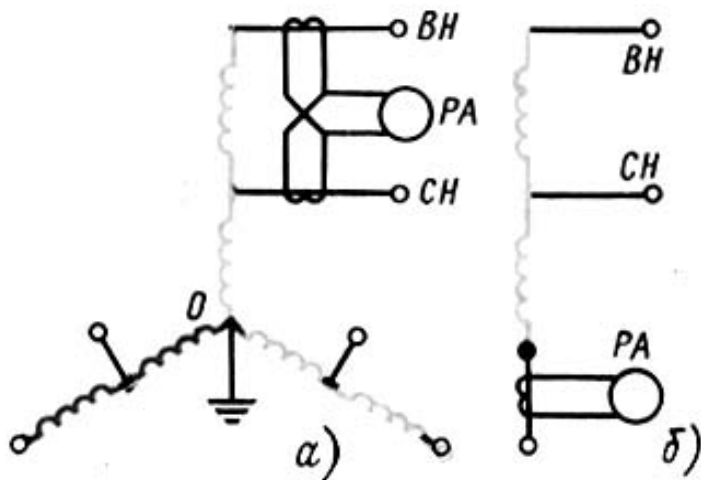
Рис. 1.2. Схема включения амперметра для измерения тока в общей обмотке автотрансформатора: а - трехфазного; б - однофазного
