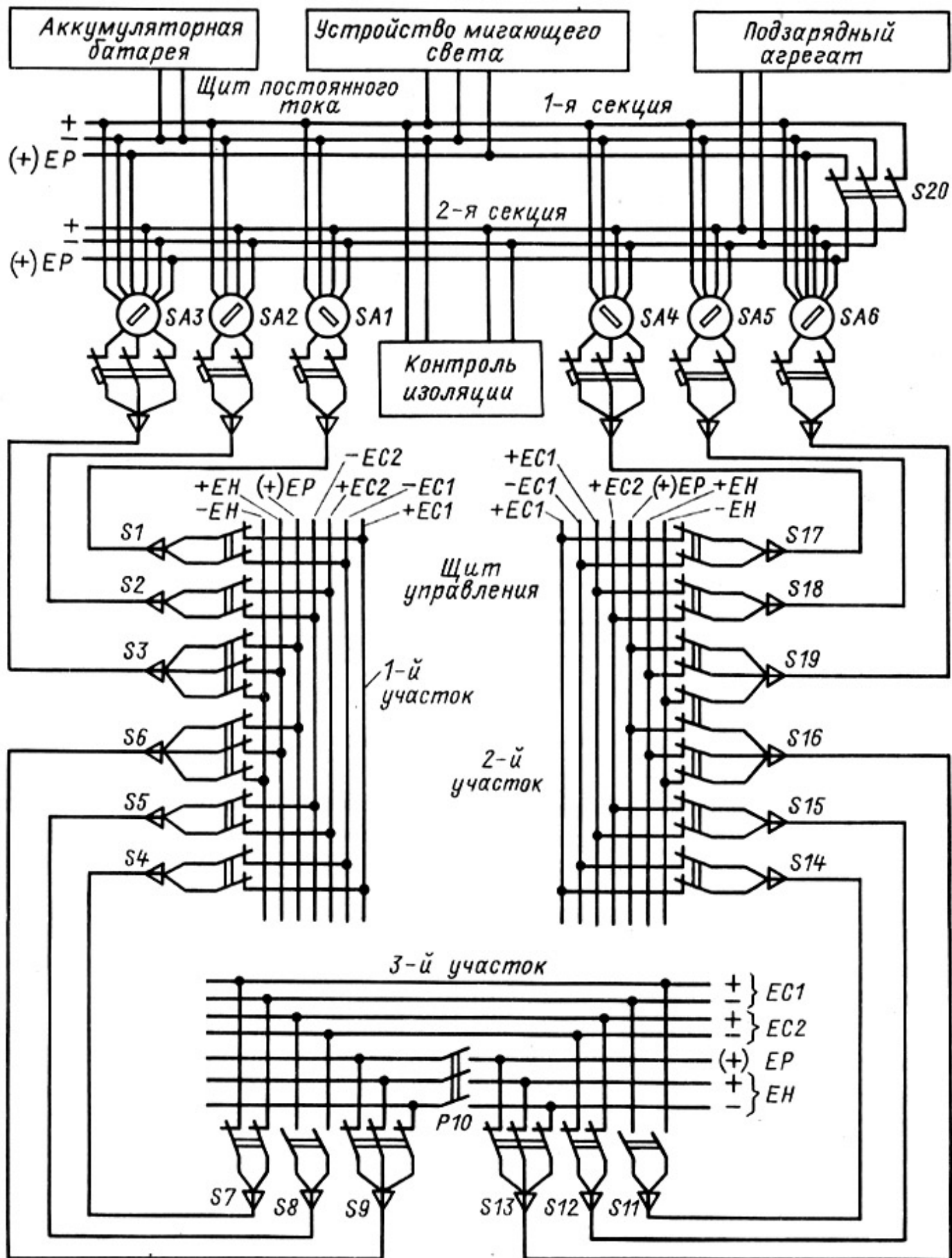
Рис. 6.11. Схема питания цепей управления и сигнализации подстанции:
