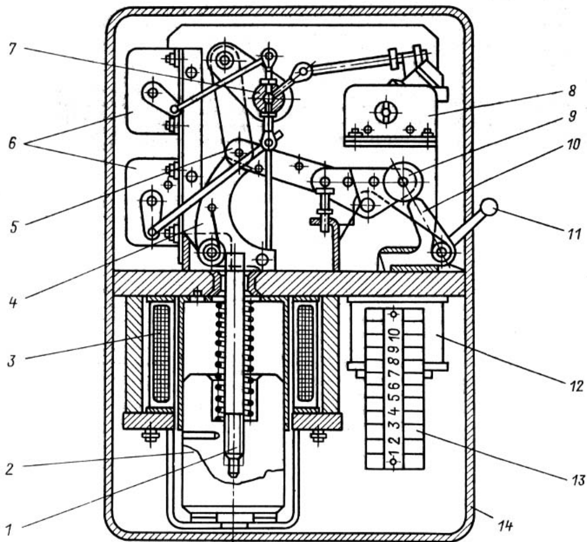
Рис. 3.1. Привод электромагнитный для маломасляных выключателей:
