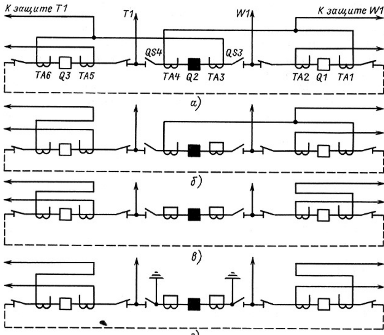
Рис. 9.13. Последовательность операций при выводе в ремонт выключателя в схеме кольцевого типа: а - отключение выводимого в ремонт выключателя Q2; б - вывод из схемы защит и автоматики трансформатора T1 токовых цепей от трансформаторов тока TA3; в - то же линии W1 от трансформатора тока TA4; г - подготовка выключателя Q2 к ремонту
