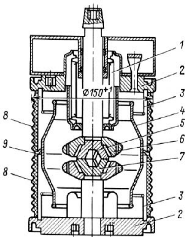
Рис. 3.12. Разрез вакуумной дугогасительной камеры 10 кВ: 1 - сильфон; 2 - фланец; 3 - электростатический экран, имеющий потенциал ввода; 4 - электростатический экран, находящийся под свободным потенциалом; 5 - подвижный контакт; 6 - дугогасящий электрод; 7 - неподвижный контакт; 8 - керамический изолятор камеры; 9 - металлическая прокладка
