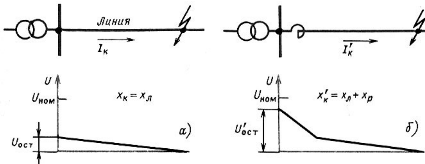
Рис. 4.12. Ограничение тока короткого замыкания и поддержание напряжения на шинах подстанции при помощи реактора: а - при отсутствии реактора; б - при наличии реактора
