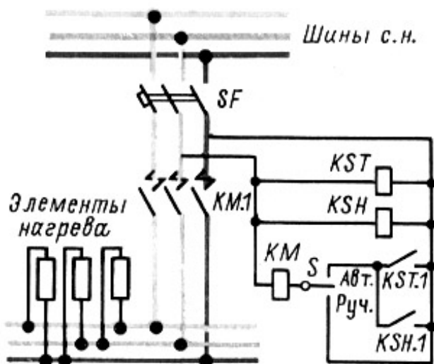
Рис. 5.7. Схема устройства для сушки воздуха и отопления в шкафах КРУ:
