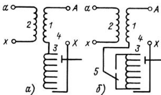
Рис. 1.11. Схемы регулирования на трансформаторах без реверсирования (а) и с реверсированием (б) регулировочной обмотки: 1, 2 — первичная и вторичная обмотки соответственно; 3 — регулировочная обмотка с отведениями; 4 — переключающее устройство; 5 — реверсор
