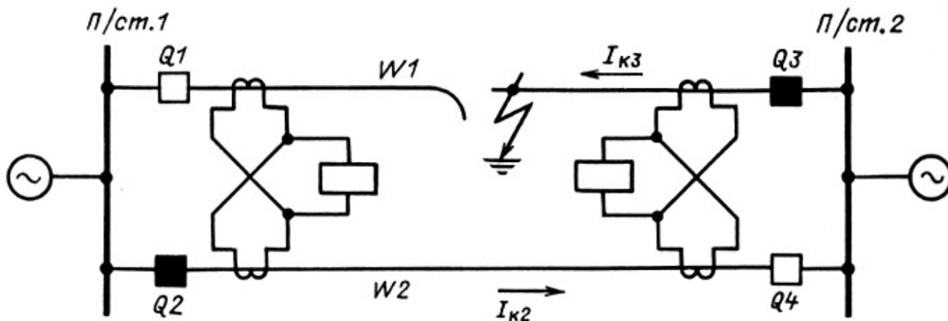
Рис. 7.23. Срабатывание защиты при обрыве провода линии с односторонним КЗ на землю
