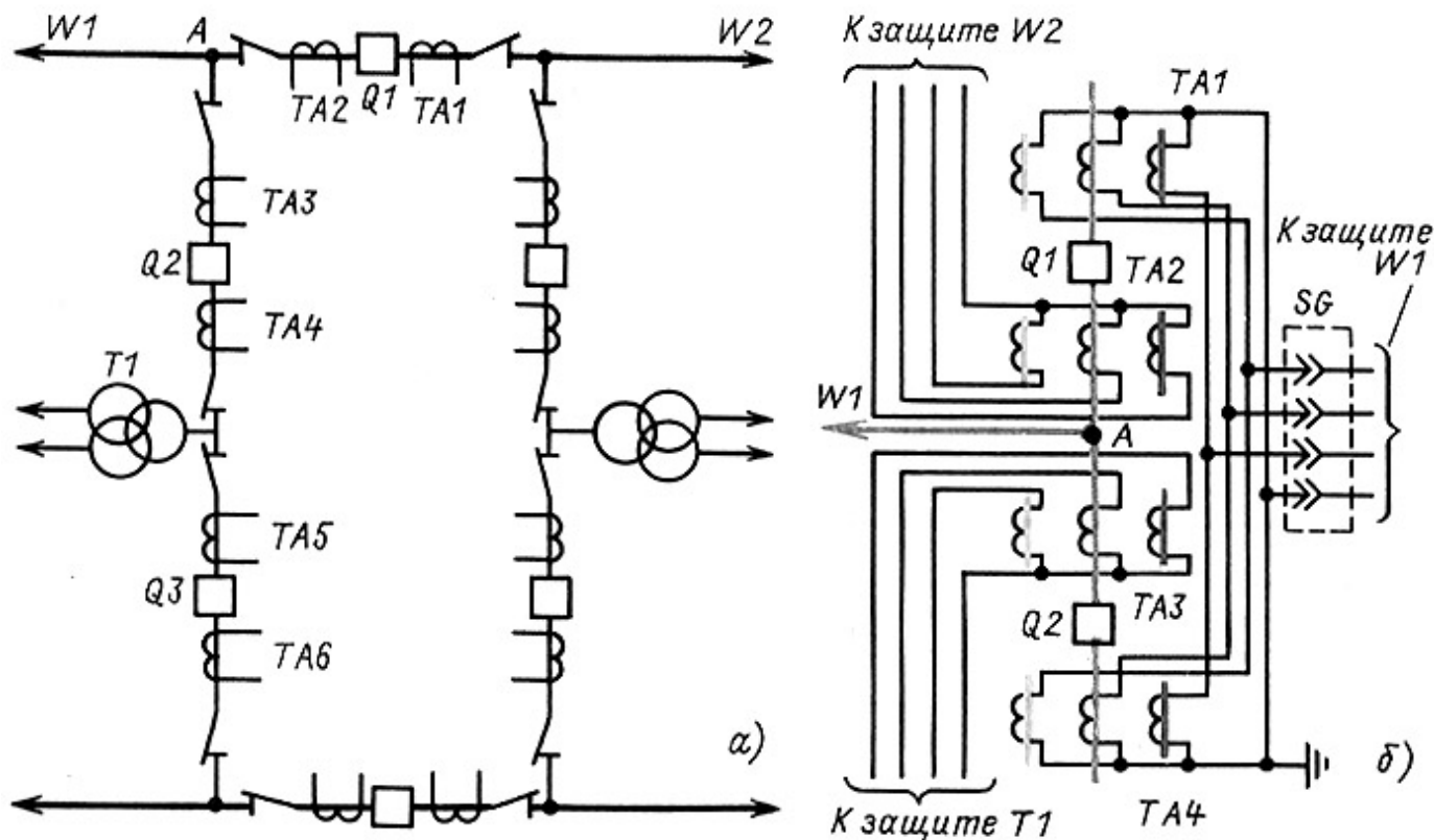
Рис. 9.12. Схема подстанции кольцевого типа (шестиугольник): а - схема первичных соединений; б - схема включения защит электрических цепей
