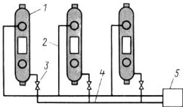
Рис. 3.10. Схема соединения распределительного шкафа с выключателем серии ВВБ:
