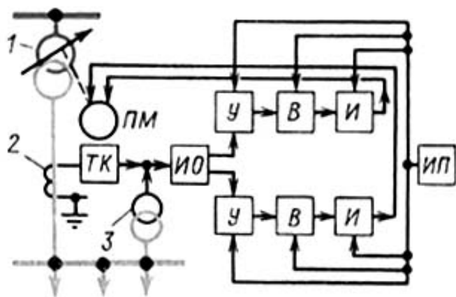
Рис. 1.18. Структурная схема автоматического регулирования напряжения: 1 - регулируемый трансформатор; 2 - трансформатор тока; 3 - трансформатор напряжения; ТК - устройство токовой компенсации; ИО - измерительный орган; У - орган управления; В - орган выдержки времени; И - исполнительный орган; ИП - источник питания; ПМ - приводной механизм
