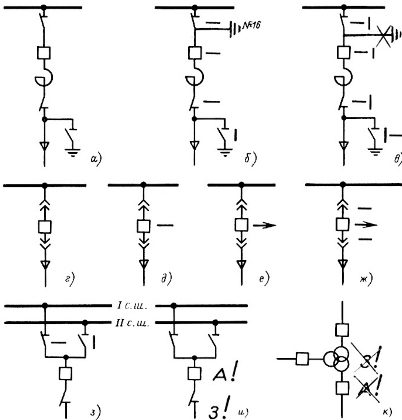
Рис. 12.2. Примеры нанесения условных знаков на оперативных схемах подстанций:
