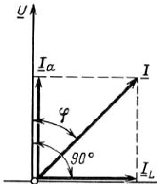
Рис. 2.1. Разложение вектора полного тока на активную и реактивную составляющие
