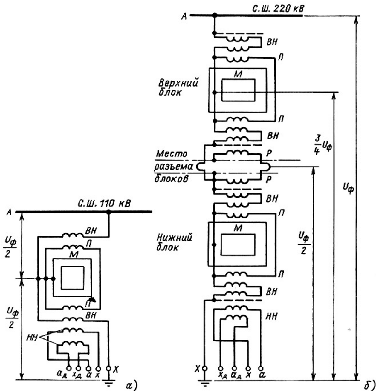
Рис. 4.1. Схемы трансформаторов напряжения типов НКФ-110 (а), НКФ-220 (б):
