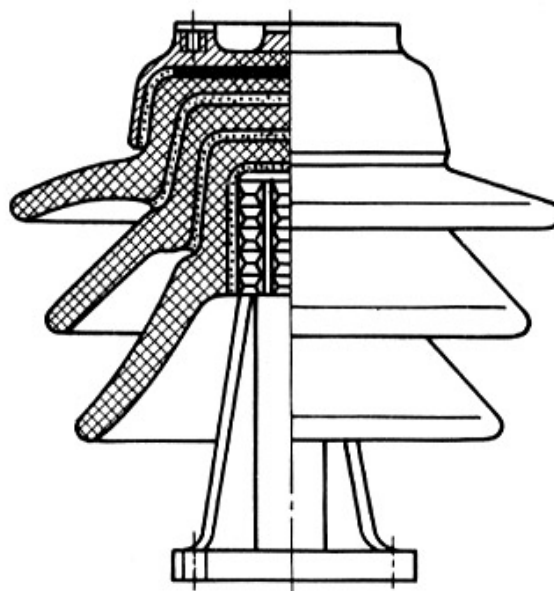
Рис. 5.3. Опорно-штыревой изолятор на напряжение 35 кВ серии ОНШ
