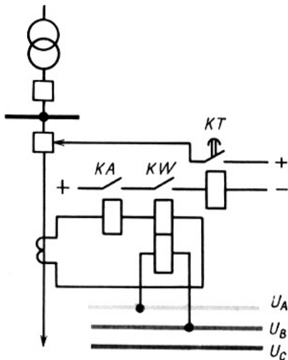
Рис. 7.7. Принципиальная схема максимальной направленной защиты линии:
