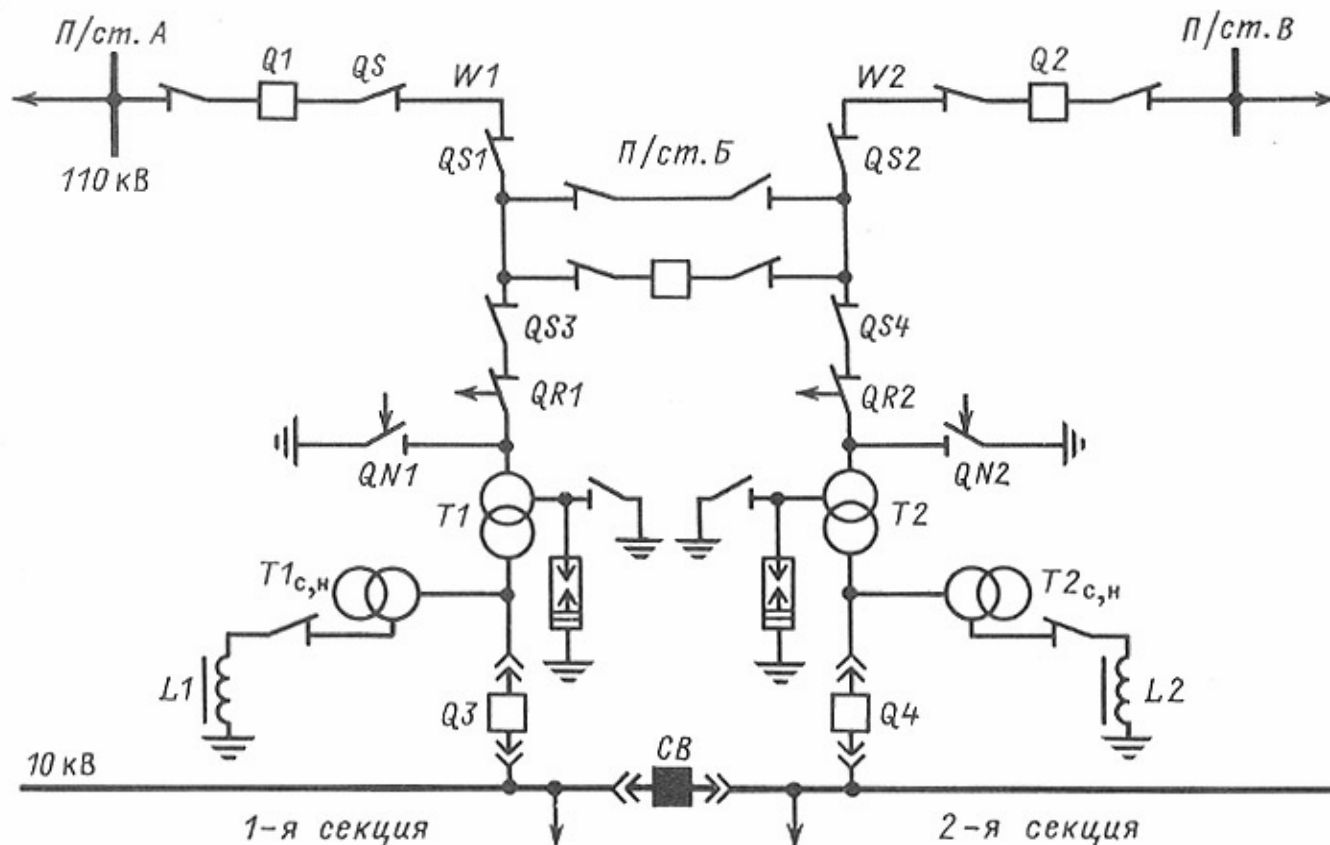
Рис. 9.5. Схема двух блоков с отделителями и неавтоматической перемычкой со стороны линий
