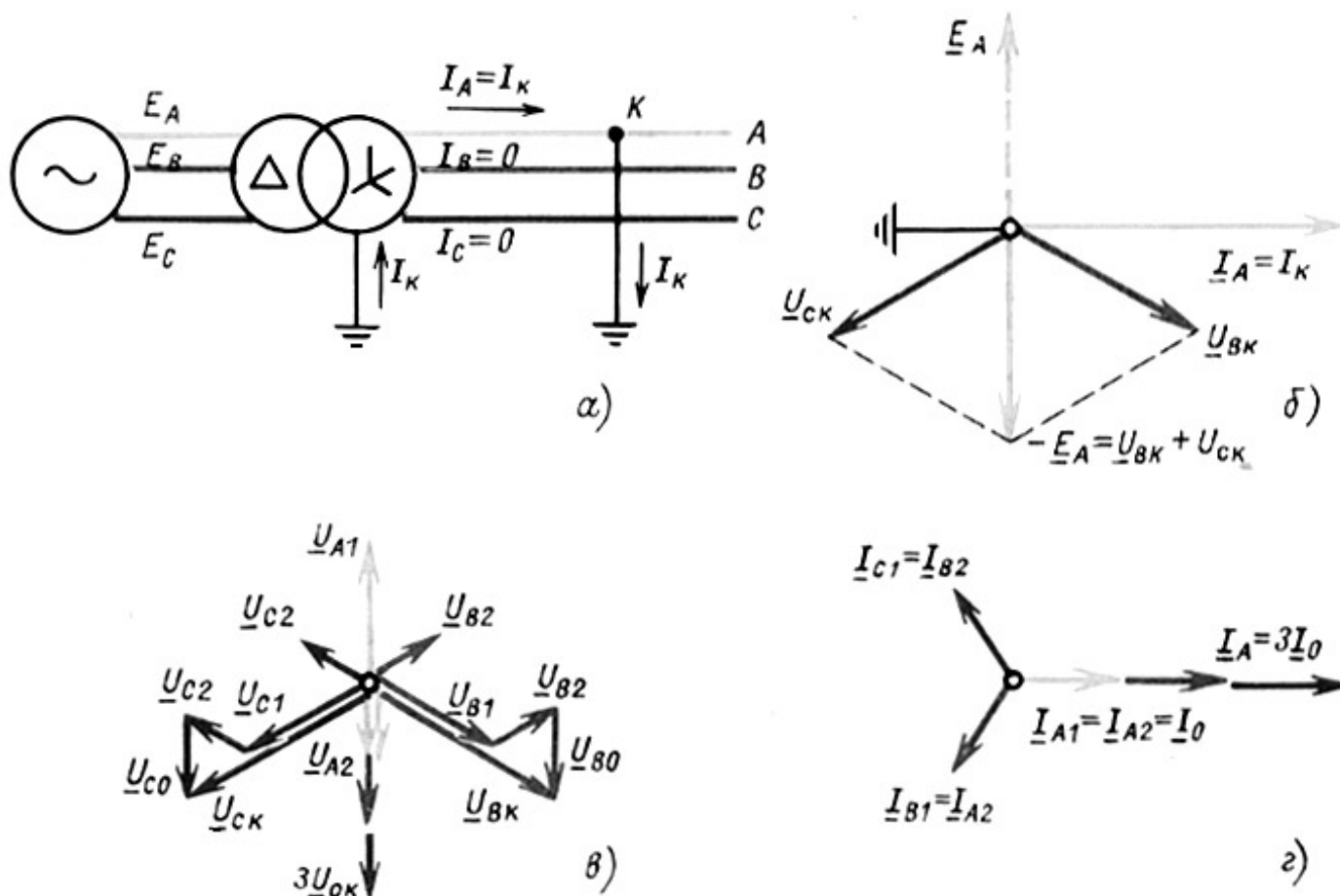
Рис. 7.10. Однофазное КЗ на землю на ненагруженной линии с односторонним питанием:
