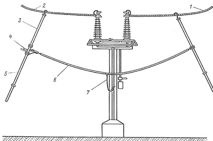
Рис. 8.8. Фазировка прямым методом индикатором Ленэнерго:
