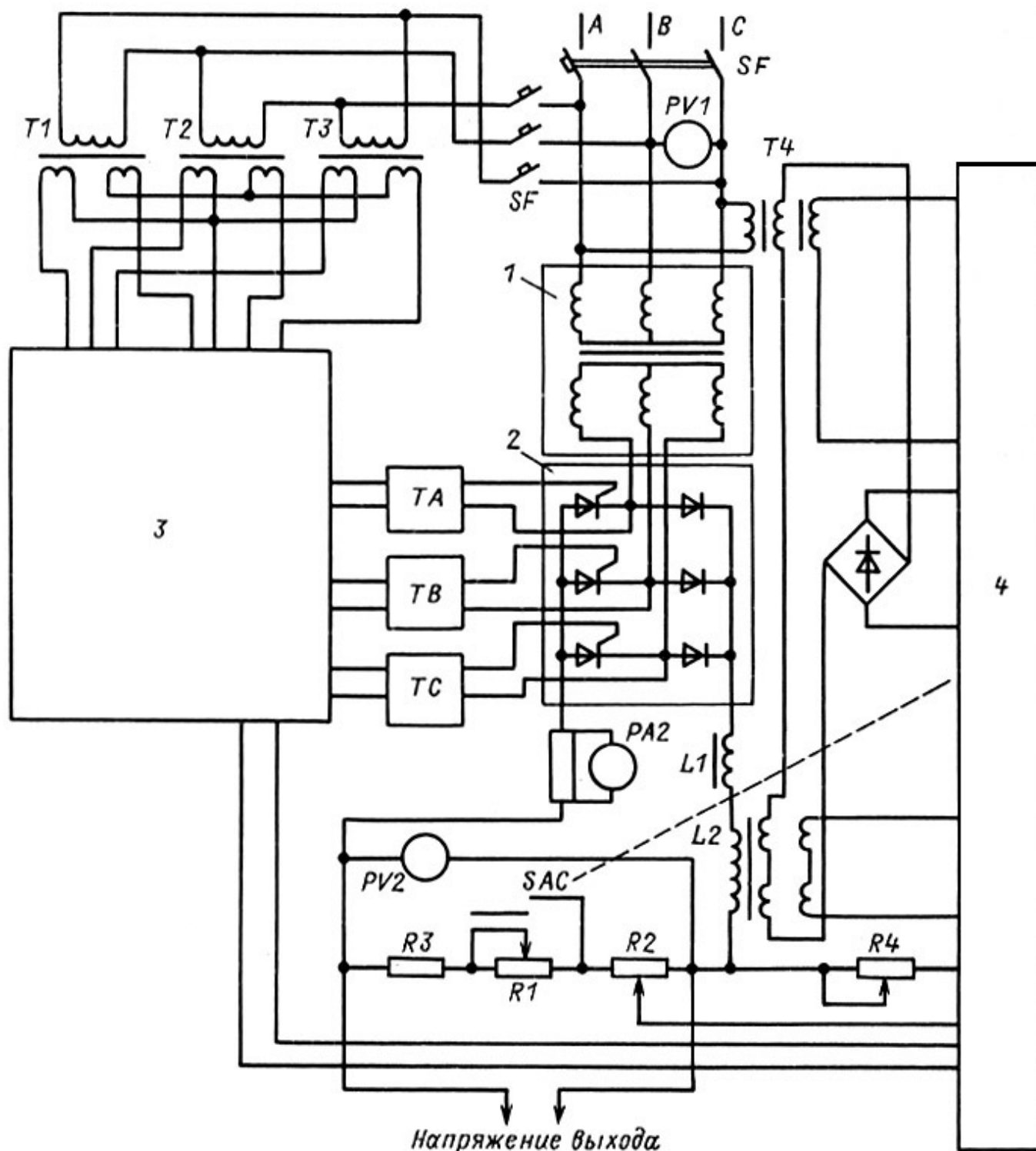
Рис. 6.7. Упрощенная структурная схема выпрямительного зарядно-подзарядного агрегата ВАЗП-380/220-40/80:
