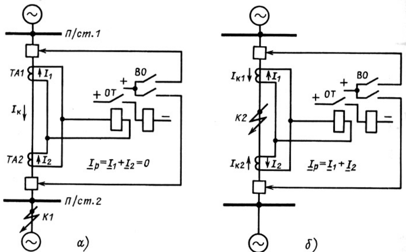
Рис. 7.17. Принцип выполнения продольной дифференциальной защиты линии и прохождение тока в органе тока при внешнем КЗ (а) и при КЗ в защищаемой зоне (б)
