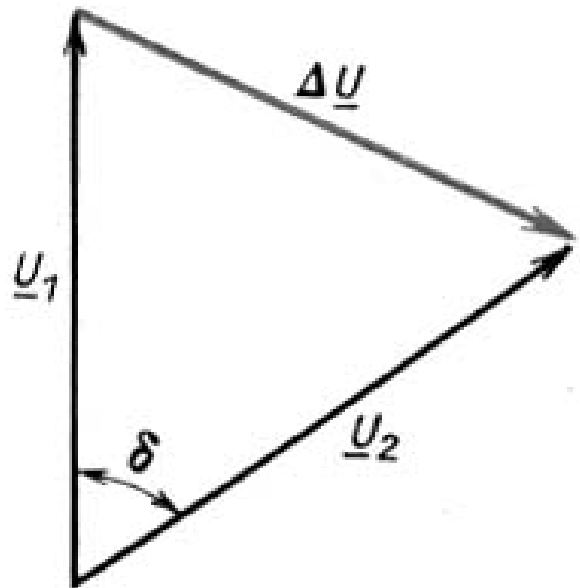
Рис. 1. 8. Разность напряжений \Delta U при сдвиге векторов вторичных напряжений U_1 и U_2 по фазе на угол \delta
