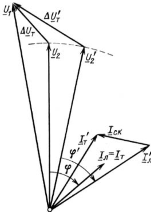
Рис. 2.5. Поддержание неизменного уровня напряжения на шинах подстанции при изменении тока нагрузки потребителей
