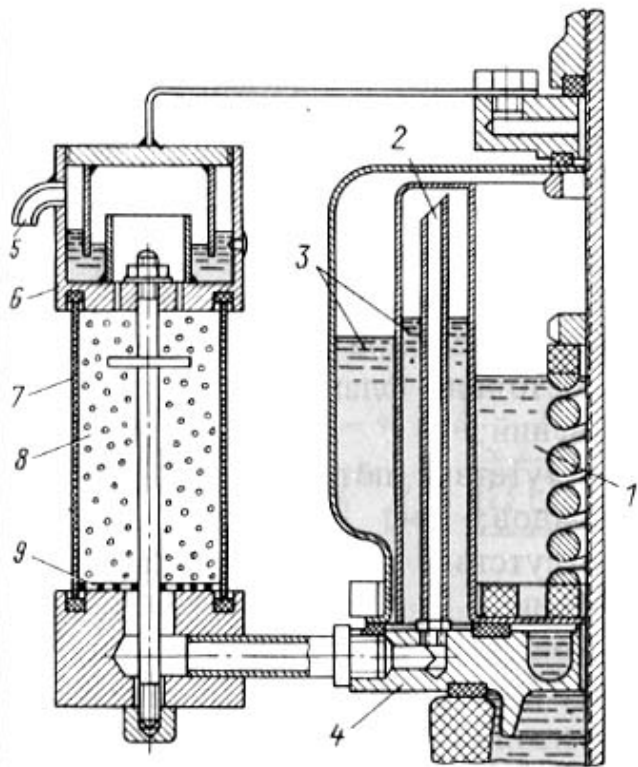
Рис. 1.27. Расширитель масляного ввода 110 кВ: 1 - масло во вводе; 2 - дыхательная трубка масляного затвора ввода; 3 - масло в затворе; 4 - поддон; 5 - дыхательная трубка воздухоочистителя; 6 - масляный затвор воздухоочистителя; 7 - стеклянная трубка; 8 - силикагель; 9 - сетка
