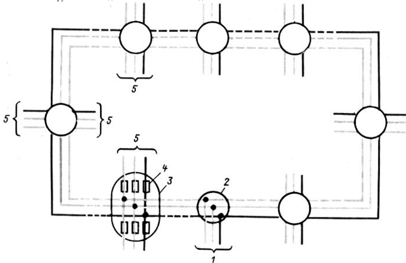
Рис. 1.6. Схема питания электродвигателей вентиляторов системы охлаждения Д
