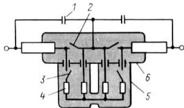
Рис. 3.9. Принципиальная электрическая схема выключателя серии ВВБ:
