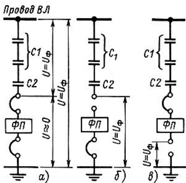
Рис. 4.9. Схема распределения потенциалов в цепи 50 Гц конденсаторов связи:
