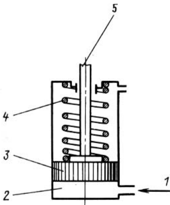
Рис. 3.4. Принципиальная схема поршневого пневматического блока одностороннего действия:
