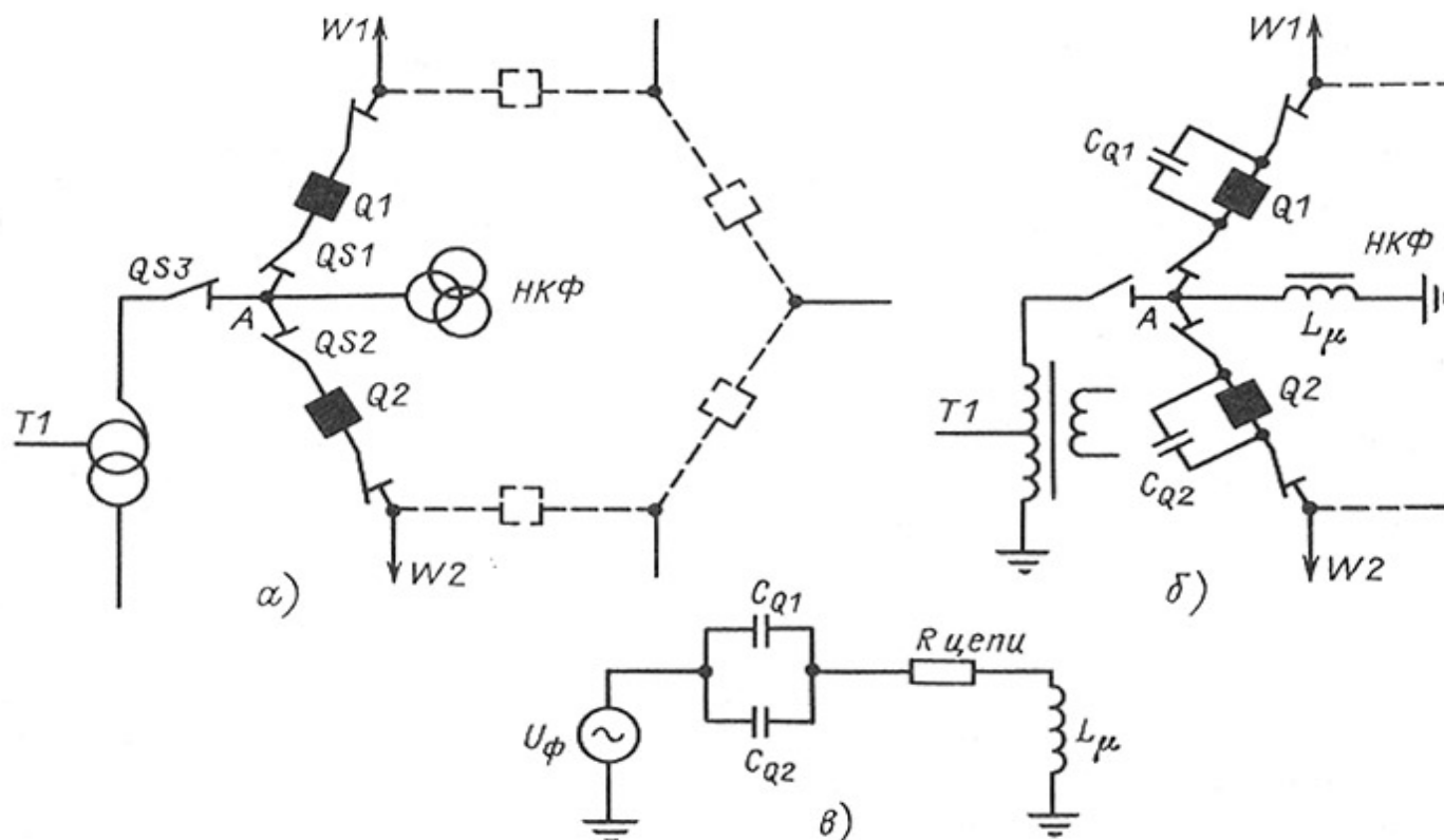
Рис. 10.5. Образование феррорезонансного контура при отключении автотрансформатора: а - положения коммутационных аппаратов; б - электрические элементы контура; в - схема замещения
