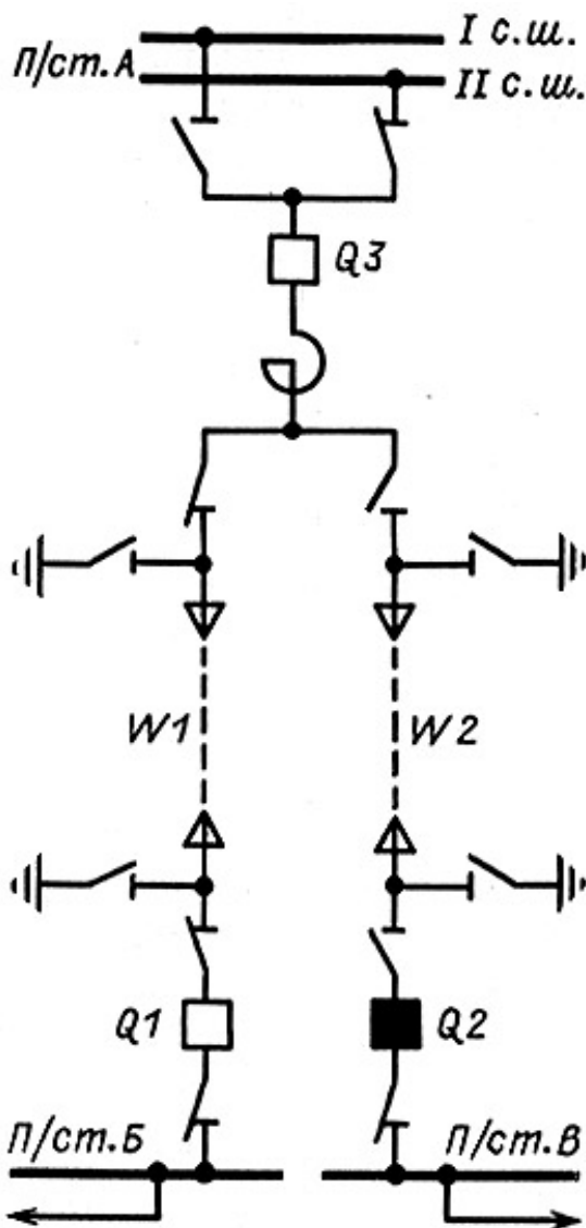
Рис. 9.3. Схема спаренных кабельных линий, находящихся в различных оперативных состояниях: линия W1 включена; линия W2 отключена
