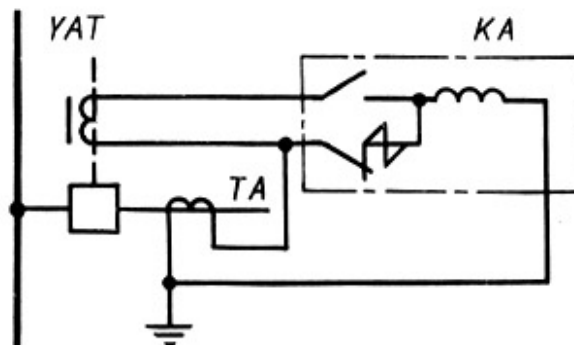
Рис. 6.1. Схема питания оперативных цепей от трансформатора тока
