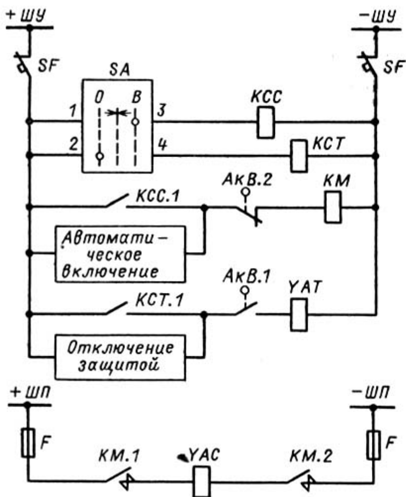
Рис. 3.3. Схема управления выключателем с электромагнитным приводом
