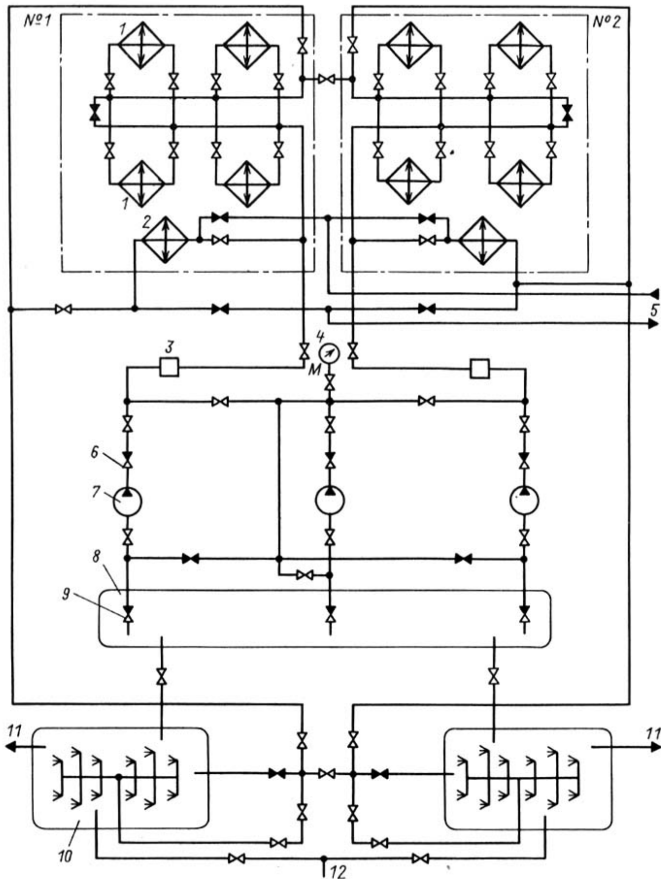
Рис. 2.10. Схема водоснабжения двух синхронных компенсаторов серии КСВ:
