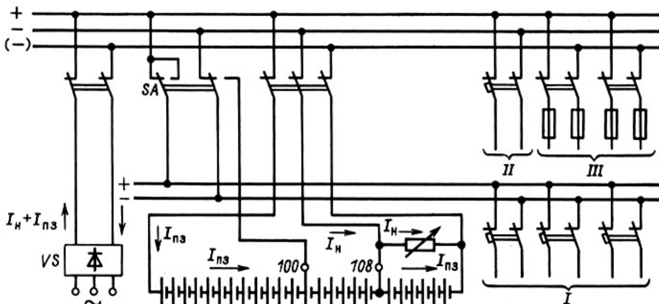
Рис. 6.9. Схема аккумуляторной установки без элементарного коммутатора, работающей в режиме постоянного подзаряда:
