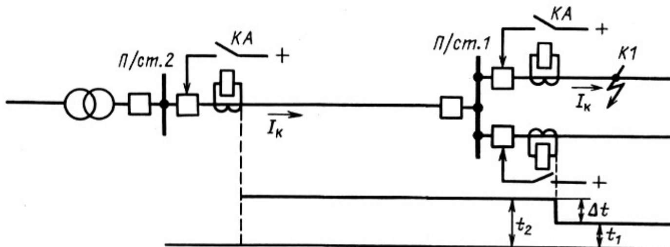
Рис. 7.5. Применение максимальных токовых защит в сети с односторонним питанием
