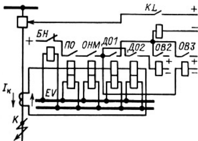
Рис. 7.16. Принципиальная схема дистанционной защиты со ступенчатой характеристикой выдержки времени
