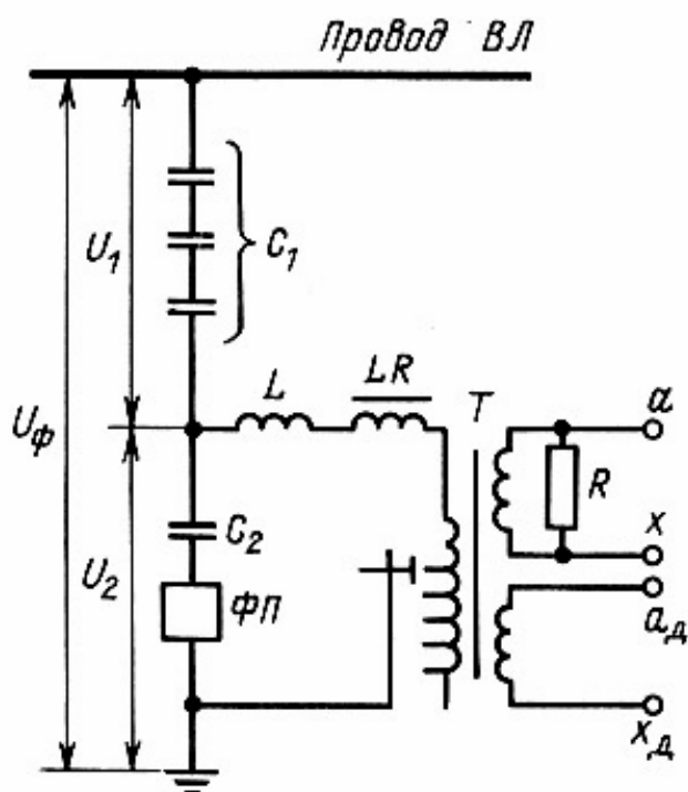
Рис. 4.2. Схема включения емкостного делителя напряжения типа НДЕ-500
