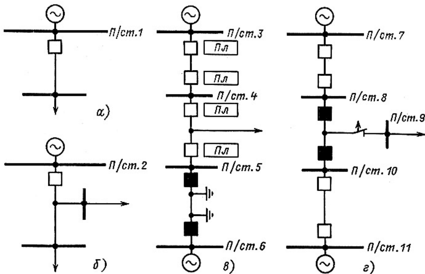
Рис. 11.1. Схемы линий с односторонним и двухсторонним питанием:
