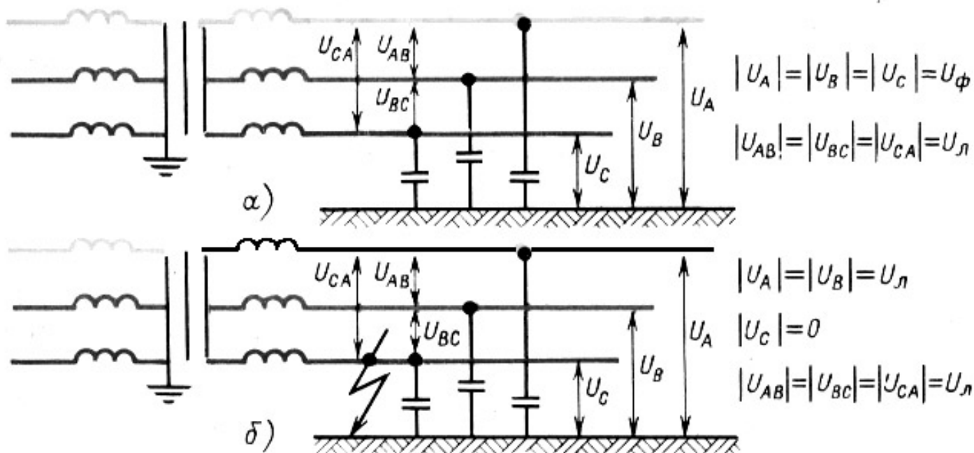
Рис. 7.2. Нормальный (а) и утяжеленный (б) режимы работы электрической сети с изолированной нейтралью
