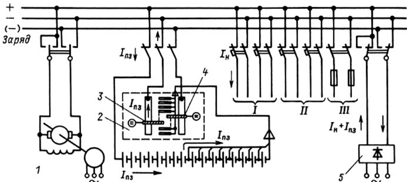
Рис. 6.8. Схема аккумуляторной установки с элементарным коммутатором:
