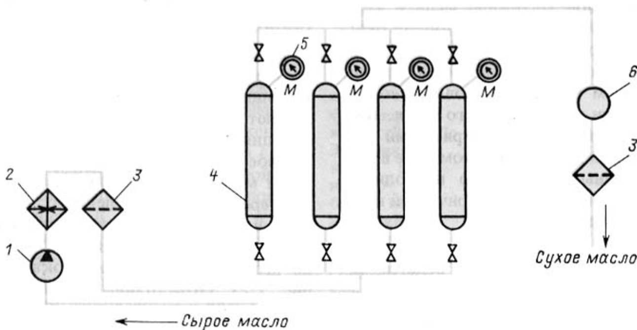
Рис. 1.23. Схема цеолитовой установки для осушки масла: 1 - маслonaсос; 2 - маслоподогреватель; 3 - фильтр механической очистки; 4 - цеолитовый фильтр-адсорбер; 5 - манометр; 6 - расходомер
