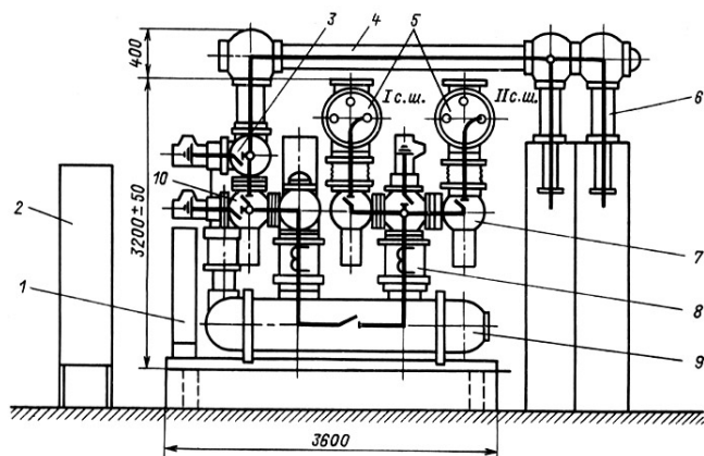
Рис. 5.8. Полус ячейки КРУЭ 110 кВ со схемой электрических соединений
