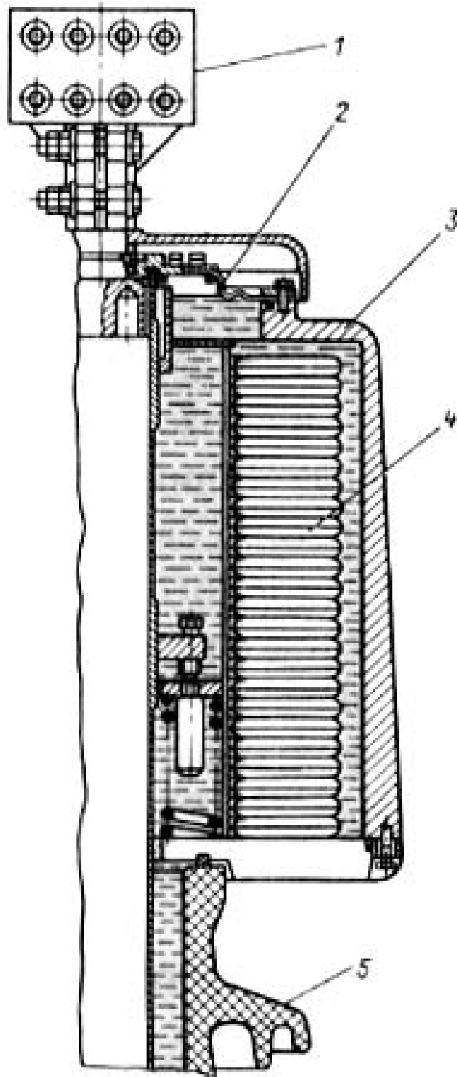
Рис. 1.28. Размещение сифона в расширителе герметичного ввода конденсаторного типа: 1 - контактный зажим ввода; 2 - защитная мембрана; 3 - корпус расширителя; 4 - металлический герметичный сифон, заполненный инертным газом; 5 - фарфоровая крышка ввода
