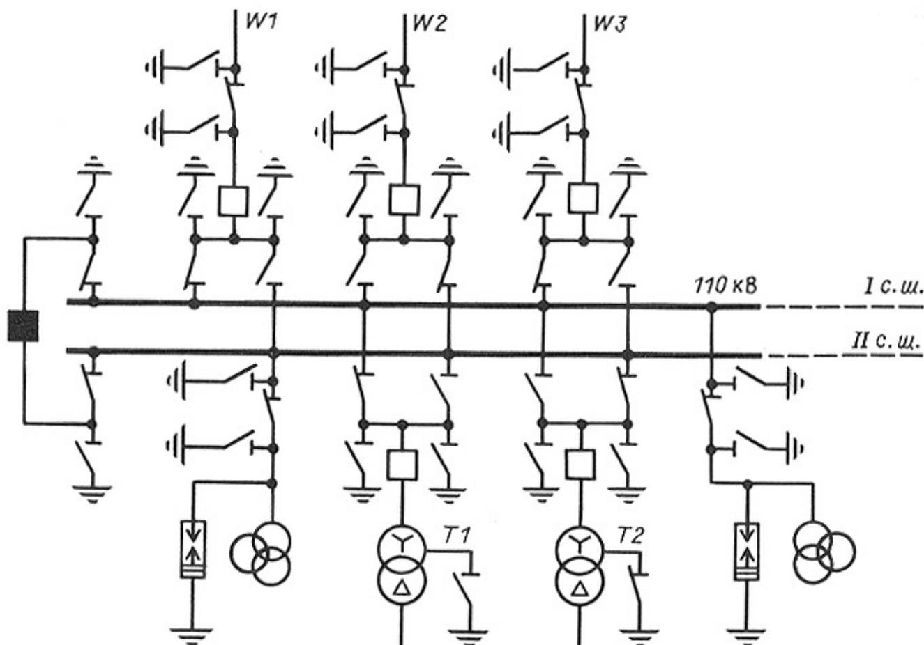
Рис. 9.7. Схема РУ 110 кВ с двумя рабочими системами шин
