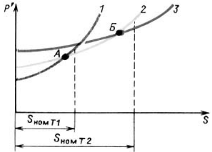
Рис. 1. 9. Кривые приведенных потерь трансформаторов: 1 - для трансформатора T1 ; 2 - для T2 ; 3 - для обоих трансформаторов, включенных параллельно
