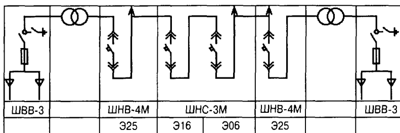
Рис. 7.9. Однолинейные схемы КТП с выходом на магистраль [выключатели «Электрон»: Э06, Э16, Э25, Э40; шкафы: высоковольтного (ШВВ) и низковольтного (ШНВ) вводов, секционный (ШНС) и низковольтный линейный (ШНЛ)]
