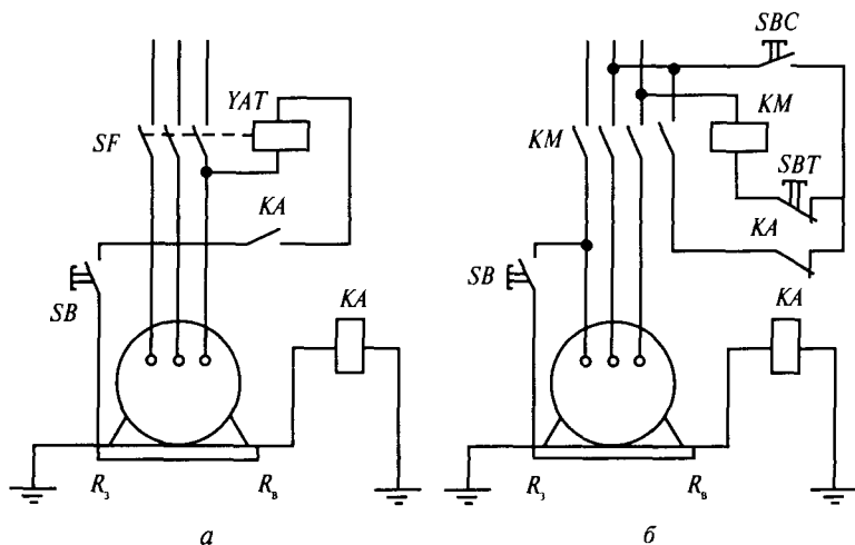
Рис. 16.7. Схемы защитного отключения при напряжении корпуса относительно земли:
