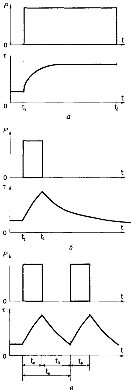
Рис. 3.1. График нагрузки и изменения температуры корпуса двигателя для продолжительного (а), кратковременного (б) и повторно-кратковременного (в) режимов работы
