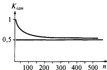
Рис. 3.8. График зависимости K_{\text{одн}} = f(n)
