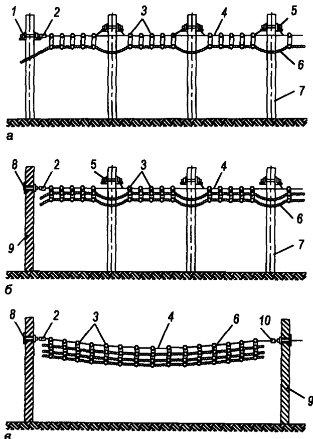
Рис. 8.14. Схемы прокладки кабелей на канате:
