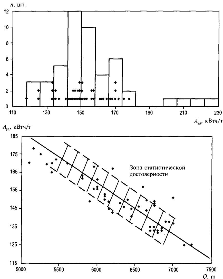
Рис. 18.1. Двухмесячные суточные расходы электроэнергии комплекса доменной печи во время неустойчивой работы:
