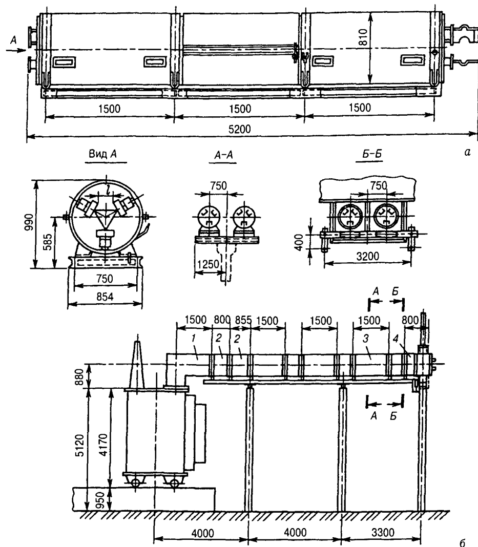
Рис. 8.19. Магистральный комплектный шинопровод
