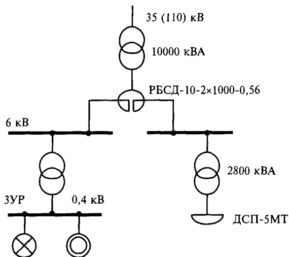
Рис. 5.14. Схема питания ДСП с использованием двояного реактора
