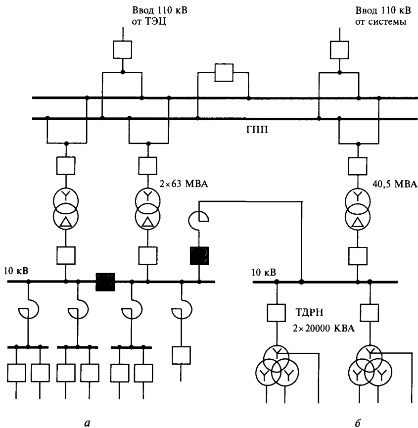
Рис. 5.10. Структурная схема электроснабжения блюминга 1300: а — общецеховые нагрузки; б — ионный привод
