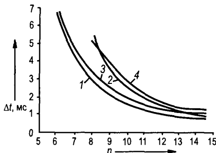
Рис. 14.22. Зависимости шага дискретизации от разрядности АЦП:
