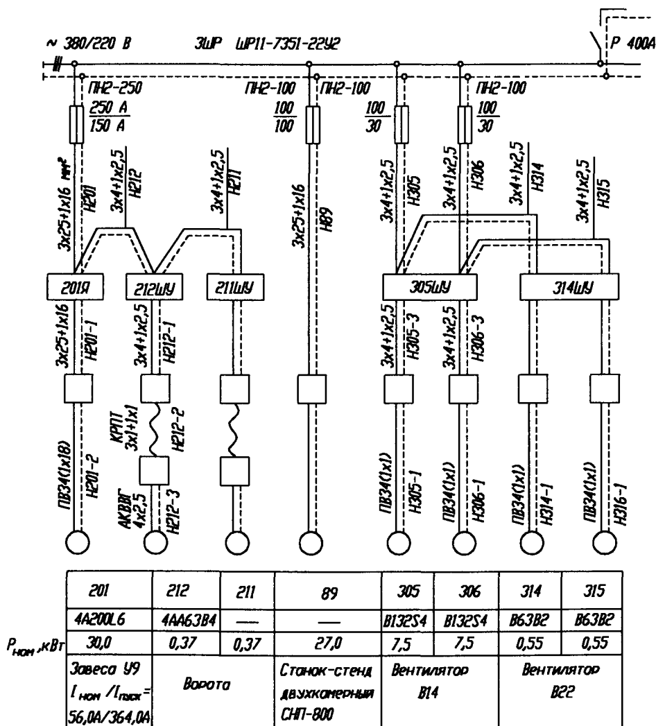
Рис 2.6. Однолинейная схема 2УР
