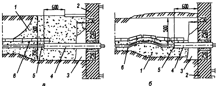
Рис. 8.9. Ввод кабеля через трубу в здания или кабельные сооружения
