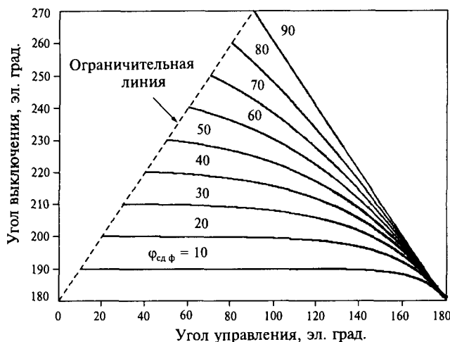
Рис. 6.4. Зависимости угла выключения тиристоров от угла управления и угла сдвига фаз ( \varphi_{сд\ \phi} ) нагрузки
