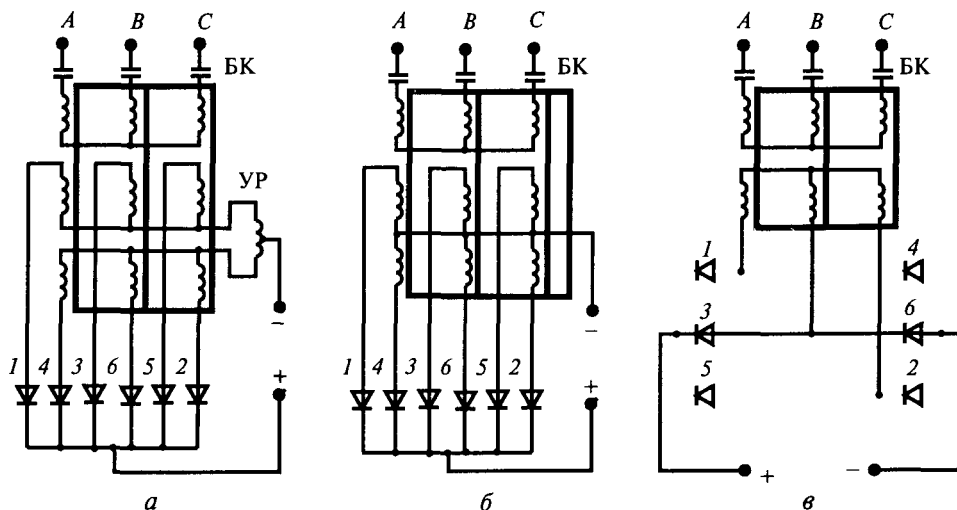
Рис. 6.21. Принципиальные схемы шестифазных СКП: а — нулевого с уравнивательным реактором; б — нулевого с дополнительным стержнем в магнитопроводе трансформатора; в — мостового
