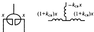
Рис. 9.2. Схема замещения сдвоенного реактора
