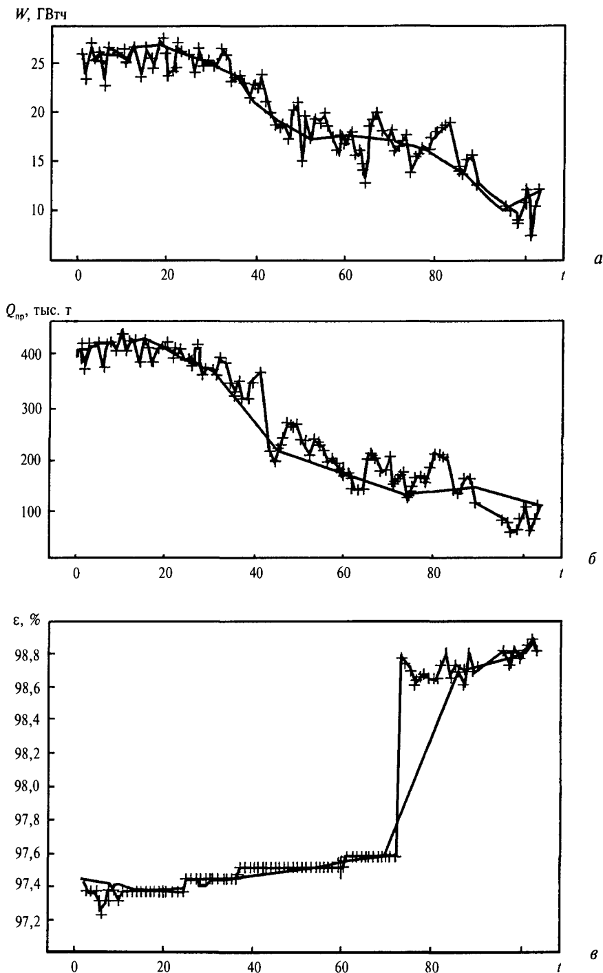
Рис. 17.1. Тенденции изменения месячного электропотребления (а), объема производства (б) и относительного обжата (в) листопрокатного цеха
