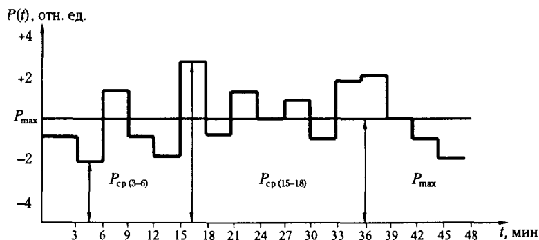
Рис. 3.4. График нагрузки P = f(t) с интервалом осреднения \Delta t = 3 мин:
