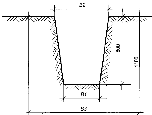
Рис. 8.3. Размеры траншеи для прокладки кабелей 1–10 кВ: B_1 — на дне траншеи; B_2 — размер у поверхности земли; B_3 — размер зоны отвода
