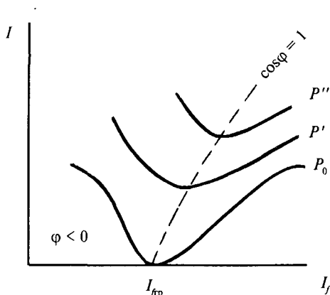
Рис. 13.3. U -образные характеристики синхронного генератора ( U_0 = \text{const} , активная нагрузка P = 0; P'; P'' )
