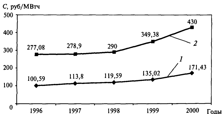
Рис. 18.10. Ценовые показатели электроэнергии:
