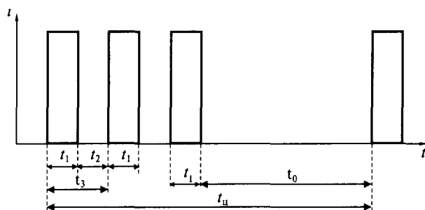
Рис. 3.3. График нагрузки сварочной машины: t_1 — время сварки, t_2 — пауза между сварочными импульсами, t_3 — цикл собственно сварки в автоматическом режиме, t_0 — время на замену детали, t_{\text{ц}} — цикл сварки
