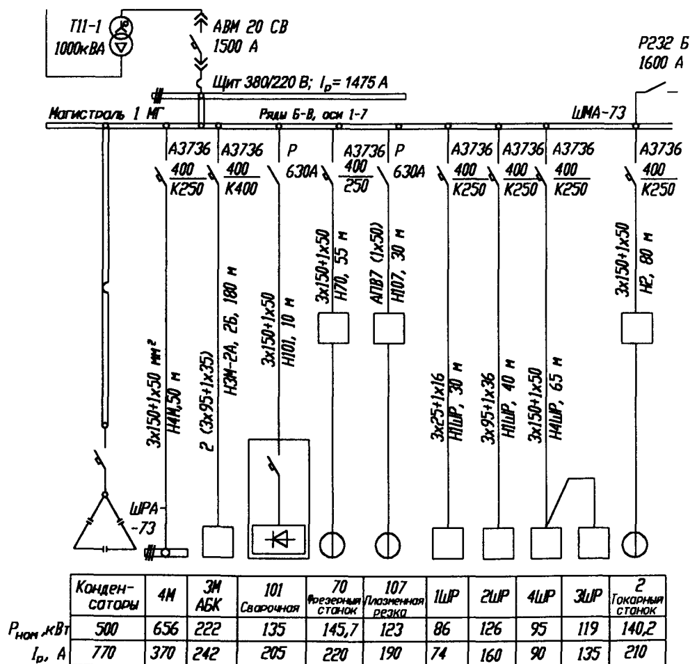
Рис. 2.5. Схема 0,4 кВ трансформаторной подстанции ЗУР с трансформаторами 2х1000 кВА
