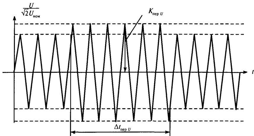
Рис. 21.8. Временное перенапряжение
