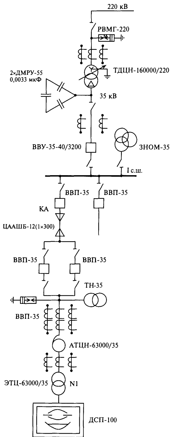
Рис.5.13. Схема электроснабжения крупного ЭСПЦ
