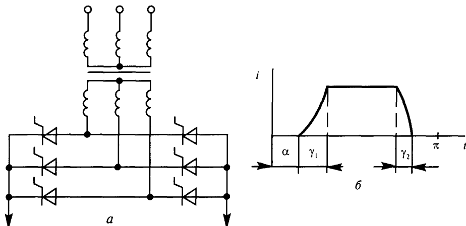
Рис. 13.6. Схема 6-пульсного ВП (а) и кривая тока в фазе ВП (б):
