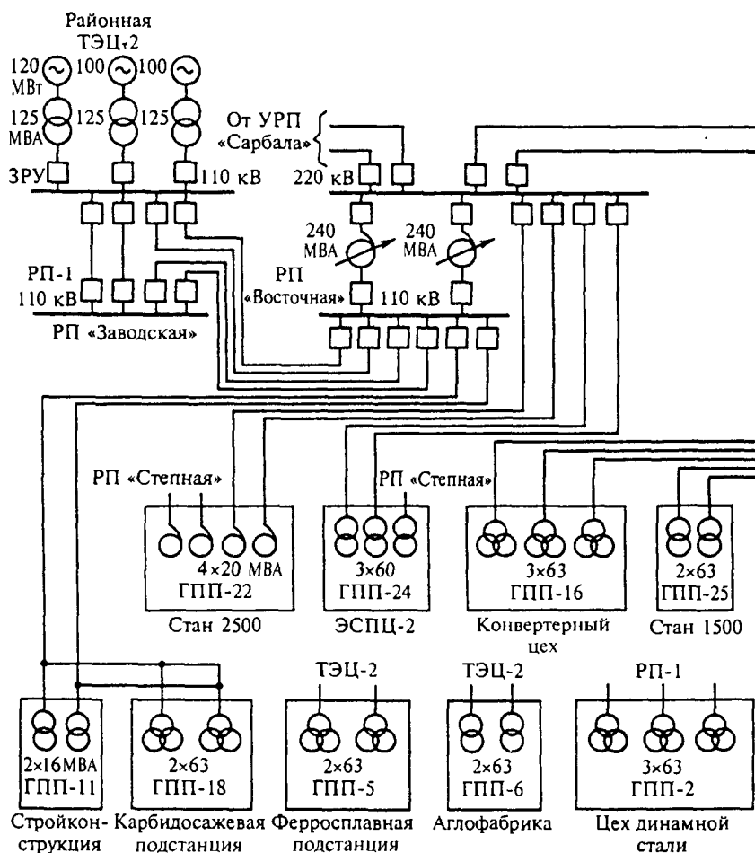
Рис. 2.2. Схема электроснабжения крупного предприятия: 6УР — граница раздела предприятие—
