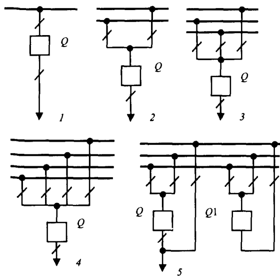
Рис. 4.1. Схемы присоединения потребителей к подстанциям энергосистемы: 1, 2, 3, 4 — соответственно с одной, двумя, тремя и четырьмя системами сборных шин; 5 — с двойной и обходной системами шин
