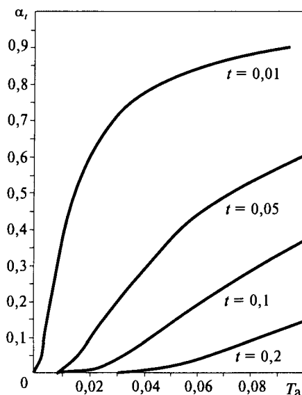
Рис. 9.3. Кривые для определения коэффициента затухания периодической составляющей тока КЗ
