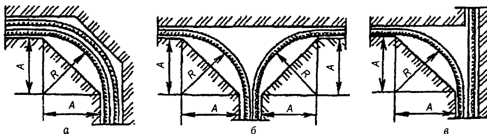
Рис. 8.7. Поворот и разветвление кабельных трасс:
