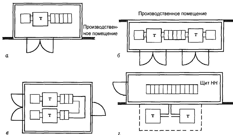
Рис. 7.7. Компоновка КТП с одним и двумя трансформаторами а — однотрансформаторная ТП встроенного типа, б — двухтрансформаторная ТП пристроенного типа, в — ТП отдельно стоящая, г — ТП с наружной установкой трансформаторов
