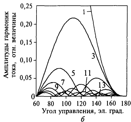
Рис. 6.7. Спектр напряжения (а) и тока (б) при угле сдвига фаз, равном 60 эл. град.
