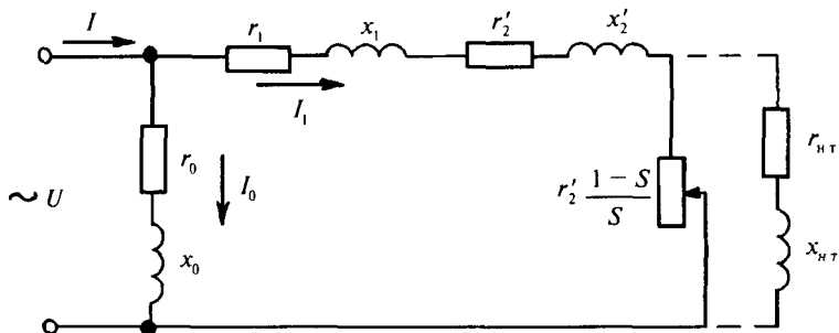
Рис. 13.4. Г-образная схема замещения АД с нагрузкой r_2^1 и трансформатора с нагрузкой r_{\text{нТ}} , x_{\text{нТ}}
