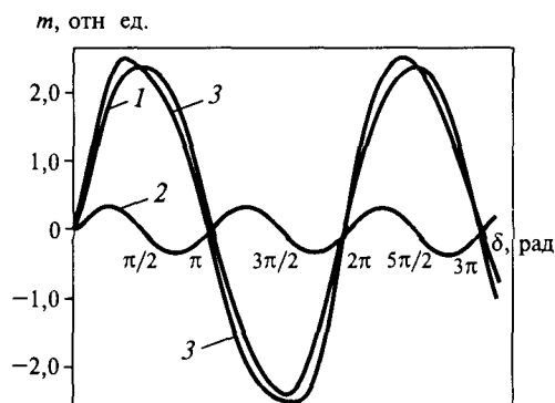
Рис. 11.8. Синхронизирующие моменты СД: 1 — синхронный M_c ; 2 — явнополюсности M_a ; 3 — результирующий
