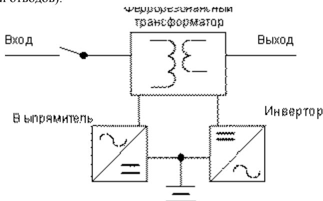
Рис. 7. Феррорезонансный ИБП.
