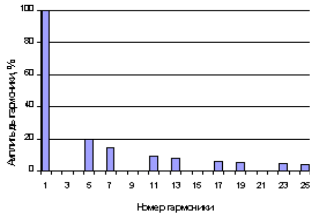
Рис.34. Спектр тока 6-импульсного выпрямителя
