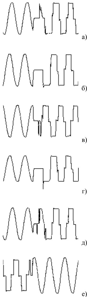
Рис. 10. Переключение ИБП с переключением с режима работы от сети на режим работы от батареи (а-д) и обратно (е).
