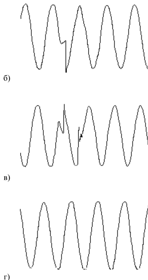
Рис. 13. Осциллограммы переключения "сеть-батарея" (а, б, в) и "батарея-сеть" (г) для ИБП, взаимодействующего с сетью.
