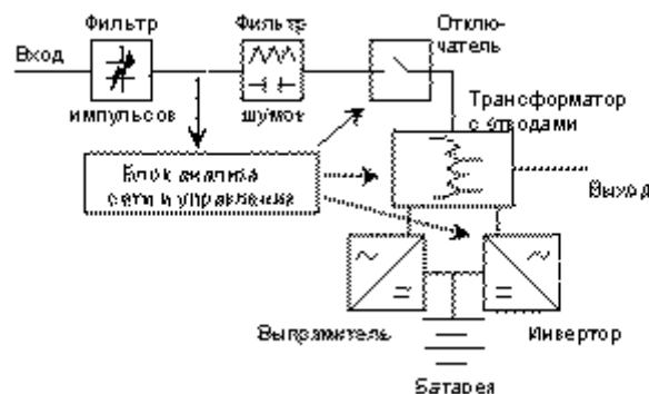
Рис. 12. Блок-схема ИБП, взаимодействующего с сетью.
