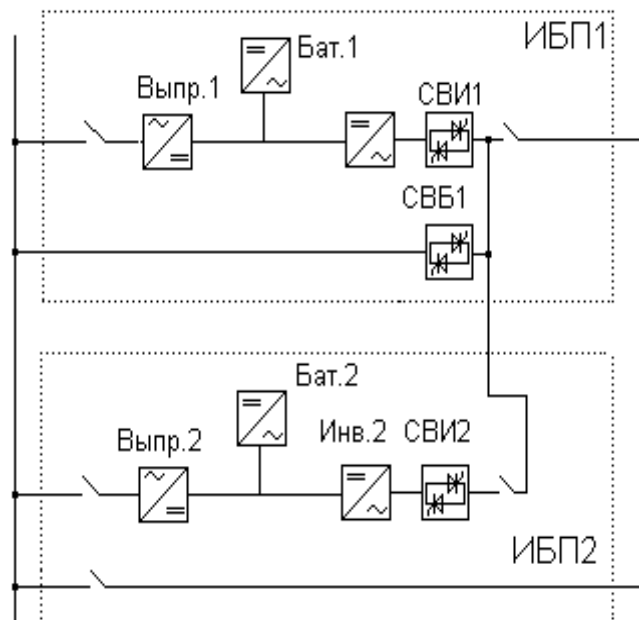
Рис.196. Трехфазный ИБП с горячим резервированием
