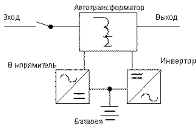
Рис. 6. ИБП, синхронизированный с сетью.
