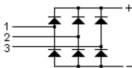
Рис. 33. Трехфазный мост
