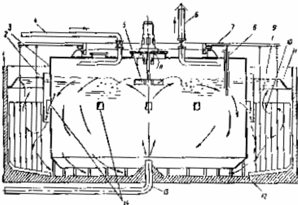
Рис. 16. Схема окситенка
