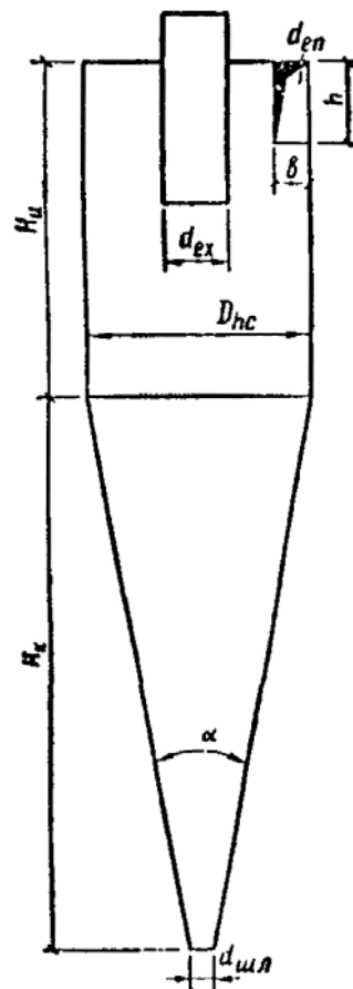
Рис. 10. Схема напорного гидроциклона
