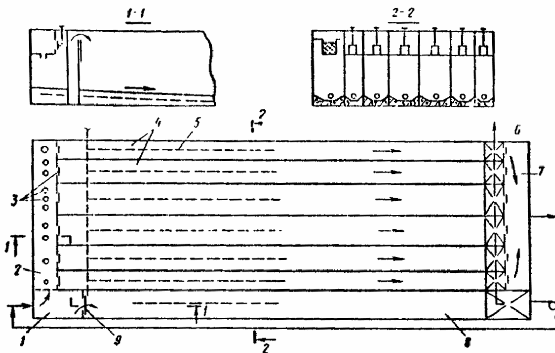
Рис. 1. Схема многоканального усреднителя
