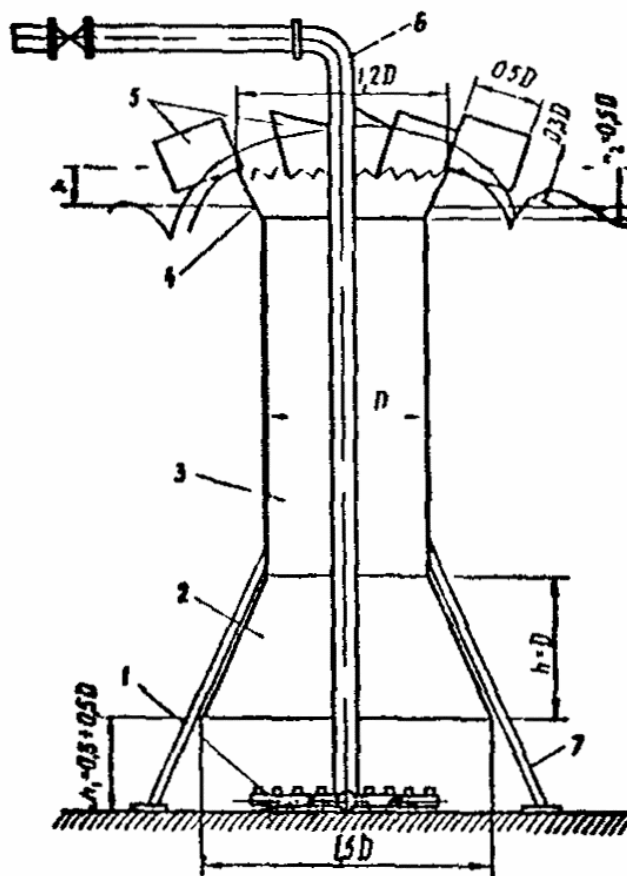
Рис. 14. Схема эрлифтного аэратора
