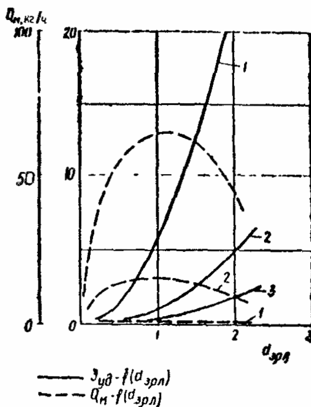
Рис. 15. Зависимость удельных энергозатрат и производительности по кислороду от диаметра эрлифтных аэраторов при различных значениях интенсивности аэрации
