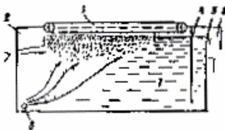
Рис. 18. Схема горизонтального флотационного илоотделения
