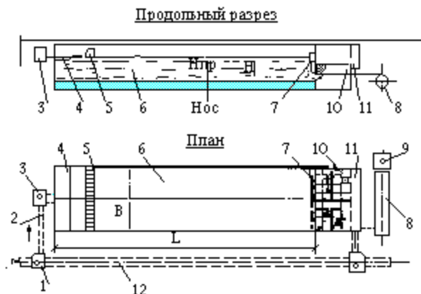
Рис. 7. Схема двухсекционного очистного сооружения закрытого типа
