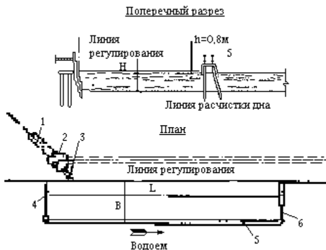
Рис. 6. Схема стационарного щитового заграждения
