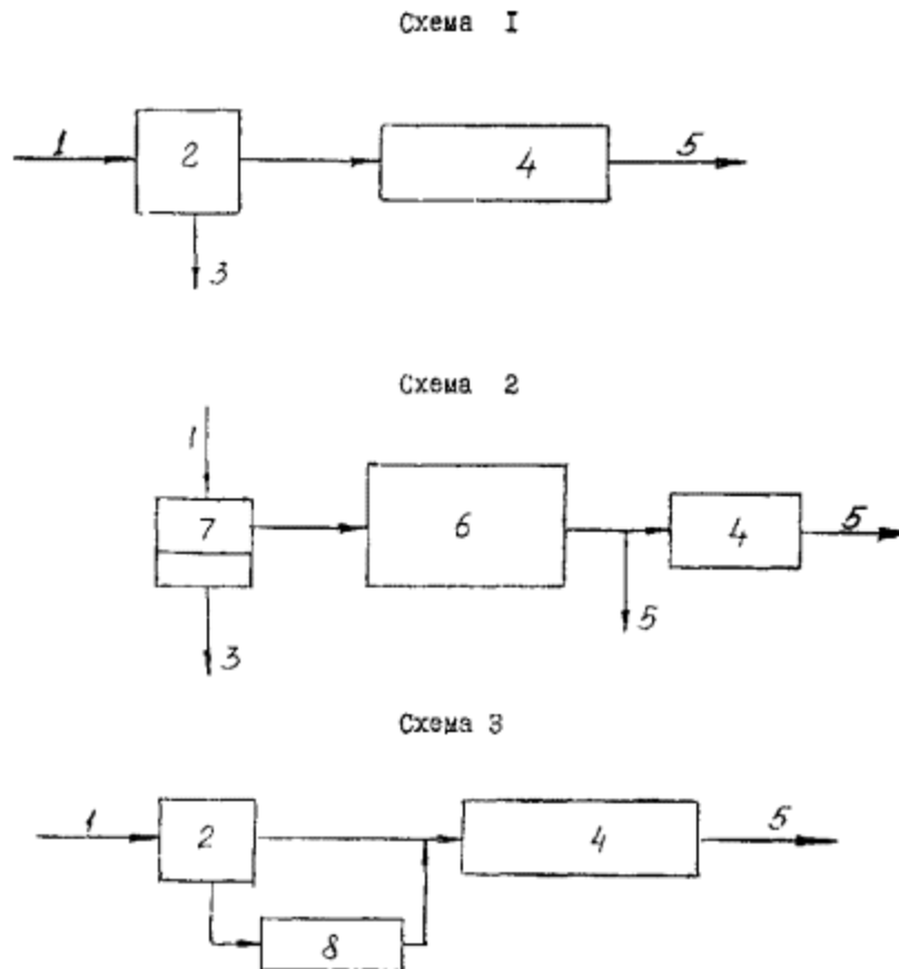
Рис. 1. Принципиальные схемы разделения дождевого стока перед очистными сооружениями:
