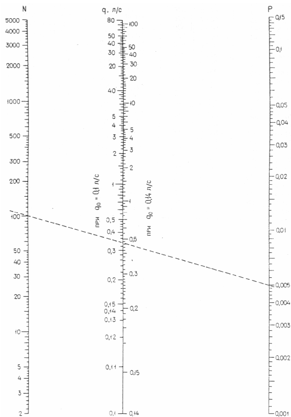
Черт. 1. Номограмма для определения секундных расходов воды q при q_0 = 0,1 и 0,14 \text{ л/с} и P \leq 0,15
