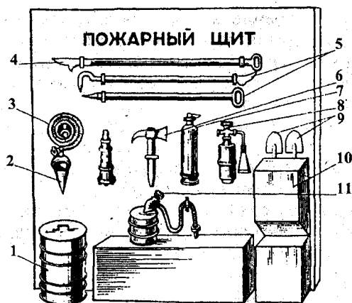
Рис. 11.6.1. Пожарный инвентарь:
