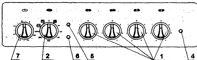
Рис. 11.5.3 б. Панель управления плиты «Гефест» моделей 2142 и 2162:
