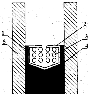
Рис. 8.8.8. Принципиальная схема конструкции традиционного изолирующего стеклопакета:
