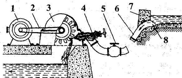
Рис. 10.3.2. Схема гидроэлектростанции (ГЭС) с ковшовой (активной) турбиной;
