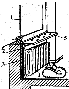
Рис. 8.8.7. Утепление радиаторной стенки с установкой отражающего экрана из алюминиевой фольги и обдув стекла поднимающимся от радиатора теплым воздухом через отверстие в подоконнике:
