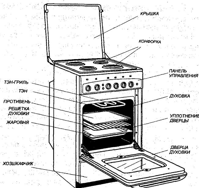
Рис. 11.5.1а. Электрическая плита с чугунными конфорками «Гефест»
