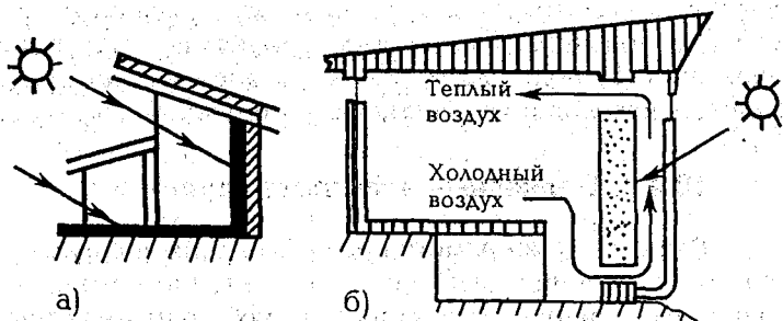
Рис. 10.4.3. Пассивные солнечные нагреватели:
