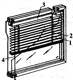
Рис. 8.8.6. а — Межстекольная штора-жалюзи:
