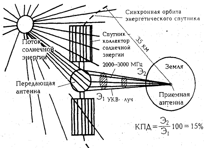
Рис. 10.4.7. Схема солнечной электростанции на искусственном спутнике
