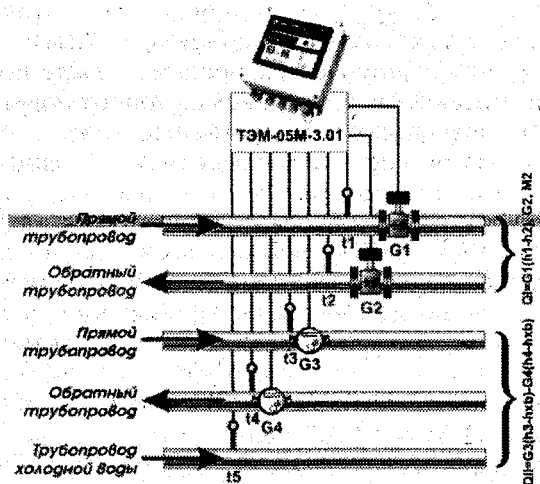
Рис. 8.3.3. Схема установки ТЭМ-05МЗ
