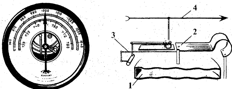
Рис. 11.4.3. Барометр (анероид)
