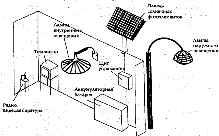
Рис. 10.4.6. Фотоэлектрическая солнечная установка для энергообеспечения дома в сельской местности
