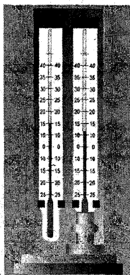
Рис. 11.4.1 б – психрометр
