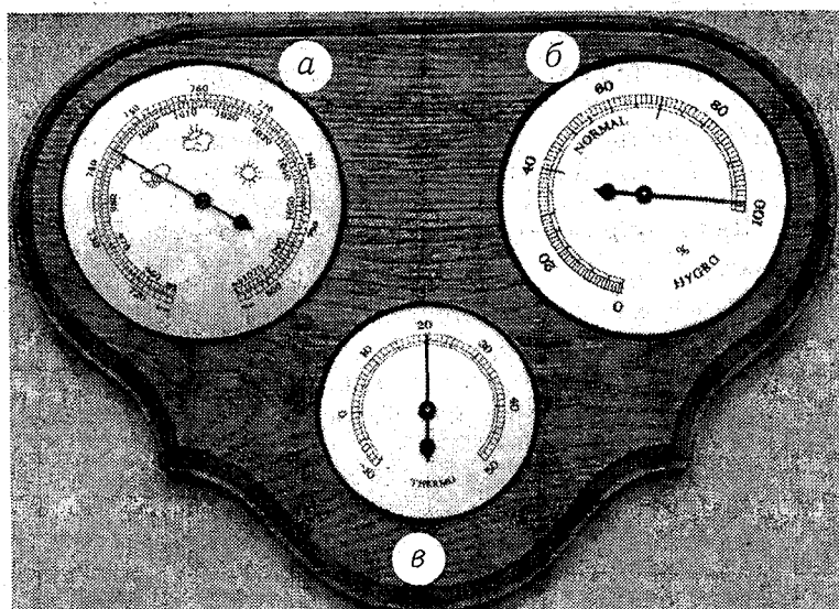
Рис. 11.4.5. Комплект приборов: а – барометр, б – гигрометр, в – термометр
