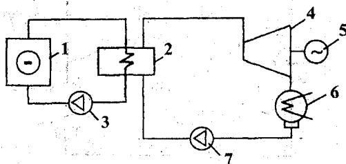
Рис. 10.3.4. Тепловая схема простейшей двухконтурной атомной электростанции (АЭС) 1 — ядерный реактор, 2 — теплообменник-парогенератор, 3 — главный циркуляционный насос, 4 — турбина, 5 — электрогенератор, 6 — конденсатор, 7 — питательный насос
