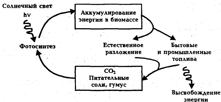
Рис. 9.5.1. Система планетарного круговорота биомассы
