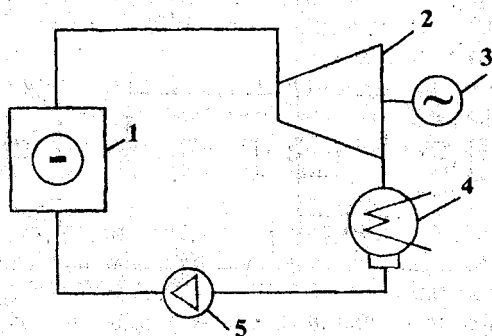
Рис. 10.3.3. Тепловая схема простейшей одноконтурной атомной электростанции (АЭС):
