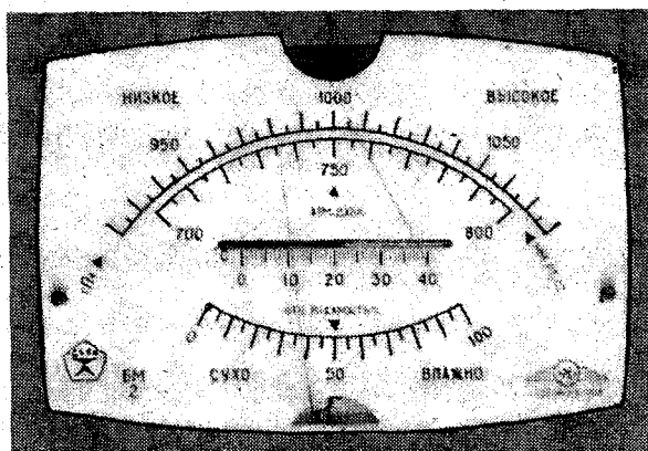
Рис. 11.4.4. Баротермогигрометр
