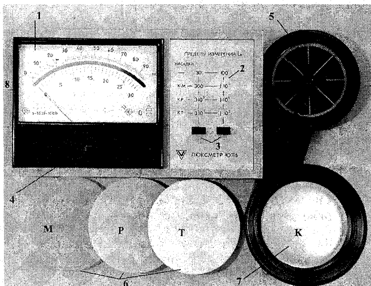
Рис. 11.1.1. Люксметр Ю-116
