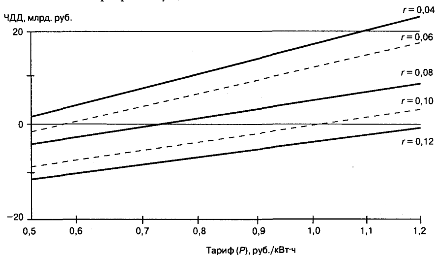
Рис. 17.1. Зависимость интегрального эффекта от тарифа на электроэнергию
