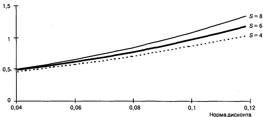
Рис. 17.2. Зависимость предельного тарифа от нормы дисконта и продолжительности строительства
