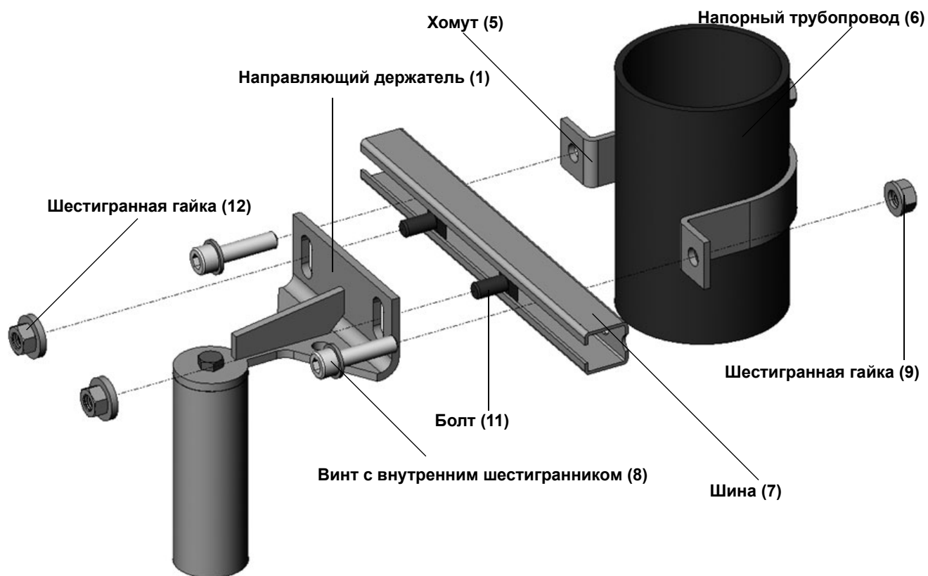
Рис. Q-3: Монтаж направляющего держателя при креплении труб
