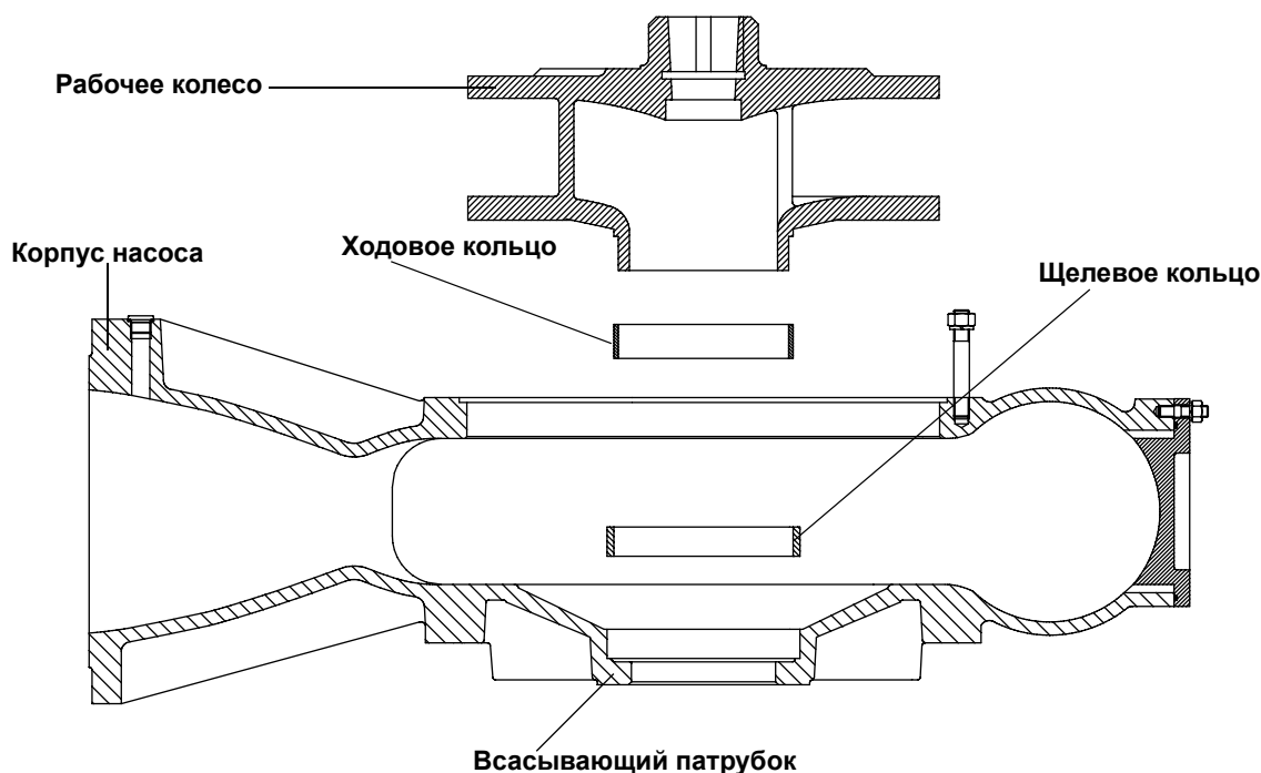
Рис. 7-4: Замена щелевого и ходового колец
