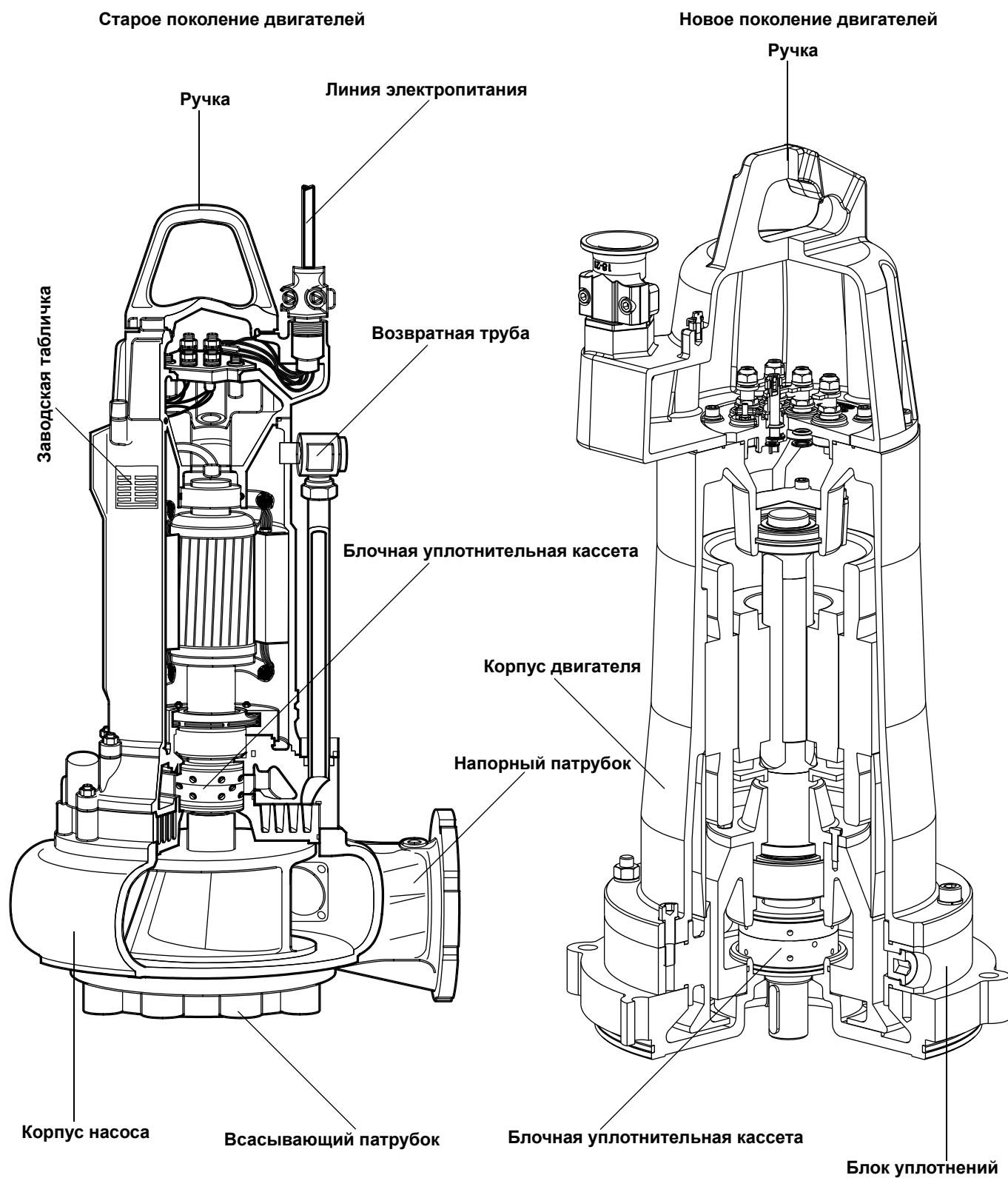
Рис. 3-2: Конструкция оборудования
