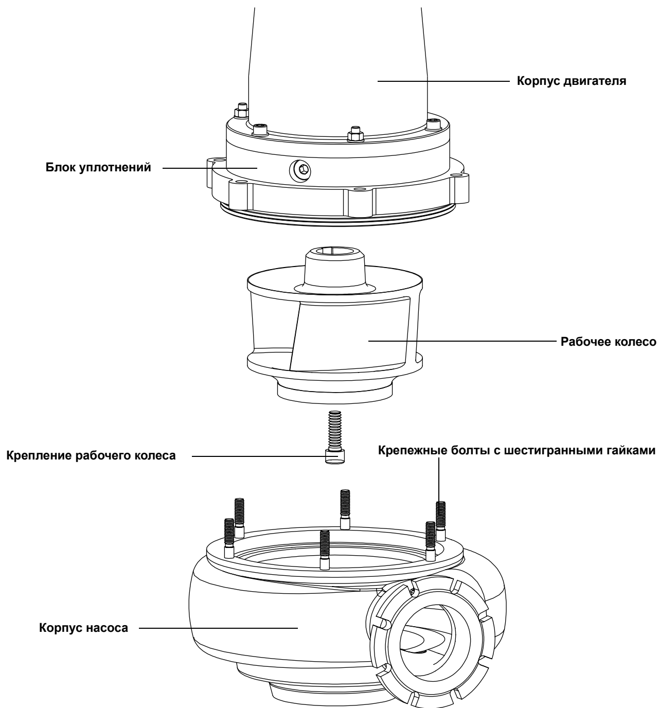
Рис. 7-3: Замена рабочего колеса – вариант 1:
