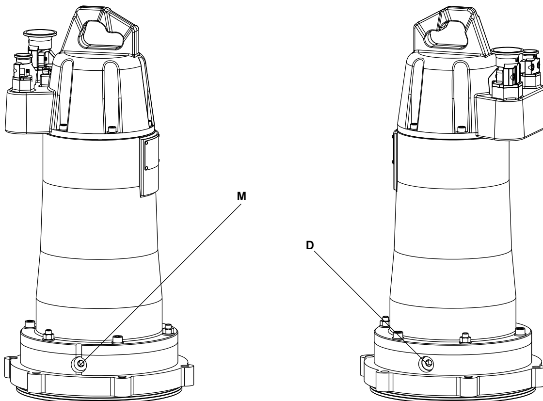
Рис. 7-2: Положение отдельных резьбовых пробок (новое поколение двигателей)
