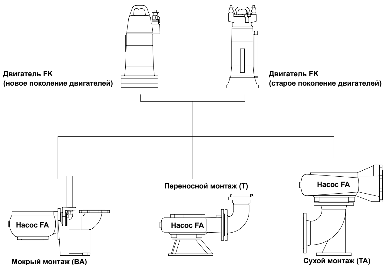
Рис. 3-1: Внешний вид различных агрегатов
