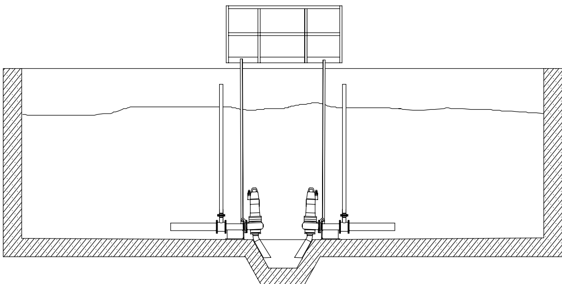
Рис. Р-2: Монтаж струйного аэратора
