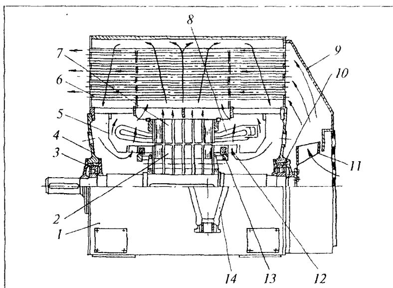
Рис. 2. Электродвигатель ДАЗО 4-450Х-8У1:
