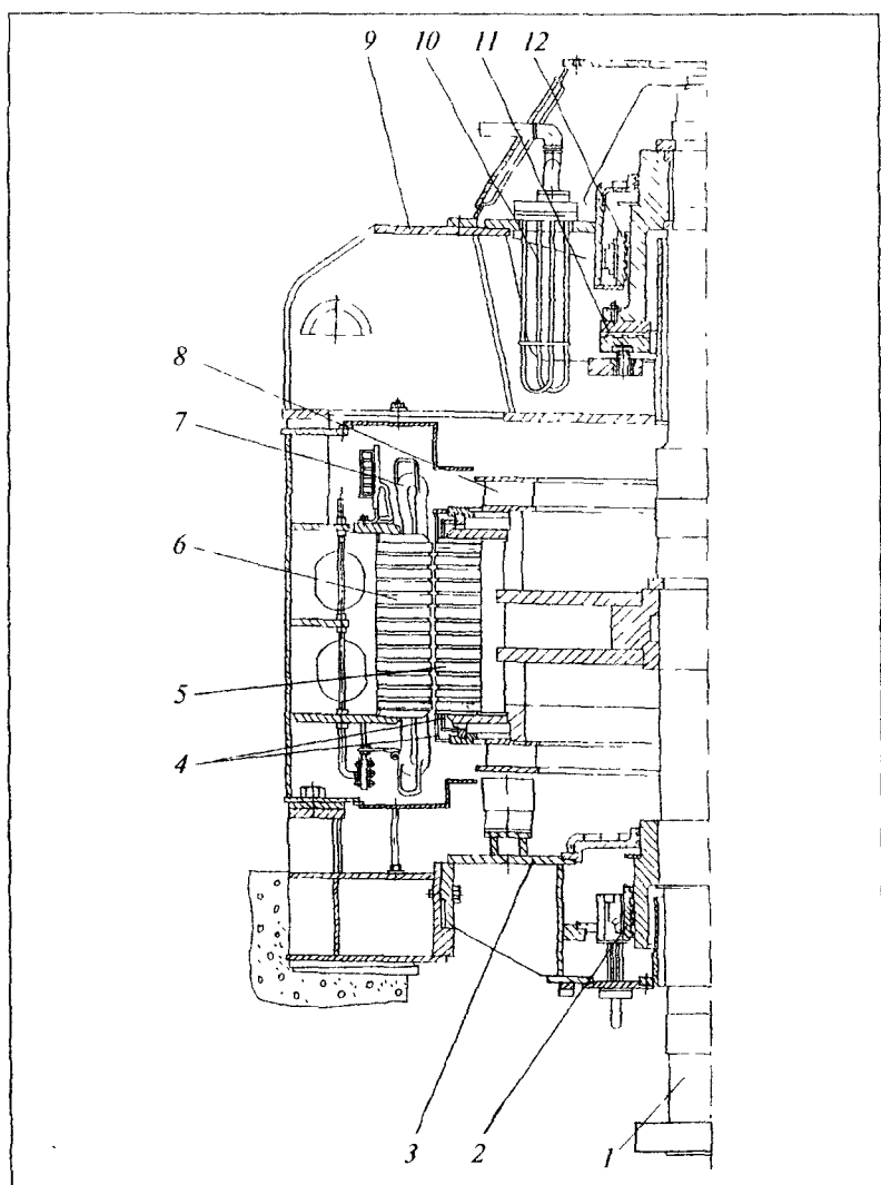
Рис. 3. Двухскоростной электродвигатель вертикального исполнения ДВДА-260/99-20-24У4 ( P = 4000/2500 кВт, n = 300/250 мин -1 , U = 6 кВ):
