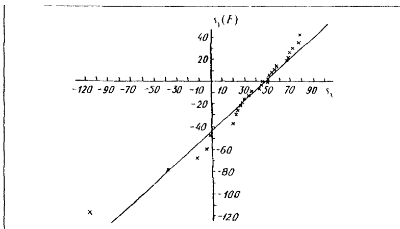
Рис 10 Графическая проверка согласия эмпирического распределения с теоретическим сроком службы подшипника скольжения со стороны свободного конца вала электродвигателя АР-500
