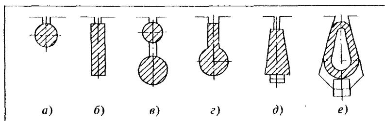
Рис. 6. Типы исполнений короткозамкнутых обмоток асинхронных электродвигателей:
