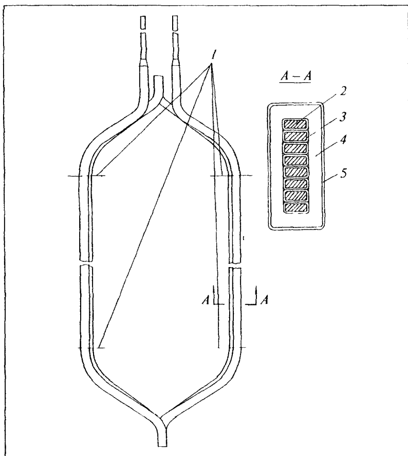
Рис. 15. Катушка обмотки статора электродвигателя типа СДМЗ-20-49-60:
