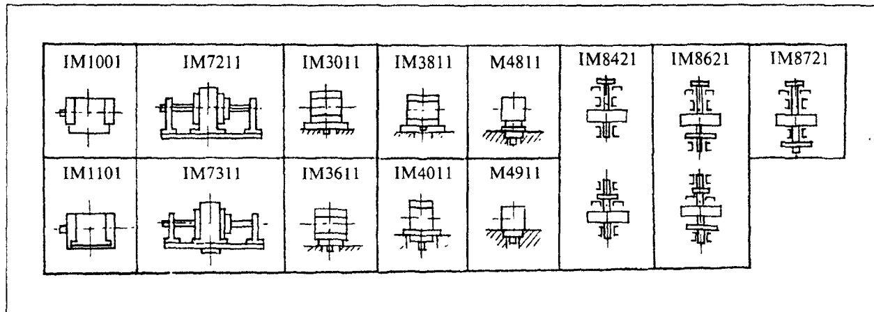
Рис. 1. Некоторые типы конструктивного исполнения электродвигателей по способу монтажа:
