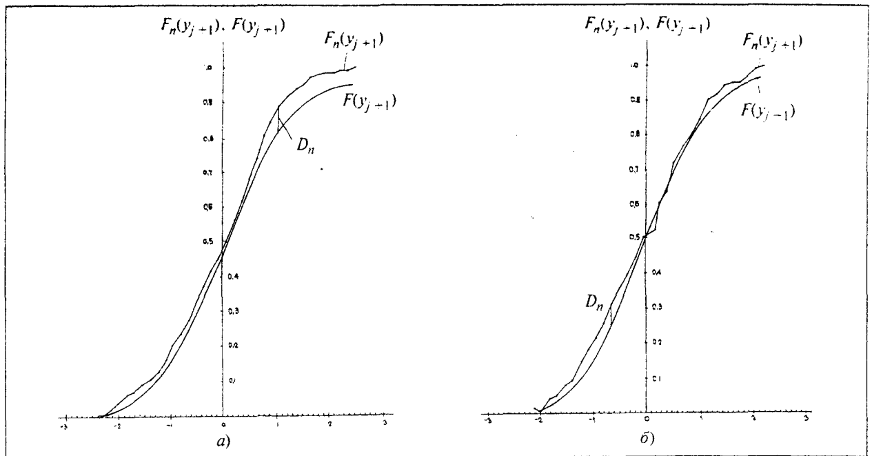
Рис. 14. Функция опытного F_n(y) и теоретического F(y) распределения пробивных напряжений изоляции обмотки статора:
