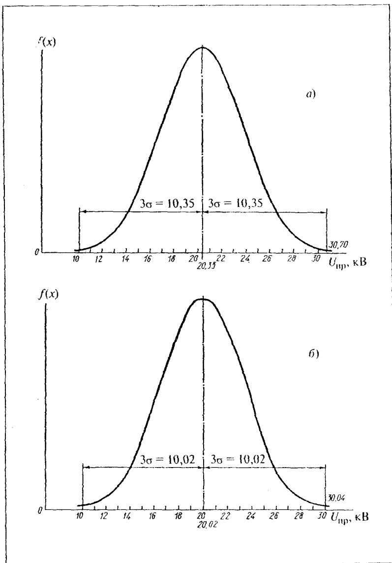
Рис. 24. Нормальные кривые (кривые Гаусса) плотности распределения пробивных напряжений обмоток статоров электродвигателей типа ДВ/Д-215/39-12-16: а — электродвигатель № 1 после наработки 126215 ч; б — электродвигатель № 2 после наработки 130688 ч
