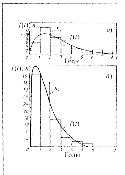
Рис. 28. Гистограмма и теоретические кривые плотности вероятности срока службы подшипников № 322 (а) и № 2322 (б) электродвигателя А-112-4М
