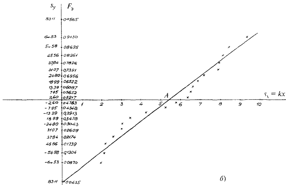
Рис 21 Графическая проверка согласия эмпирического распределения отказов в СВО электродвигателей АВ-8000/6000УЗ с теоретическим и определение их параметров при помощи вероятностных сеток:
