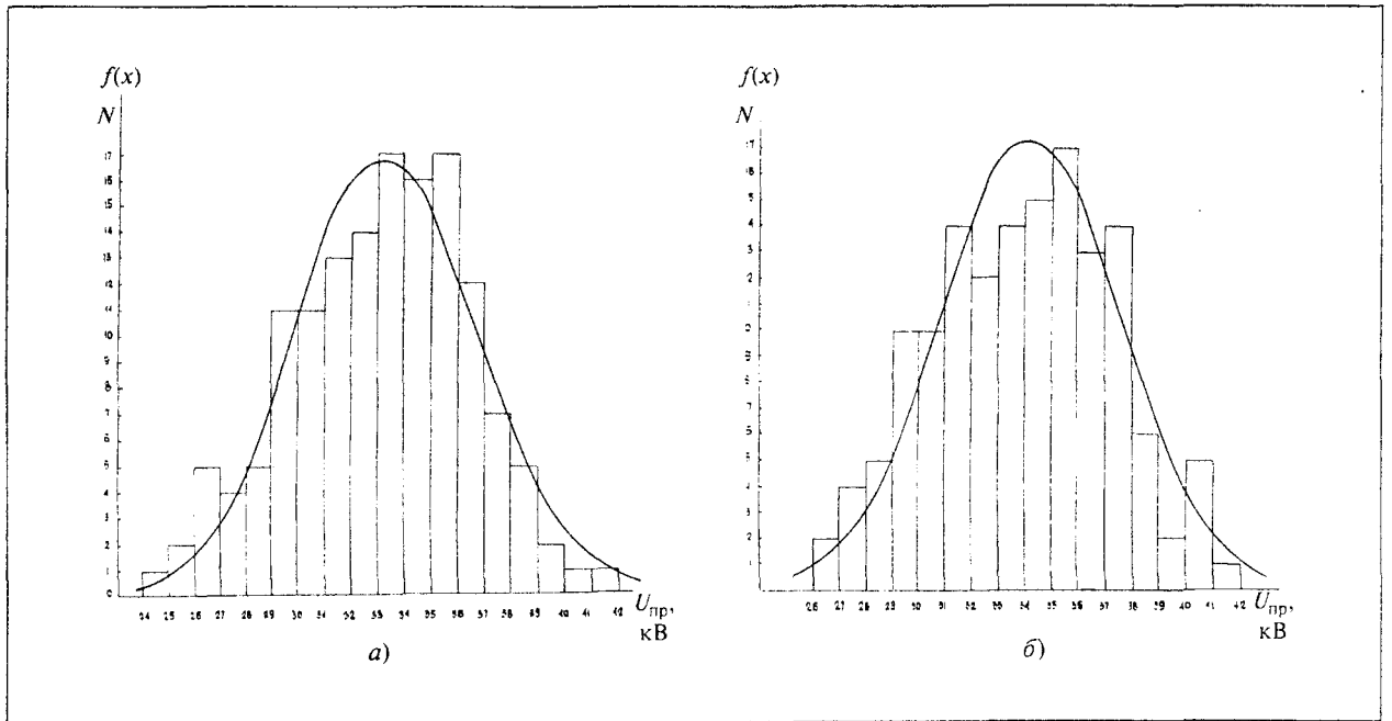
Рис. 13. Гистограмма, совмещенная с кривой нормальной плотности вероятности значений пробивных напряжений изоляции обмотки статора:
