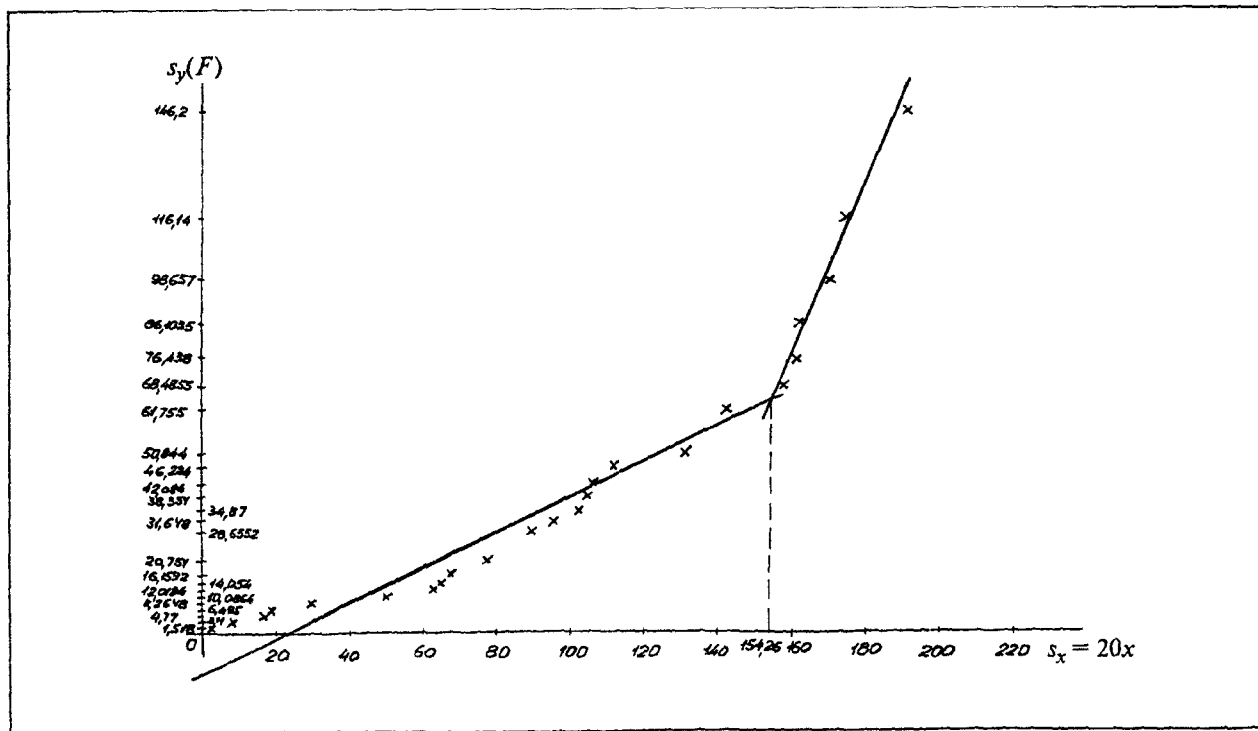
Рис. 25. Определение времени перехода от периода нормальной эксплуатации к периоду износовых отказов обмотки статора электродвигателя СДМЗ-20-49-60
