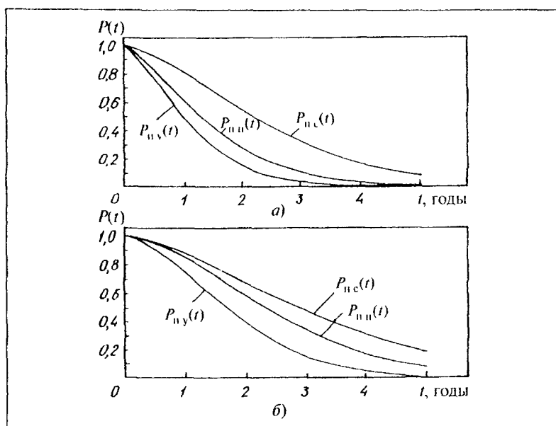
Рис 11 Кривые вероятности безотказной работы подшипниковых узлов: а — электродвигателя типа А-112-4М (НРТ), б — электродвигателя типа АР-500 (БПН)
