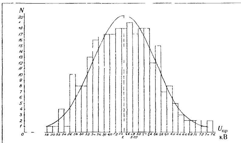
Рис. 16 Гистограмма, совмещенная с кривой нормальной плотности вероятности пробивных напряжений витковой изоляции обмотки статора электродвигателей типа СДМЗ-20-49-60
