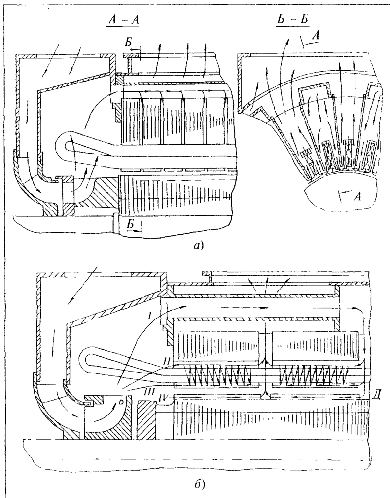
Рис. 8. Система охлаждения электродвигателей серии АТД 4 мощностью 315 – 500 кВт (а) и 630 – 1600 кВт (б)
