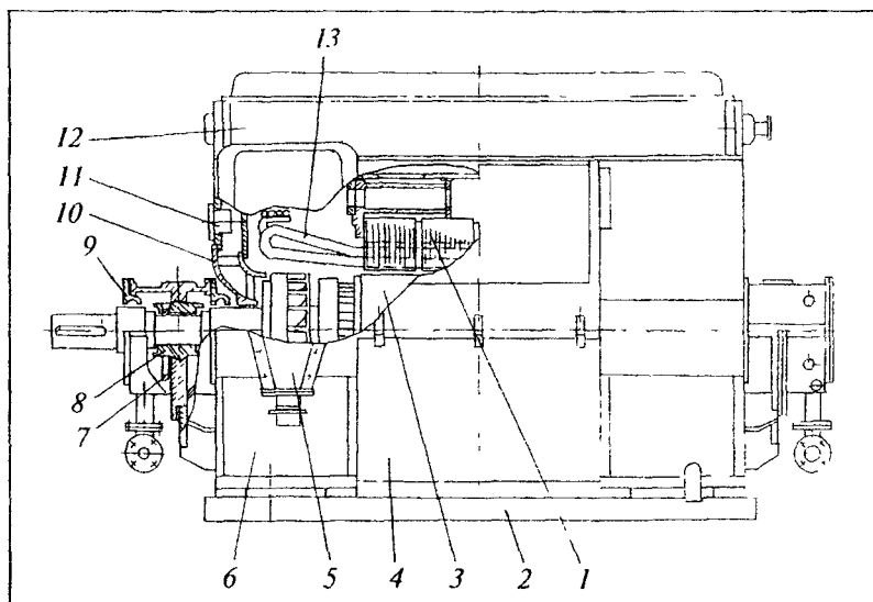
Рис. 7. Электродвигатель 4АЗМ-1600/6000УХЛ4 с встроенными подшипниками скольжения:
