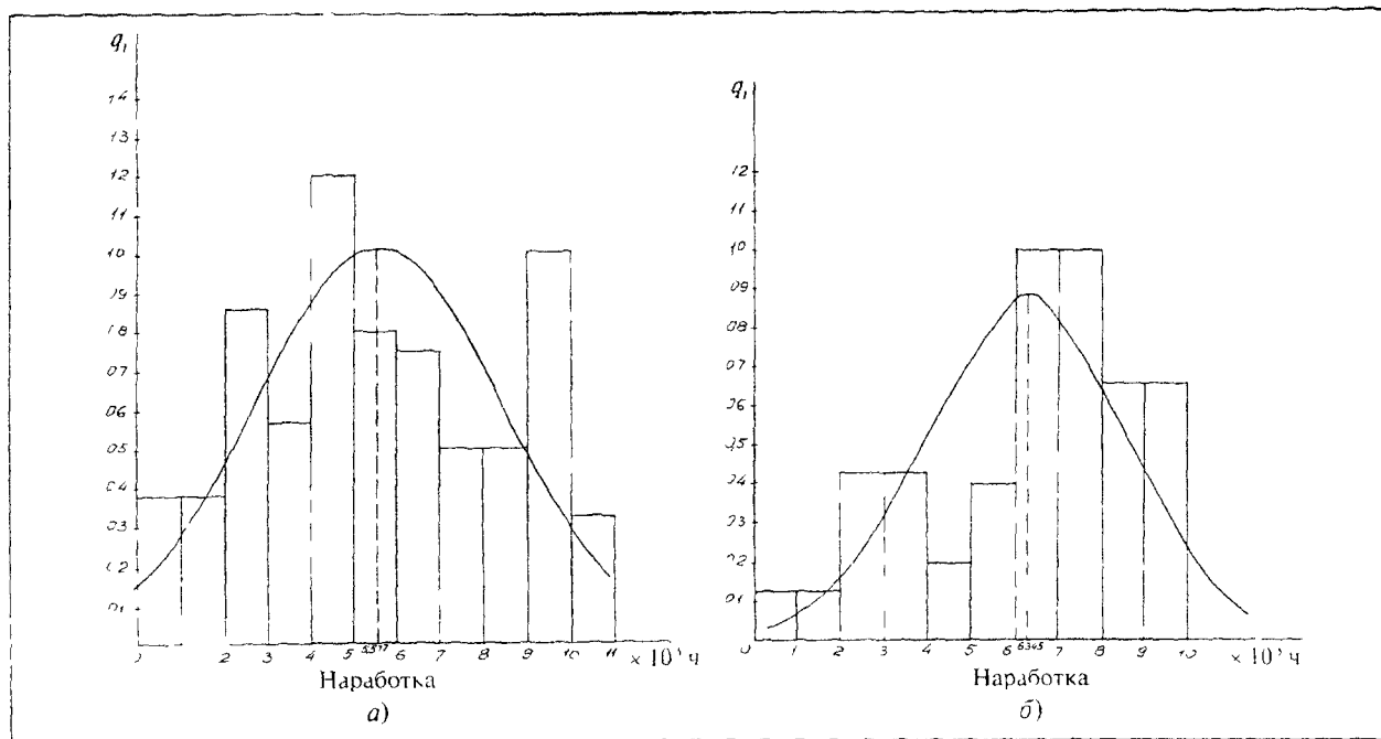
Рис. 19 Гистограмма удельной повреждаемости и теоретические кривые плотности нормального распределения отказов СВО электродвигателей АВ-8000/6000УЗ:
