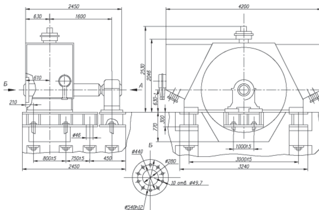
СДКП2-19-39-16УХЛ4
