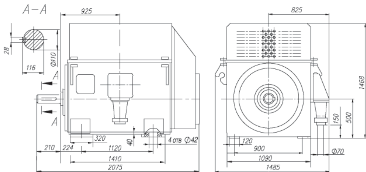
Габаритный чертёж двигателя ДАЗО4 10000 В, 50 Гц
