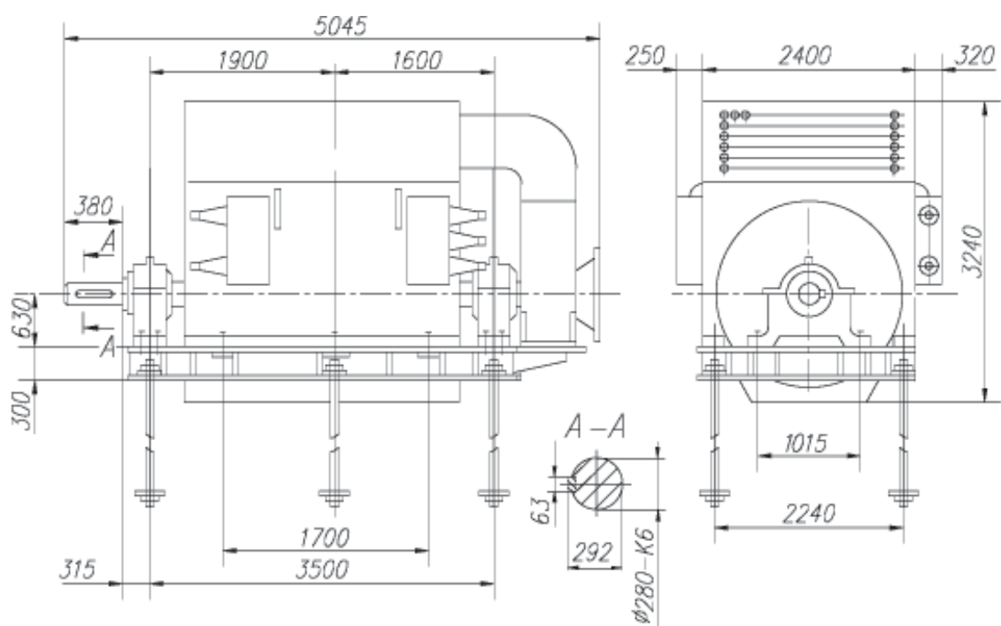
AO2-18-120-8/10Y
