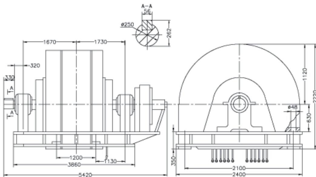
ДАФЗ-16-94-8УХЛ4
