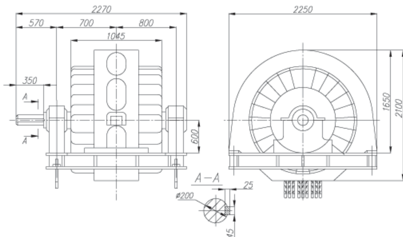
СДМ-500-6,3/3,15-250УХЛ4
