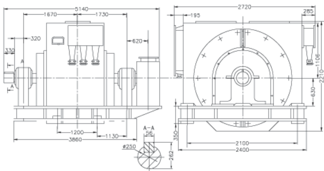
ДАФЗ-4000-6-750УХЛ4
