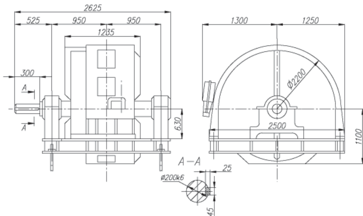
СДН32-18-34-24УХЛ4
