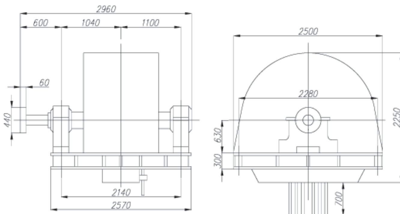
АН32-18-66-12Т3
