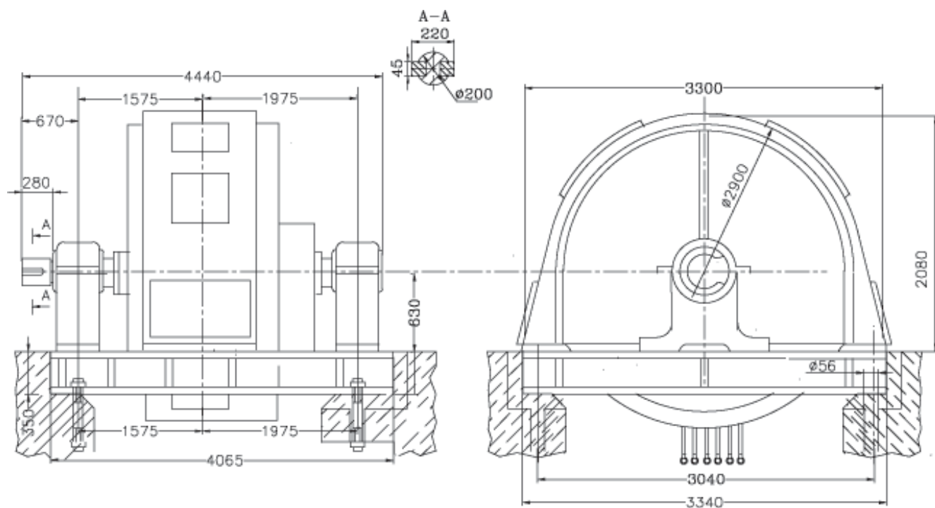
СДСЗ-17-64-6
