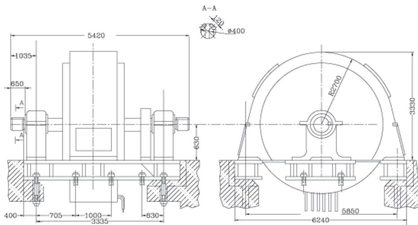
СДМ32-22-56-60
