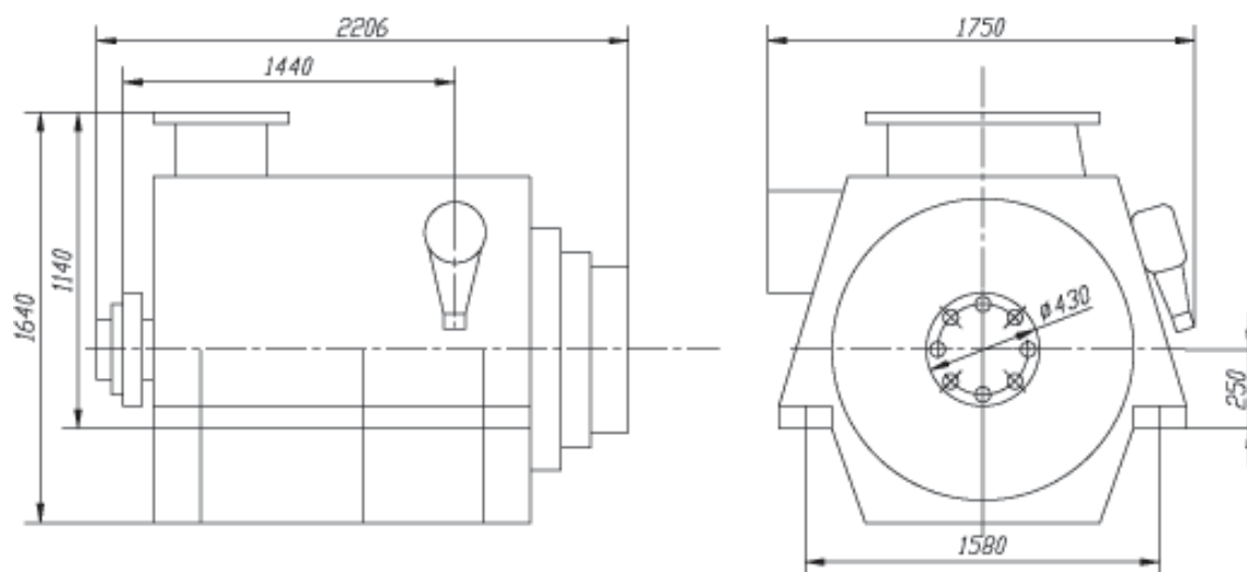
ГСБ-1120-6,3-1000УХЛ2
