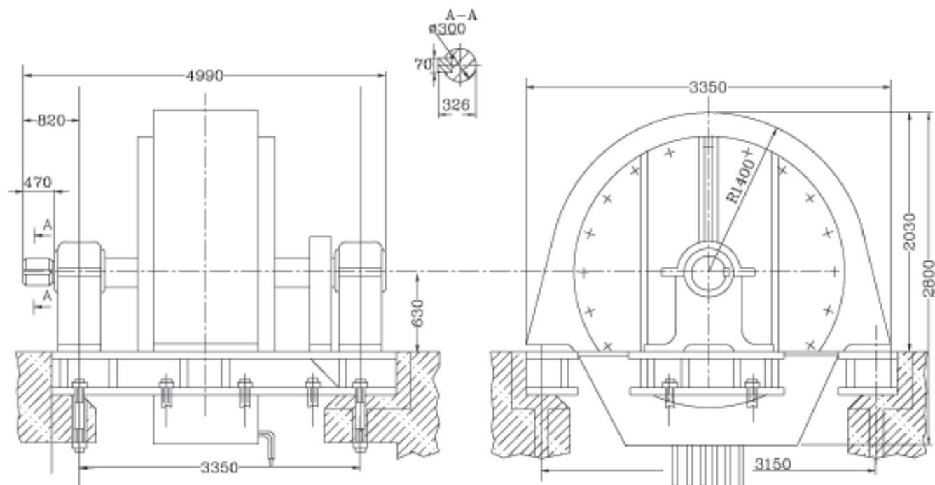
СДМЗ-3150-10-500
