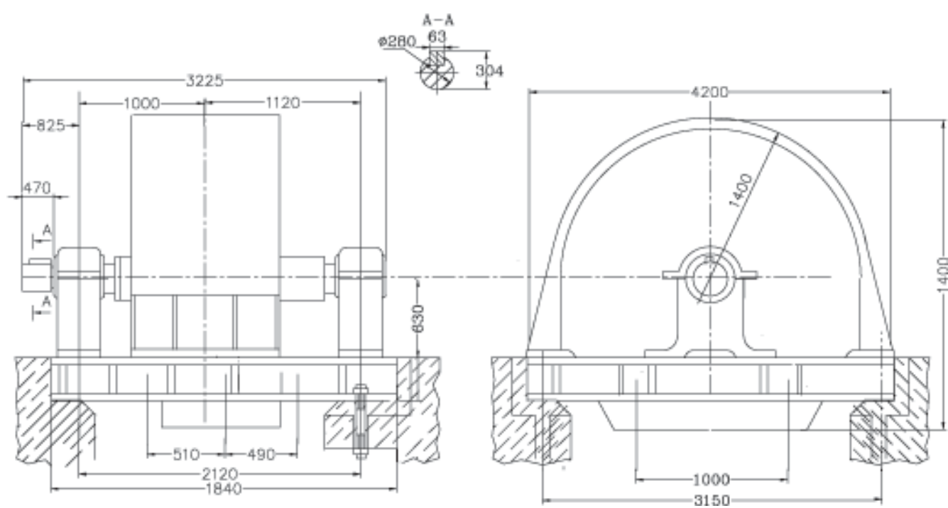
СДНЗ-2-19-49-24
