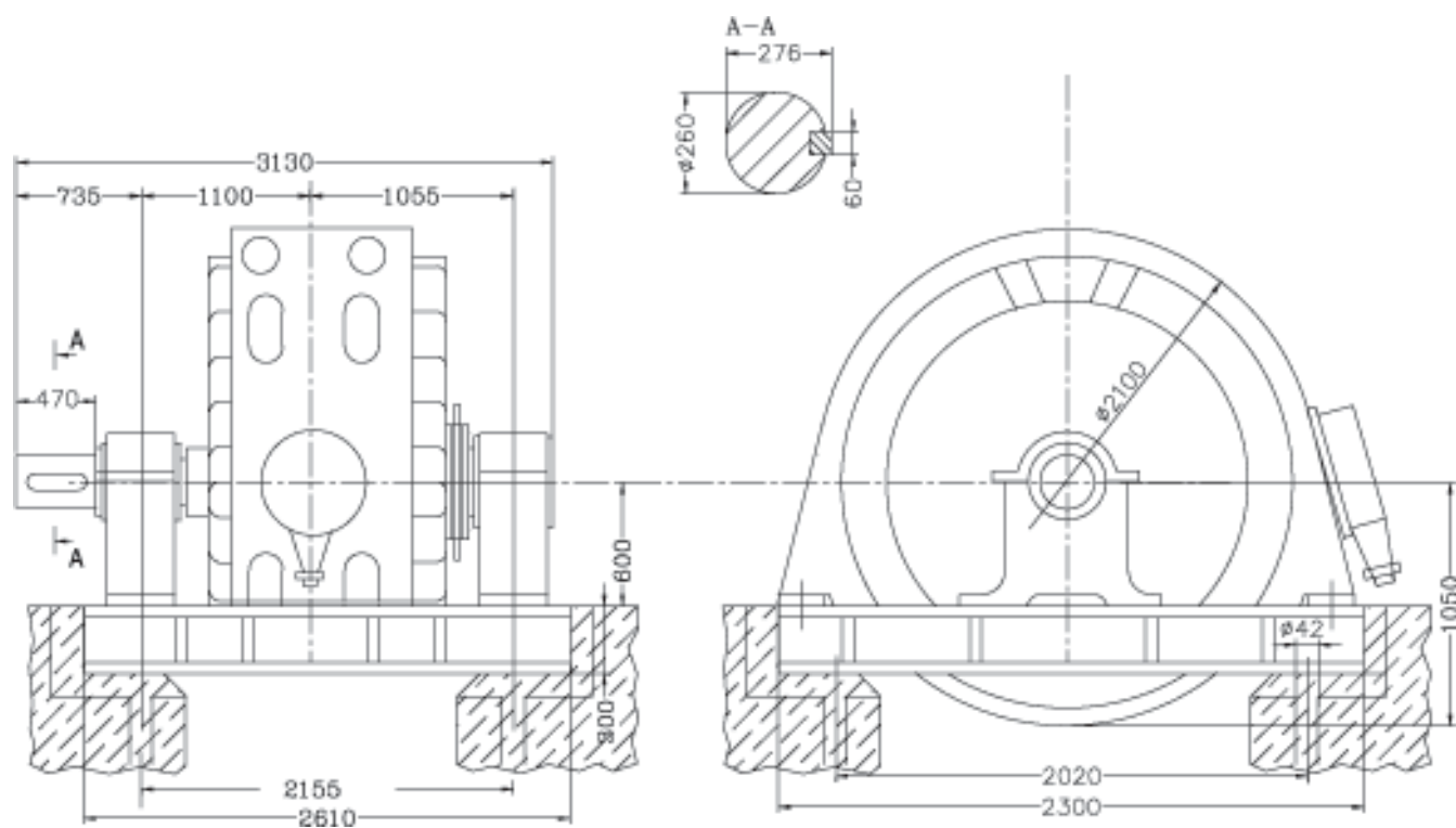
СДН2-18-64-12УХЛ4
