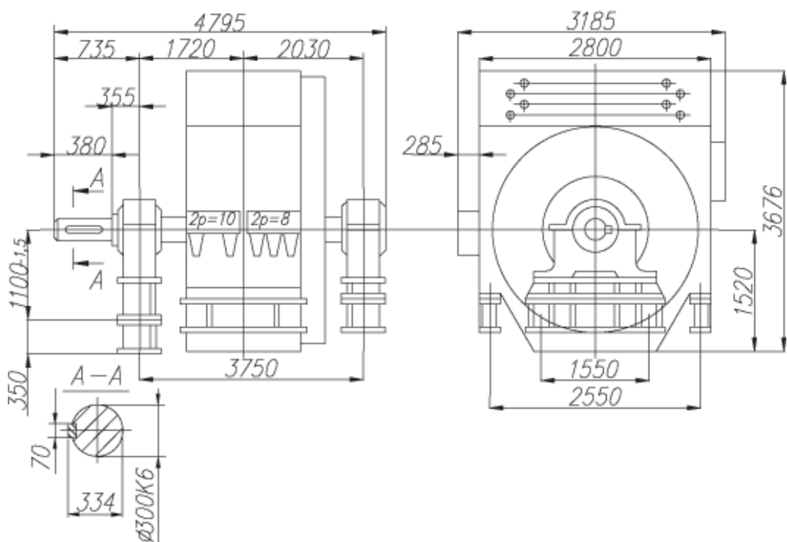
AO-5000/2500-750/600Y1
