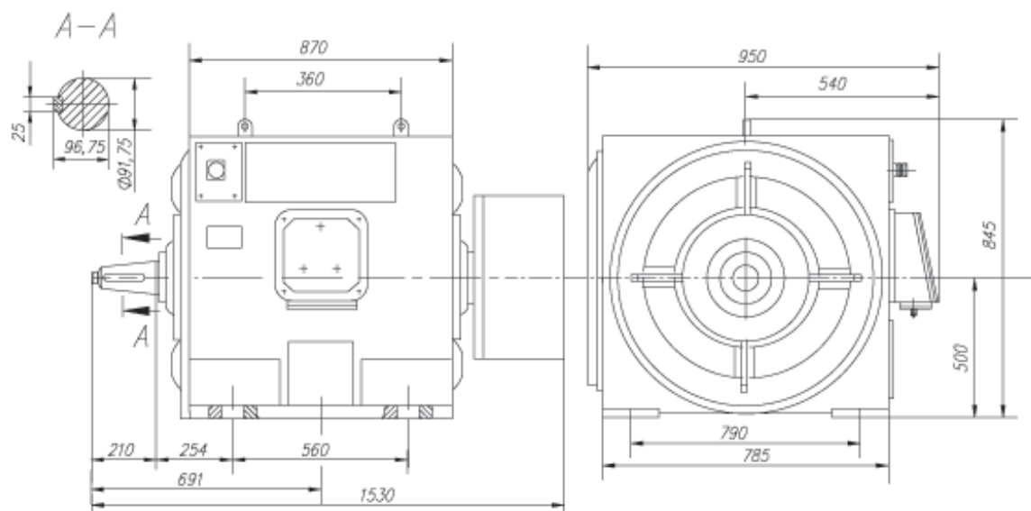
АКЭ-160-0,38-600
