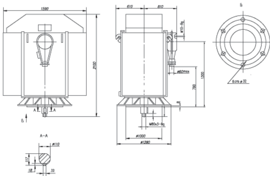
4АОВ-400У-4У3
