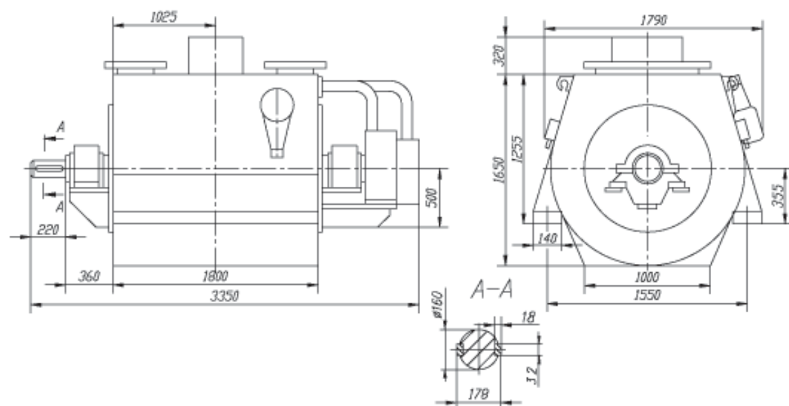
ГСБ-1800-6,3-1500УХЛ2
