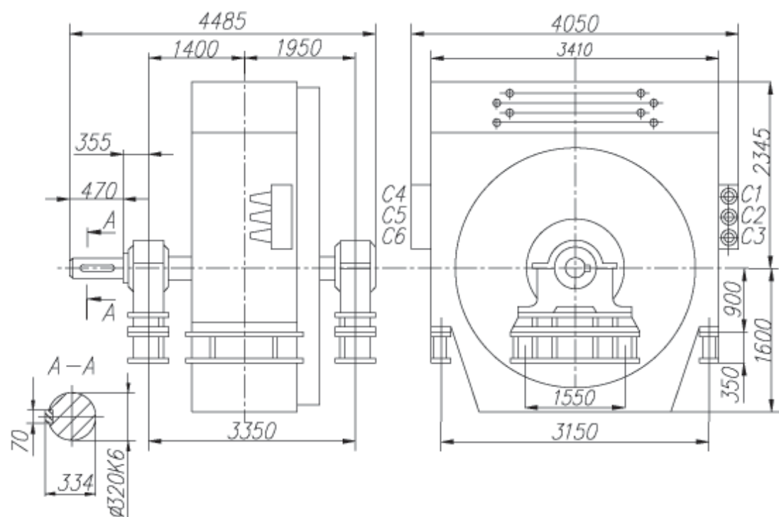
AO2-20-83-12Y1
