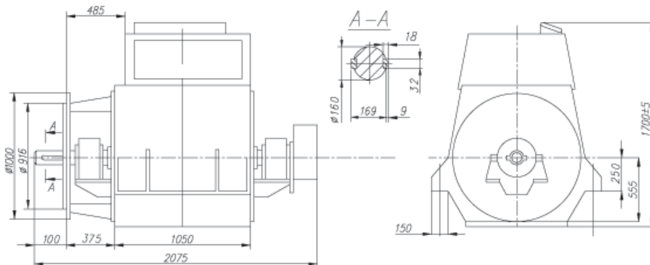
СГ-1250-1500У2
