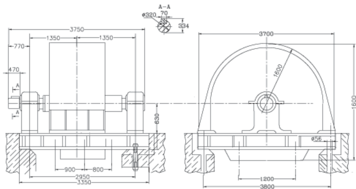
СДНЗ-2-20-49-20
