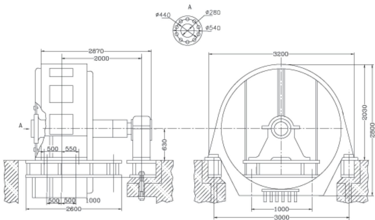
СДК-2-19-51-16УХЛ4
