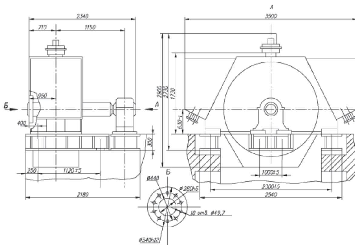
СДКП2-18-51-16ФУХЛ4
