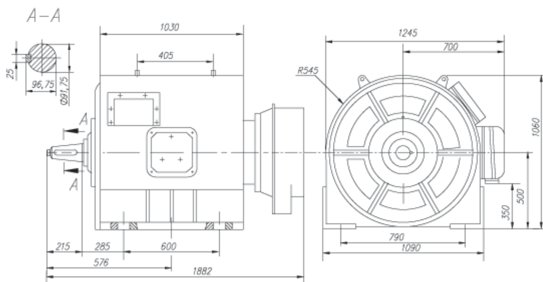
АКЭ-200-0,38-600
