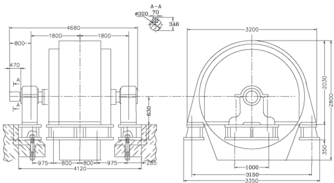
СДНЗ-2-19-104-10
