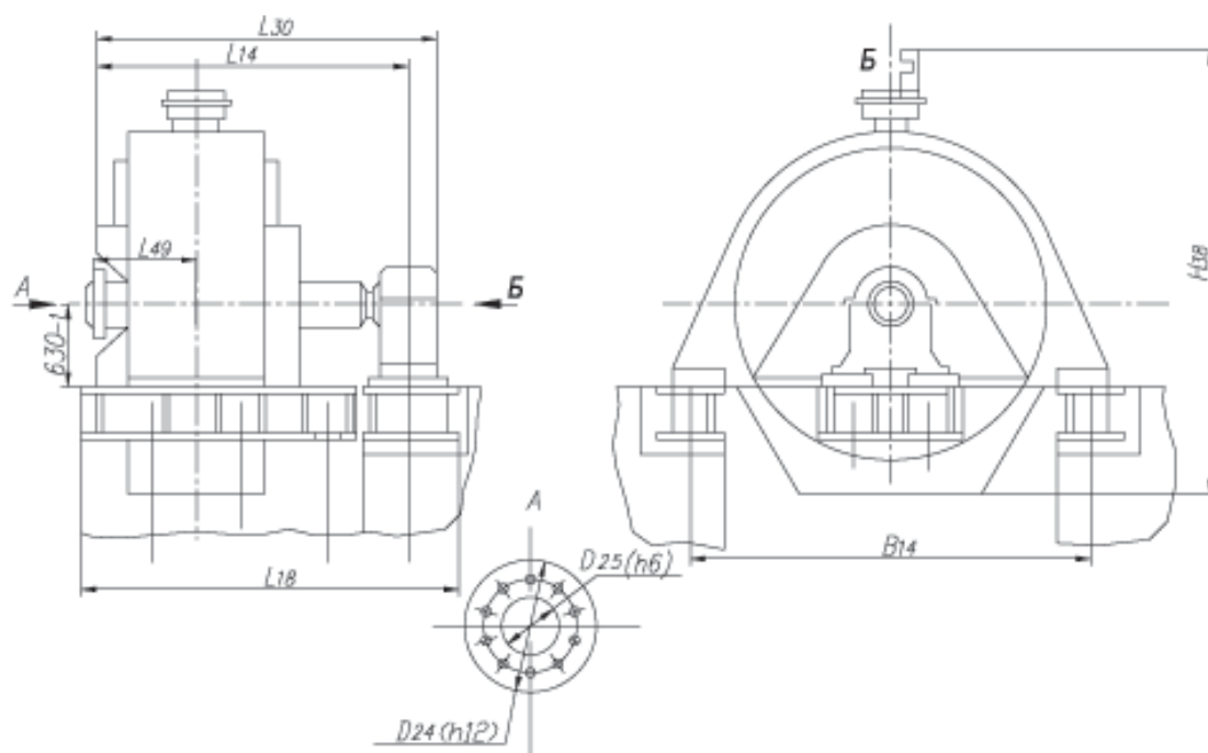
СДКП2-19-39-16УХЛ4
