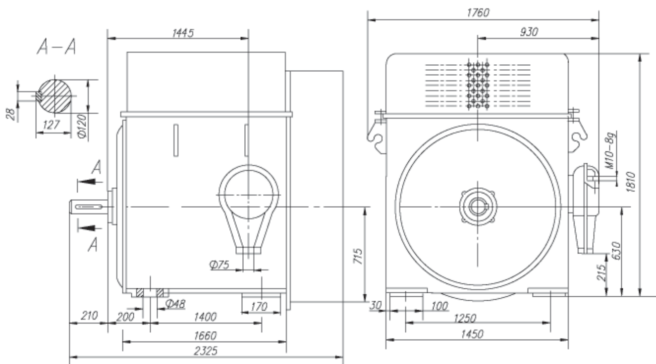
Электродвигатель АЗО-200-375
