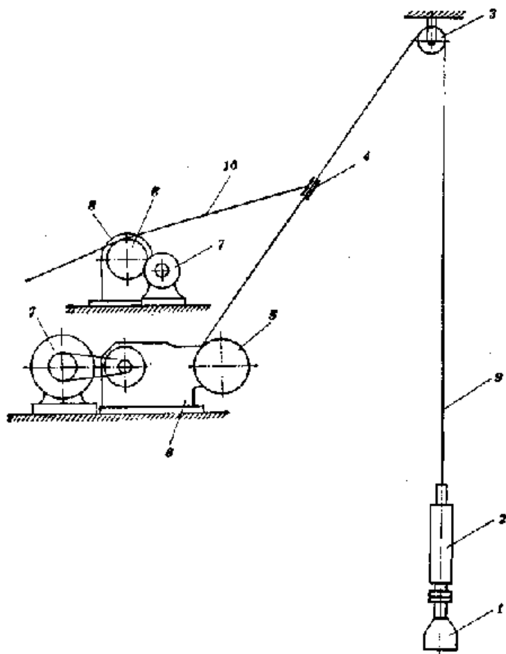
Рис. 35. Схема установки для ударно-канатного бурения: 1 — долото; 2 — ударная штанга; 3 — блок; 4 — подвижный захват; 5 — канатный барабан; 6 — барабан для веревки; 7 — электродвигатель; 8 — редуктор; 9 — канат; 10 — веревка
