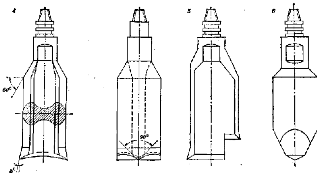
Рис. 22. Буровые долота: 1 — зубильное (плоское); 2 — двутавровое; 3 — крестовое; 4 — скругляющее; 5 — эксцентричное; 6 — пирамидальное
