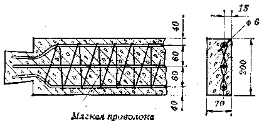
Рис. 15. Железобетонная пластина
