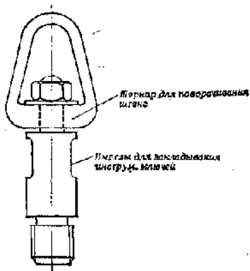
Рис. 30. Вертлюг
