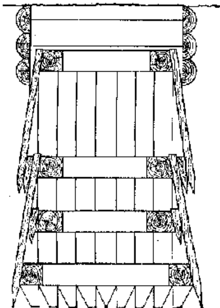
Рис. 8. Изоляция плавуну косым шпунтом
