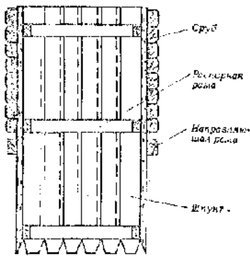
Рис. 6. Изоляция плывуна шпунтовым ящиком
