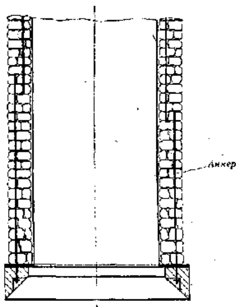
Рис. 16. Армирование кирпичных и каменных колодцев анкерными тягами
