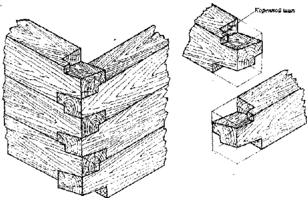
Рис. 4. Угловое соединение брусьев сруба
