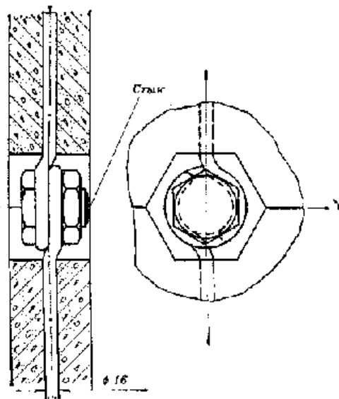
Рис. 13. Соединение бетонных колец стержнями
