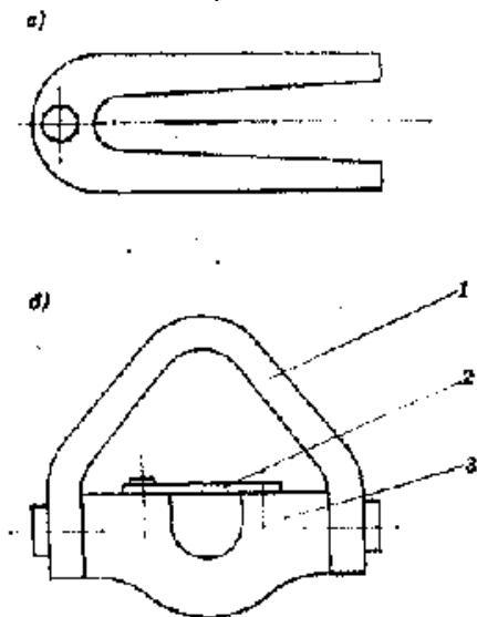
Рис. 27. Принадлежности для штанг: а — подкладная вилка; б — фарш-туль; 1 — серьга; 2 — щеколда; 3 — траверса
