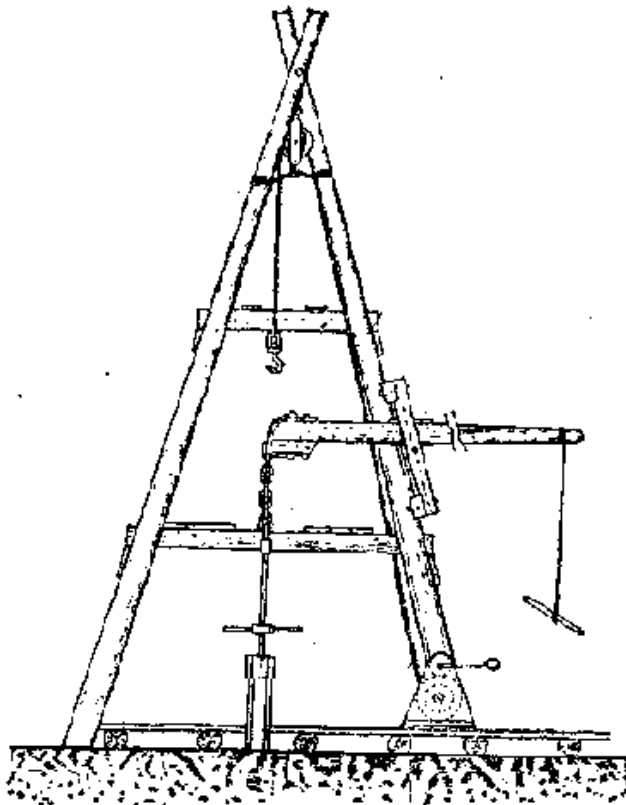
Рис. 29. Буровая вышка
