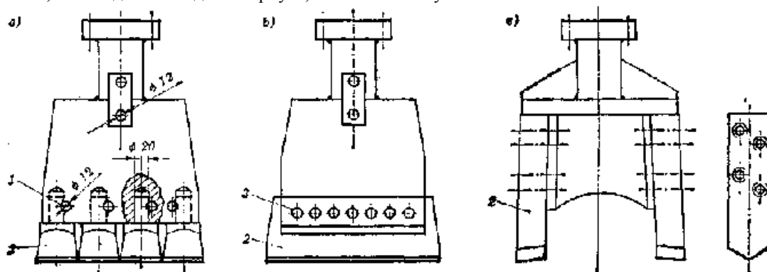
Рис. 23. Составные самодельные долота: 1 — клин; 2 — вставное лезвие; 3 — заклепка
