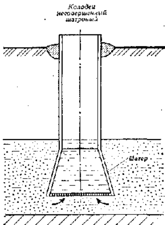
Рис. 3. Несовершенный шатровый колодец
