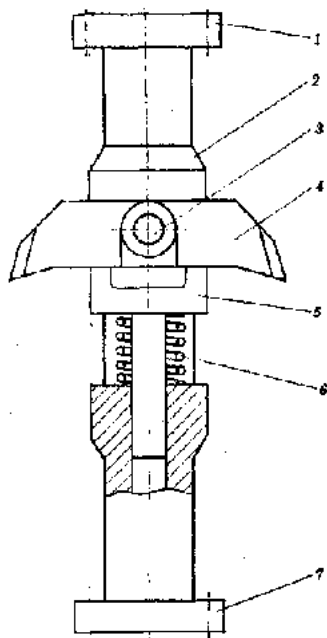
Рис. 37. Расширитель скважины: 1 — верхний фланец; 2 — корпус; 3 — ось; 4 — резец; 5 — гонд(лгд-ка; 6 — пружина; 7 — нижний фланец
