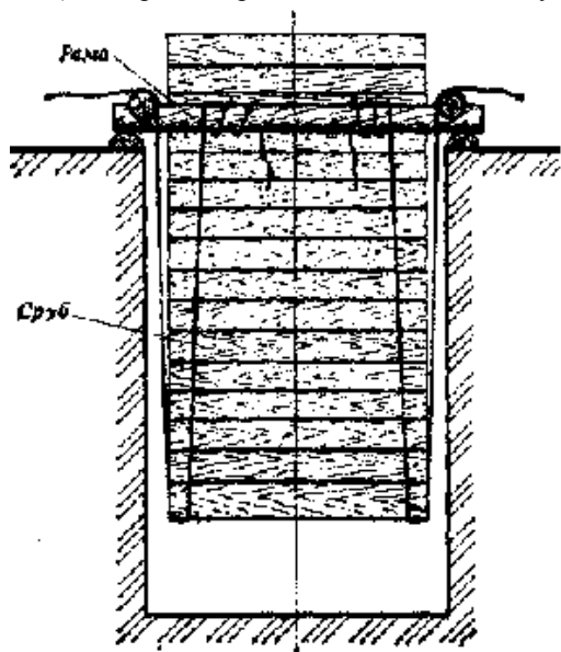
Рис. 5. Сруб, подвешенный в шахте на веревках
