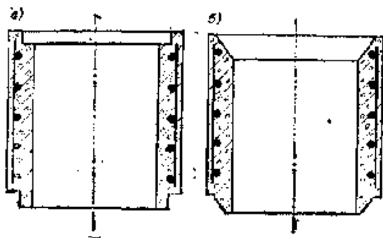
Рис. 11. Бетонные кольца, соединяемые в четверть (а) и в раструб (б)
