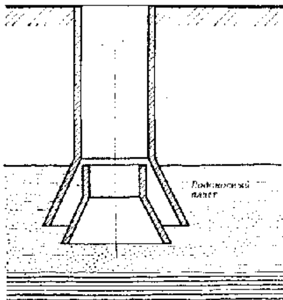
Рис. 9. Двойной шатер в водоприемной части
