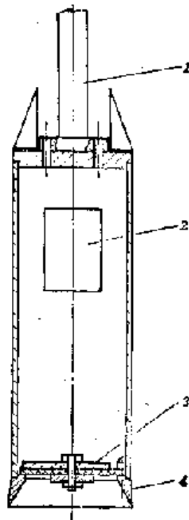
Рис. 25. Самодельная желонка: 1 — ударная штанга; 2 — окно; 3 — клапан; 4 — башмак
