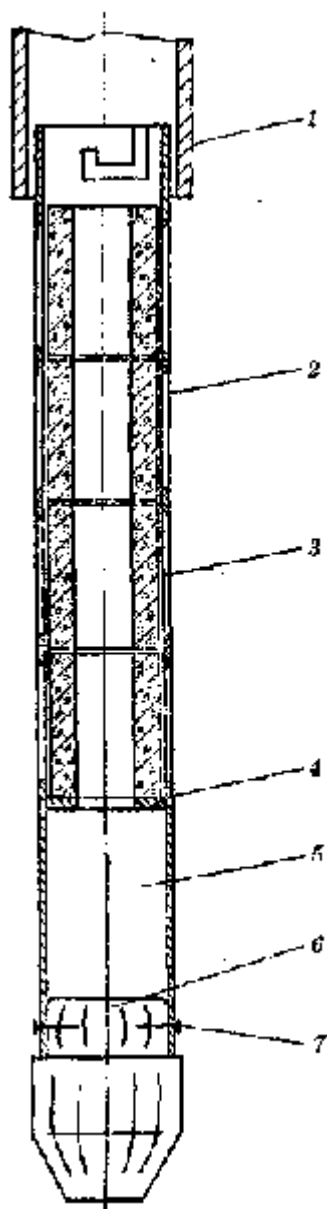
Рис. 40. Фильтр из крупнопористого бетона с наружным стальным каркасом: 1 — обсадная труба; 2 — фильтрующий блок; 3 — каркас с окнами; 4 — опора; 5 — оголтовник; 6 — пробка; 7 — гвоздь
