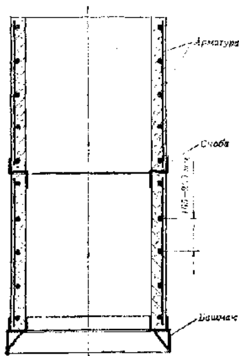
Рис. 10. Ствол (крепление) из бетонных колец впритык
