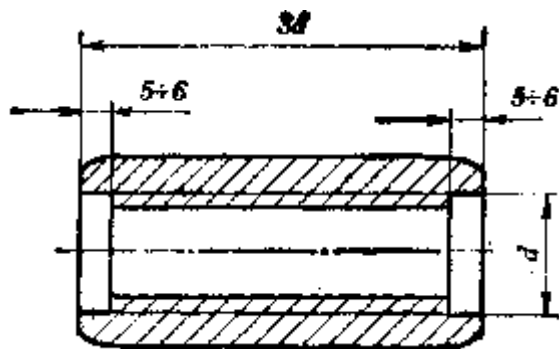
Рис. 26. Муфта
