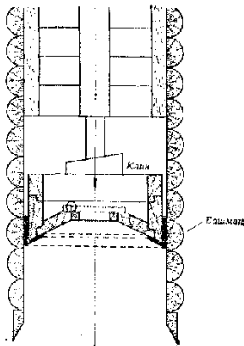
Рис. 7. Донный ящик
