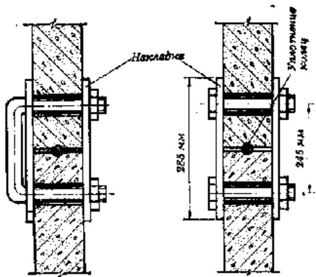
Рис. 12. Соединение бетонных колец скобами и болтами
