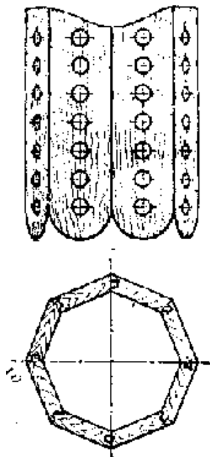
Рис. 32. Обсадная труба из досок
