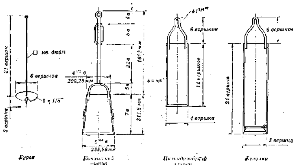
Рис. 31. Буровой снаряд Шитца
