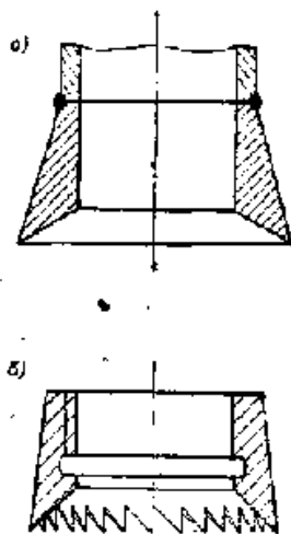
Рис. 38. Трубный башмак: а — гладкий; б — фрезер
