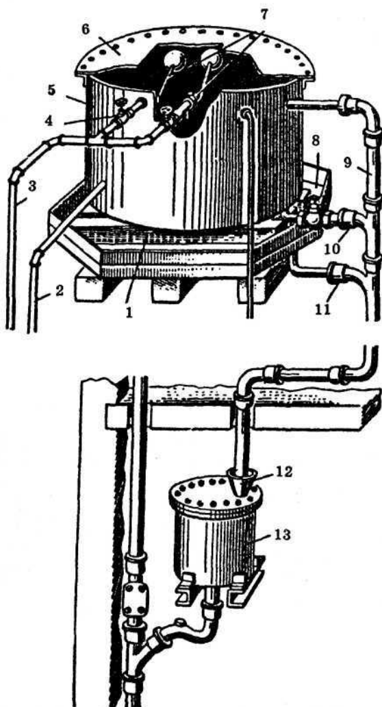
Рис. 4. Водонапорный бак:
