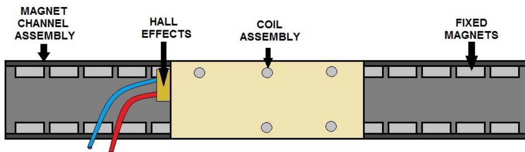
LINEAR MOTOR
