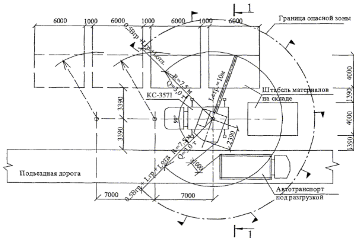
Рисунок 5 - Горизонтальная привязка крана КС-3571 (КС-3571А)
