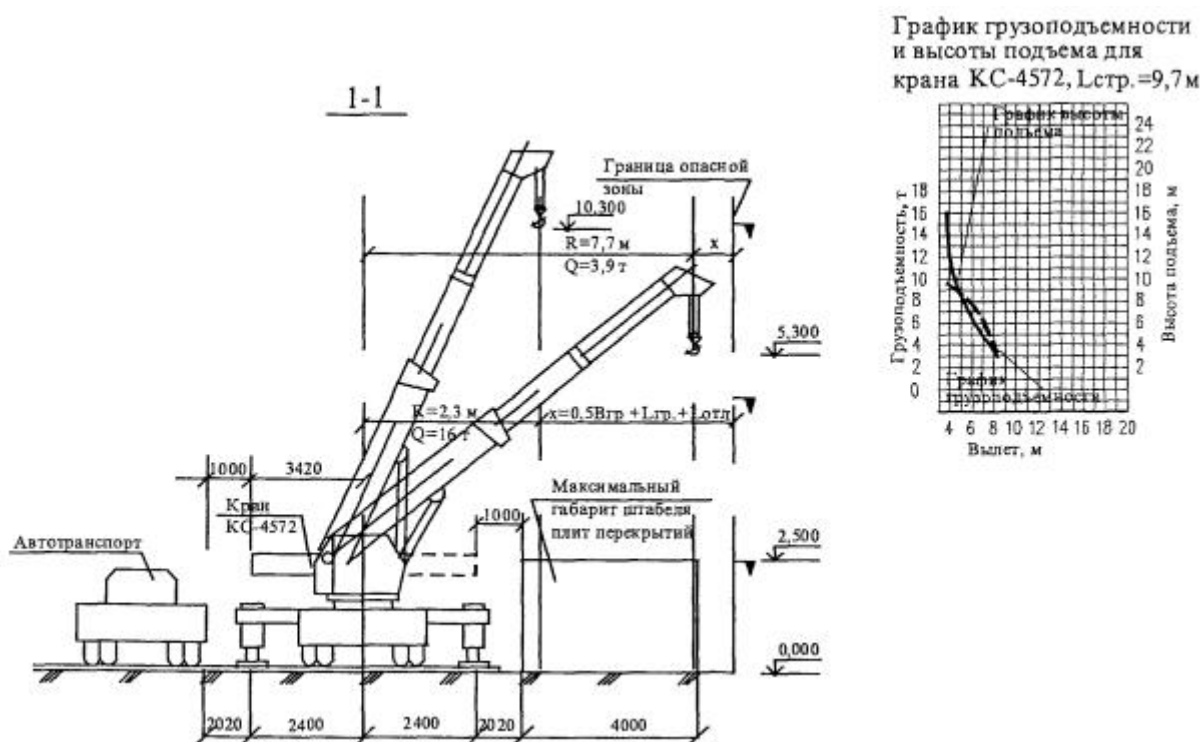
Рисунок 26 - Вертикальная привязка крана KC-4572 (KC-4572A, KC-4579)
