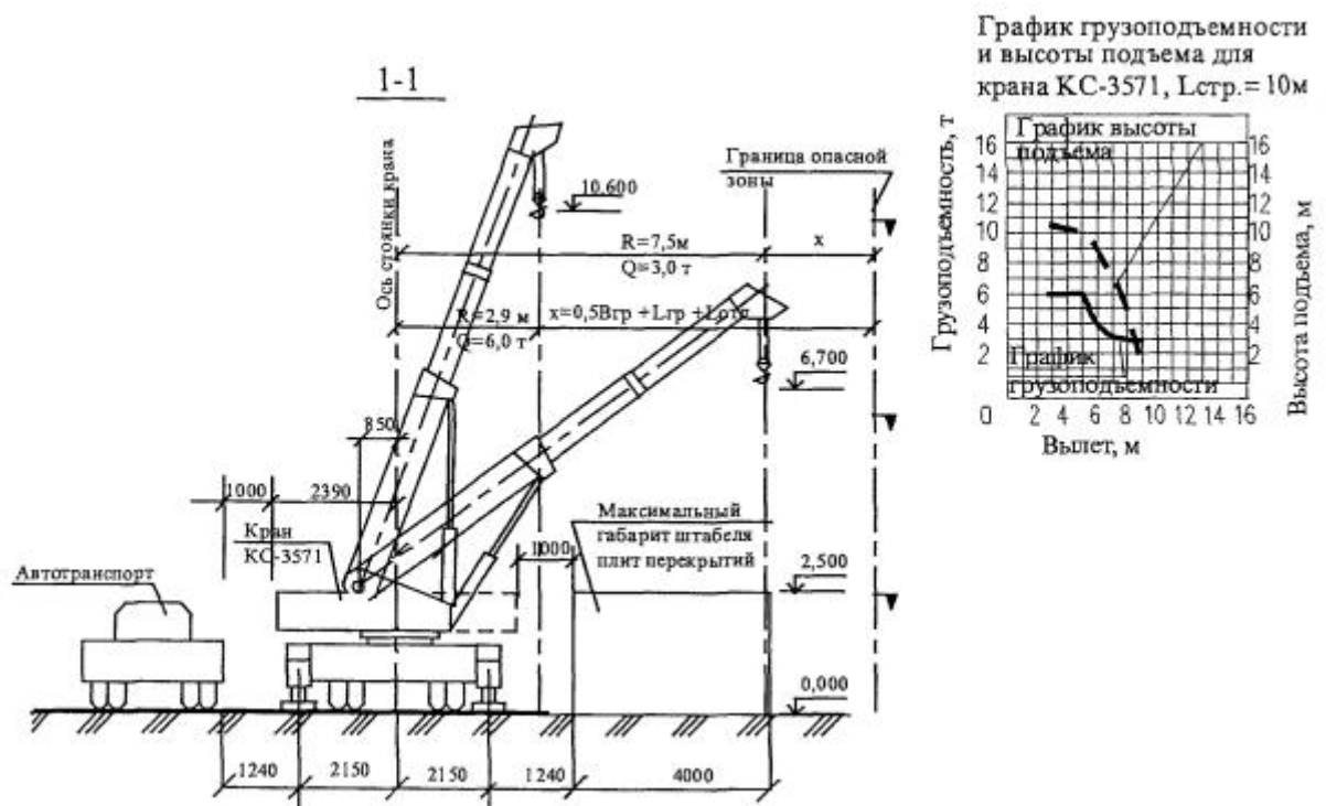
Рисунок 6 - Вертикальная привязка крана КС-3571 (КС-35714)
