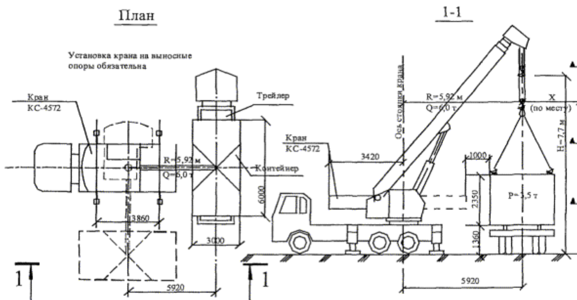
Рисунок 27 - Погрузка и разгрузка контейнеров массой до 5 т краном KC-4572
