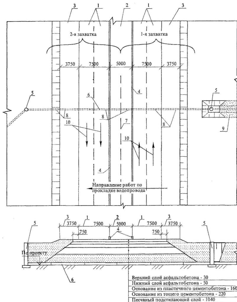
Рисунок 1 - Возможная схема перехода водопровода через проезжую часть автодороги
