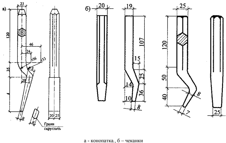
Рисунок 18 - Конопатки и чеканки.
