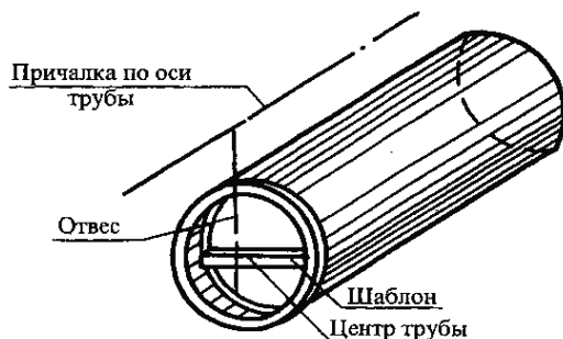
Рисунок 11 - Центровка труб со стороны раструба
