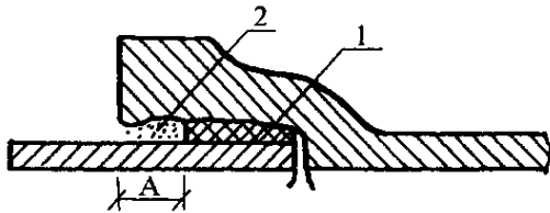
1 - уплотнение из пенковой пряди; 2 - асбестоцементный замок (размер А); А = 35 - 40 мм для труб диаметром 65 - 400 мм
