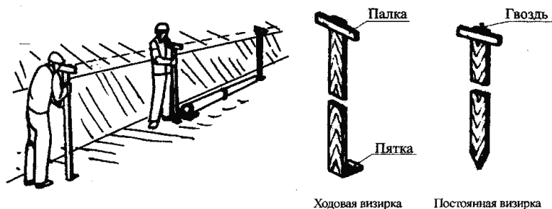
Рисунок 5 - Схема подготовки основания
