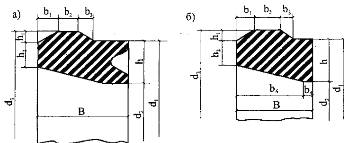
а - манжета с «ласточкин хвостом» Б-1 и Б-2 для труб по ТУ 14-3-1247-83; б - манжета укороченная 1-Б-1 и 1-Б-2 и универсальная облегченная БХ для труб по ТУ 14-3-1247-83
