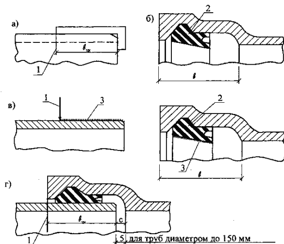
а - нанесение линии ограничения ввода цилиндрического конца трубы; б - установка манжеты в раструб; в - смазка наружной поверхности цилиндрического конца трубы и внутренней поверхности манжеты; г - смонтированный стык; l - линия ограничения ввода цилиндрического конца трубы; 2 - манжета; 3 - смазка; l_{цк} - длина цилиндрического конца трубы
