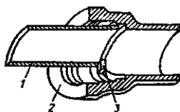
1 - гладкий конец трубы; 2 - раструб; 3 - вкладыш-ограничитель.
