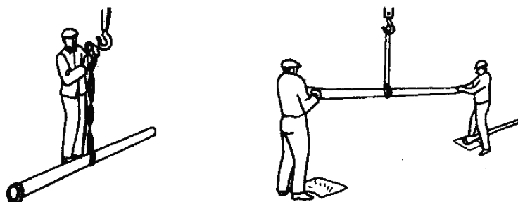
Рисунок 7 - Строповка труб и опускание в траншею
