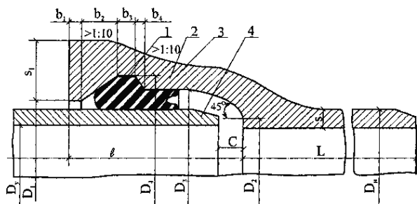
1 - трапециевидный кольцевой паз; 2 - раструб; 3 - резиновая уплотнительная манжета; 4 - гладкий конец с фаской
