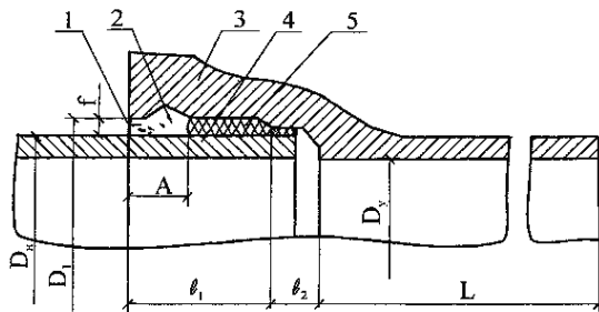
Рисунок 3 - Раструбное стыковое соединение чугунных напорных труб (ГОСТ 9583-75*) с устройством замка
