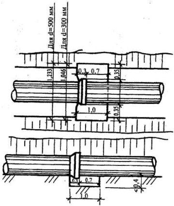
Рисунок 4 - Схема организации приямков
