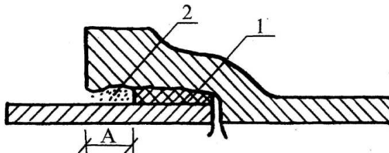
1 - уплотнение из пенковой пряди; 2 - асбестоцементный замок (размер А);
