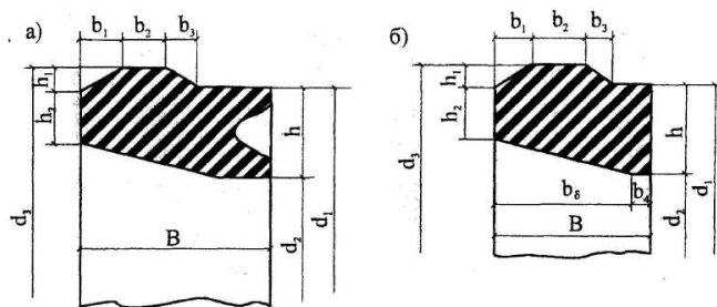
а - манжета с «ласточкиным хвостом» Б-1 и Б-2 для труб по ТУ 14-3-1247-83; б - манжета укороченная 1-Б-1 и 1-Б-2 и универсальная облегченная БХ для труб по ТУ 14-3-1247-83
