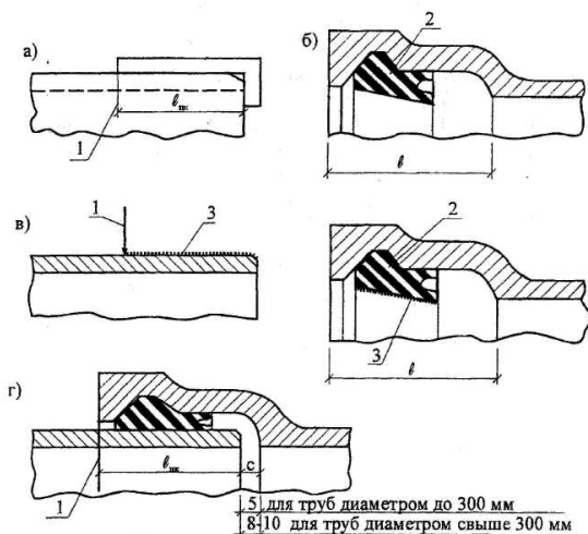
а - нанесение линии ограничения ввода цилиндрического конца трубы; б - установка манжеты в раструб; в - смазка наружной поверхности цилиндрического конца трубы и внутренней поверхности манжеты; г - смонтированный стык;
