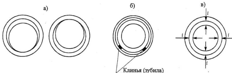
а) положение трубы в раструбе до центрирования; б) подкладка зубил для центрирования; в) конечное положение трубы в раструбе при правильном центрировании, i - величина кольцевого зазора
