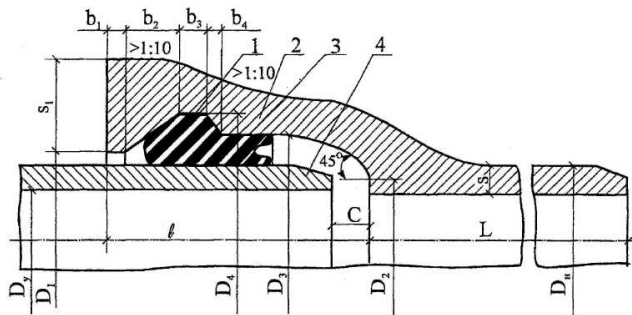
1 - трапециевидный кольцевой паз; 2 - раструб; 3 - резиновая уплотнительная манжета; 4 - гладкий конец с фаской Рисунок 1 - Раструбное соединение чугунных напорных труб (ТУ 14-3-1247-83) без устройства замка
