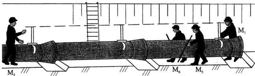
Рисунок 12 - Схема проверки правильности укладки трубы
