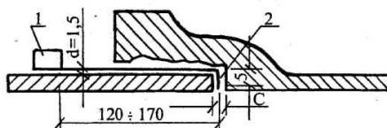
1 - проволочный щуп, 2 - зазор между торцами стыкуемых труб (размер С)
