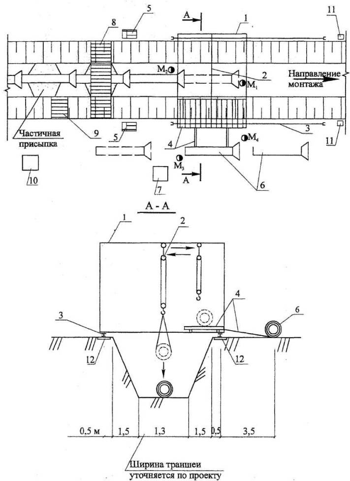
1 - металлическая рама; 2 - электродаль; 3 - рельсы; 4 - лежни с площадкой; 5 - электролебедка; 6 - чугунные трубы; 7 - ящик для цементного раствора; 8 - инвентарный переходный мостик; 9 - инвентарная лестница; 10 - передвижная электростанция; 11 - блок; 12 - полупалпы ○ - рабочее место монтажников
