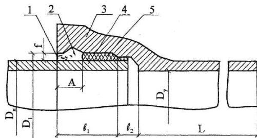
1 - битумная мастика; 2 - асбестоцементный замок глубиной А; 3 - раструб; 4 - гладкий конец трубы; 5 - уплотнительная пряжа. Рисунок 3 - Раструбное стыковое соединение чугунных напорных труб (ГОСТ 9583-75*) с устройством замка
