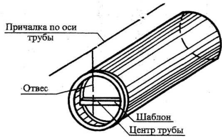
Рисунок 9 - Центровка труб со стороны раструба
