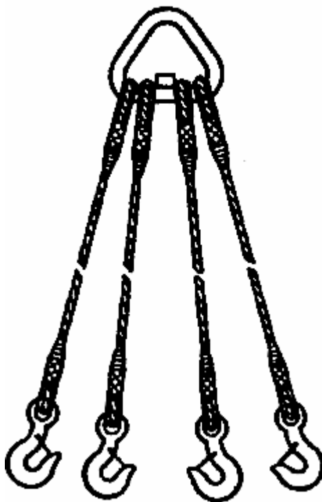
Рис.39. Четырехветевой 4СК1
