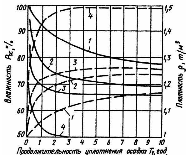
Рис. 2. Средние значения влажности и плотности осадка станций обезжелезивания или реагентного умягчения воды при многолетнем уплотнении
