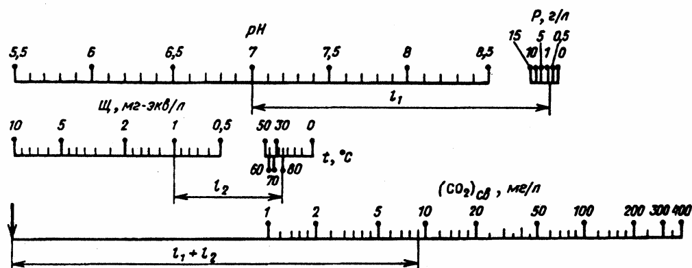
Рис. 2. Номограмма для определения концентрации свободной двуокиси углерода в природной воде (или pH)
