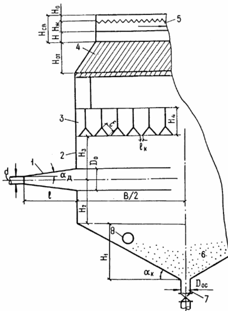
Черт. 35. Тонкослойный осветитель системы АзНИИВП-2
