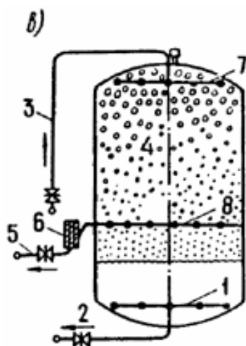
Черт. 30. Фильтры с плавающей пенополистирольной загрузкой
