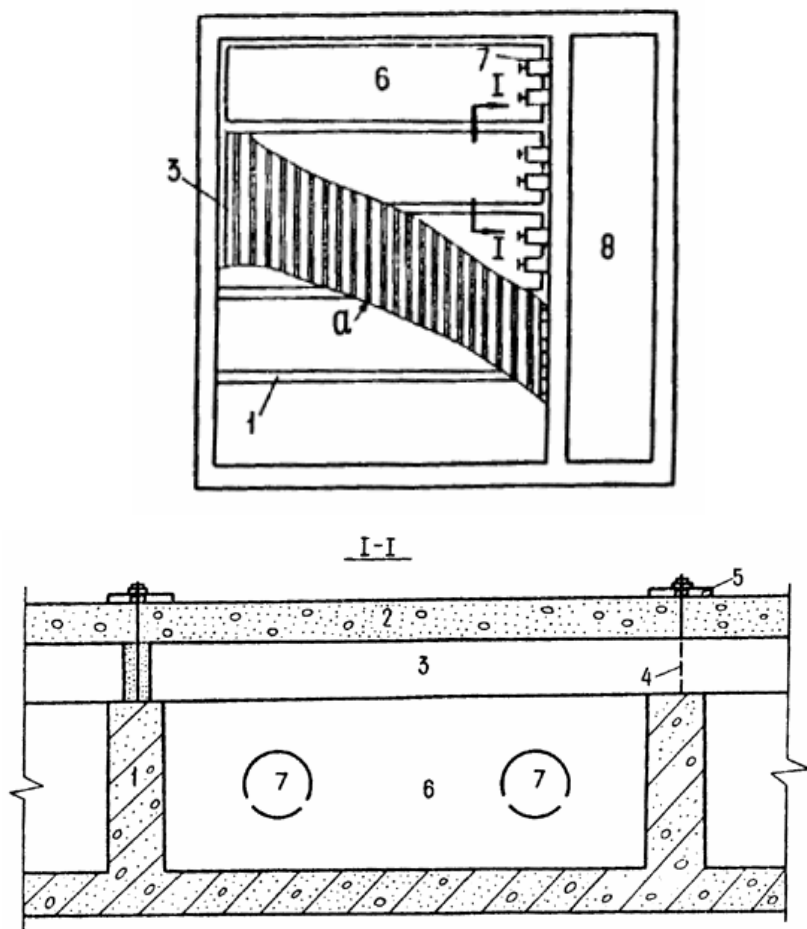
ерт. 29. Дренаж из монолитного полимербетона
