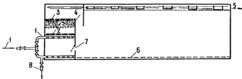
Черт. 11. Горизонтальный отстойник с контактной камерой хлопьеобразования
