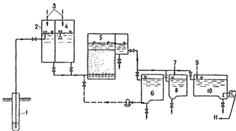
Черт. 41. Принципиальная схема работы станции обесфторивания воды
