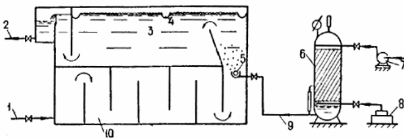
Черт. 18. Флотационная установка
