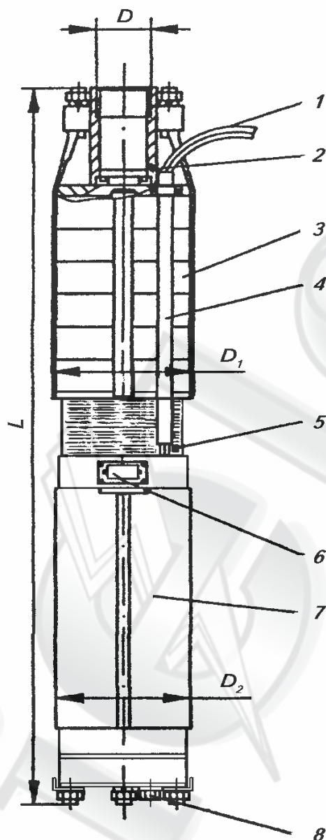
Рис. 16. Общий вид электронасоса ЭЦВ
