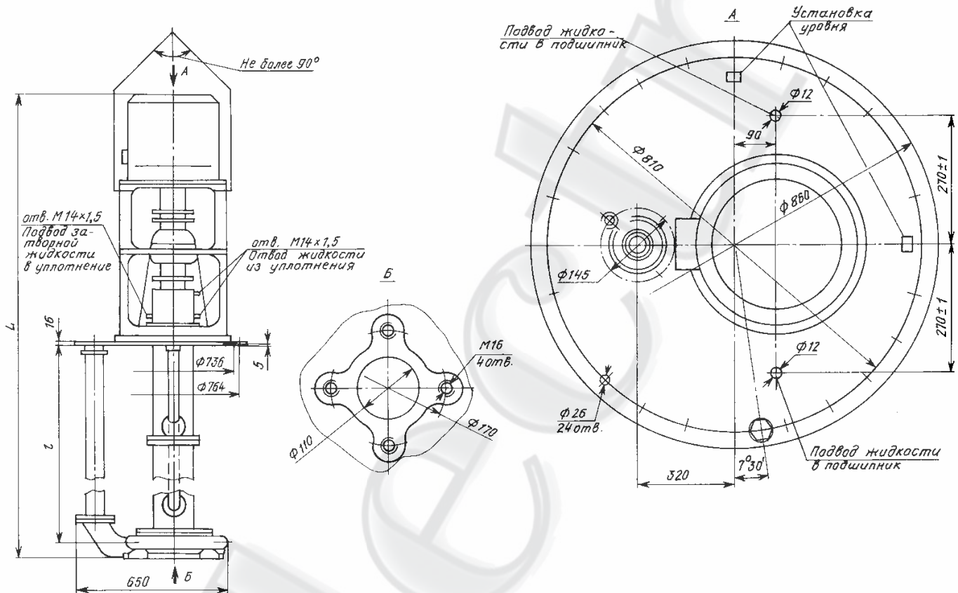
Рис. 1. Габаритные, установочные размеры и схема подвода затворной жидкости в уплотнение вала и подшипники, масса насоса 1НВ50/50 и электродвигателей для различных вариантов глубины погружения
