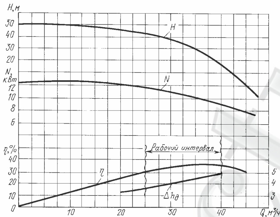
Рис. 4. Характеристика электронасоса 1CBH-80A
