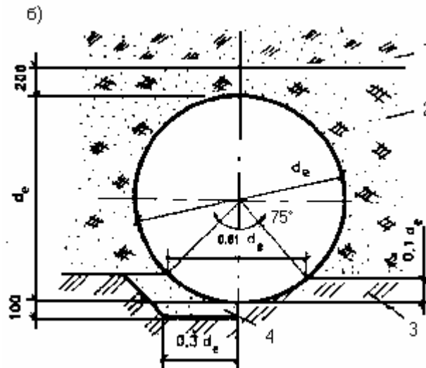
Рис. 1. Способы опирания труб на основание а - плоское грунтовое основание; б- профилированное грунтовое основание с углом охвата 75°; I - с песчаной подушкой; II - без песчаной подушки; 1 - засыпка местным грунтом без уплотнения; 2 - засыпка местным грунтом с нормальной или повышенной степенью уплотнения; 3 - естественный грунт; 4 - подушка из песчаного грунта
