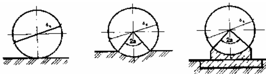
Рис. 2. Способы опирания трубопроводов a - на плоское грунтовое основание; б - на грунтовое профилированное основание с углом охвата 2\alpha ; в - на бетонный фундамент
