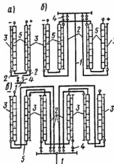
Рис. 5. Схема ввода электролитов в коллекторы электролизной установки, обладающая минимальными токами утечки a, б, в — схемы с двумя, четырьмя и шестью рядами электролизеров соответственно; 1 — труба ввода электролита в цех; 2 — труба ввода электролита в коллектор; 3 — рядовой коллектор электролита; 4 — вентиль; 5 — электролизеры
