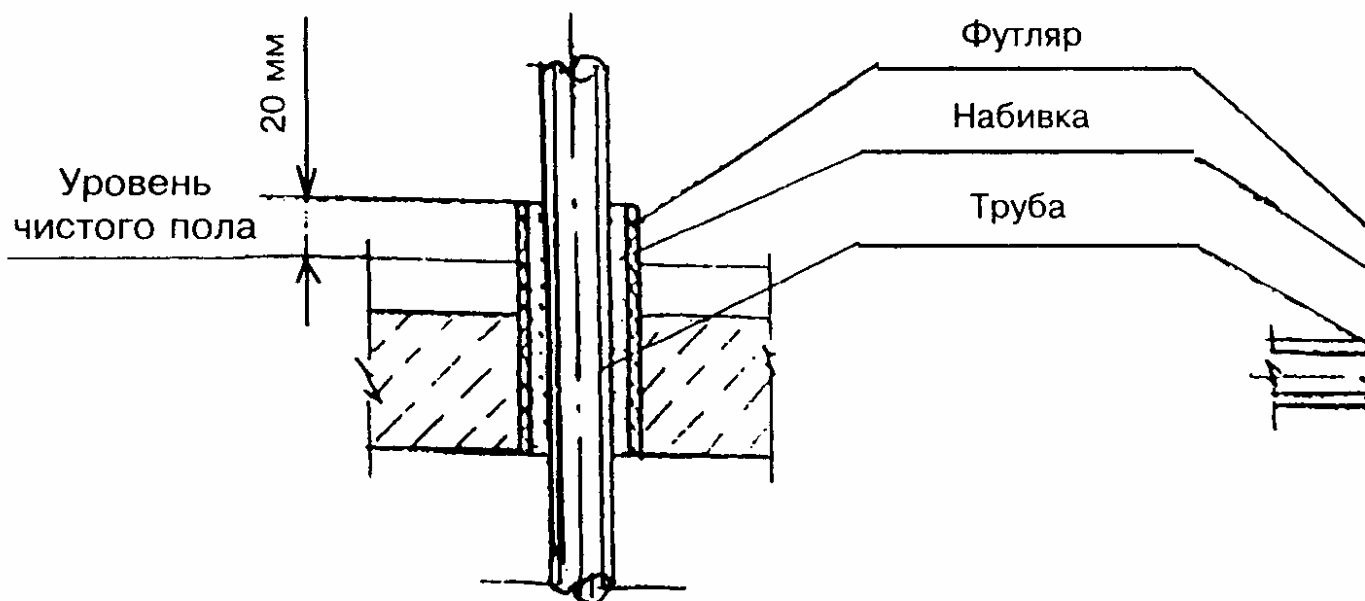
Рисунок 6 — Установка футляров для прохода труб через перекрытия
