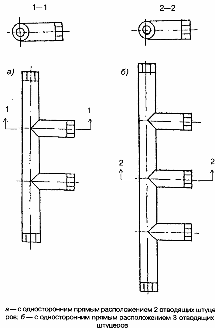
Рисунок 1 — Стальной распределительный коллектор
