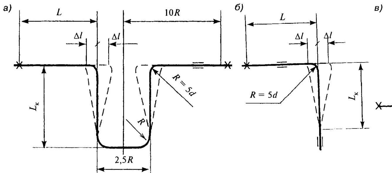
Рисунок 5 — Устройство компенсаторов П-образного (а), Г-образного (б), петлеобразного (в), п
