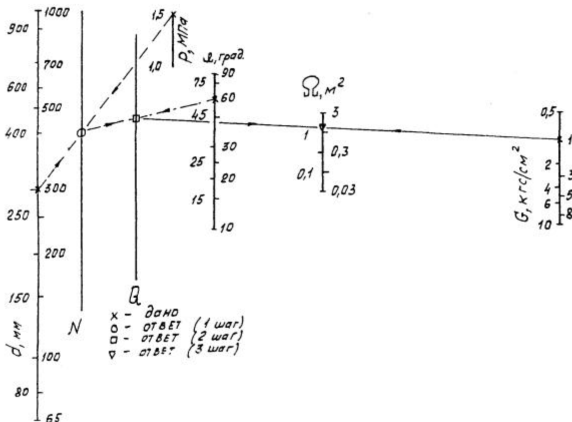
Рисунок В.1 - Номограмма для выбора опорной площади упоров W на трубопроводе водоснабжения диаметром d из труб из высокопрочного чугуна с шаровидным графитом с раструбными соединениями, находящемся под внутренним давлением p , при угле поворота трассы \alpha с опорой на грунт прочностью G
