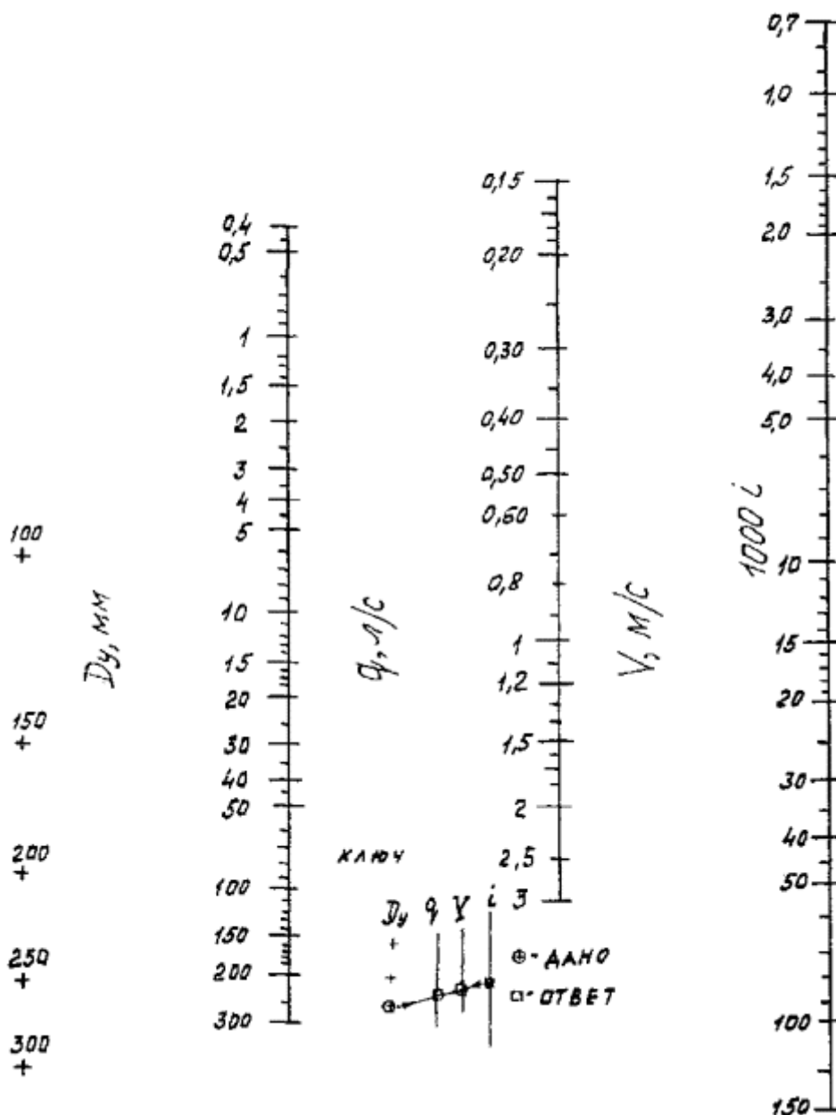
Рисунок А.1 - Номограмма расчета труб с внутренним цементно-песчаным покрытием
