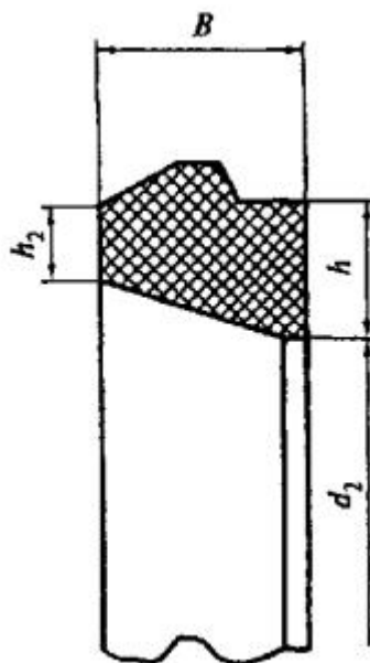
Рисунок 5 - Резиновое кольцо (размеры по таблице 8 )
