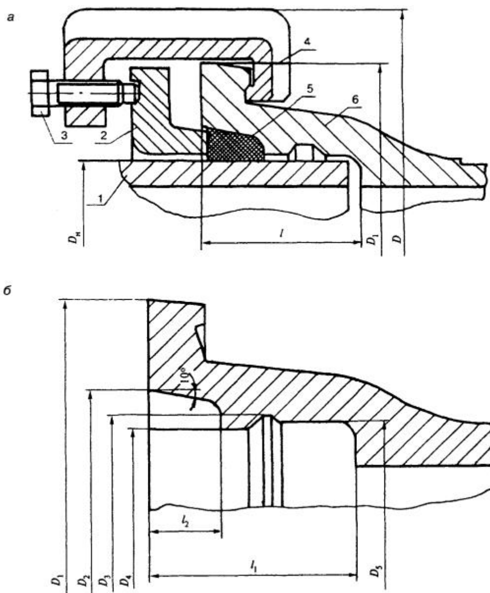
а - раструбное соединение; б - раструб трубы с резиновым кольцом
