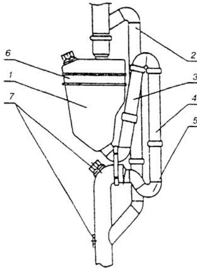
1 - емкость; 2 - вентиляционный стояк; 3 - подъемная труба; 4 - вакуумная труба; 5 - гидрозатвор; 6 - крепёжная лента; 7 - прочистка
