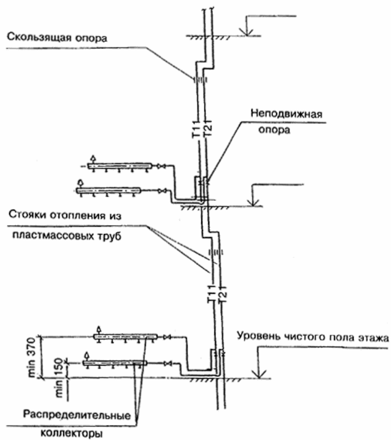
Рисунок 8 - Вариант подсоединения распределительных коллекторов к стоякам из металлополимерных труб
