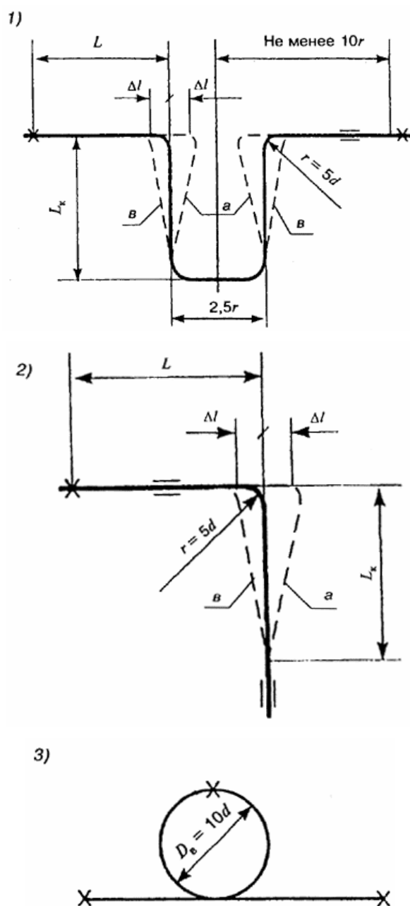
Рисунок 10 - Диаграмма для определения удлинения труб
