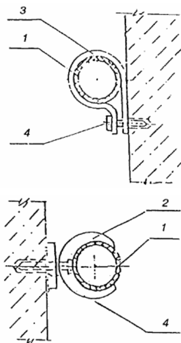
1 - труба; 2 - фиксатор; 3 - хомут; 4 - шуруп (дюбель)
