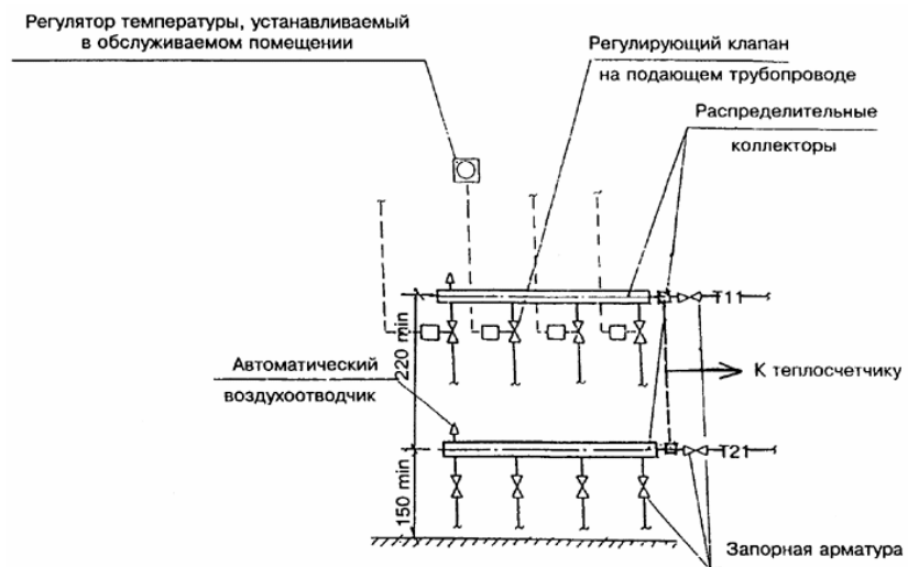
Рисунок 7 - Распределительный коллектор системы отопления
