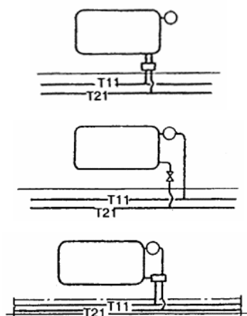
Рисунок 5 - Узлы подсоединения отопительных приборов к двухтрубной системе отопления
