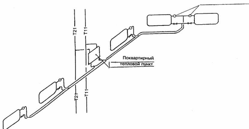
Рисунок 4 - Система отопления с горизонтальными двухтрубными ветками для группы параллельно-последовательно соединенных отопительных приборов
