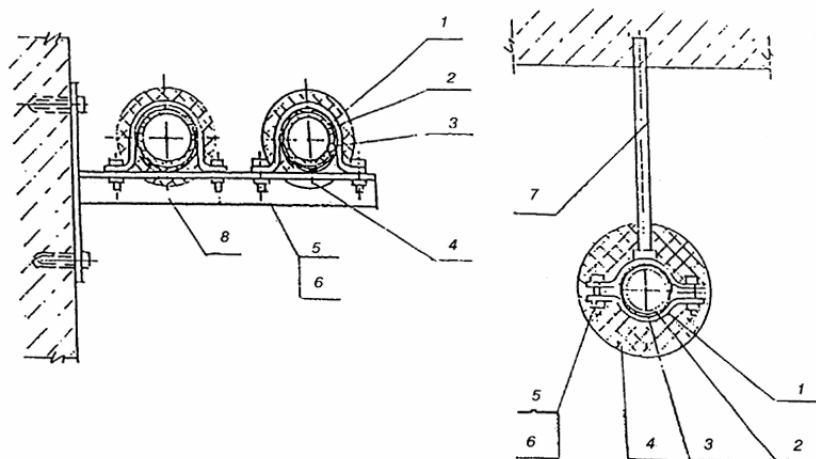
Рисунок 17 - Крепление труб к стенам и перегородкам
