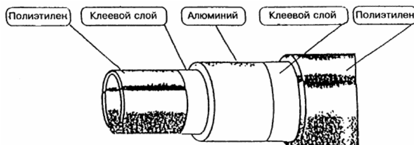
Рисунок 1 - Структура металлополимерной трубы
