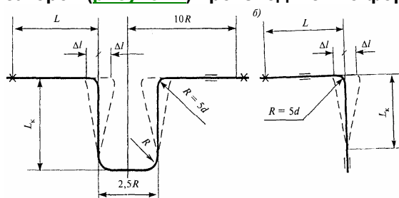
Рисунок 1 — Устройство П-образного (а) и Г-образного (б) компенсаторов
