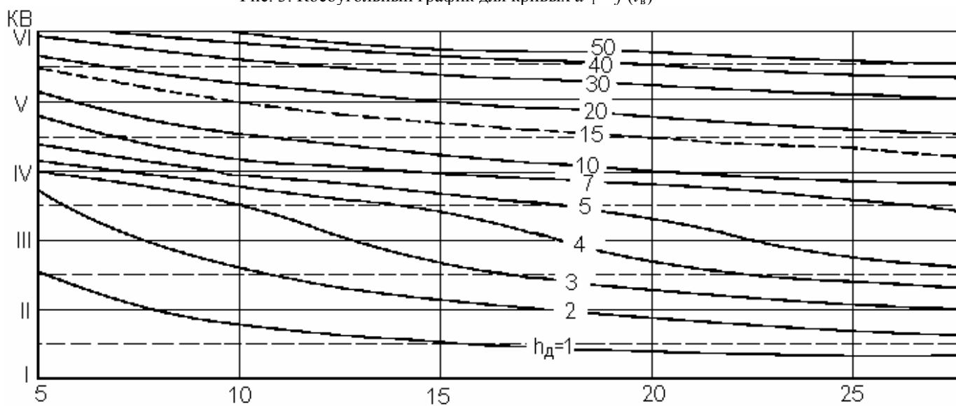
Рис. 4. График для определения категории впитывания почвы (KB) по опытам с дождеванием
