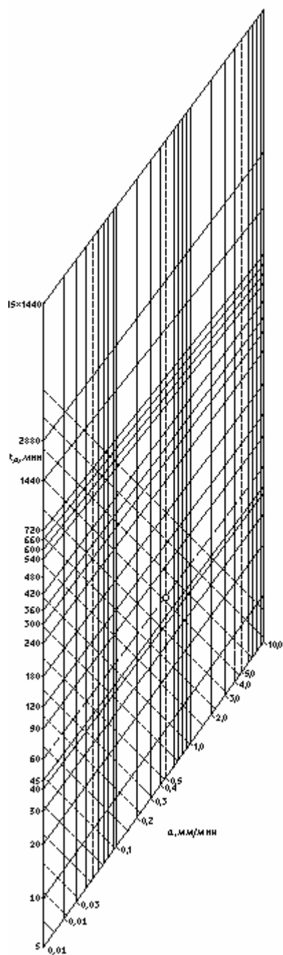
Рис. 3. Косоугольный график для кривых a_1 = f(t_v)
