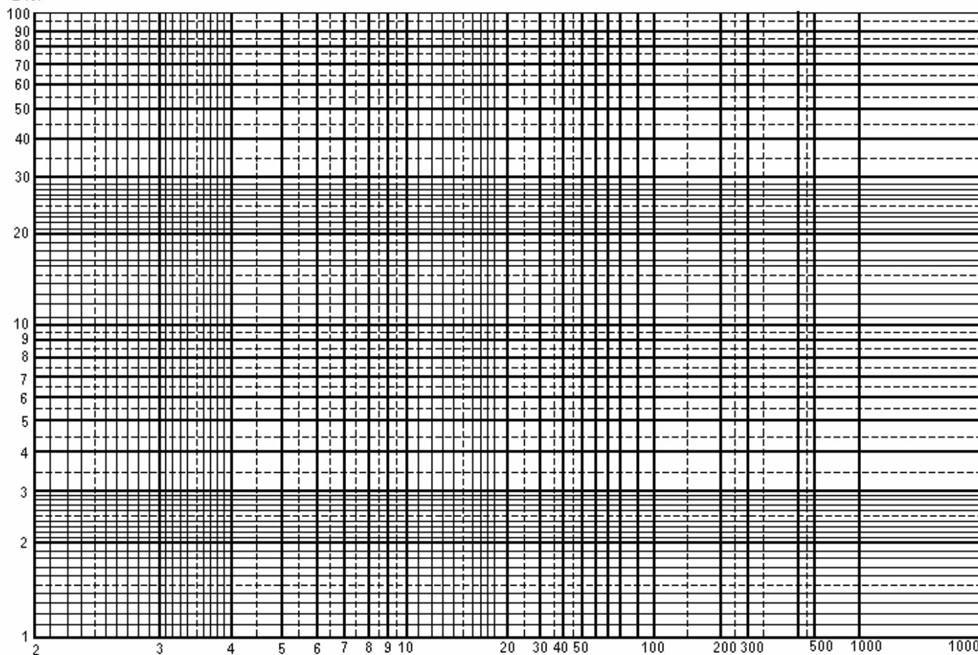
Рис. 7. Спрямяющая клетчатка для распределения суточного максимума осадков
