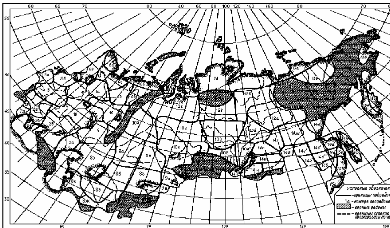
Рис. 1. Схема ливневых подрайонов – границы подрайонов; – границы стока по промерзшей почве; – горные районы. Цифры с буквами – номера подрайонов
