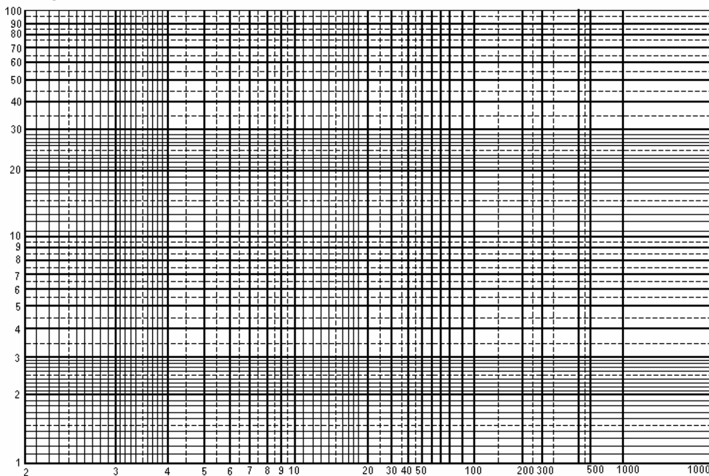
Рис. 5. Спрямяющая клетчатка для распределения пятиминутных и максимальных интенсивностей осадков
