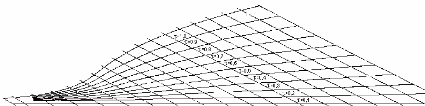
Рис. 6. Типовые лекала для кривых a_d = f(t_d)
