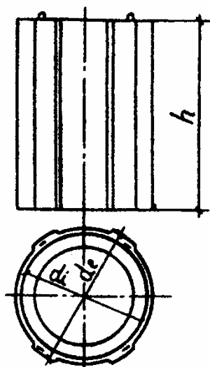
"Рабочая камера типа КВГ"
