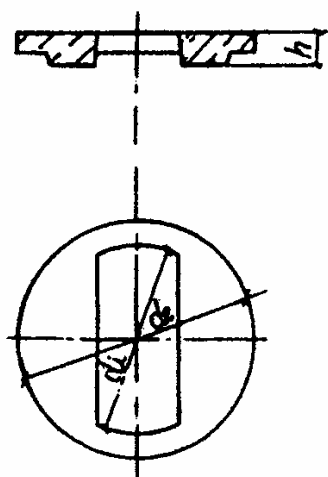
"Плита перекрытия для водоприемных колодцев"
