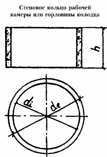
"Стеновое кольцо рабочей камеры или горловины колодца"
