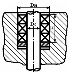
Узел сальника
