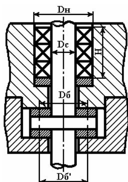
Узел сальника
