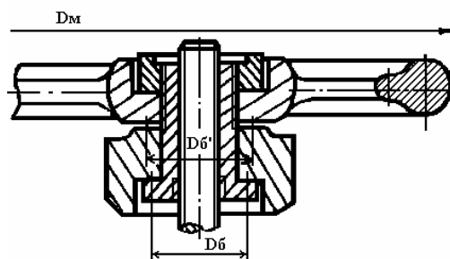
Узел резьбовой втулки
