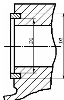
Уплотняющее кольцо корпуса
