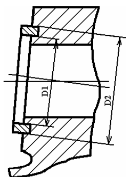
Рисунок В.1 – Схемы задвижки и ее расчетных узлов
