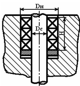
Узел сальника
