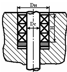
Узел сальника
