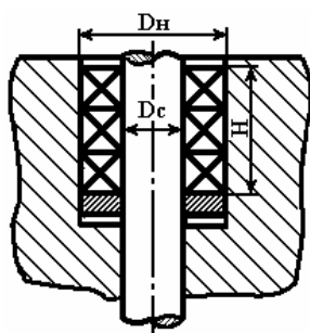
Узел сальника
