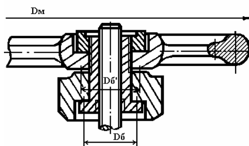
Узел резьбовой втулки
