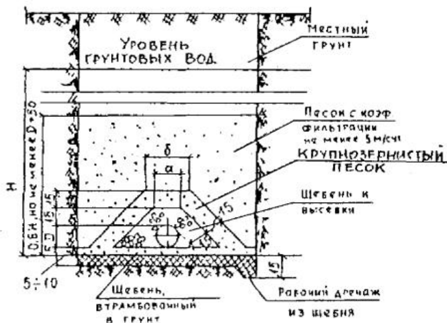
Рис. 1 Дренаж совершенного типа
