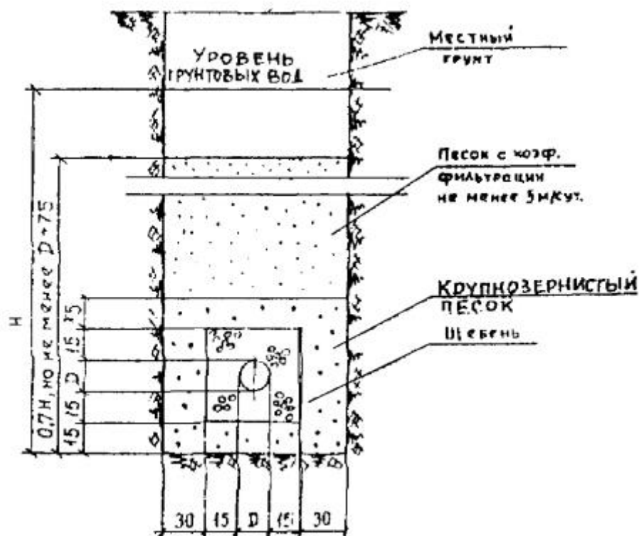
Рис. 2 Дренаж несовершенного типа
