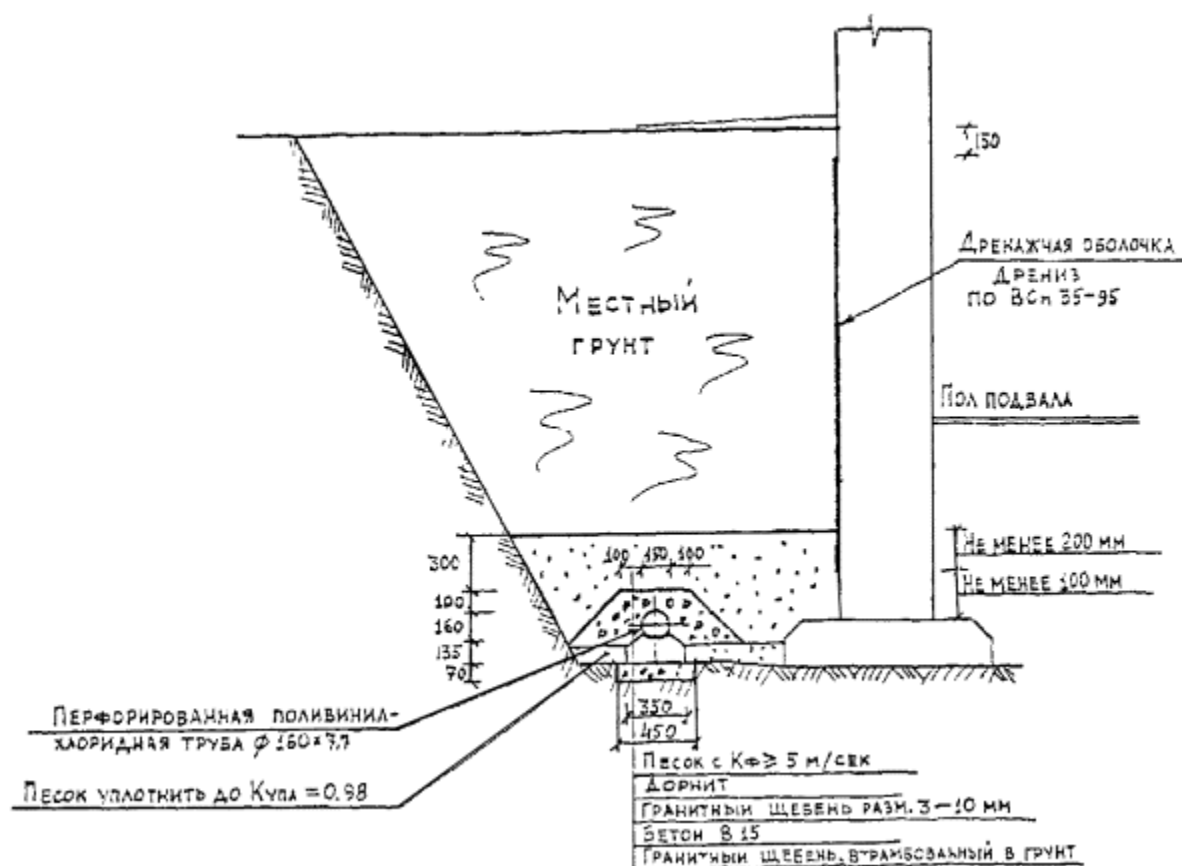
Рис. 14 Пристенный дренаж с применением поливинилхлоридных труб на бетонном основании и дренажной оболочки «Дрениз»
