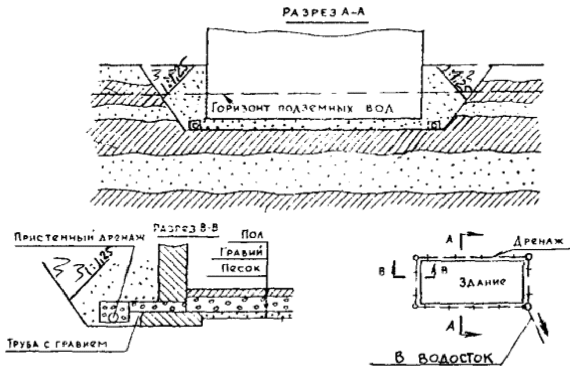
Рис. 9 Схема пластового дренажа
