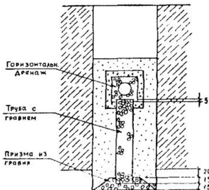
Рис. 5 Комбинированный дренаж с вертикальным самоизливающимся колодцем
