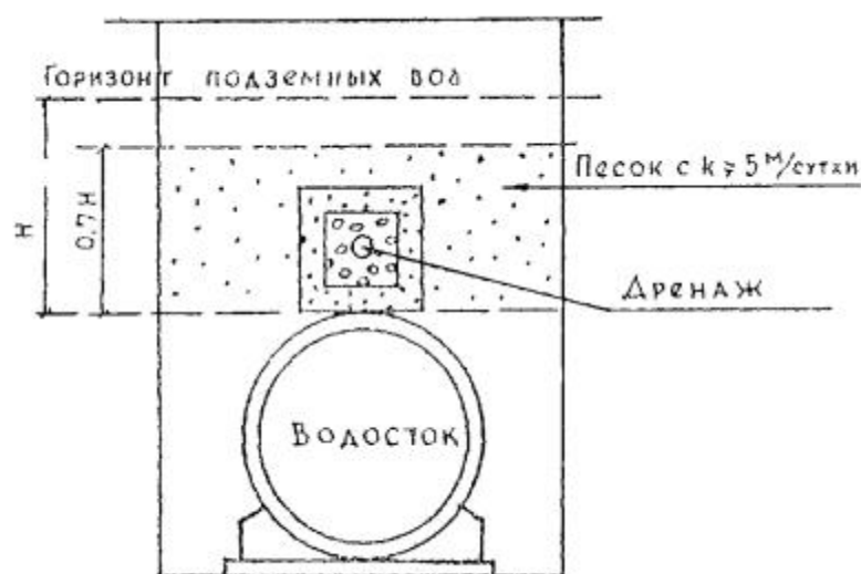
Рис. 10 Схема прокладки дренажа над водосток
