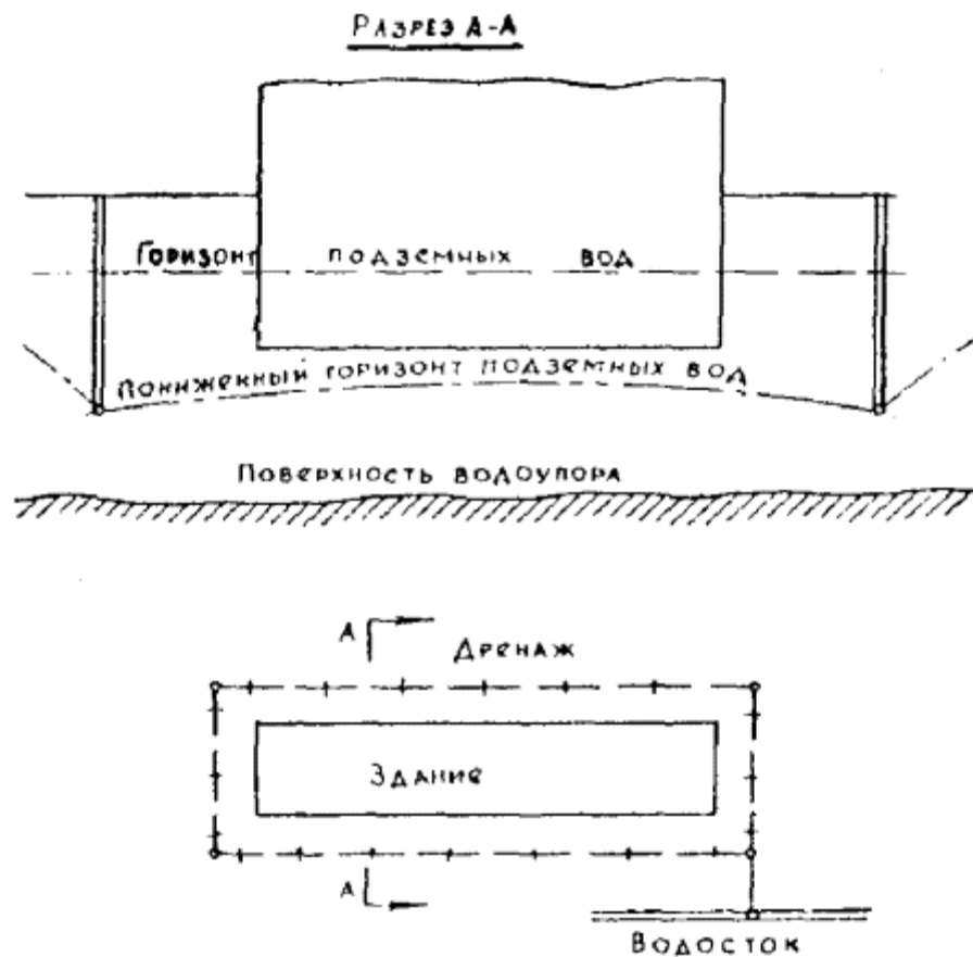
Рис. 8 Схема кольцевого дренажа
