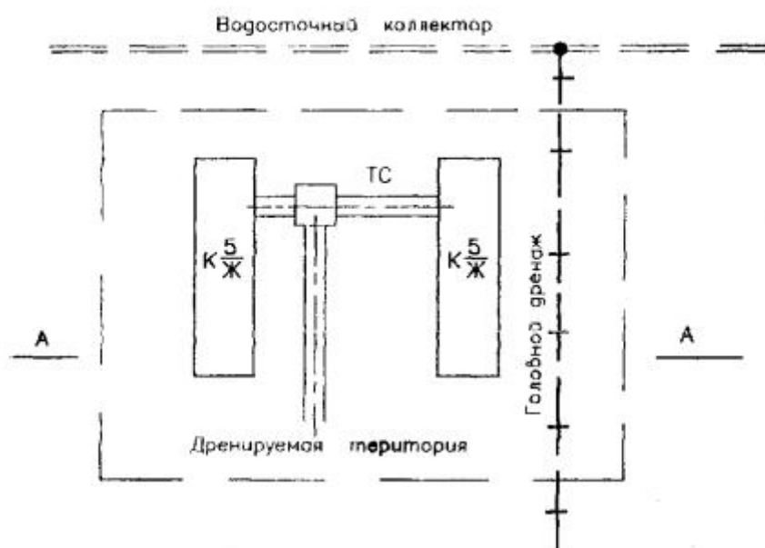
Рис. 3 Схема головного дренажа
