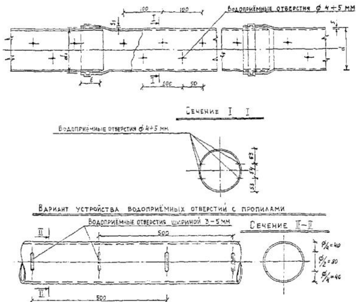
Рис. 12 Труба поливинилхлоридная с водоприемными отверстиями и с заделкой стыков
