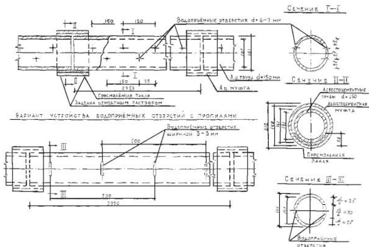
Рис. 11 Труба асбестоцементная с водоприемными отверстиями и с заделкой стыков
