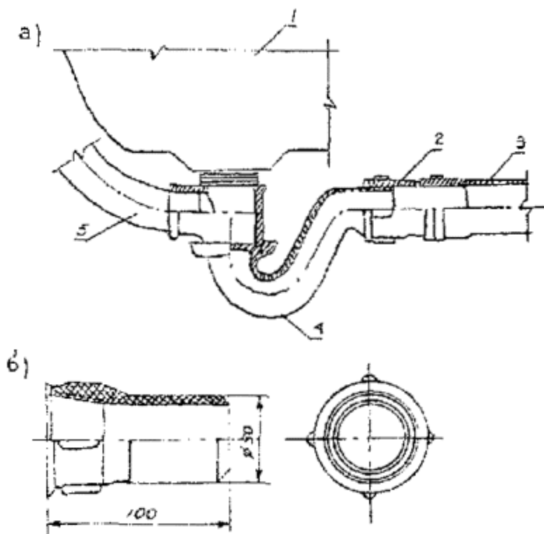
Рис. 7. Узел соединения (а) ванны с отводным трубопроводом из ПВХ:
