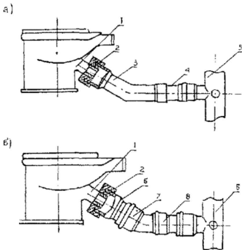
Рис. 4. Резиновая манжета для подсоединения сифона
