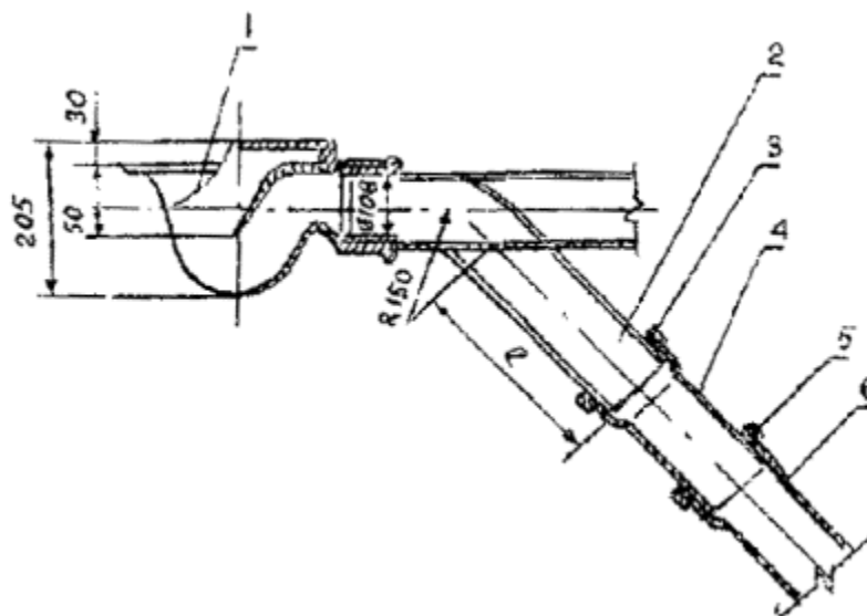
Рис. 8. Узел соединения чугунного эмалированного трапа с трубами из ПВХ:
