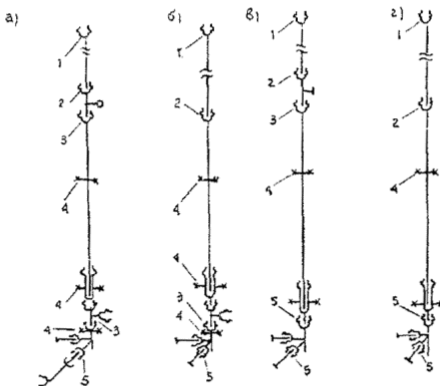
Рис. 13. Монтажные схемы (а, б, в, г) канализационных стояков:
