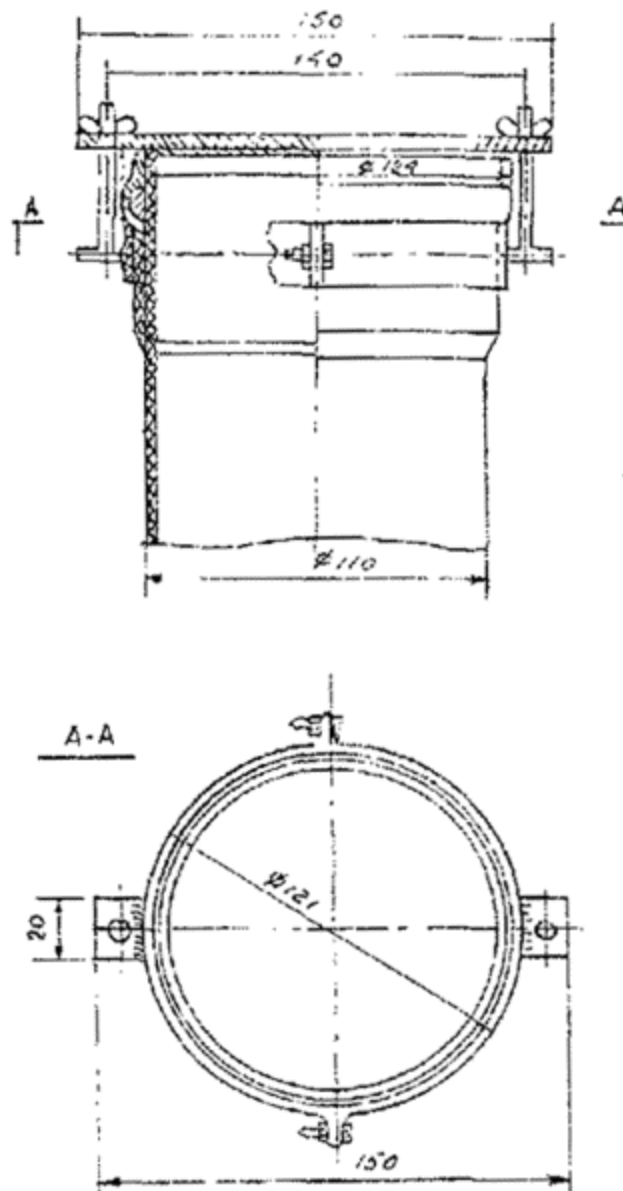
Рис. 16. Фиксатор для крепления заглушек в раструбах патрубков или фасонных частей из ПВХ
