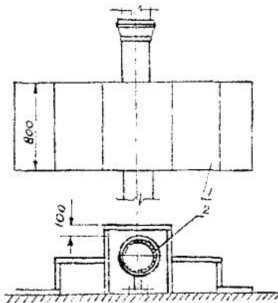
Рис. 17. Узел пересечения трассы из ПВХ с переходным мостиком:
