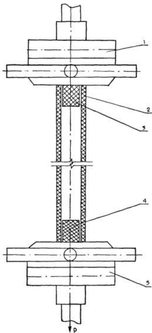
Рис 6. Схема испытаний трубного образца на растяжение:
