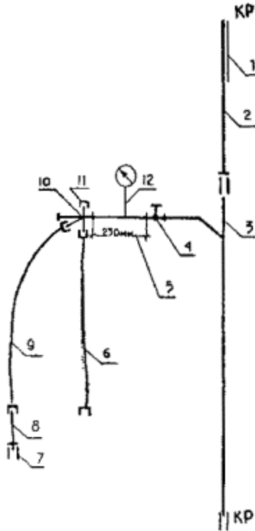
Рис. 1 (а, б, в). Схема коллекторной системы холодного водопровода с водосчетчиком, с поквартирным запорно-распределительным краном и полиэтиленовыми подводками к санитарным приборам в санитарно-технических кабинах:
