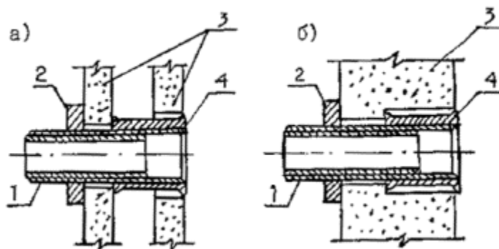
Рис. 5. Конструкция узла для подсоединения полиэтиленовой подводки к настенному смесителю ванны для санитарно-технических кабин из асбестоцемента (а) и гипсобетона (б):
