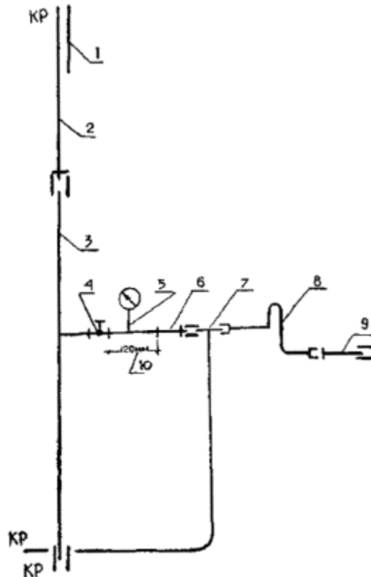
Рис. 2. Схема водопровода горячего водоснабжения со счетчиком расхода воды и с медной подводкой к смесителю каины и умывальника (марка кабины 1К-1М):
