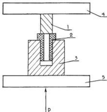
Рис. 8. Схема испытаний прочности наплавливаемых буртов на сдвиг:
