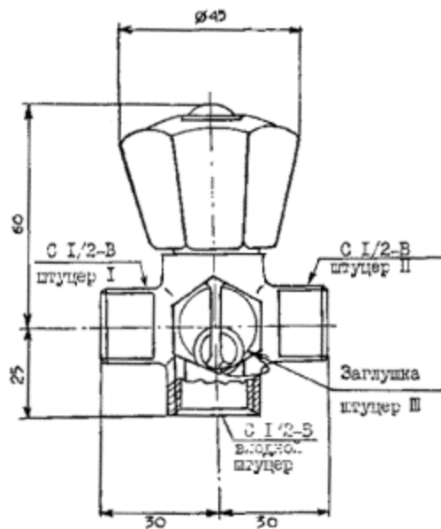
Рис. 3. Латунный запорно-распределительный кран (КЗР)
