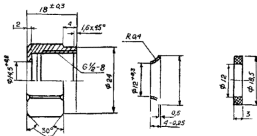
Рис. 4. Конструкция полиэтиленовой водопроводной подводки с наплавляемыми буртами: а) конец подводки с наплавленным буртом; б) накладная гайка из латуни и детали соединений:
