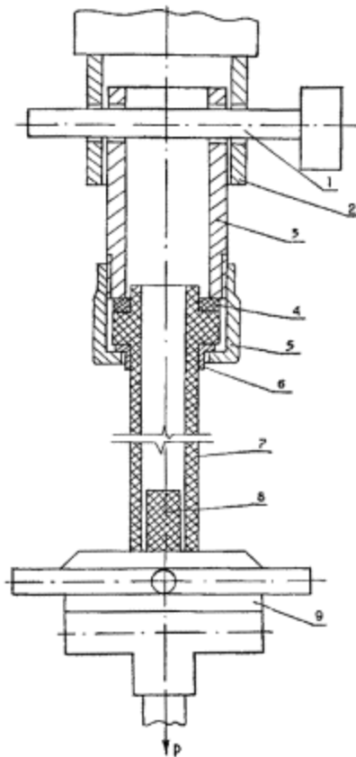
Рис. 7. Схема испытаний при определении прочности соединения полиэтиленовой трубы с наплавляемым буртом:
