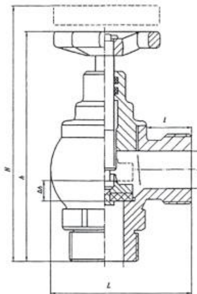
Рисунок 1. Клапан пожарного крана
